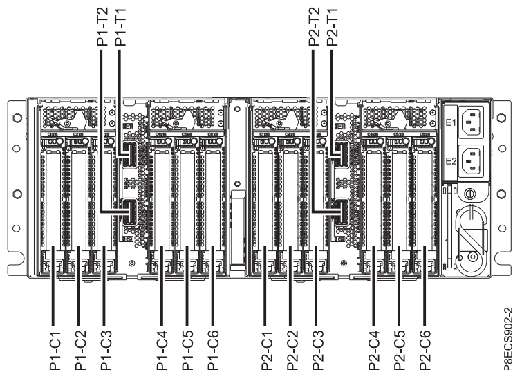
図 1. PCIe スロットのロケーション・コード付きの EMX0 PCIe3 拡張ドロワーの背面図
