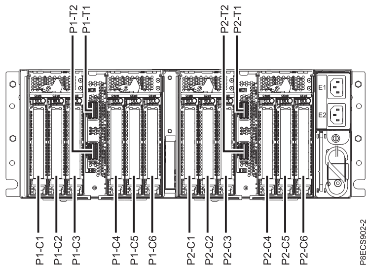
図 2. PCIe スロットのロケーション・コード付きの EMX0 PCIe3 拡張ドロワーの背面図
