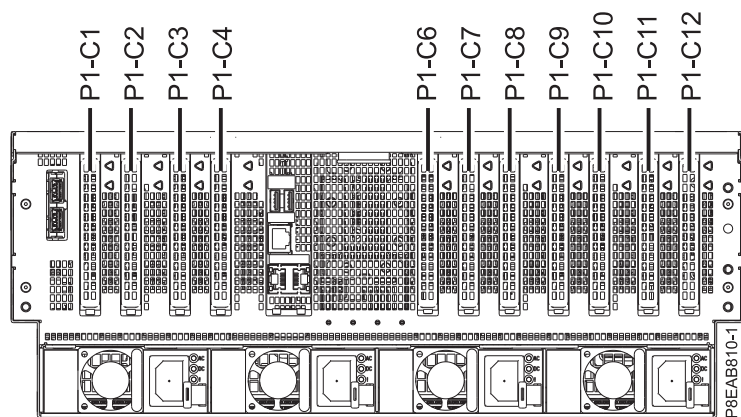
図 1. PCIe スロットのロケーション・コード付きの 8408-44E または 8408-E8E システムの背面図
