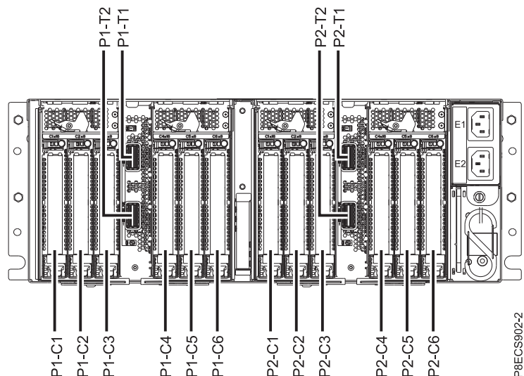
図 4. PCIe スロットのロケーション・コード付きの EMX0 PCIe3 拡張ドロワーの背面図
