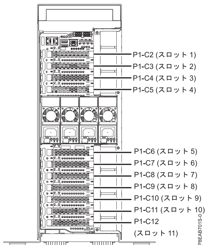
図 3. PCIe スロットのロケーション・コード付きのスタンドアロン型 8286-41A システムの背面図
