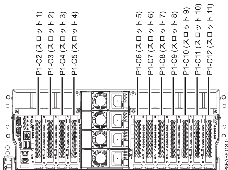
図 1. PCIe スロットのロケーション・コード付きのラック・マウント型 8247-42L システムの背面図
