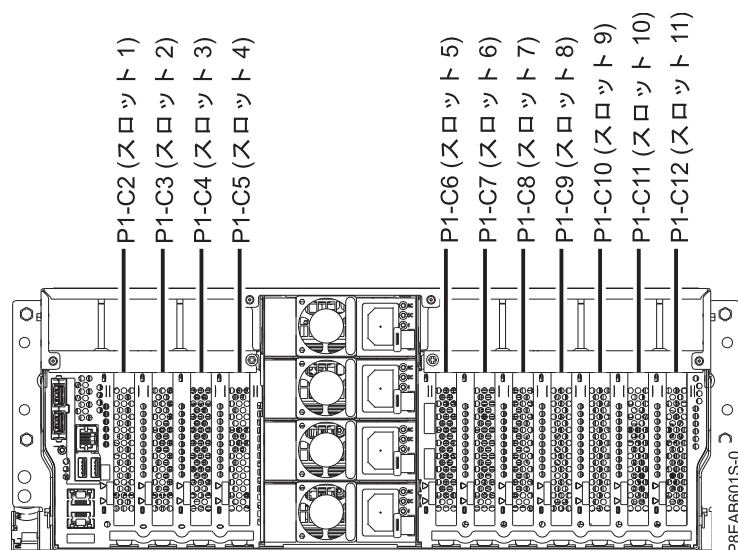
図 2. PCIe スロットのロケーション・コード付きのラック・マウント型 8286-41A システムおよび 8286-42A システムの背面図
