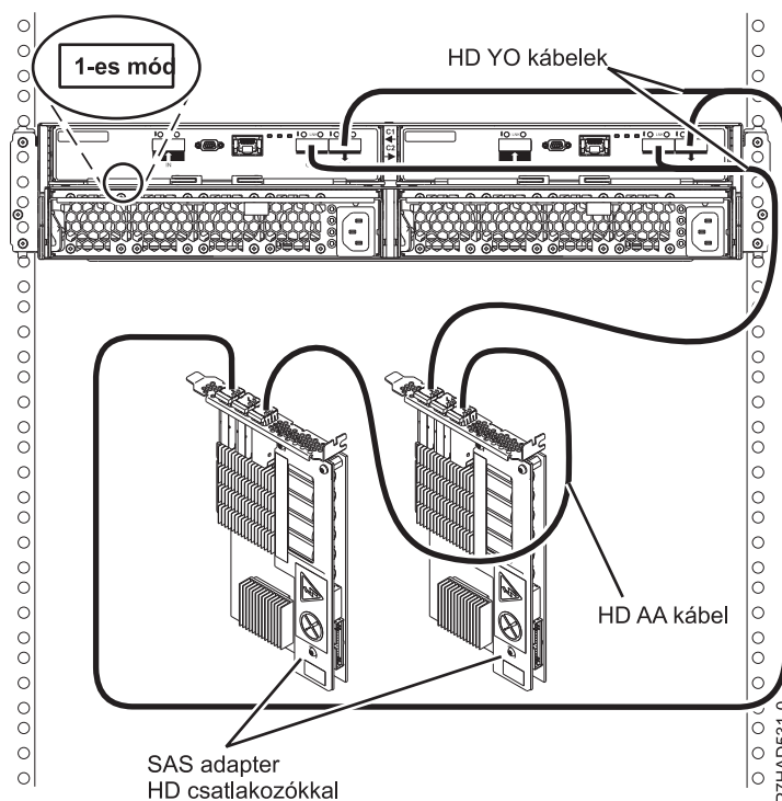
104. ábra: 5887 ház 1. módú csatlakoztatása két PCIe2 SAS adapterhez HD csatlakozókkal
