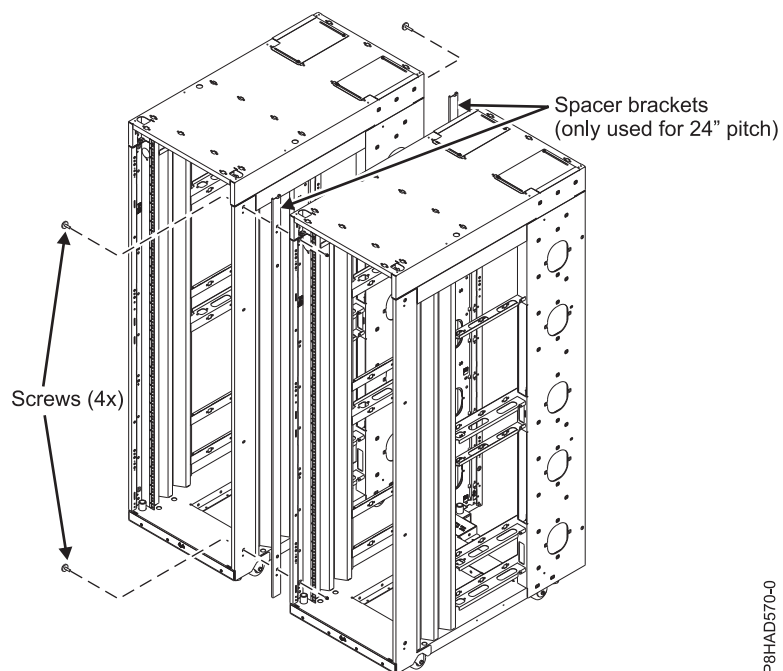
54. ábra: Több rack szekrény csatlakoztatása
