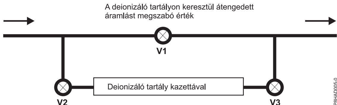
122. ábra: Víz ionmentesítése a hűtőkörbe szerelt ionmentesítő kazettákkal
