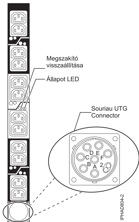
70. ábra: PDU dugaszolóaljzat grafikája
