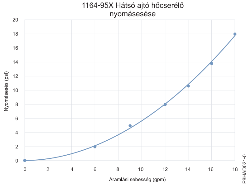
57. ábra: Nyomásesés (szabványos mértékegységek)
