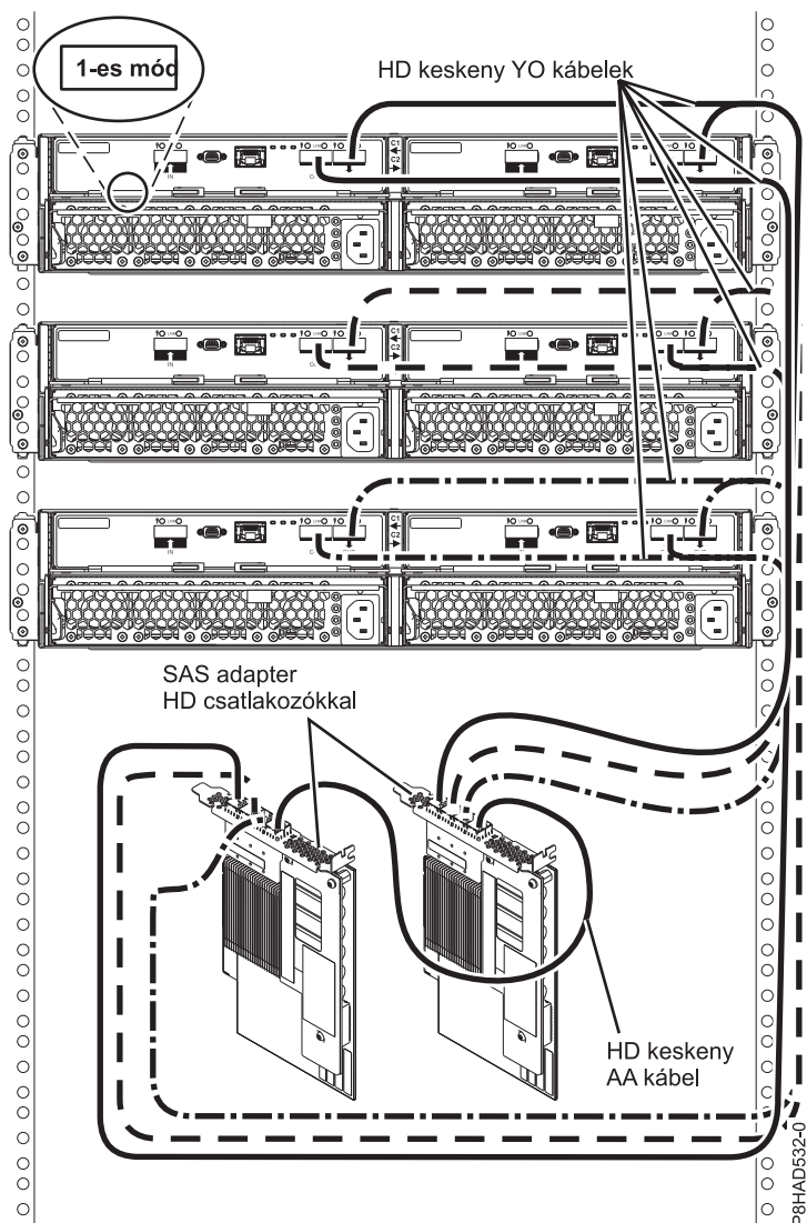
110. ábra: Három 5887 ház 1. módú csatlakoztatása két PCIe3 SAS adapterhez HD keskeny csatlakozókkal
