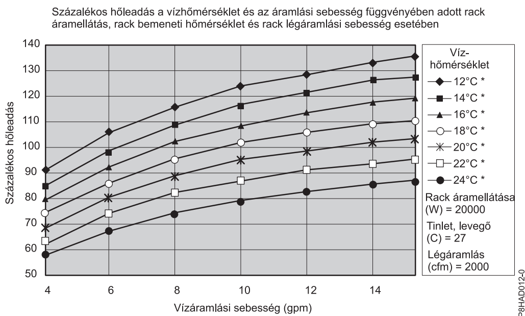
39. ábra: A hőcserélő tipikus teljesítménye, 20 kW hőterhelés
