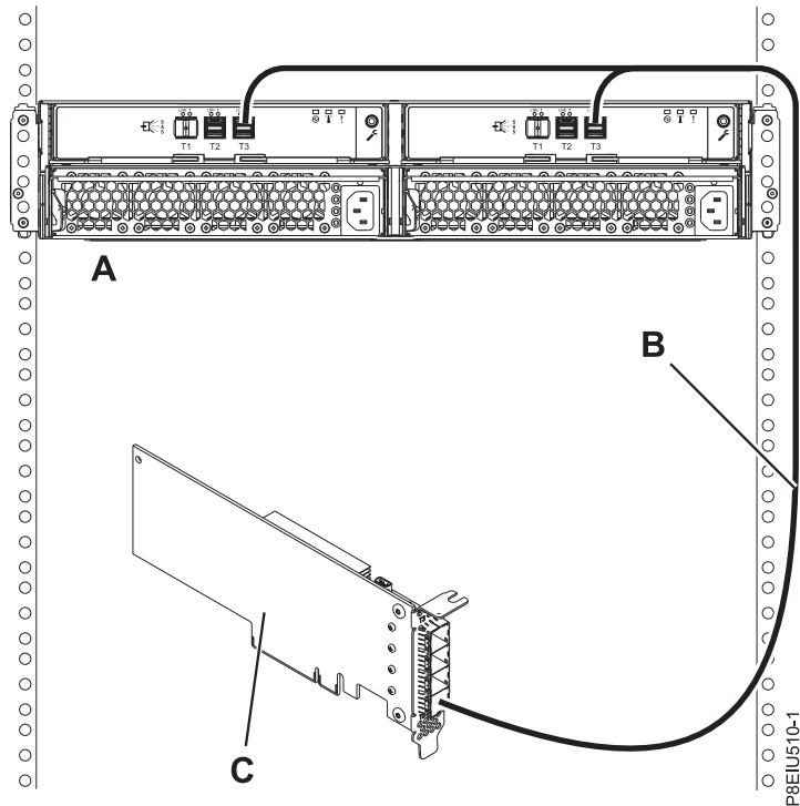
114. ábra: Egy ESLL or ESLS storage enclosure 1-es módú csatlakoztatása egyetlen SAS csatolóhoz YO12 kábel használatával
