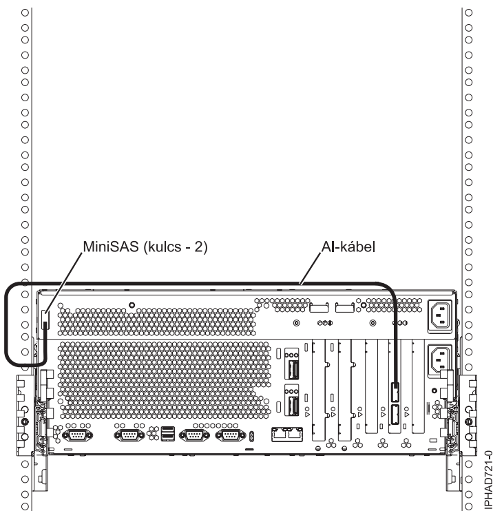
86. ábra: SAS csatló összekapcsolása belső SAS lemez bővítőhellyel a rendszer külső SAS portján keresztül.
