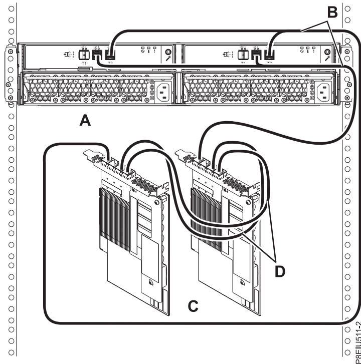
116. ábra: Egy ESLL or ESLS storage enclosure csatlakoztatása egy pár SAS csatolóhoz YO12 kábelek használatával
