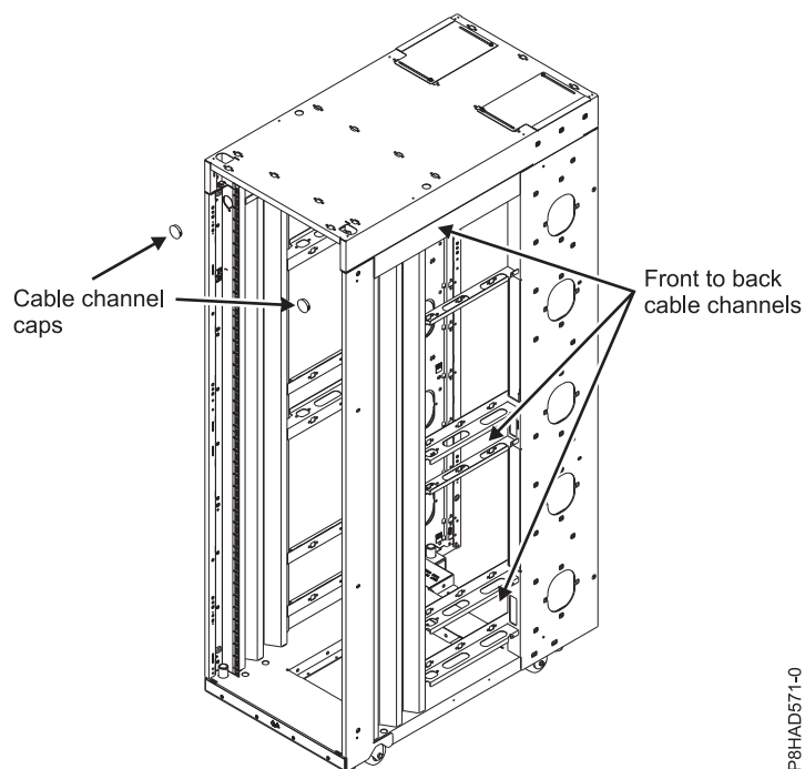
51. ábra: Kábelezés a rack szekrényen belül
