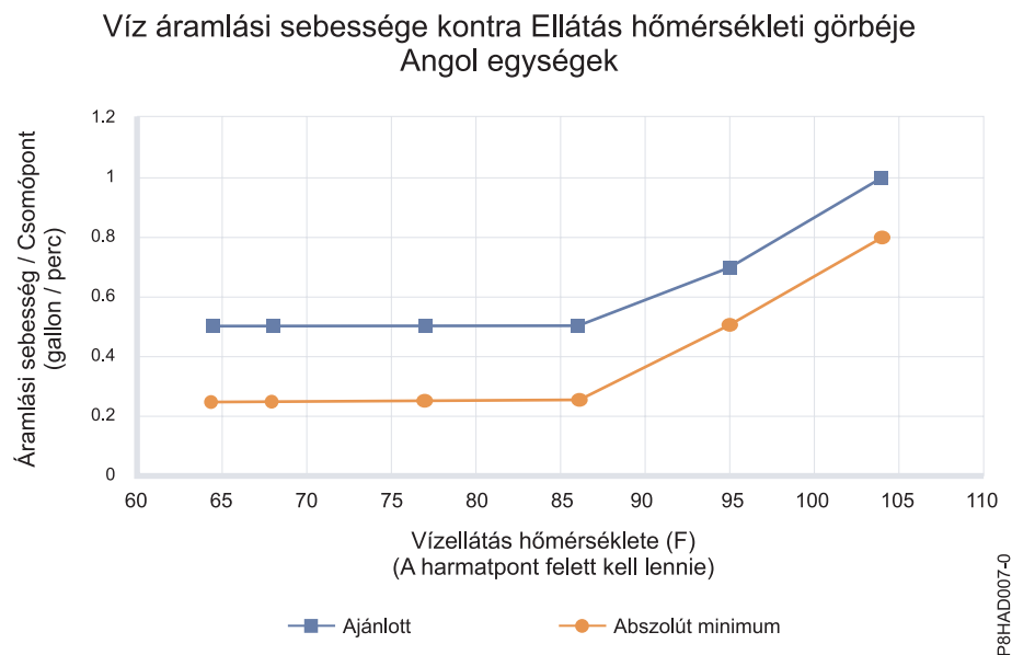
3. ábra: Víz áramlási sebessége az betáplálás és a hőmérséklet függvényében (szabvány egységek)
