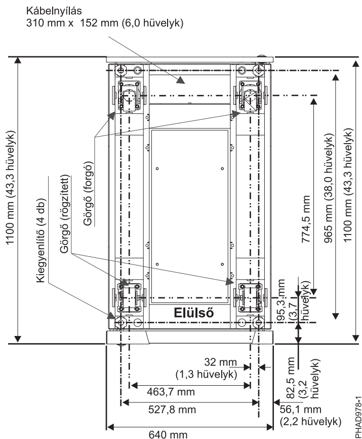
11. ábra: Görgők és kiegyenlítő helye
