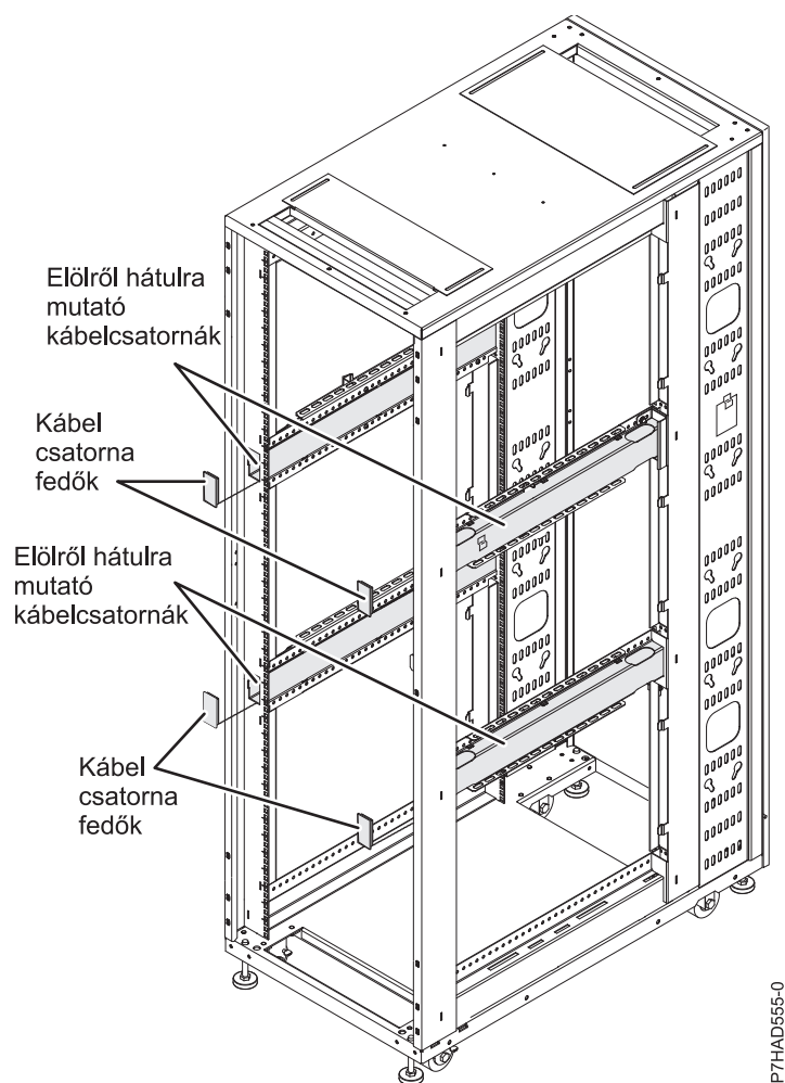
34. ábra: Kábelezés a rack szekrényen belül
