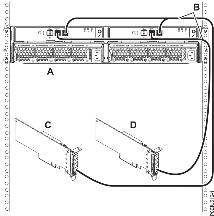
118. ábra: ESLL or ESLS storage enclosure 2-es módú csatlakoztatása két független SAS csatolóhoz YO12 kábelek használatával
