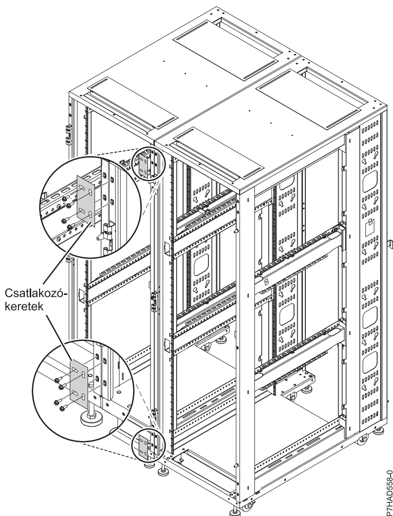
38. ábra: Csatlakozó- keretek
