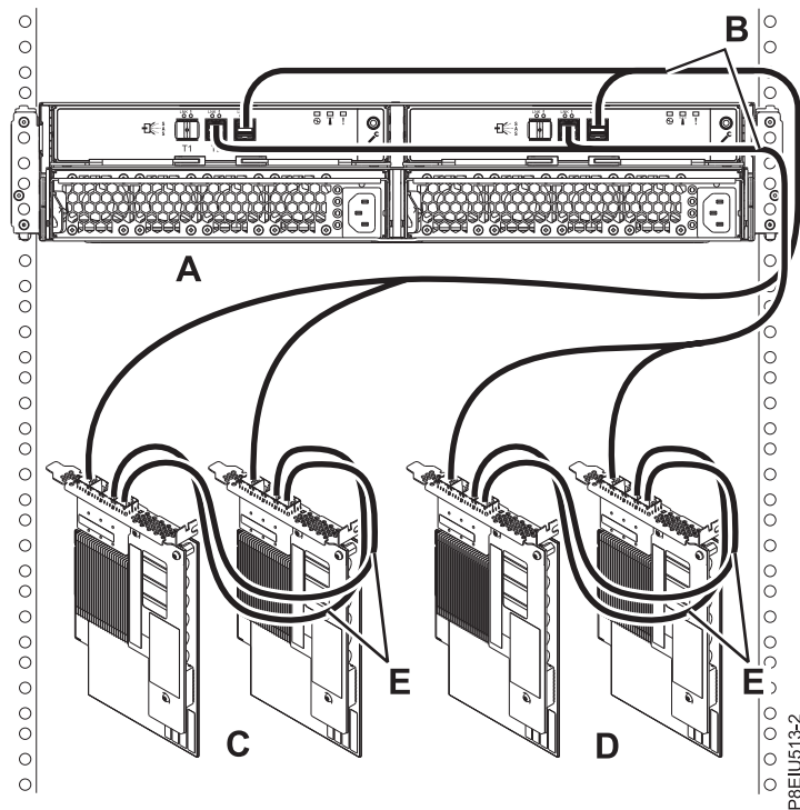
119. ábra: Egy ESLL or ESLS storage enclosure 2-es módú csatlakoztatása két pár SAS csatolóhoz X12 kábelek használatával
