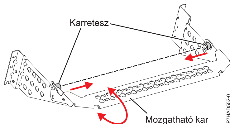
75. ábra: Kábelrendező keret
