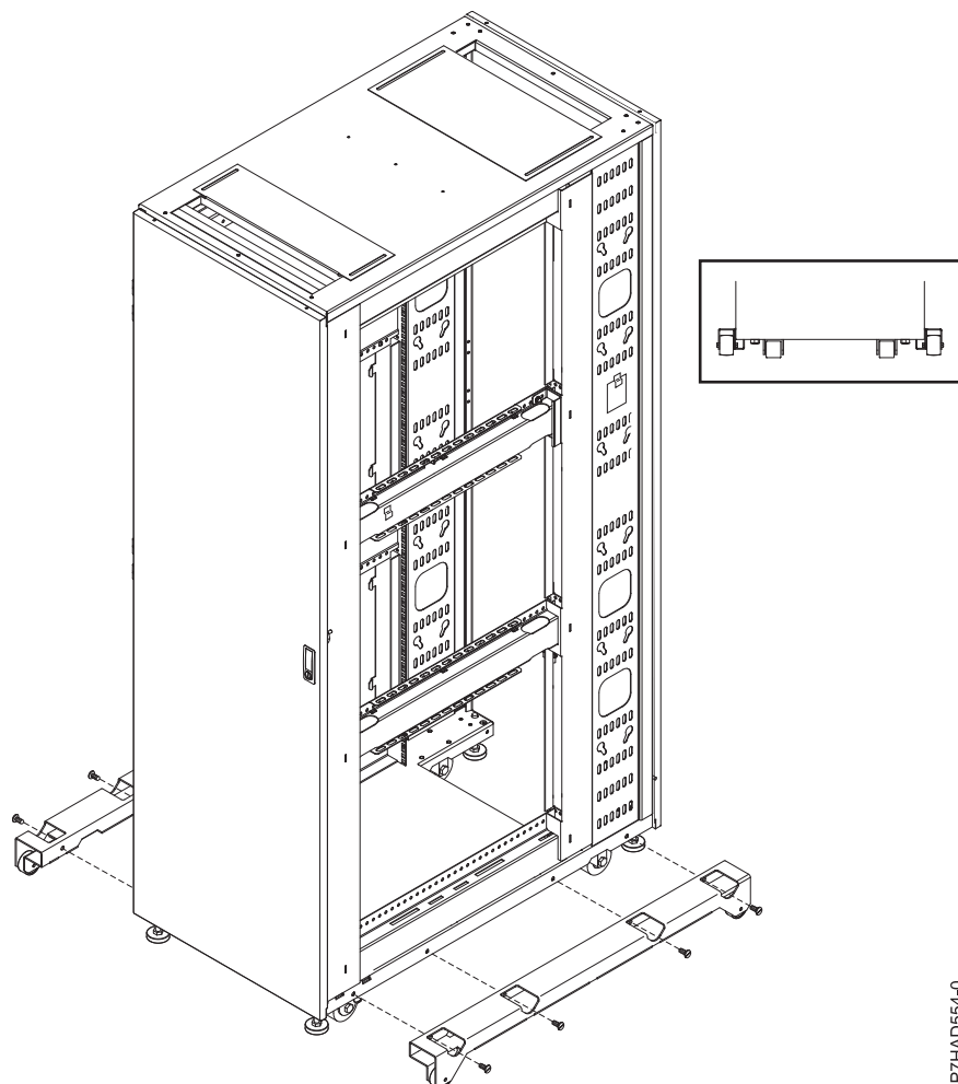
37. ábra: Tartókar helyek
