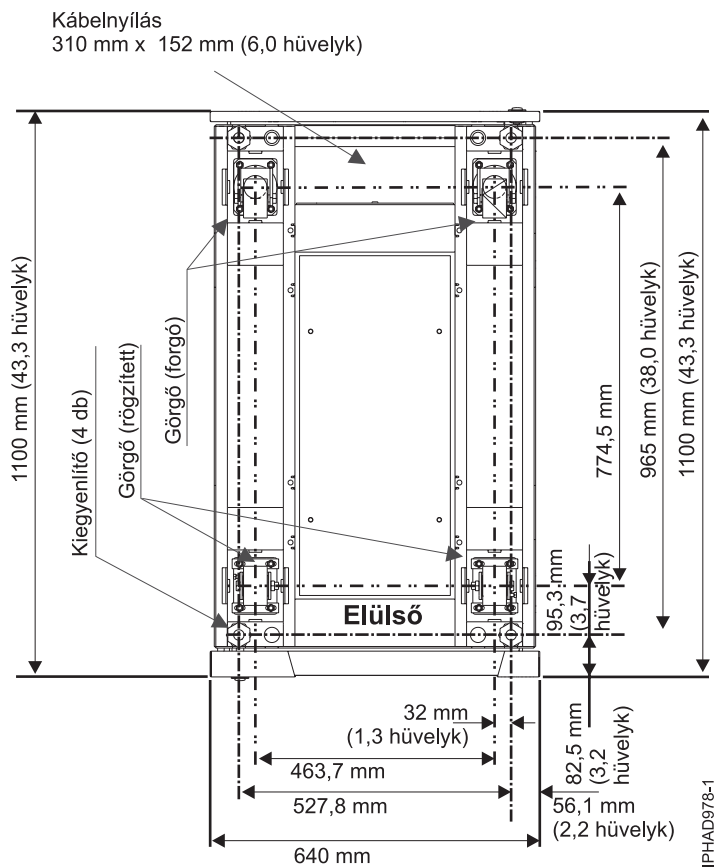
30. ábra: Görgők és kiegyenlítők helye
