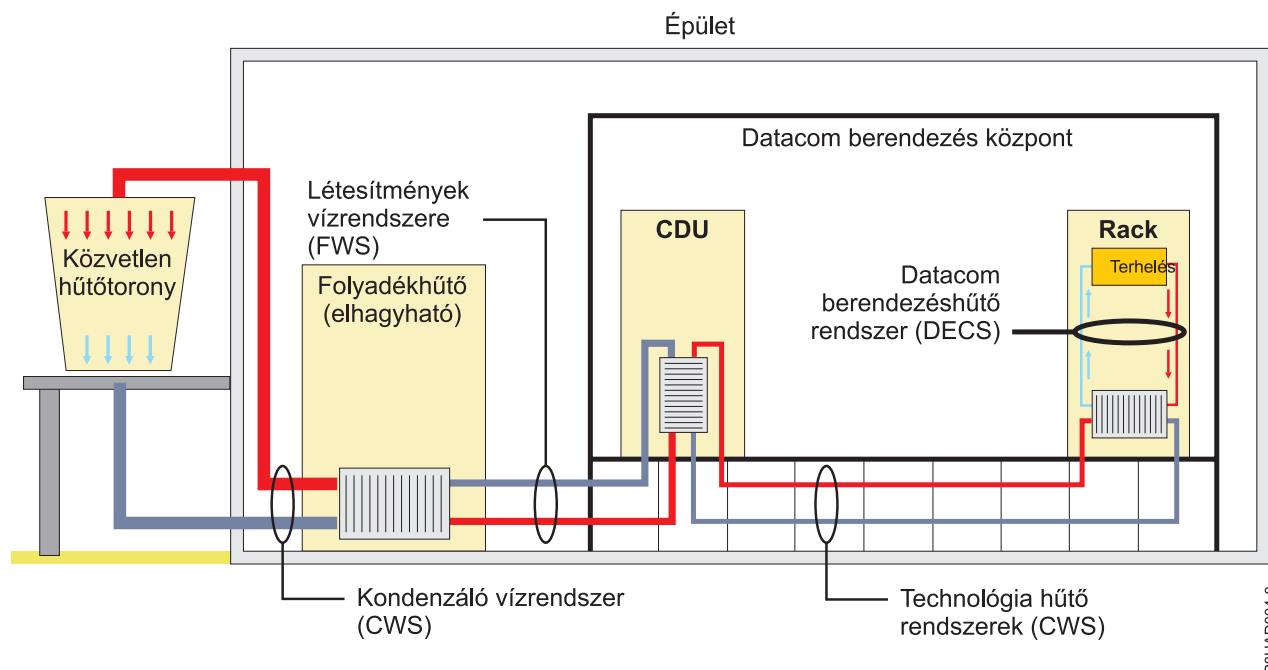
121. ábra: Példák folyadékűtéses rendszerekre és az adatközpontban lévő körökre
