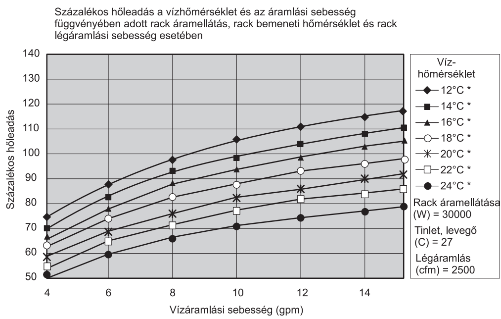
56. ábra: A hőcserélő tipikus teljesítménye, 30 kW hőterhelés
