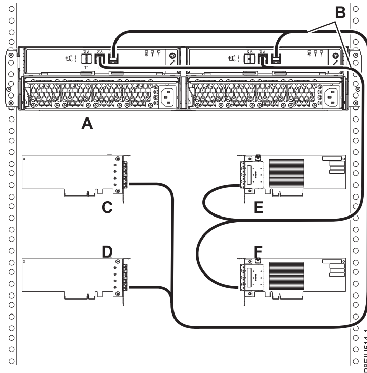
120. ábra: Egy ESSL or ESLS storage enclosure 4-es módú csatlakoztatása négy független SAS csatolóhoz X12 kábelek használatával
