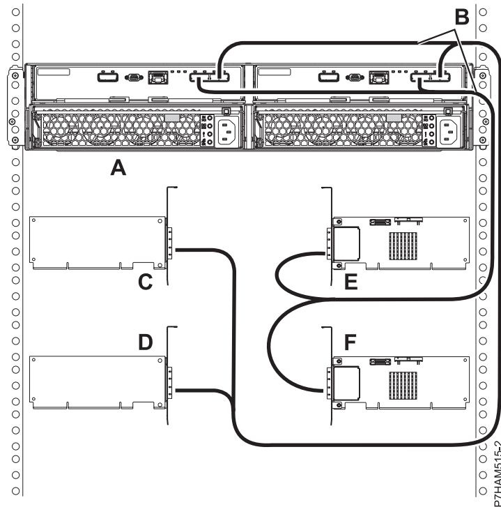
101. ábra: Egy 5887 ház 4. módú csatlakoztatása négy egyedülálló SAS adapterhez X kábelek használatával
