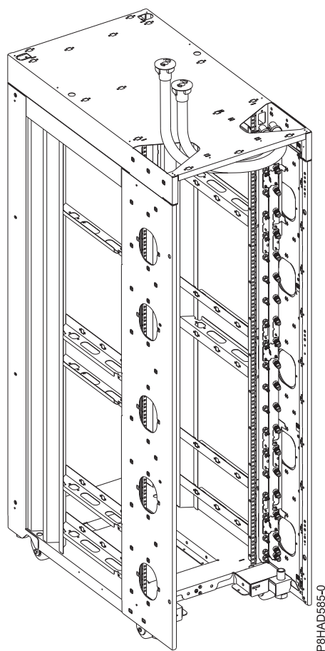
58. ábra: A rack és az elosztó a rack tetején keresztül futó bevezető és visszatérő tömlőkkel
