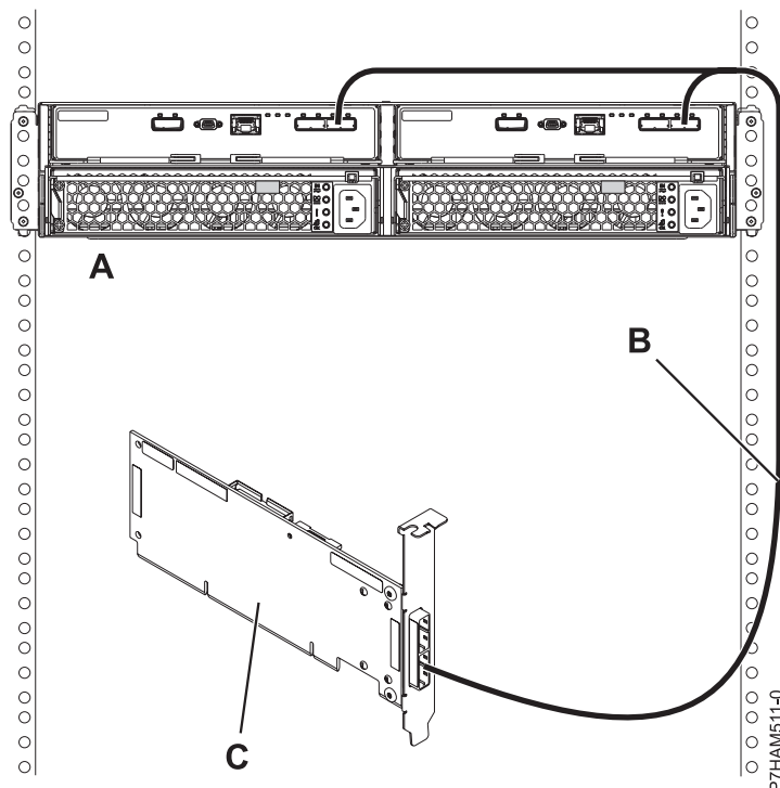
97. ábra: 5887-es ház és egy egyedülálló SAS adapter 1-es módú csatlakozása YO kábelrel
