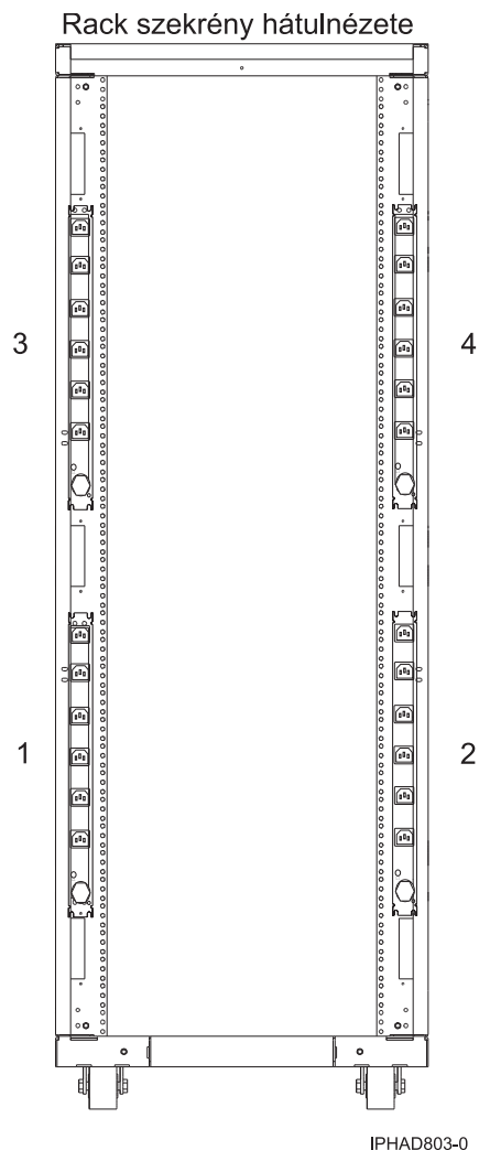
69. ábra: Az áramelosztó egység függőleges helyei
