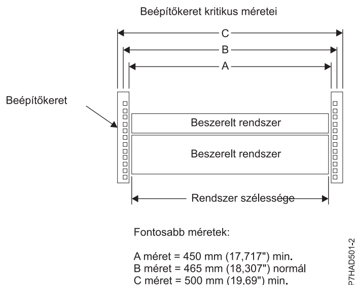
66. ábra: Kritikus beszerelési peremméretek
