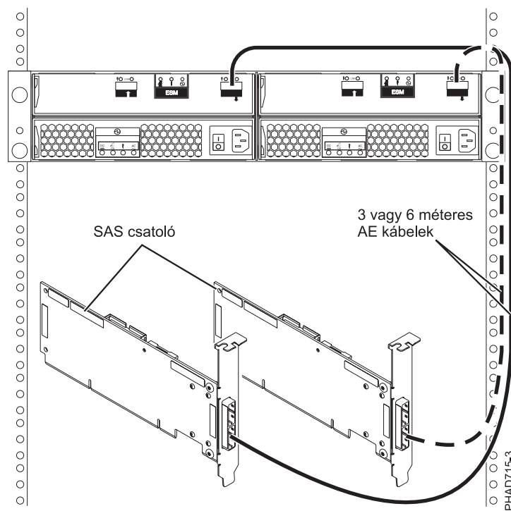
96. ábra: Két RAID SAS csatoló összekapcsolása egy lemez bővítőfiókkal több kezdeményezős HA JBOD konfigurációban
