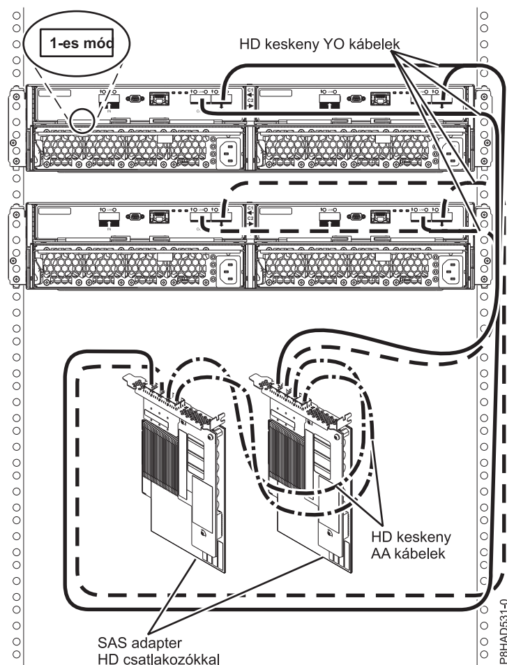
109. ábra: Két 5887 ház 1. módú csatlakoztatása két PCIe3 SAS adapterhez HD keskeny csatlakozókkal
