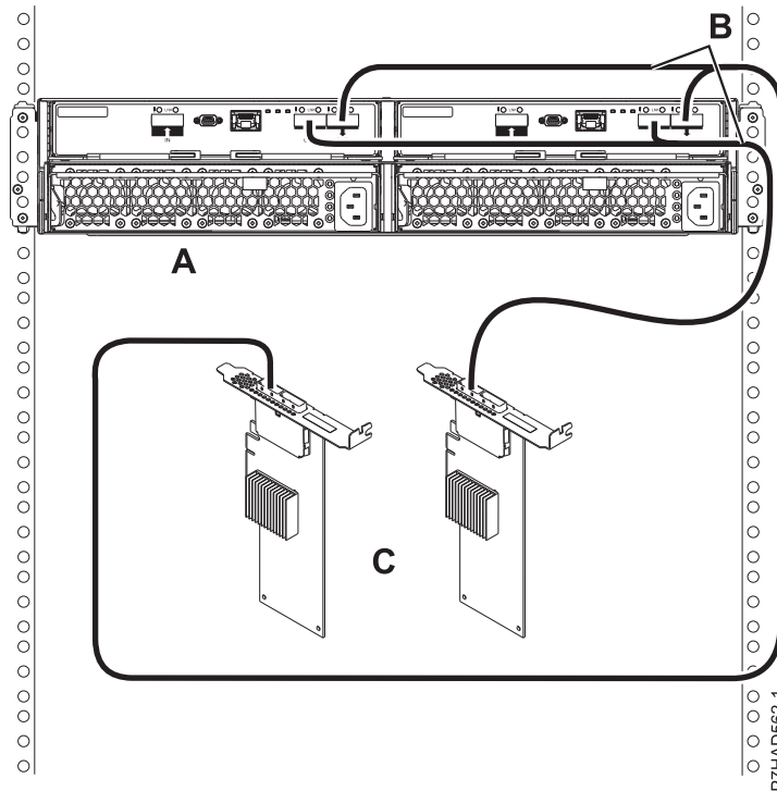
98. ábra: 5887-es ház és két SAS adapter 1-es módú csatlakozása több YO kábellel
