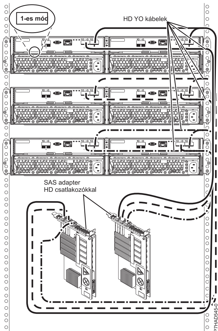
106. ábra: Három 5887 ház 1. módú csatlakoztatása két PCIe2 SAS adapterhez HD csatlakozókkal
