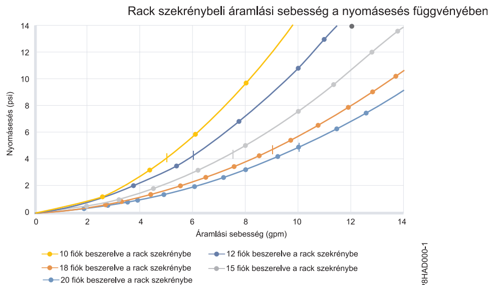
4. ábra: Áramlási sebesség a nyomásesés függvényében (metrikus mértékegységek)
