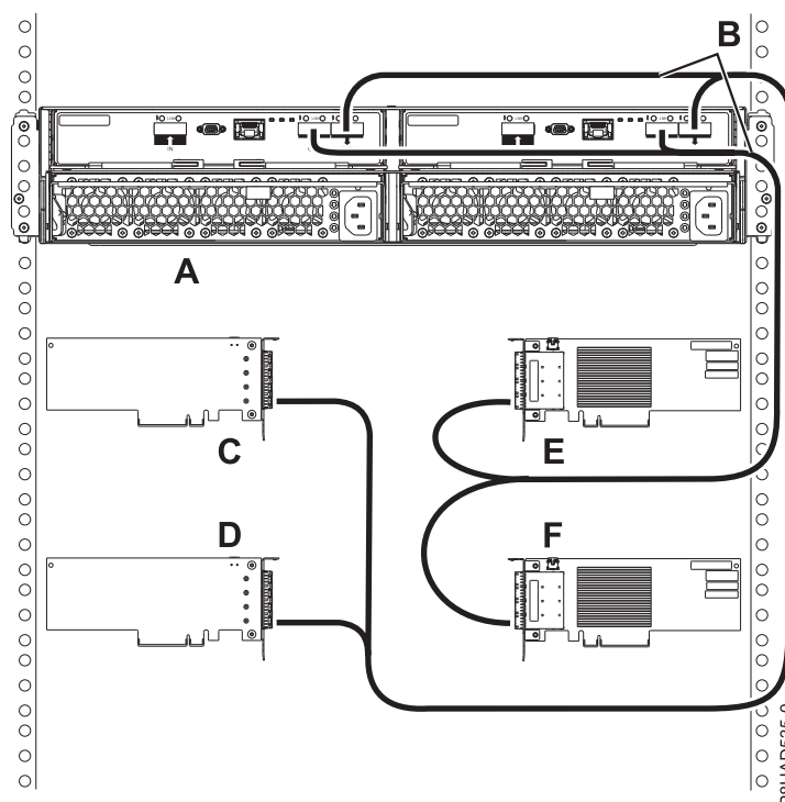
113. ábra: 5887 ház 4. módú csatlakoztatása négy egyedülálló, HD keskeny csatlakozókkal rendelkező PCIe3 SAS adapterhez X kábelek használatával
