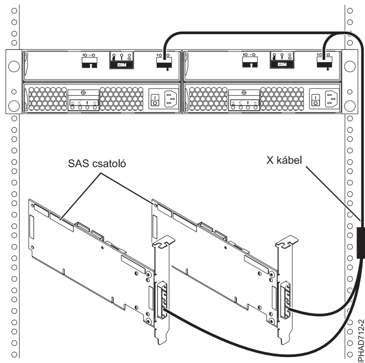
88. ábra: Két SAS RAID csatoló összekapcsolása egy lemez bővítőfiókkal több kezdeményezős HA RAID konfigurációban
