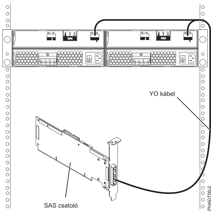
79. ábra: SAS csatoló összekapcsolása egy lemez bővítőfiókkal
