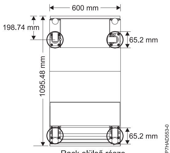
Rack elülső része 33. ábra: Görgőhelyek
