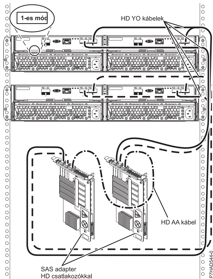
105. ábra: Két 5887 ház 1-es módú csatlakozása HD csatlakozókkal két PCIe2 SAS adapterhez
