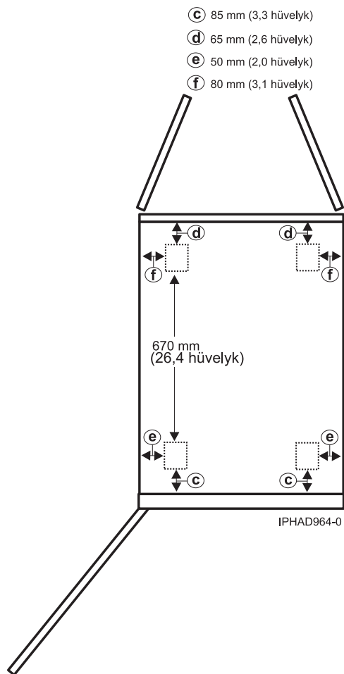
27. ábra: 0555 és 7014-S25 modell görgőhelyei
