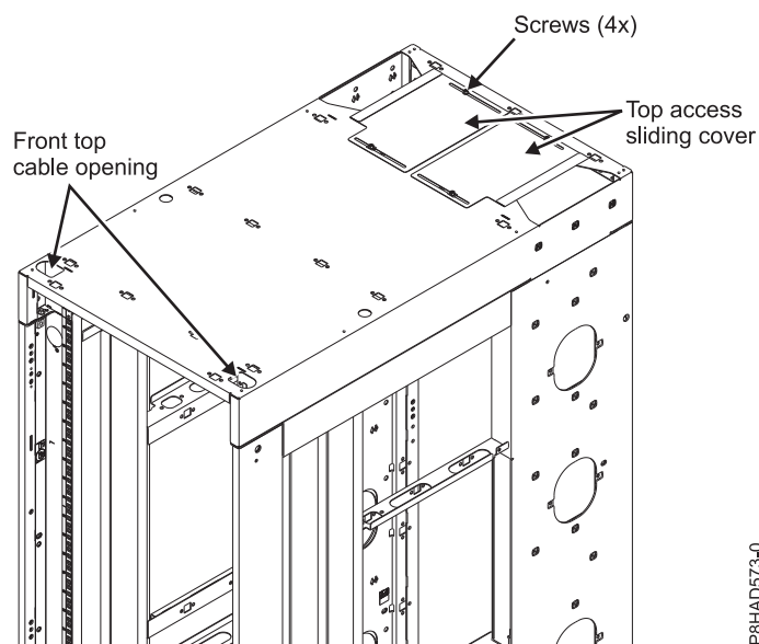
53. ábra: Kábelezés felül
