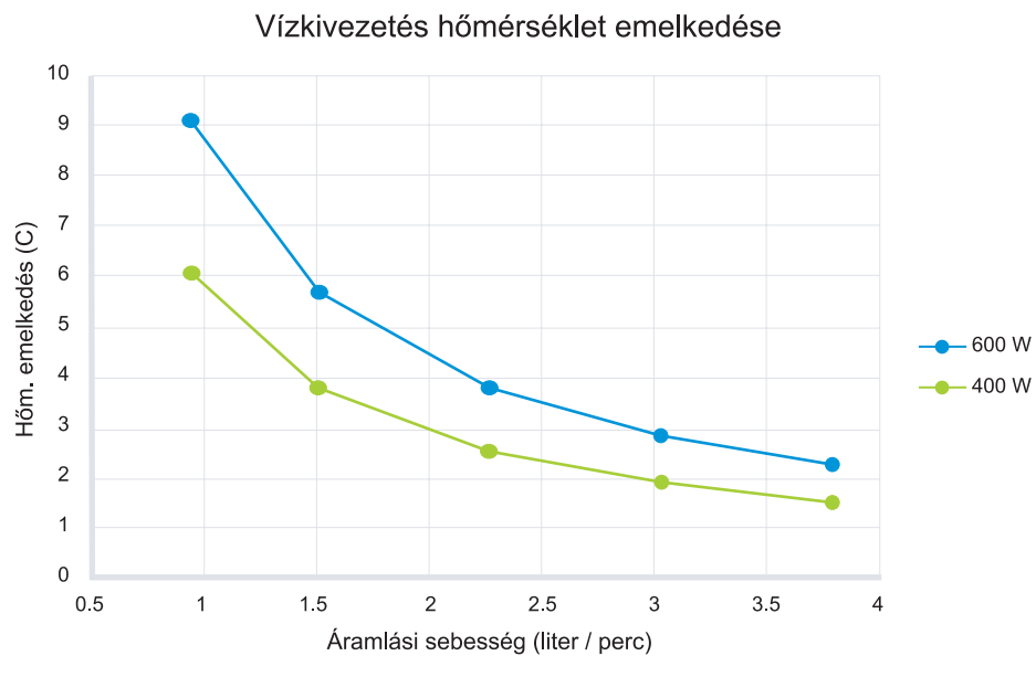
6. ábra: Víz áramlási sebessége az betáplálás és a hőmérséklet függvényében (metrikus egységek)
