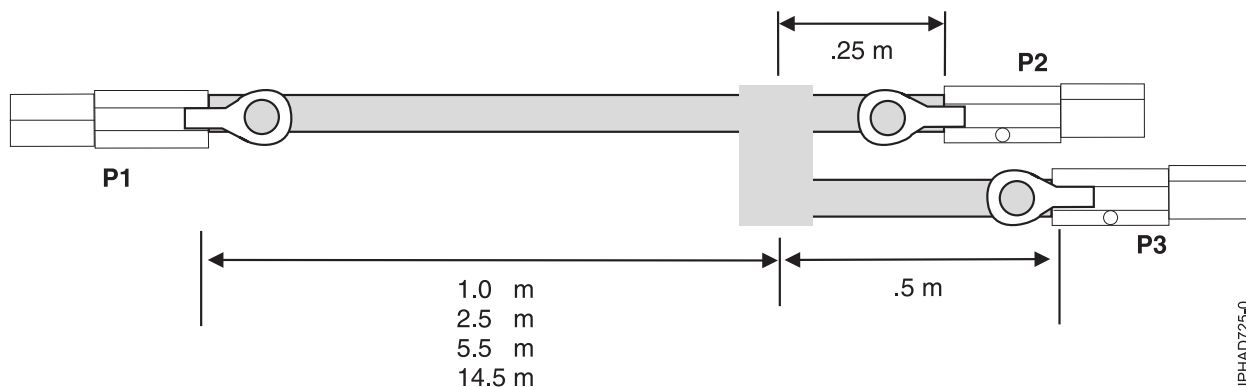
77. ábra: SAS külső YO-kábel összeállítási kábelhosszak
