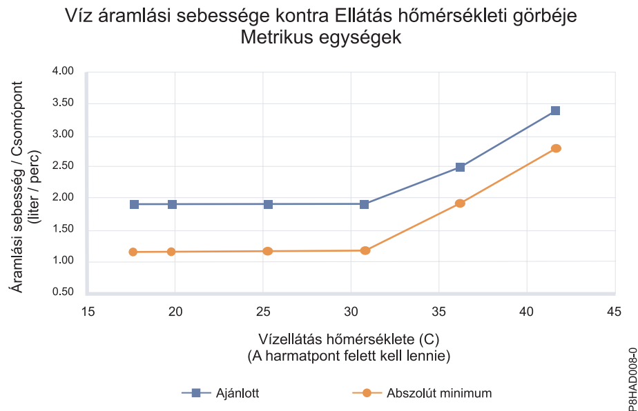
2. ábra: Víz áramlási sebessége az betáplálás és a hőmérséklet függvényében (metrikus egységek)
