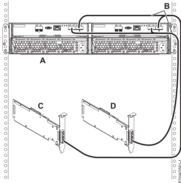
99. ábra: 5887 ház 2. módú csatlakoztatása két egyedülálló SAS adapterhez YO kábelekkel
