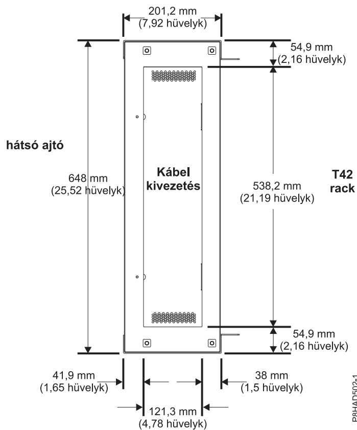
31. ábra: FC ERG0 hátulsó rack kiterjesztő (felülnézet)
