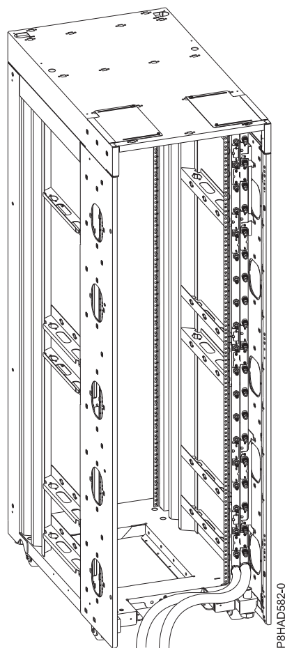
59. ábra: A rack és az elosztó a rack alján keresztül futó bevezető és visszatérő tömlőkkel
