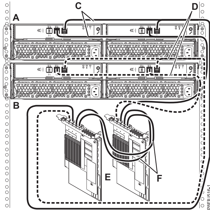
117. ábra: Két ESLL vagy ESLS tárolóház 1-es módú csatlakoztatása egy pár SAS csatolóhoz YO12 kábelek használatával
