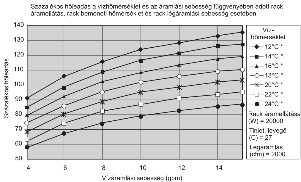
55. ábra: A hőcserélő tipikus teljesítménye, 20 kW hőterhelés
