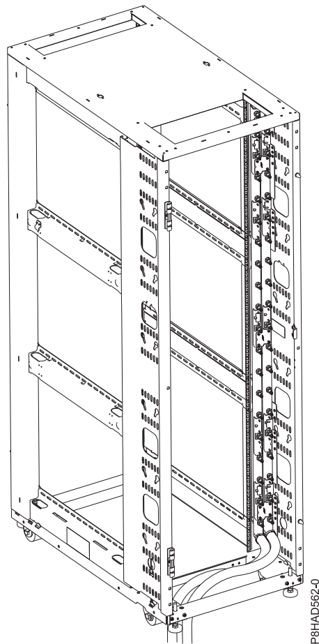
43. ábra: A rack és az elosztó a rack alján keresztül futó bevezető és visszatérő tömlőkkel
