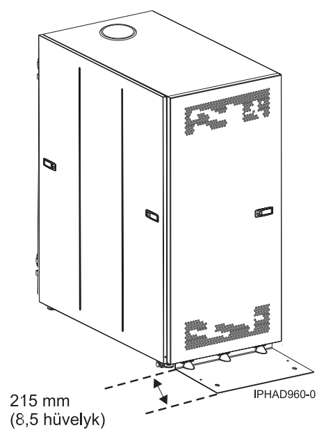
25. ábra: 0555 és 7014-S25 modell stabilizáló lábbal
