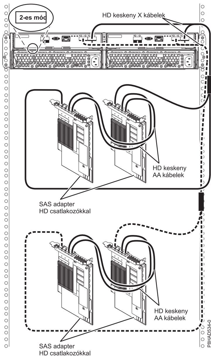
112. ábra: 5887 ház 2. módú csatlakoztatása két pár PCIe3 SAS adapterhez HD keskeny csatlakozókkal
