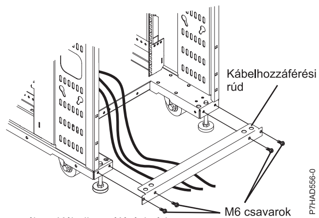
35. ábra: Kábelhozzáférési-rúd
