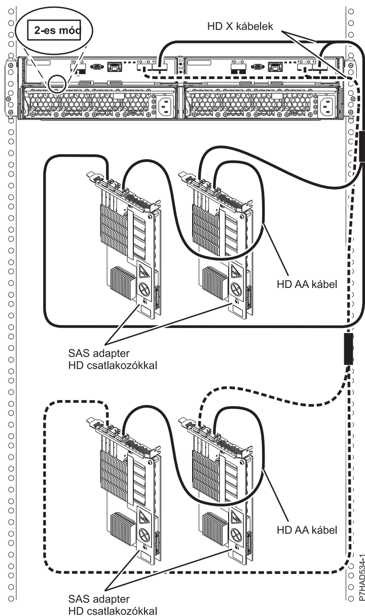
107. ábra: 5887 ház 2-es módú csatlakoztatása HD csatlakozókkal két pár PCIe2 SAS adapterhez
