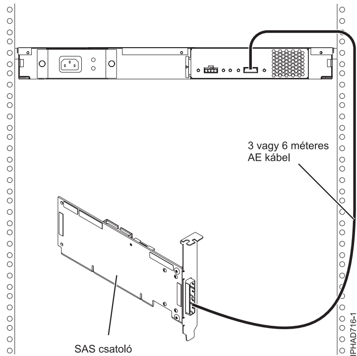
83. ábra: SAS csatoló összekapcsolása egy adathordozó bővítőfiókkal
