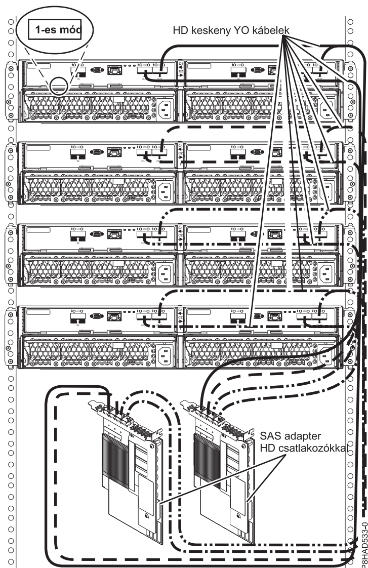
111. ábra: Négy 5887 ház 1. módú csatlakoztatása két PCIe3 SAS adapterhez HD keskeny csatlakozókkal
