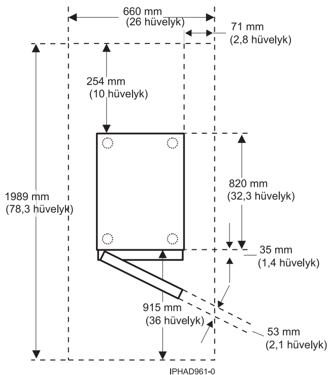
23. ábra: 0554 és 7014-S11 modell tervezési nézete
