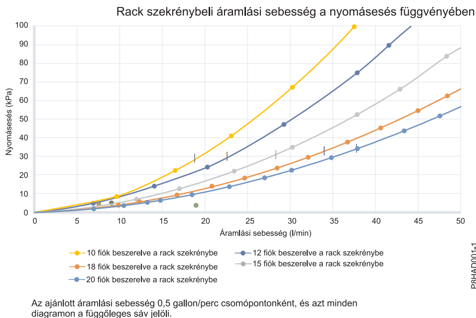
5. ábra: Áramlási sebesség a nyomásesés függvényében (szabványos mértékegységek)
