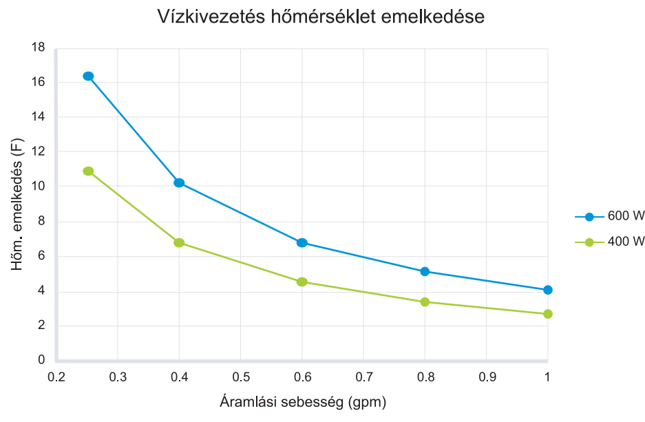
7. ábra: Víz áramlási sebessége az betáplálás és a hőmérséklet függvényében (szabvány egységek)
