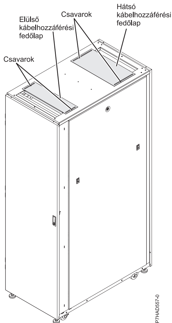
36. ábra: Kábelhozzáférési fedőlapok
