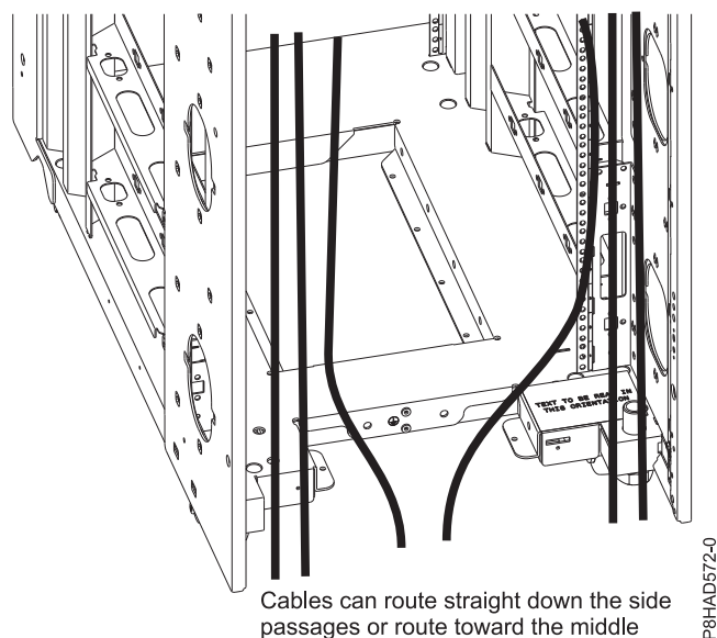
52. ábra: Kábelezés a padló alatt
