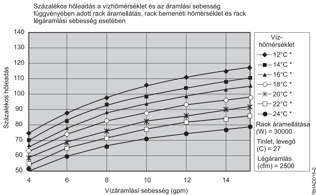
40. ábra: A hőcserélő tipikus teljesítménye, 30 kW hőterhelés
