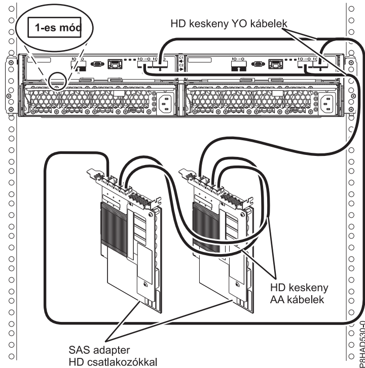
108. ábra: 5887 ház 1. módú csatlakoztatása két PCIe3 SAS adapterhez HD keskeny csatlakozókkal
