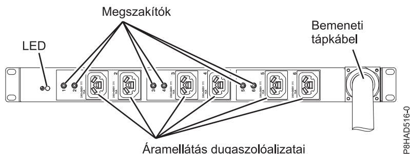
72. ábra: HVDC PDU
