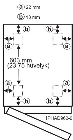
24. ábra: 0554 és 7014-S11 modell görgőhelyei
