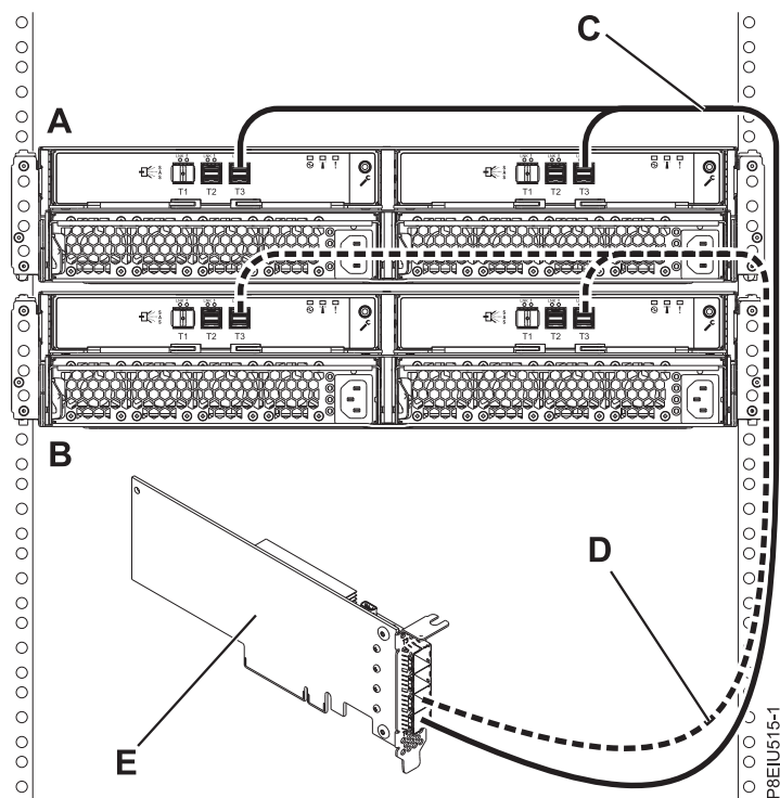
115. ábra: Két ESLL vagy ESLS tárolóház 1-es módú csatlakoztatása egyetlen SAS csatolóhoz YO12 kábelek használatával
