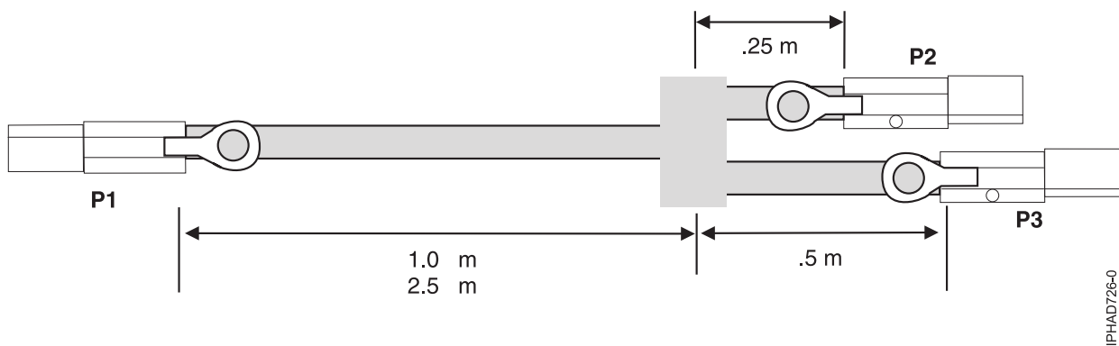
78. ábra: SAS külső YI-kábel összeállítási kábelhosszak
