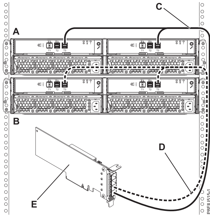
92. ábra: Két ESLL vagy ESLS tárolóház 1-es módú csatlakoztatása egyetlen SAS csatolóhoz YO12 kábelek használatával
