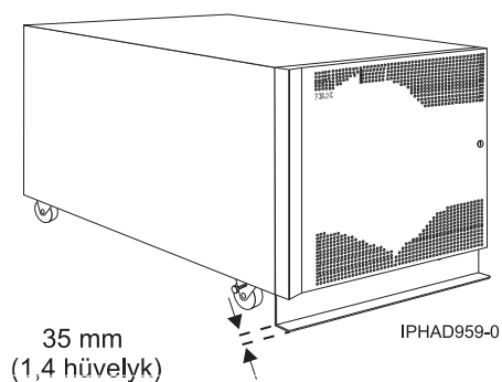
15. ábra: 0554 és 7014-S11 modell stabilizáló rúddal
