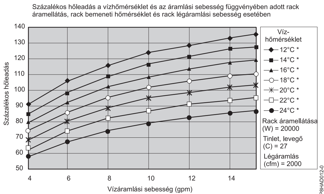
53. ábra: A hőcserélő tipikus teljesítménye, 20 kW hőterhelés
