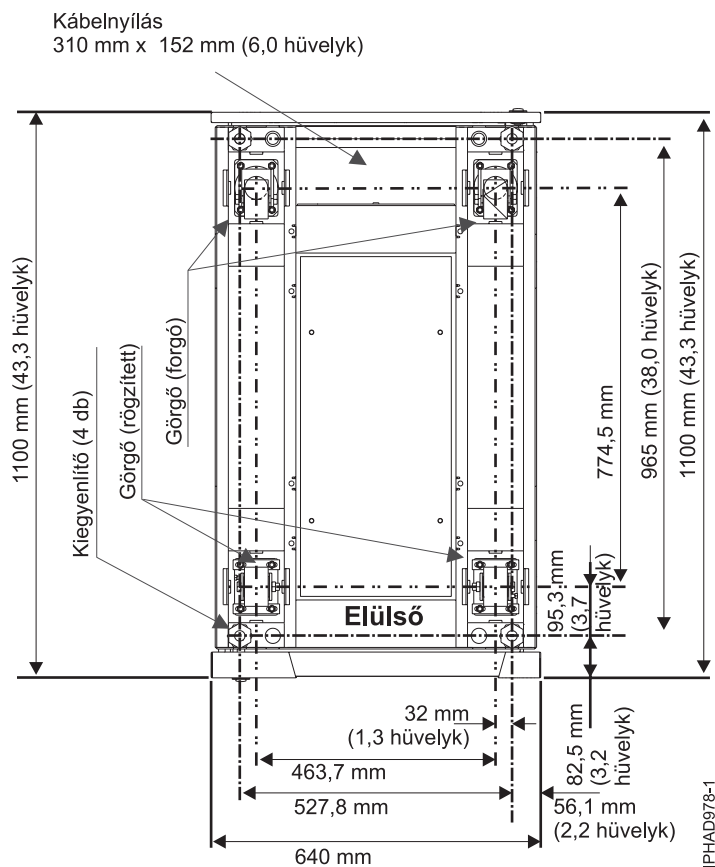
9. ábra: Görgők és kiegyenlítők helye
