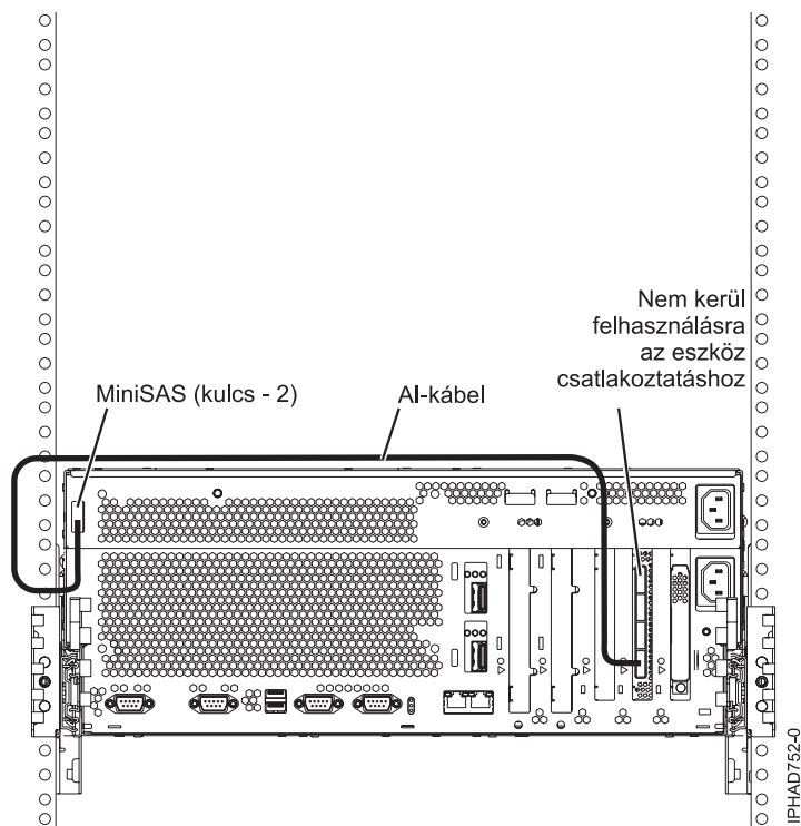
77. ábra: Lemez bővítőfiókokhoz csatlakoztatott FC5904 vagy FC5908 csatoló
