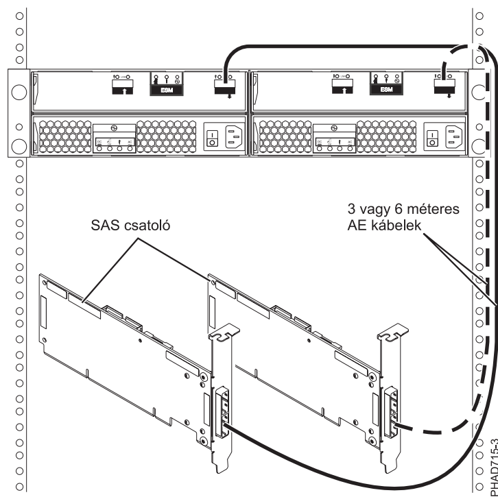
86. ábra: Két RAID SAS csatoló összekapcsolása egy lemez bővítőfiókkal több kezdeményezős HA JBOD konfigurációban
