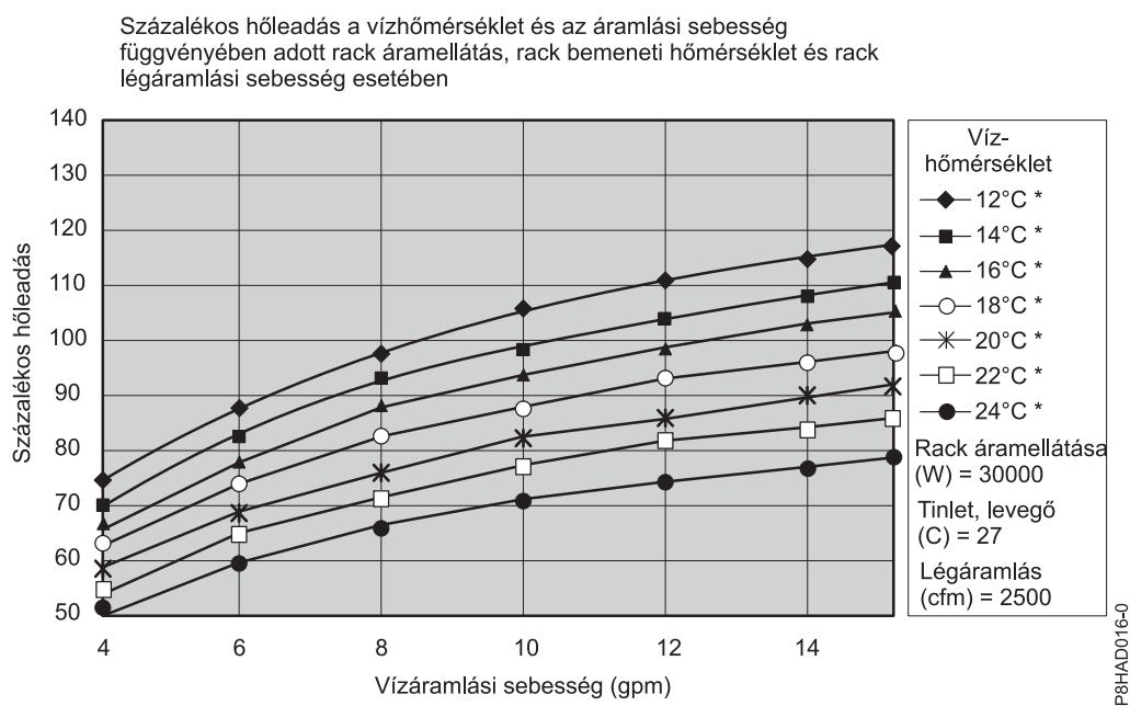
54. ábra: A hőcserélő tipikus teljesítménye, 30 kW hőterhelés
