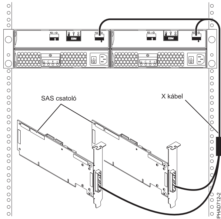
78. ábra: Két SAS RAID csatoló összekapcsolása egy lemez bővítőfiókkal több kezdeményezős HA RAID konfigurációban
