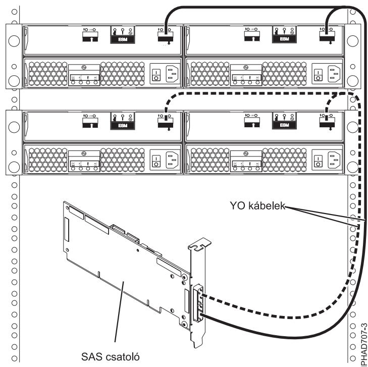
70. ábra: SAS csatoló összekapcsolása két lemez bővítőfiókkal
