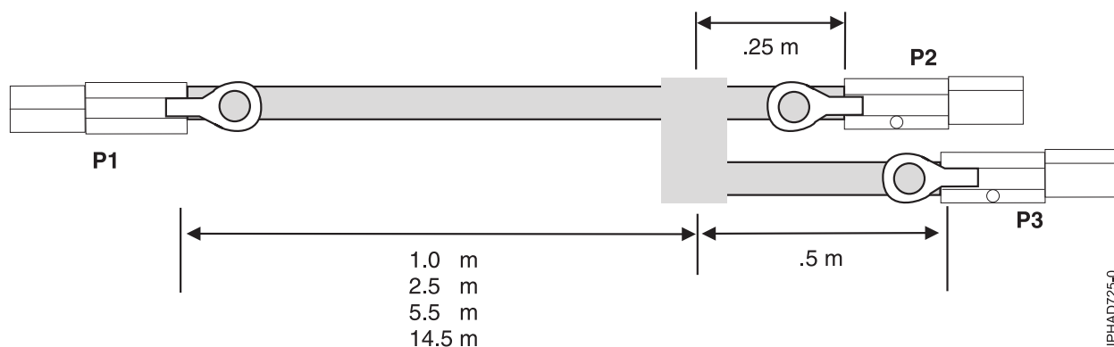
67. ábra: SAS külső YO-kábel összeállítási kábelhosszak
