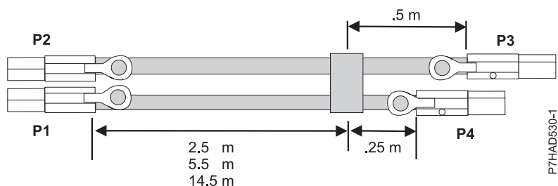
66. ábra: SAS külső X-kábel összeállítási kábelhosszak
