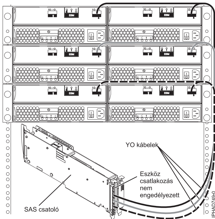
72. ábra: Háromportos SAS csatoló összekapcsolása lemez bővítőfiókokkal
