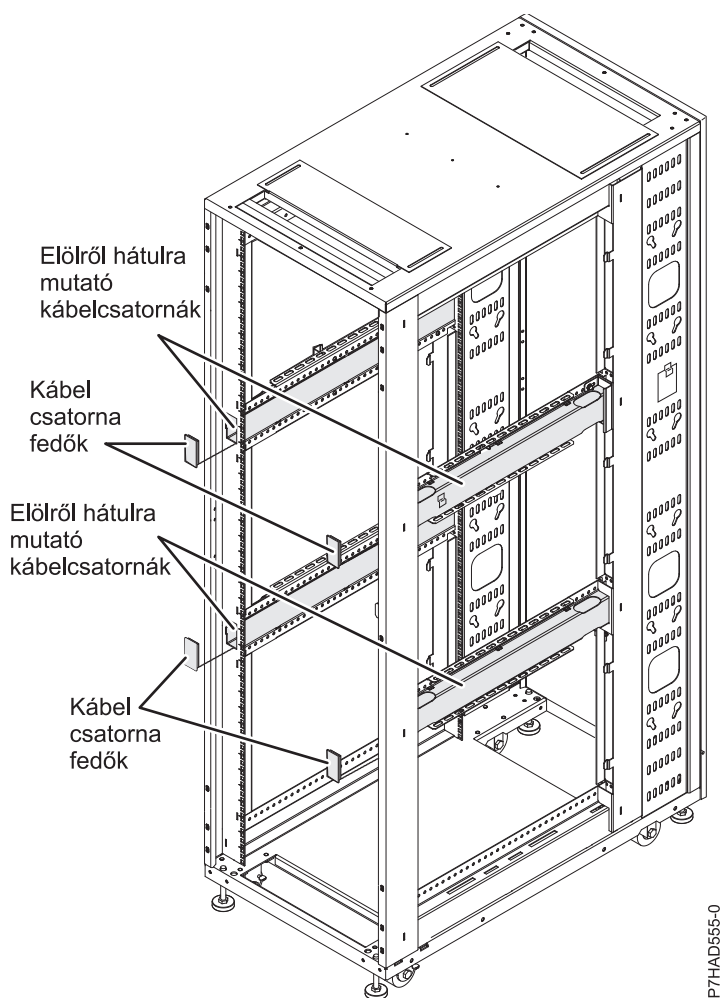
32. ábra: Kábelezés a rack szekrényen belül
