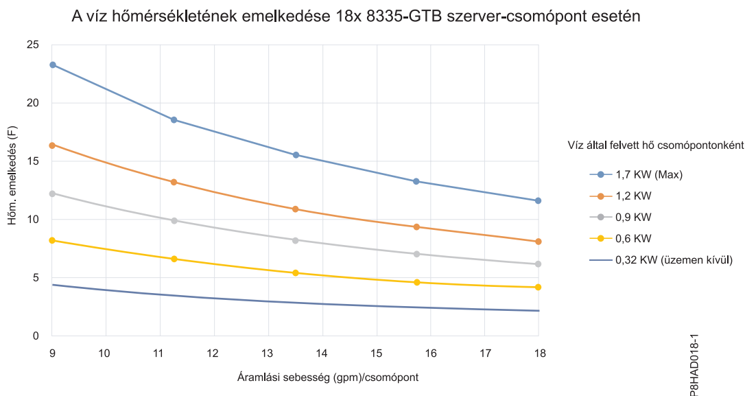
5. ábra: Vízáramlási sebesség a vízellátás hőmérsékletének függvényében - 18 szervertes teljes rack esetén
