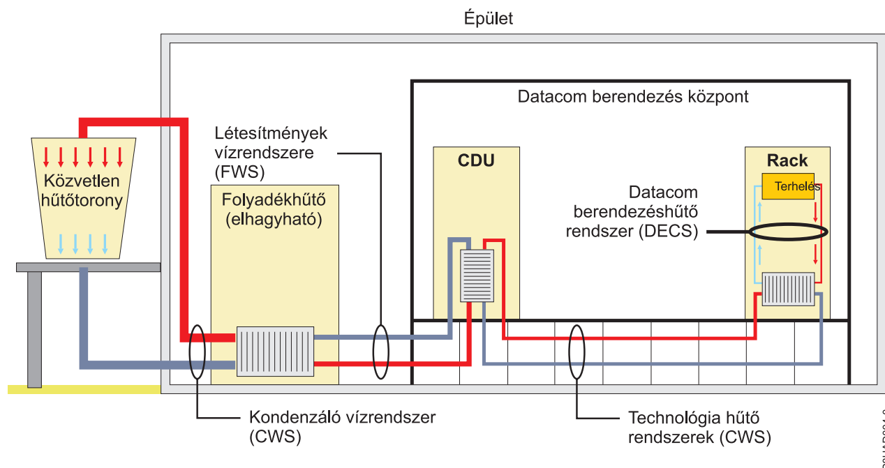
87. ábra: Példák folyadékűtéses rendszerekre és az adatközpontban lévő körökre
