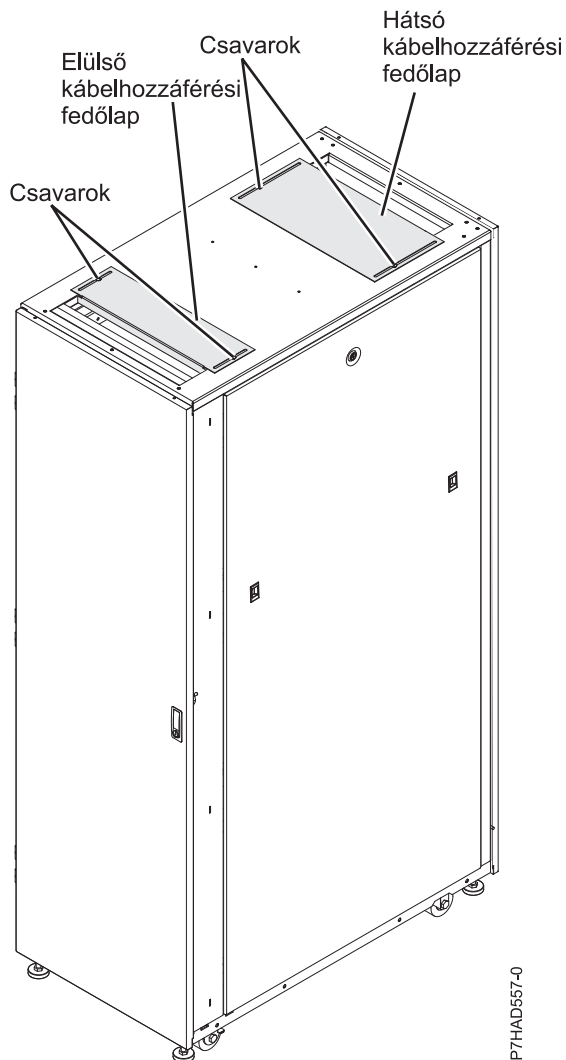
34. ábra: Kábelhozzáférési fedőlapok
