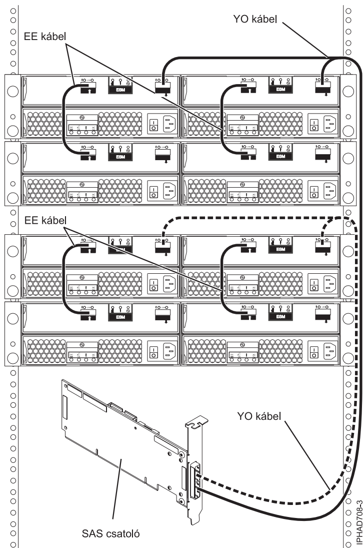
71. ábra: SAS csatoló összekapcsolása négy lemez bővítőfiókkal
