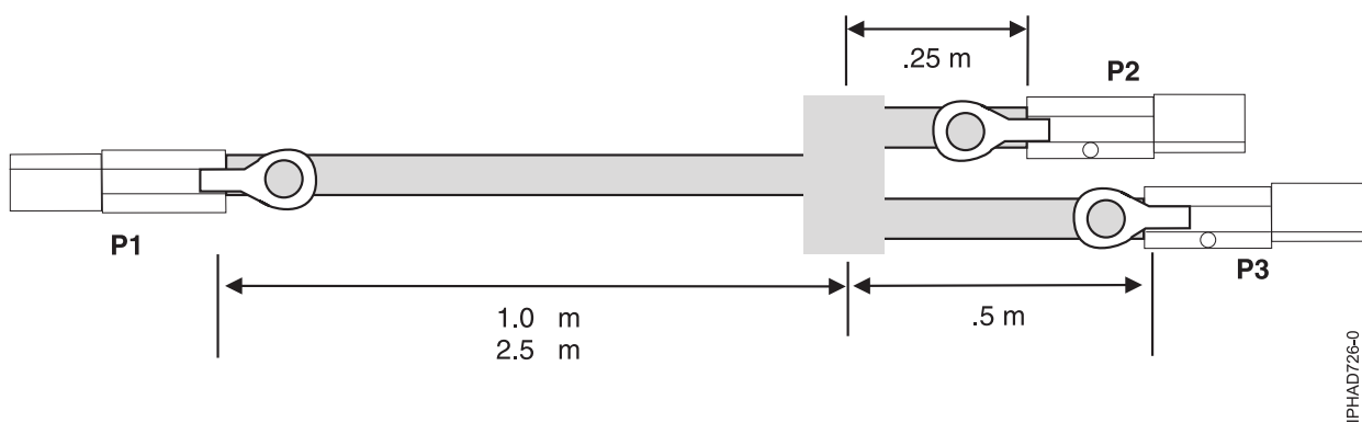
68. ábra: SAS külső YI-kábel összeállítási kábelhosszak
