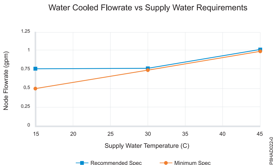
2. ábra: Vízhűtéses áramlási sebesség a vízhűtési követelmények tükrében (szabvány egységek)
