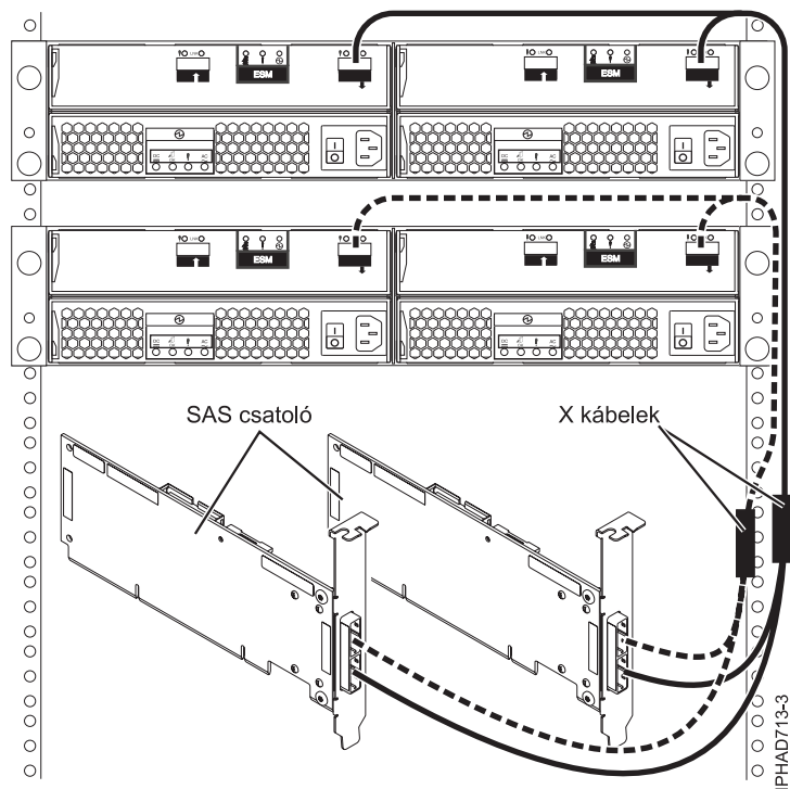
79. ábra: Két SAS RAID csatoló összekapcsolása két lemez bővítművel több kezdeményezős HA RAID konfigurációban
