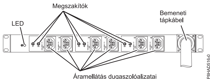
62. ábra: HVDC PDU
