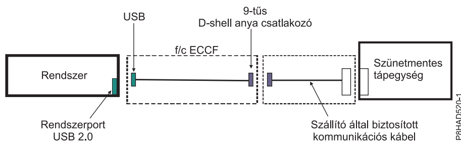
58. ábra: A 5148-21L, 5148-22L, 8247-21L, 8247-21L, 8247-22L, 8247-42L, 8284-22A, 8286-41A és 8286-42A rendszerek szűnetmentes tápegység (UPS) kábelezése
