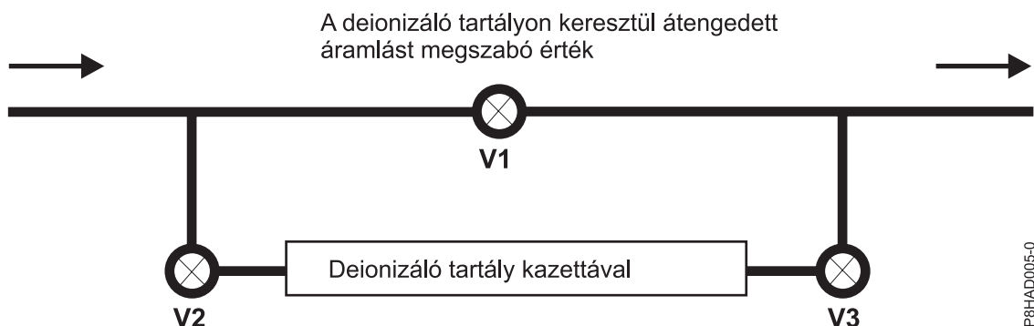
88. ábra: Víz ionmentesítése a hűtőkörbe szerelt ionmentesítő kazettákkal
