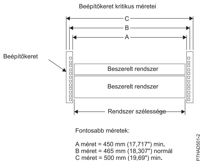
56. ábra: Kritikus beszerelési peremméretek
