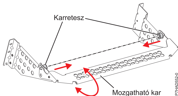
65. ábra: Kábelrendező keret
