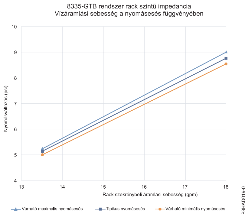
3. ábra: Áramlási sebesség a nyomásesés függvényében (szabványos mértékegységek) - 18 szerveres teljes rack esetén
