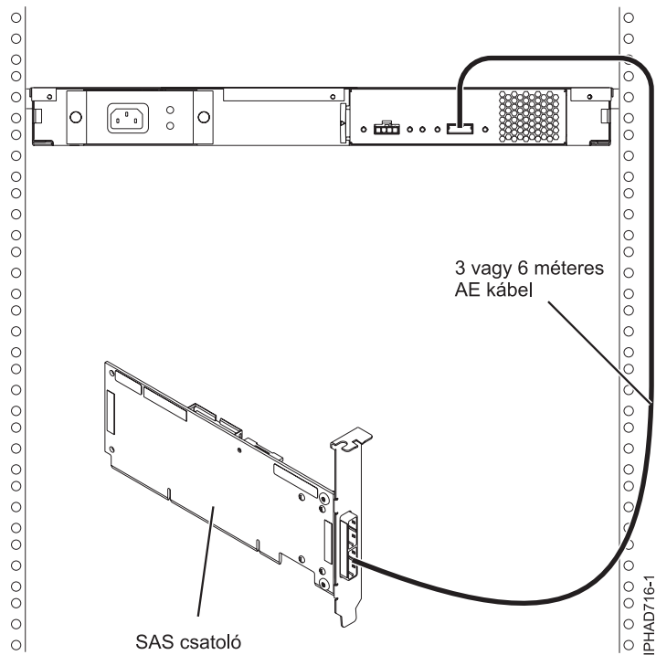
73. ábra: SAS csatoló összekapcsolása egy adathordozó bővítőfiókkal
