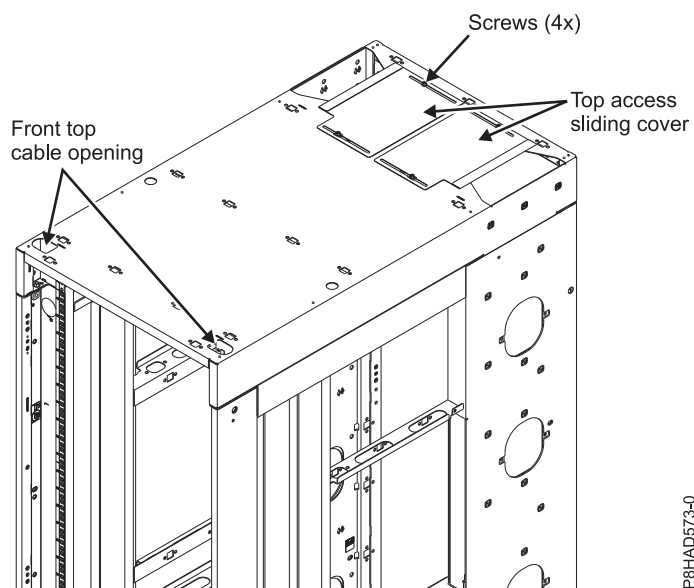
51. ábra: Kábelezés felül
