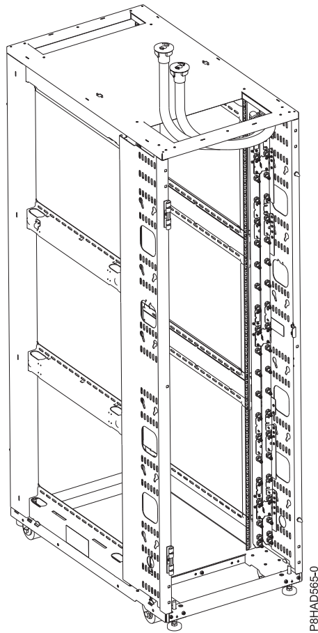
40. ábra: A rack és az elosztó a rack tetején keresztül futó bevezető és visszatérő tömlőkkel
