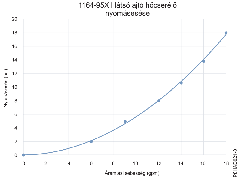
55. ábra: Nyomásesés (szabványos mértékegységek)
