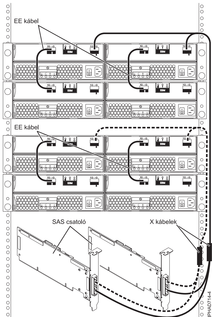
80. ábra: Két SAS RAID csatoló összekapcsolása négy lemez bővítőfiókkal több kezdeményezős HA RAID konfigurációban
