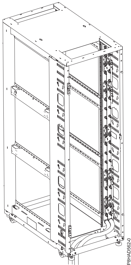
41. ábra: A rack és az elosztó a rack alján keresztül futó bevezető és visszatérő tömlőkkel
