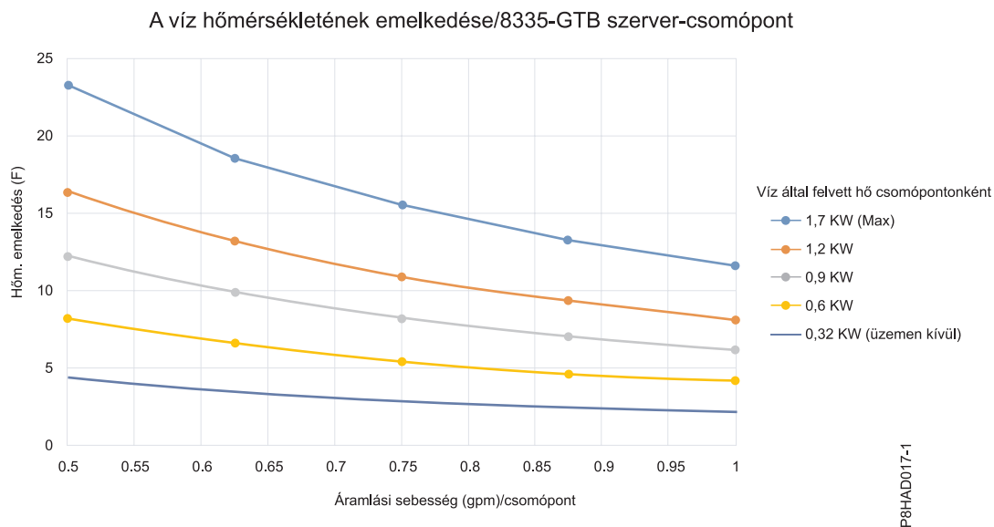
4. ábra: Vízáramlási sebesség a vízellátás hőmérsékletének függvényében - egyetlen szervert esetén (szabványos mértékegységek)
