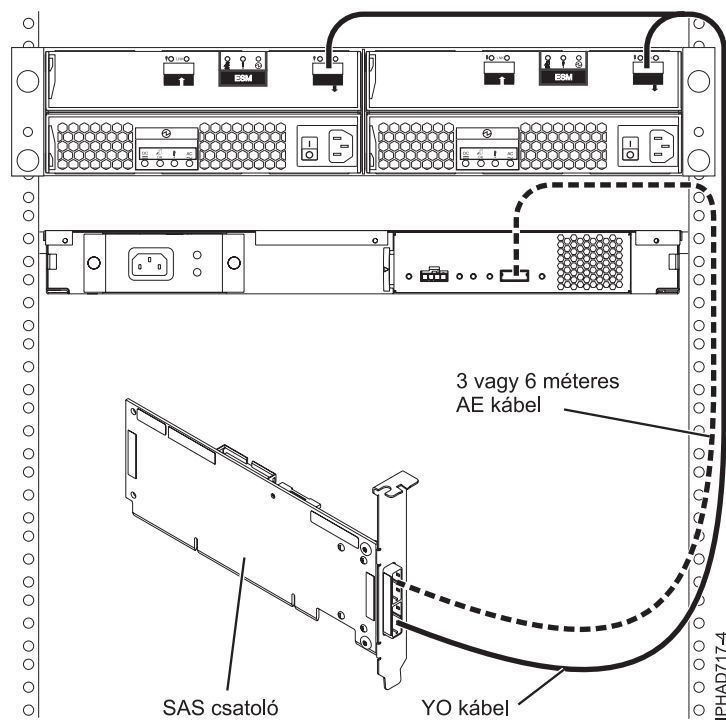
74. ábra: SAS csatoló összekapcsolása két lemez bővítőfiókkal és egy adathordozó bővítőfiókkal
