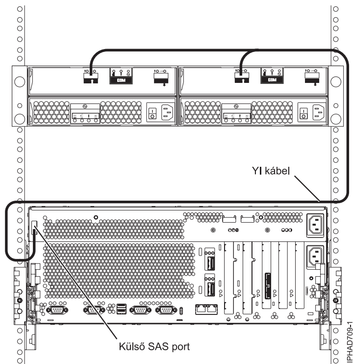
75. ábra: Külső SAS csatoló port összekapcsolása lemez bővítőfiókkal
