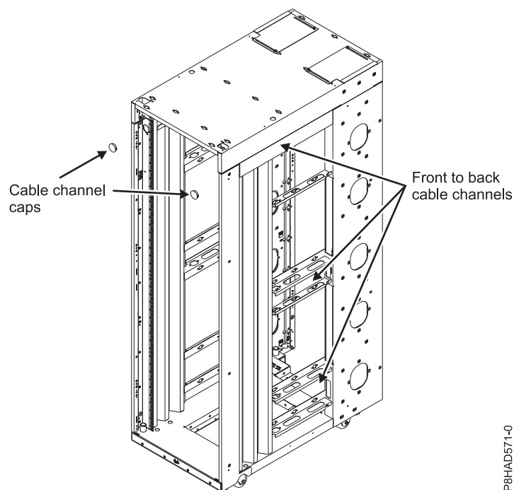
49. ábra: Kábelezés a rack szekrényen belül
