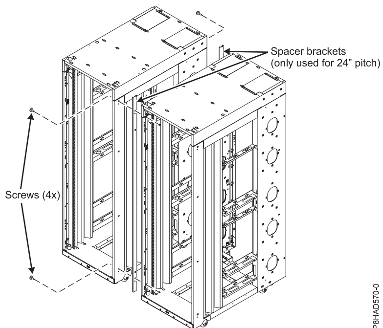
52. ábra: Több rack szekrény csatlakoztatása
