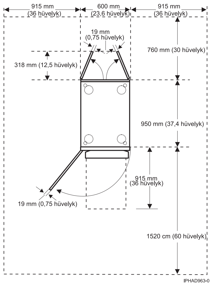
19. ábra: 0555 és 7014-S25 modell tervezési nézete
