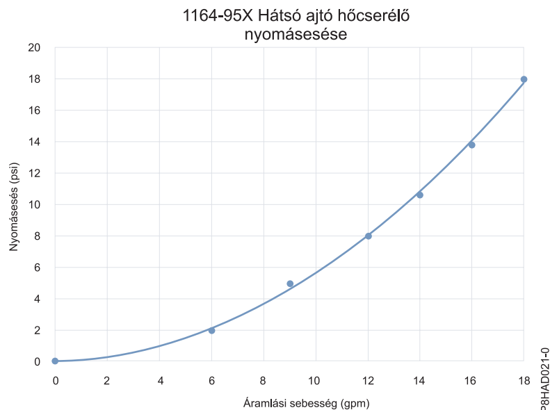
34. ábra: Nyomáscsökkentés (szabványos mértékegységek)
