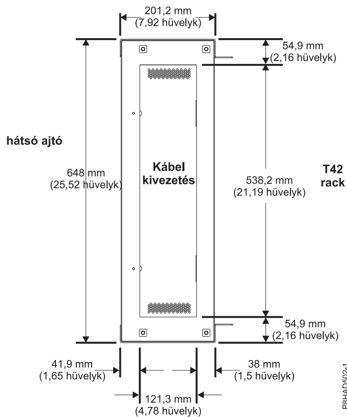
24. ábra: FC ERG0 hátulsó rack kiterjesztő (felülnézet)
