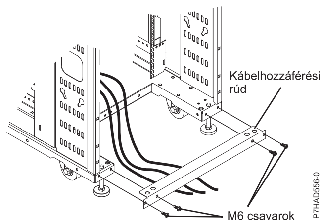
28. ábra: Kábelhozzáférési-rúd
