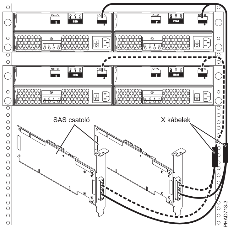
66. ábra: Két SAS RAID csatoló összekapcsolása két lemez bővítművel több kezdeményezős HA RAID konfigurációban
