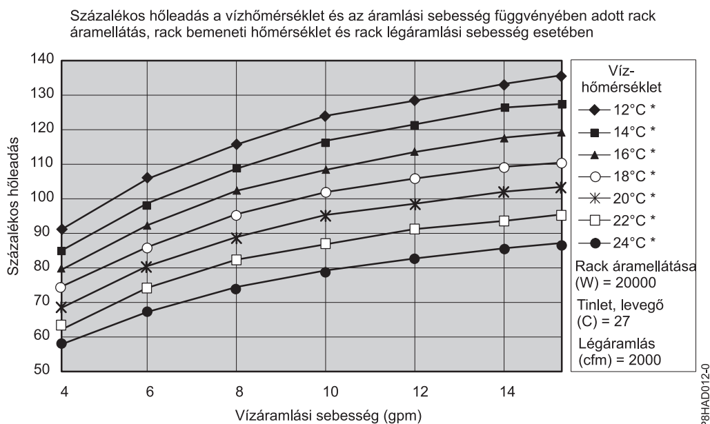
40. ábra: A hőcserélő tipikus teljesítménye, 20 kW hőterhelés
