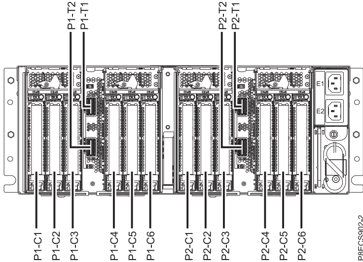
1. ábra: EMX0 PCIe3 bővítőfiók hátulnézete a PCIe bővítőhely elhelyezési kódjaival
