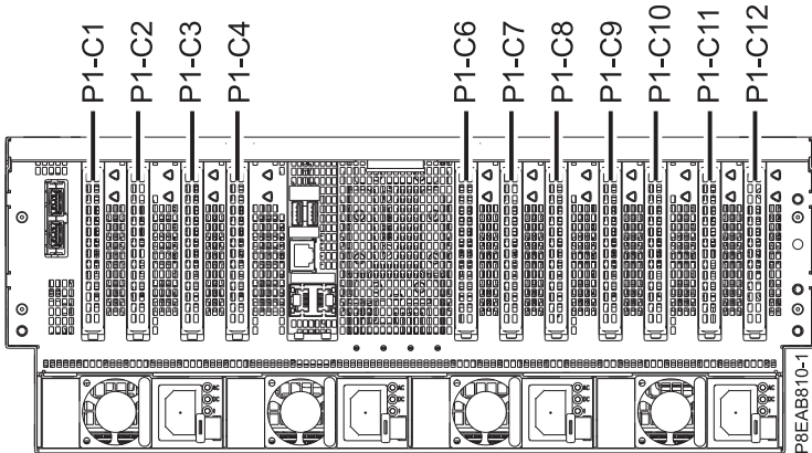
1. ábra: 8408-44E és 8408-E8E rendszer hátulnézete a PCIe bővítőhelyek elhelyezési kódjával
