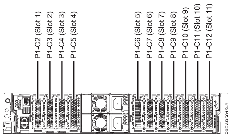
1. ábra: 5148-21L, 5148-22L, 8247-21L, 8247-22L, 8284-21A vagy 8284-22A rendszer hátulnézete PCIe bővítőhelyek elhelyezési kódjaival
