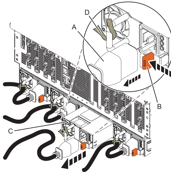
Abbildung 10. Ausbau eines Netzteils aus dem System vom Typ 8408-44E
