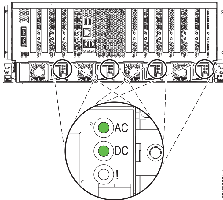
Abbildung 14. LEDs für ein funktionierendes Netzteil
