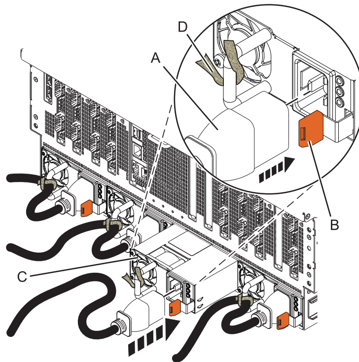
Abbildung 5. Austausch eines Netzteils im System vom Typ 8408-44E
