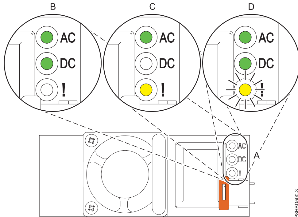
Abbildung 2. LEDs für ein funktionierendes und fehlerhaftes Netzteil
