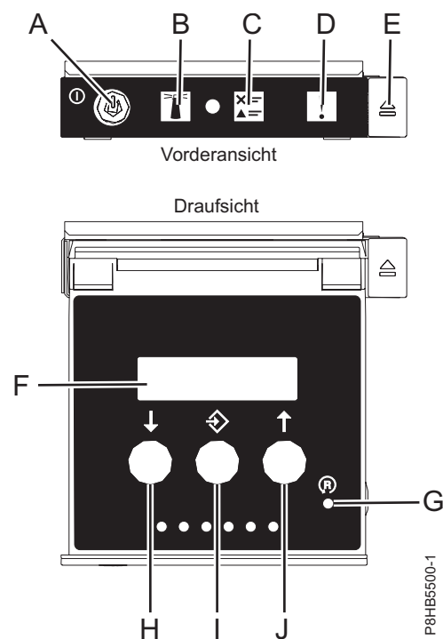
Abbildung 15. Anzeigen der Steuerkonsole
