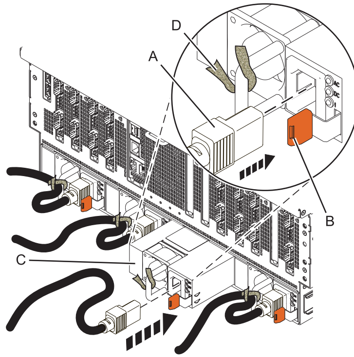
Abbildung 13. Austausch eines Netzteils im System vom Typ 8408-E8E
