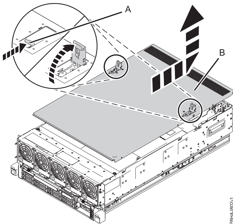
Abbildung 31. Serviceabdeckung ausbauen
