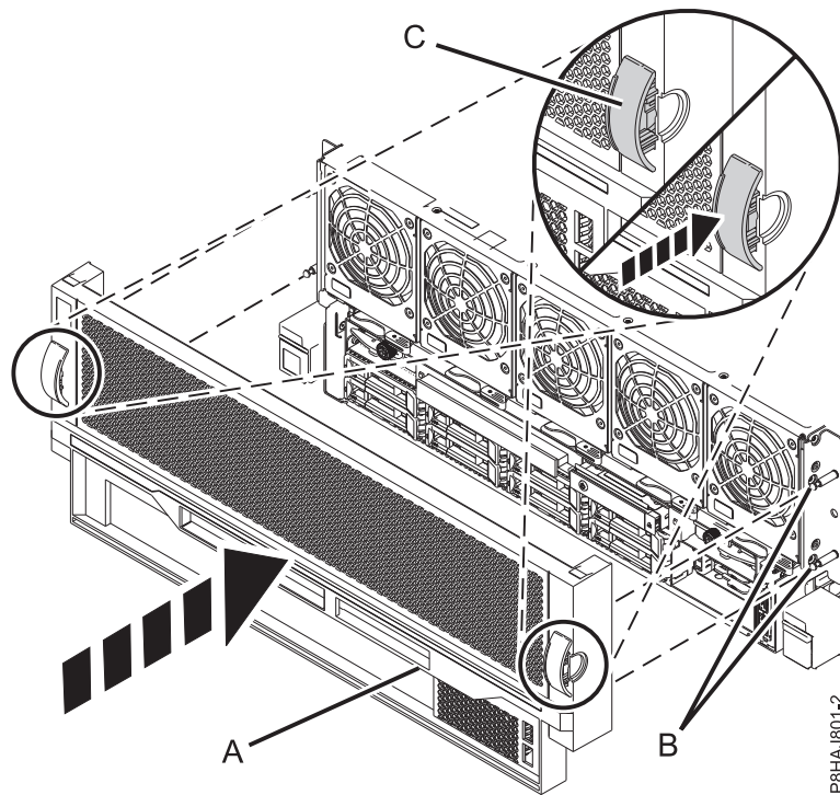
Abbildung 30. Vordere Abdeckung installieren
