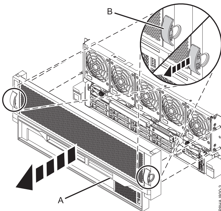
Abbildung 29. Vordere Abdeckung ausbauen
