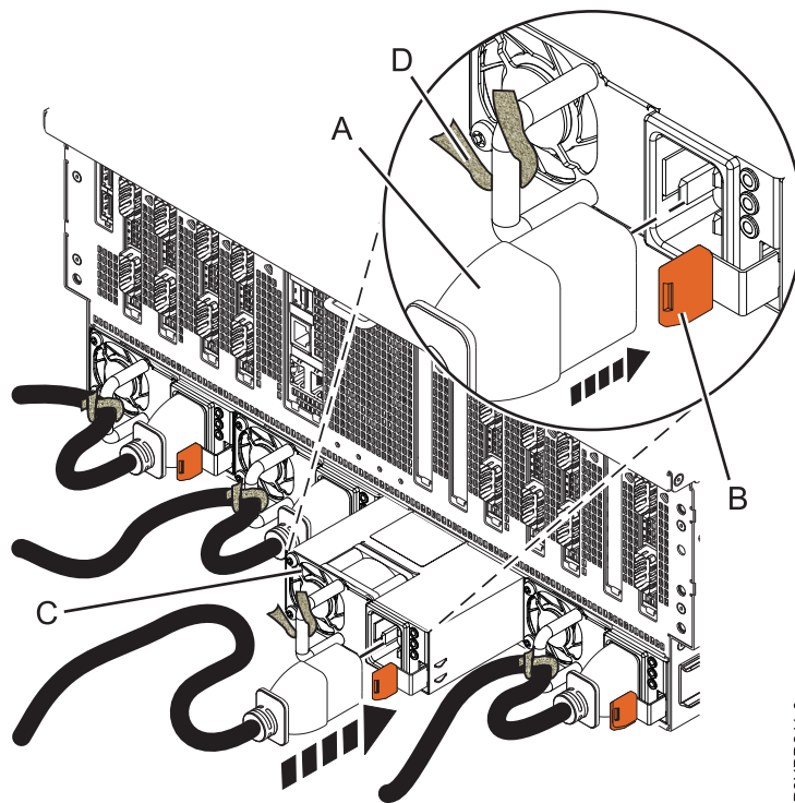
Abbildung 12. Austausch eines Netzteils im System vom Typ 8408-44E
