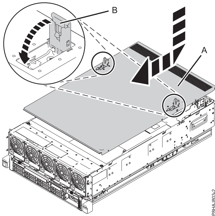
Abbildung 32. Serviceabdeckung installieren
