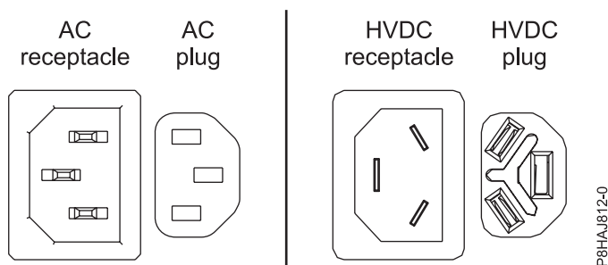
Abbildung 23. AC- und HVDC-Anschlüsse
