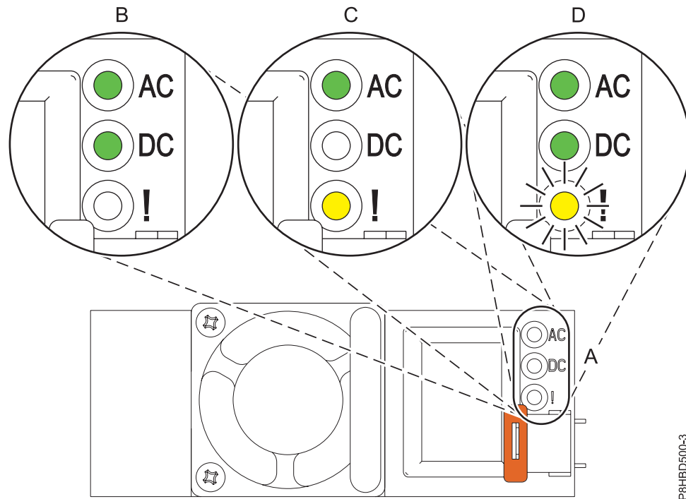
Abbildung 9. LEDs für ein funktionierendes und fehlerhaftes Netzteil
