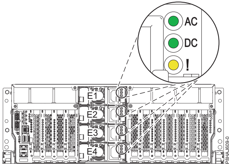
Abbildung 1. Position der Netzteile und Anzeigen in einem Einschubsystem
