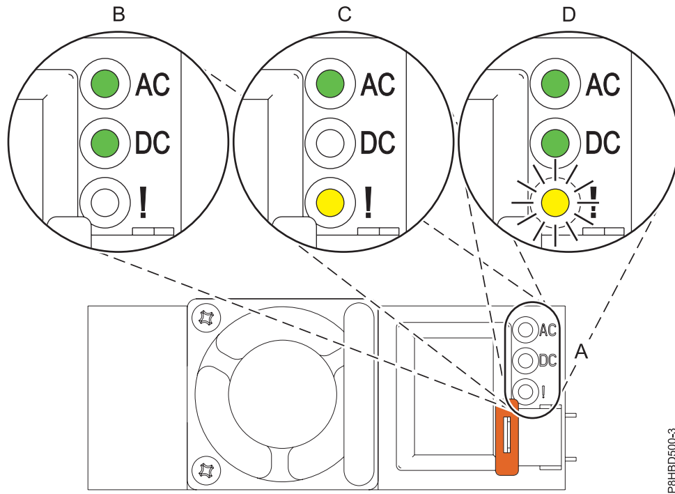
Abbildung 15. Anzeigen für ein funktionierendes und fehlerhaftes Netzteil in einem Einschubsystem
