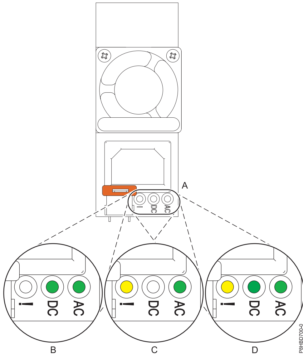
Abbildung 16. Anzeigen für ein funktionierendes und fehlerhaftes Netzteil in einem eigenständigen System
