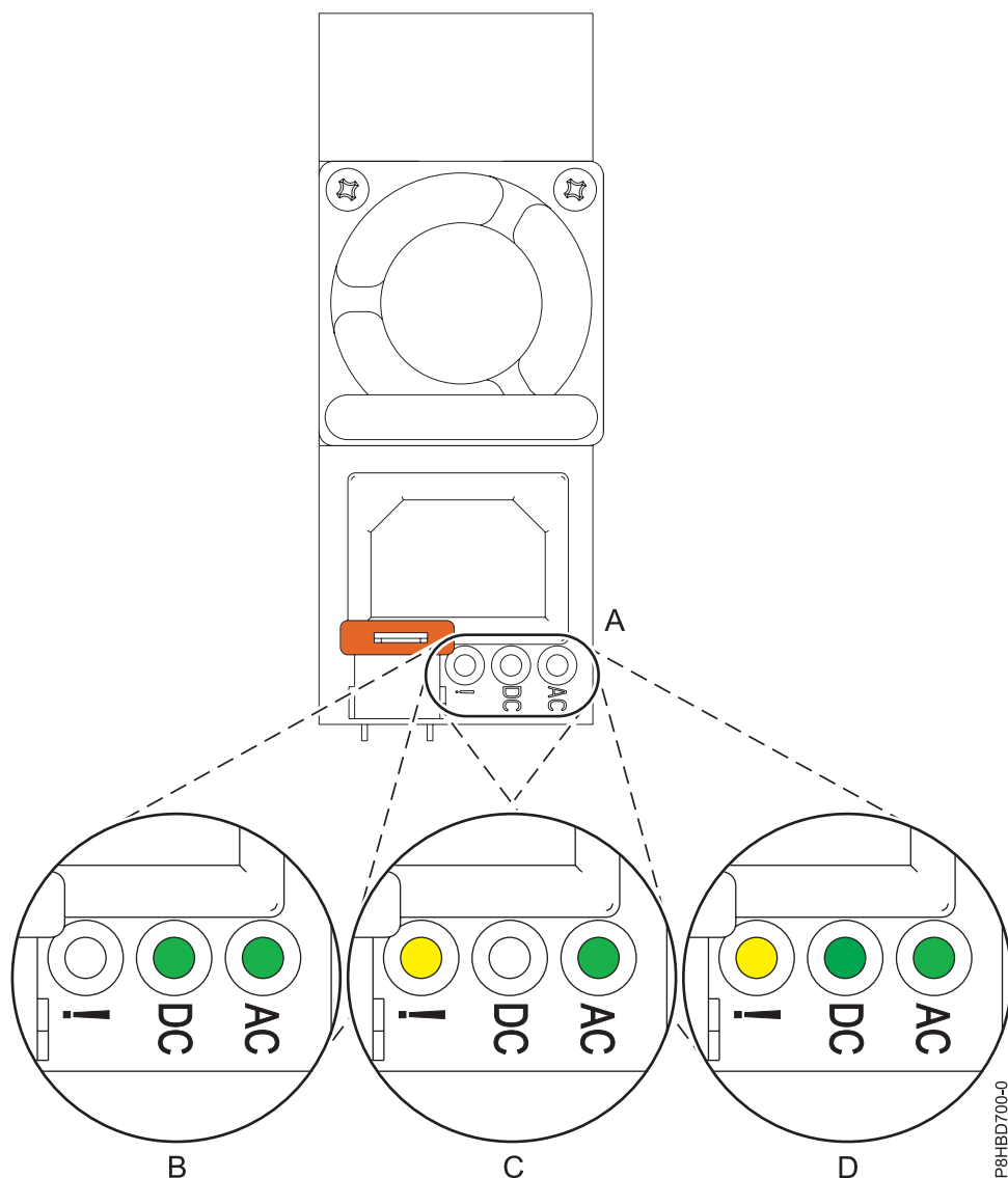
Abbildung 12. Anzeigen für ein funktionierendes und fehlerhaftes Netzteil in einem eigenständigen System
