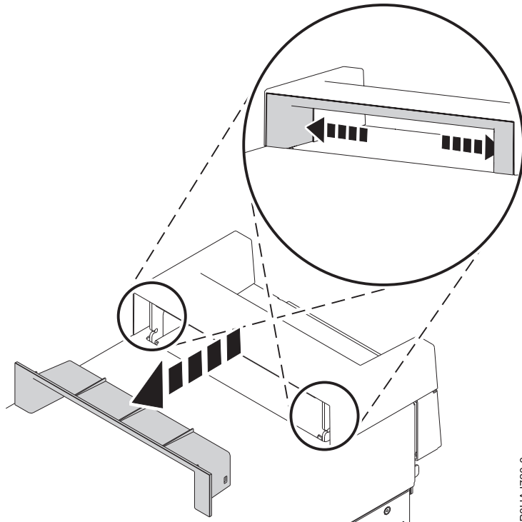
Abbildung 42. Entfernen des Elements innerhalb der Griffabdeckung bei einem Standalone-System vom Typ 8286-41A
