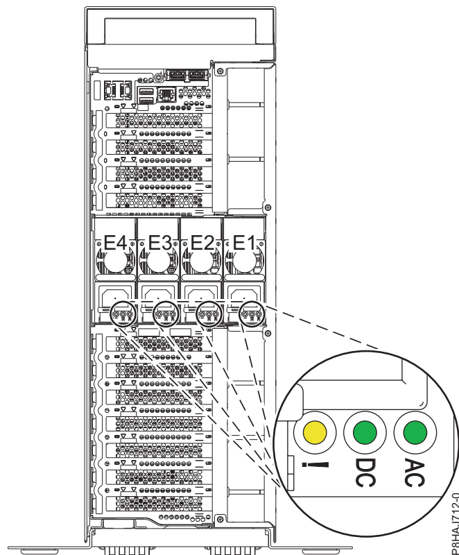
Abbildung 2. Position der Netzteile und Anzeigen in einem eigenständigen System
