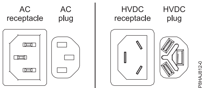
Abbildung 27. AC- und HVDC-Anschlüsse
