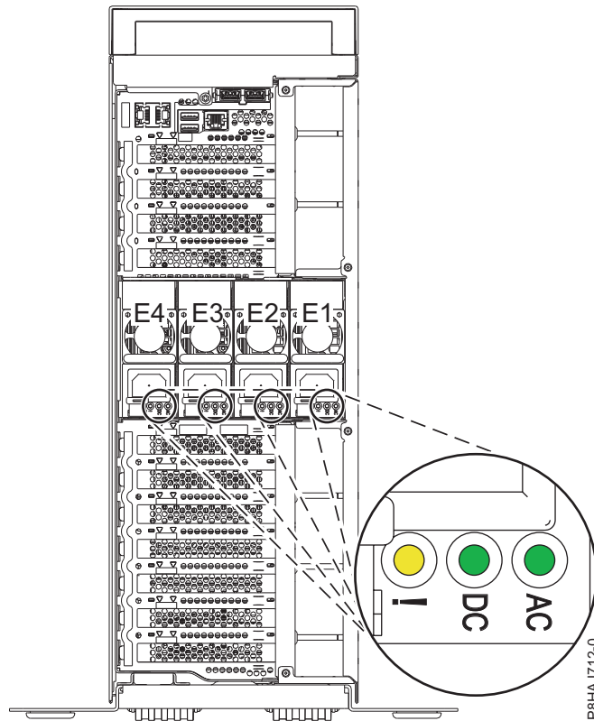
Abbildung 14. Position der Netzteile und Anzeigen in einem eigenständigen System
