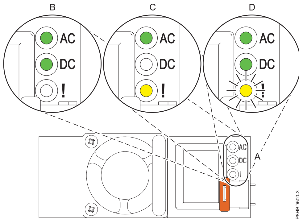
Abbildung 3. Anzeigen für ein funktionierendes und fehlerhaftes Netzteil in einem Einschubsystem
