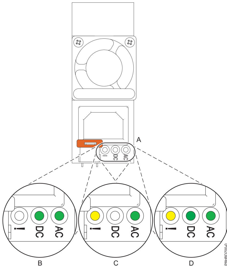
Abbildung 18. Anzeigen für ein funktionierendes und fehlerhaftes Netzteil in einem eigenständigen System
