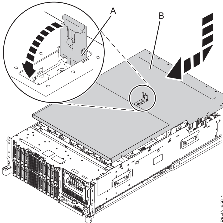
Abbildung 56. Serviceabdeckung installieren
