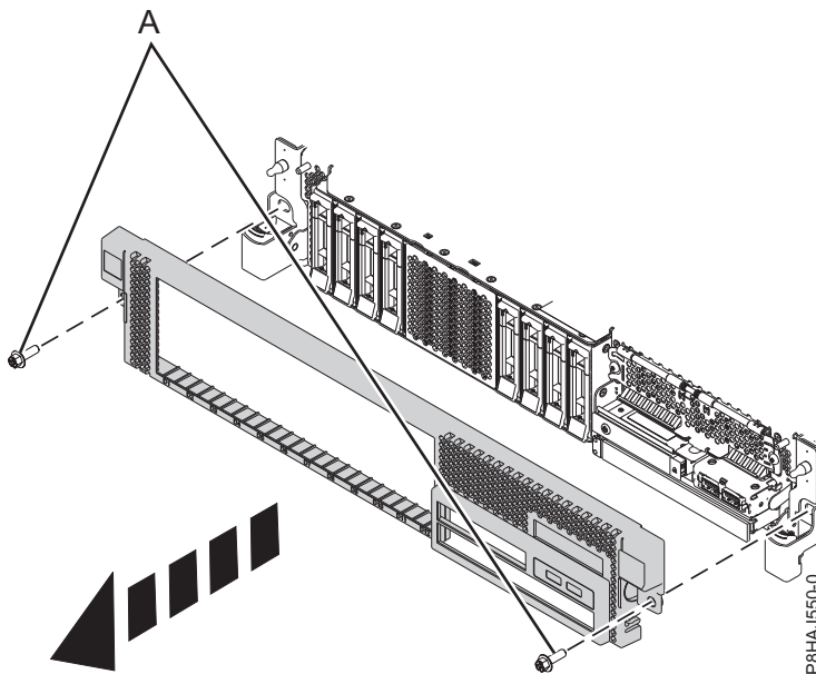
Abbildung 39. Vordere Abdeckung ausbauen
