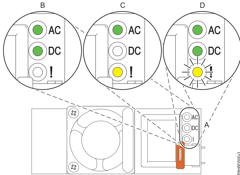
Abbildung 23. Anzeigen für ein funktionierendes und fehlerhaftes Netzteil in einem Einschubsystem
