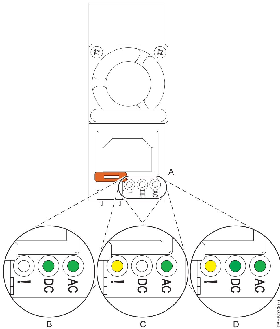
Abbildung 24. Anzeigen für ein funktionierendes und fehlerhaftes Netzteil in einem eigenständigen System
