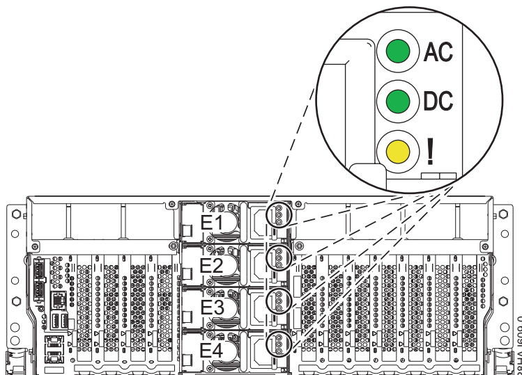
Abbildung 13. Position der Netzteile und Anzeigen in einem Einschubsystem
