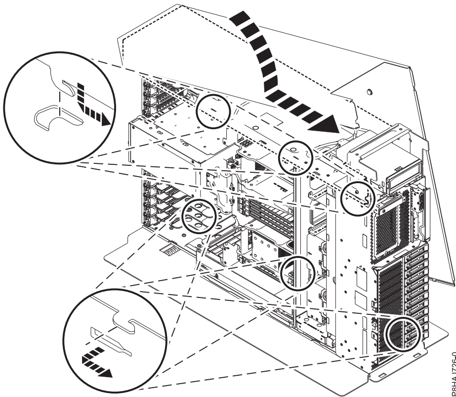
Abbildung 52. Installieren der Seitenabdeckung bei einem Standalone-System vom Typ 8286-41A
