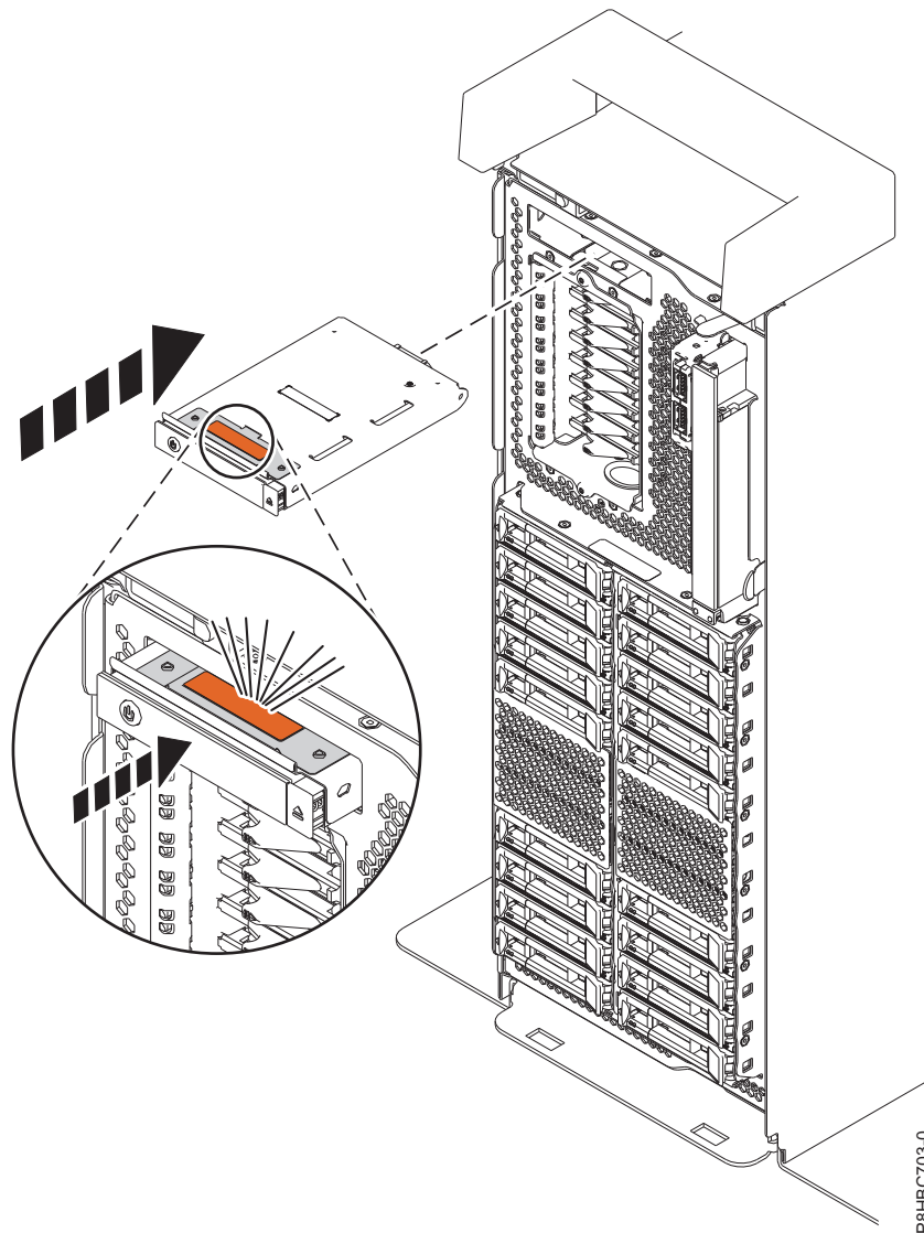
Abbildung 9. Steuerkonsole bei einem eigenständigen System austauschen
