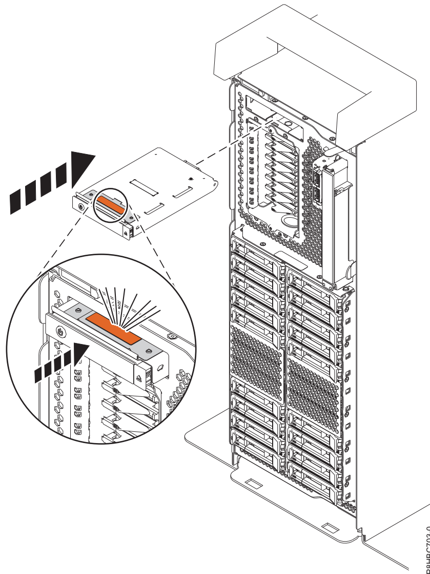
Abbildung 4. Steuerkonsole bei einem eigenständigen System austauschen
