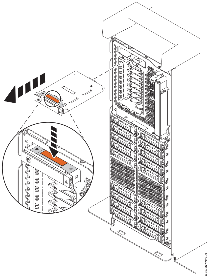
Abbildung 7. Steuerkonsole ausbauen - Eigenständiges System
