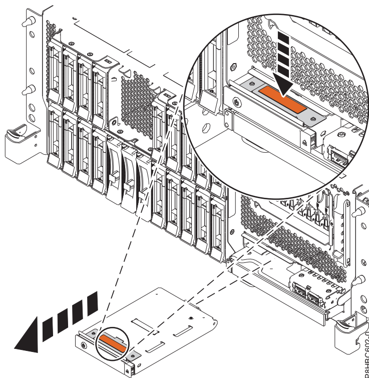
Abbildung 6. Steuerkonsole ausbauen - Einschubsystem
