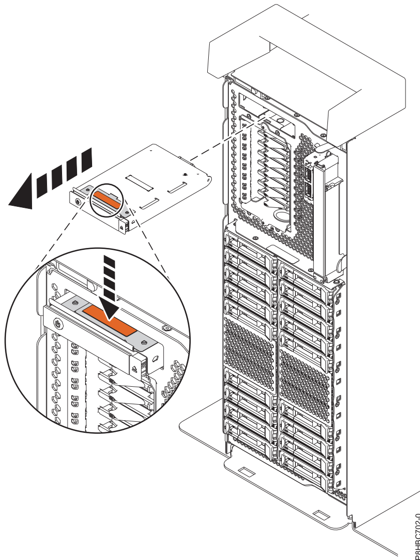
Abbildung 2. Steuerkonsole ausbauen - Eigenständiges System
