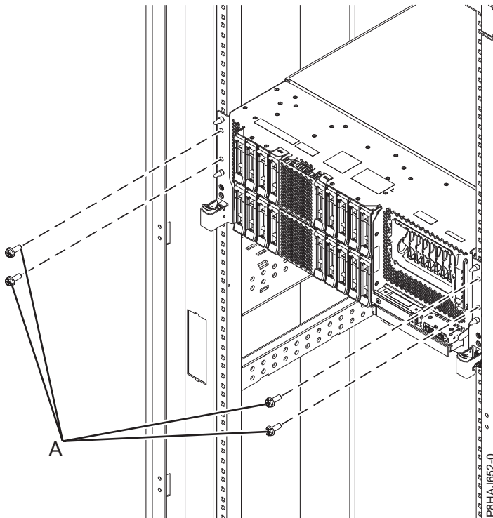
Abbildung 35. Entfernen der vorderen Schrauben
