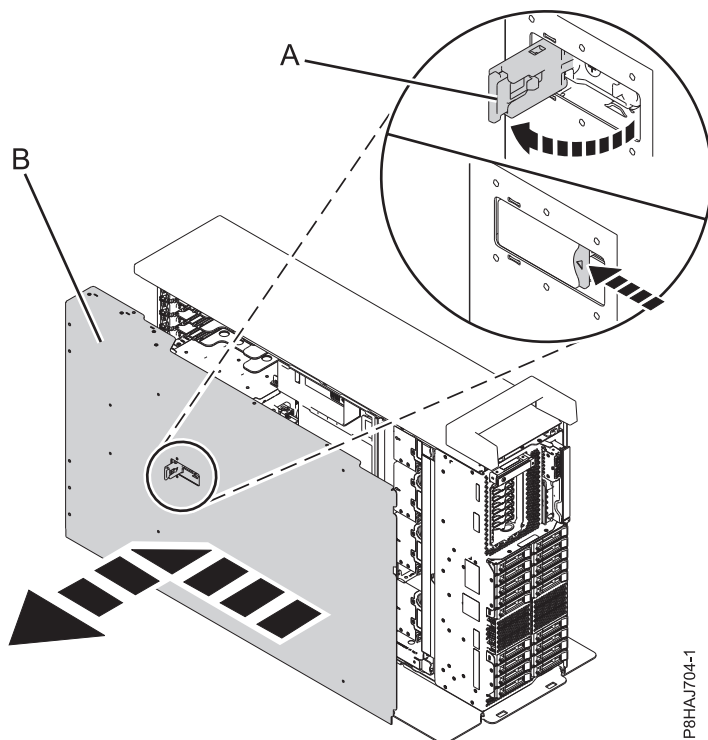
Abbildung 28. Serviceabdeckung ausbauen
