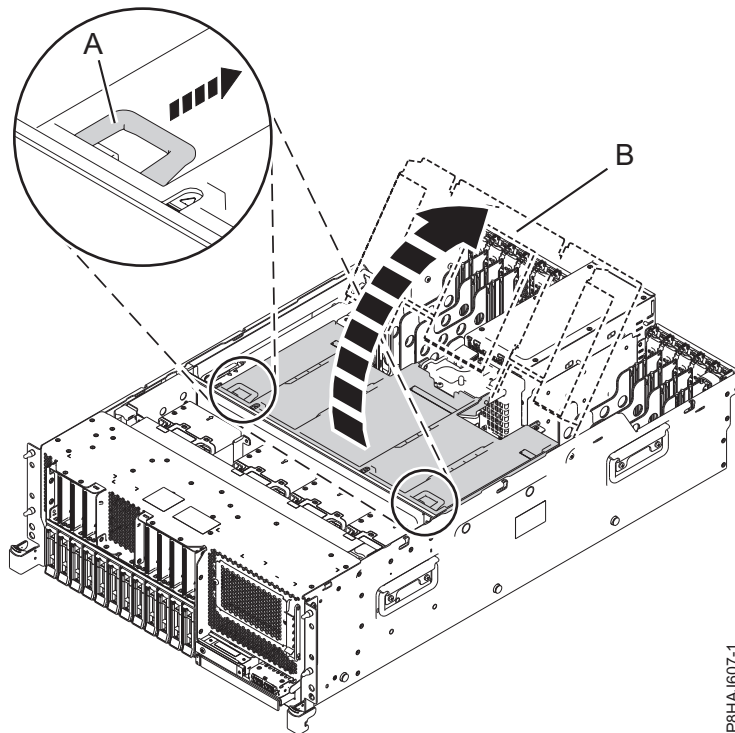
Abbildung 31. Öffnen der Luftführung
