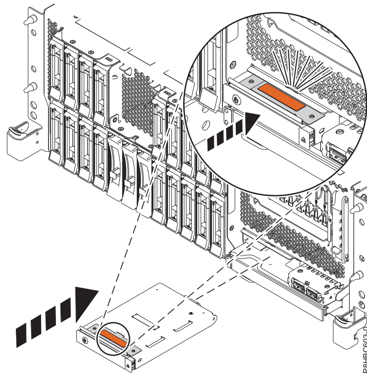
Abbildung 8. Austauschen der Steuerkonsole in einem Einschubsystem
