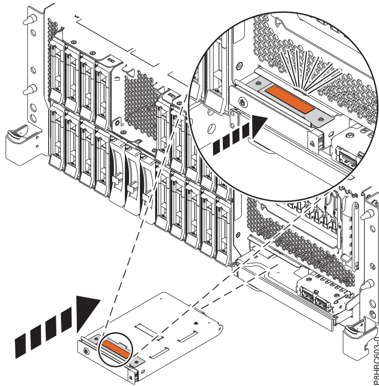
Abbildung 3. Austauschen der Steuerkonsole in einem Einschubsystem
