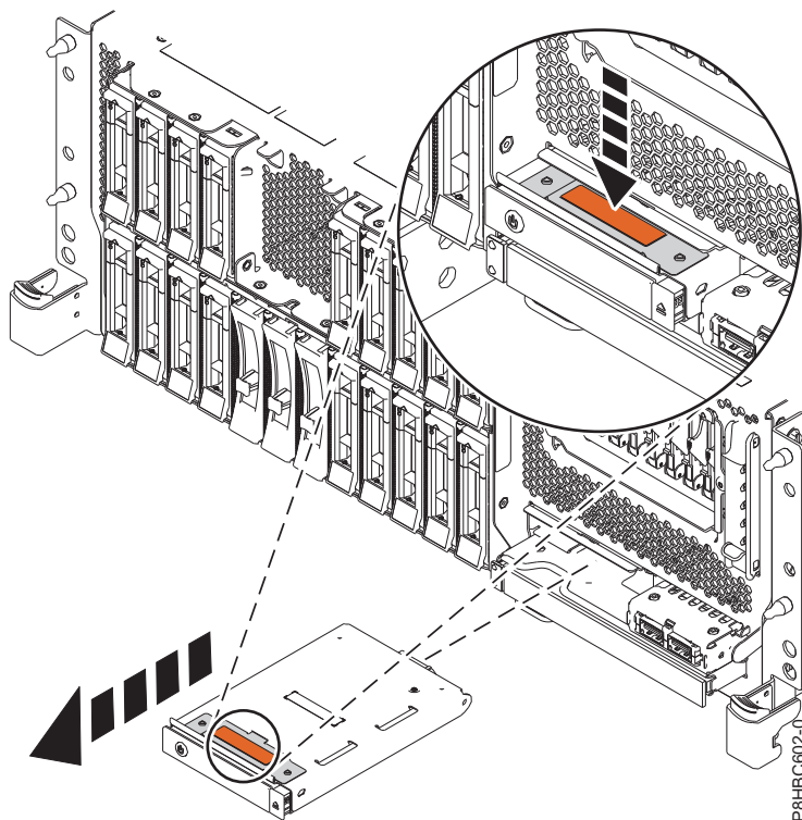
Abbildung 1. Steuerkonsole ausbauen - Einschubsystem
