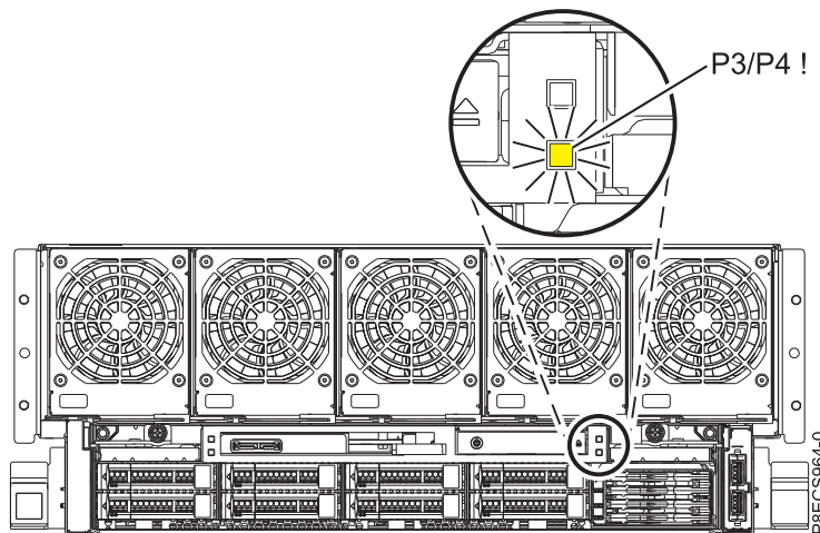
Abbildung 4. Vordere Gehäusefehleranzeige P3/P4 ! an der Vorderseite des Systems vom Typ 8408-44E oder 8408-E8E.
