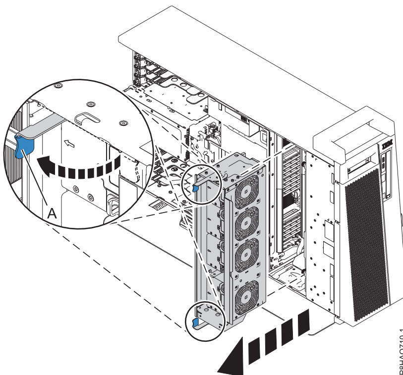
Abbildung 8. Lüfterrahmen ausbauen - Standalone-System
