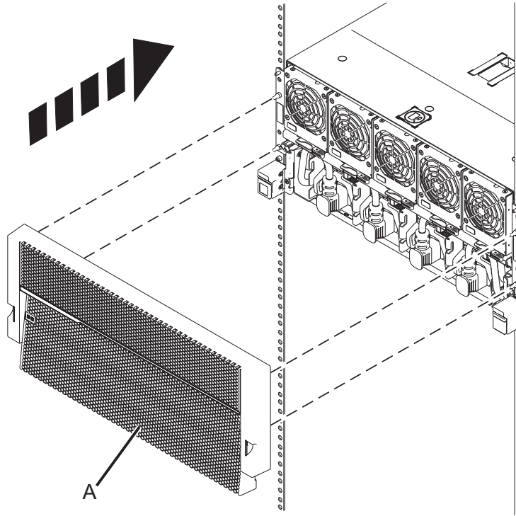
Abbildung 46. Vordere Abdeckung installieren
