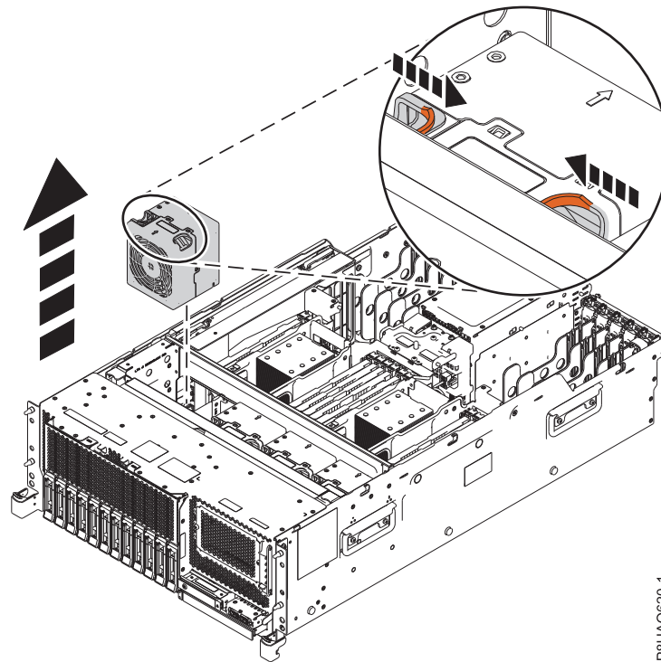
Abbildung 3. Lüfter ausbauen - Einschubsystem
