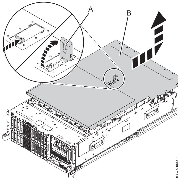
Abbildung 28. Serviceabdeckung ausbauen
