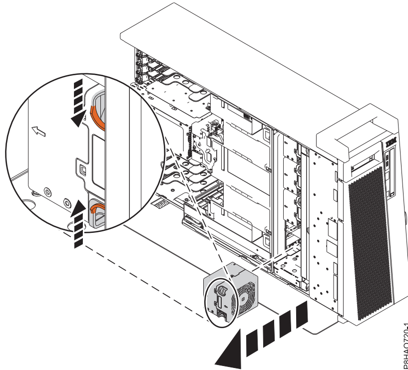
Abbildung 4. Lüfter ausbauen - Standalone-System
