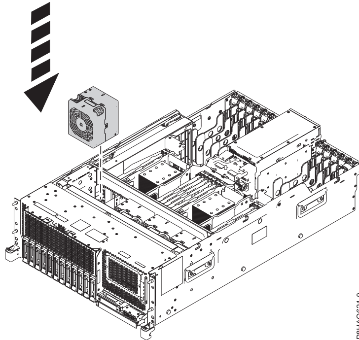
Abbildung 5. Lüfter austauschen - Einschubsystem
