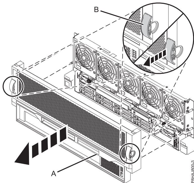
Abbildung 36. Vordere Abdeckung ausbauen
