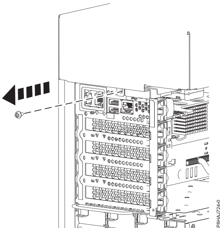
Abbildung 18. Entfernen der Schraube der Seitenabdeckung bei einem Standalone-System vom Typ 8286-41A
