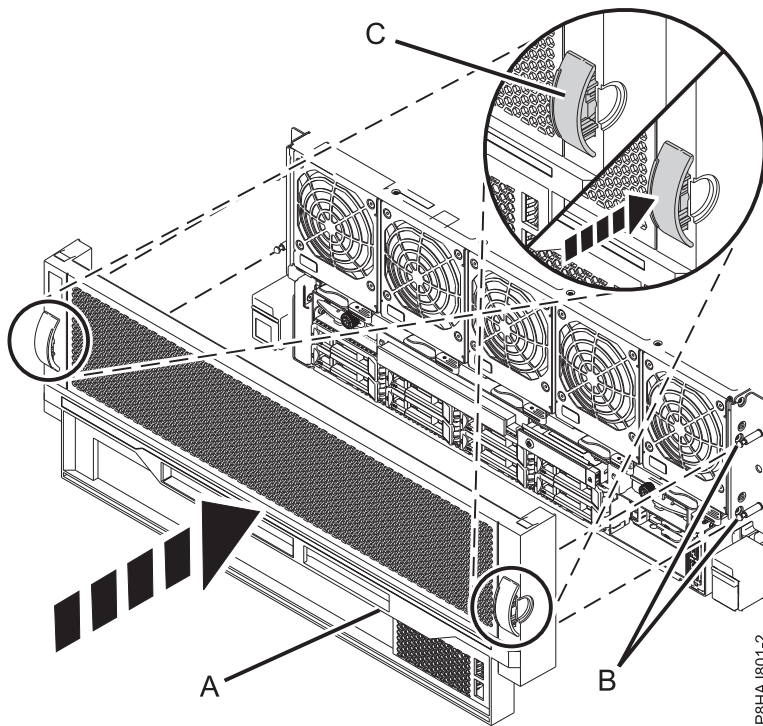
Abbildung 37. Vordere Abdeckung installieren
