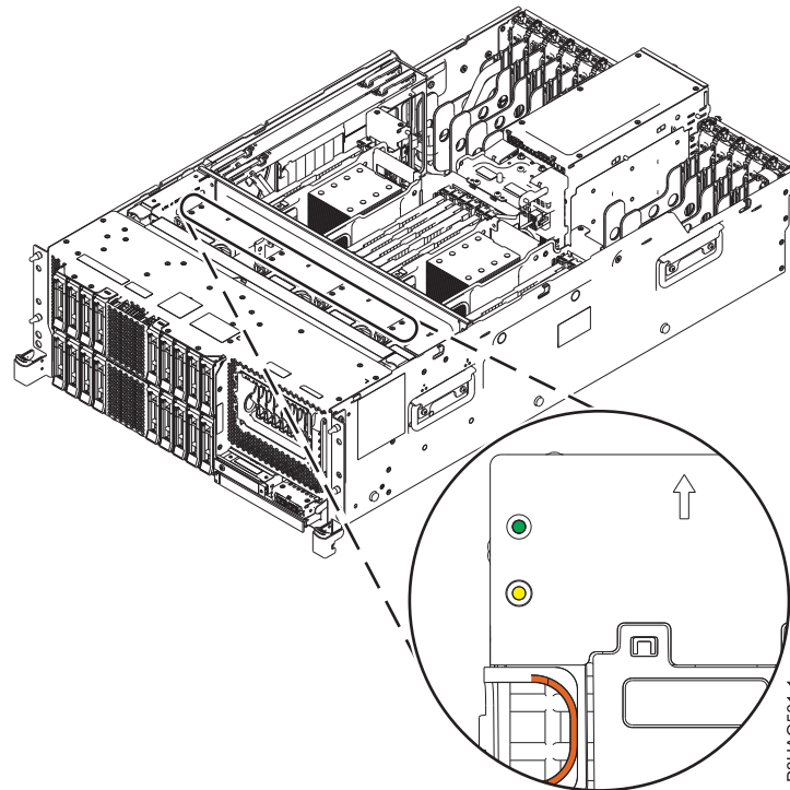
Abbildung 1. Anzeigen am Lüfterrahmen für die AMDs in einem Einschubsystem
