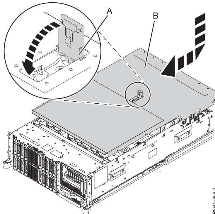
Abbildung 30. Serviceabdeckung installieren
