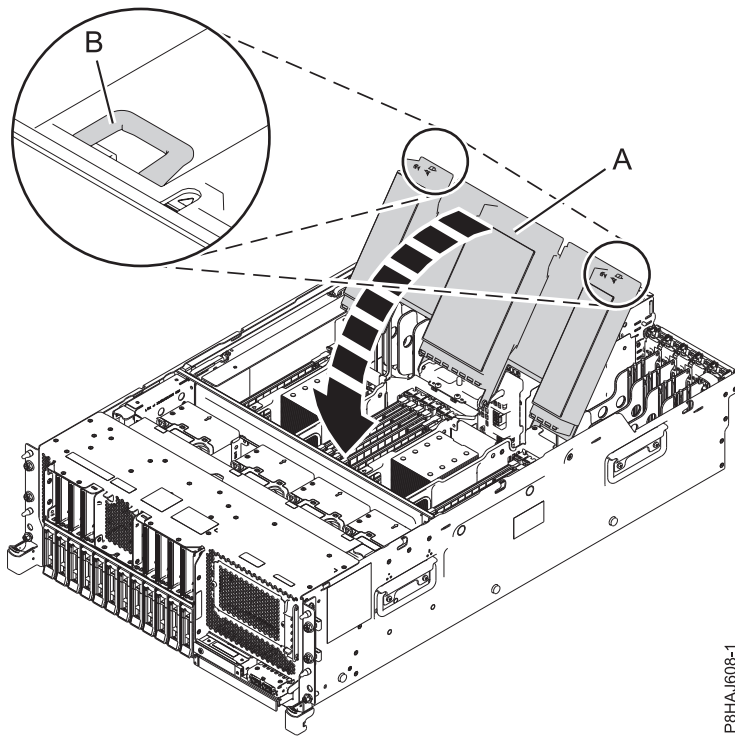
Abbildung 33. Schließen der Luftführung
