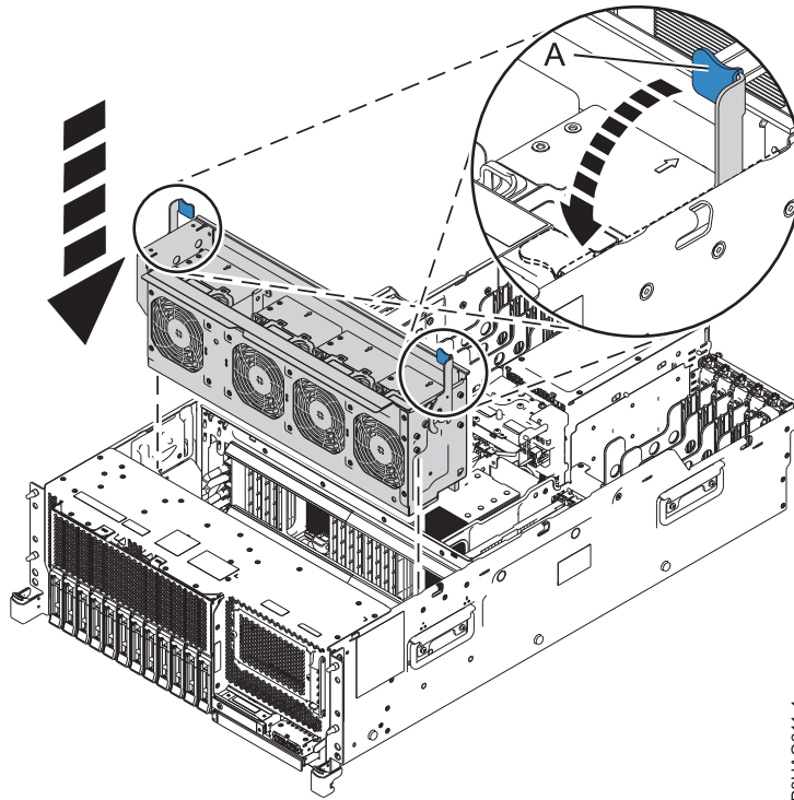
Abbildung 9. Lüfterrahmen austauschen - Einschubsystem
