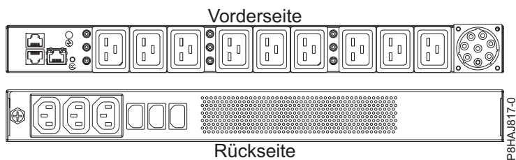
Abbildung 55. PDU beim System vom Typ 8408-44E
