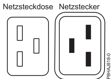
Abbildung 54. Anschlüsse beim System vom Typ 8408-44E
