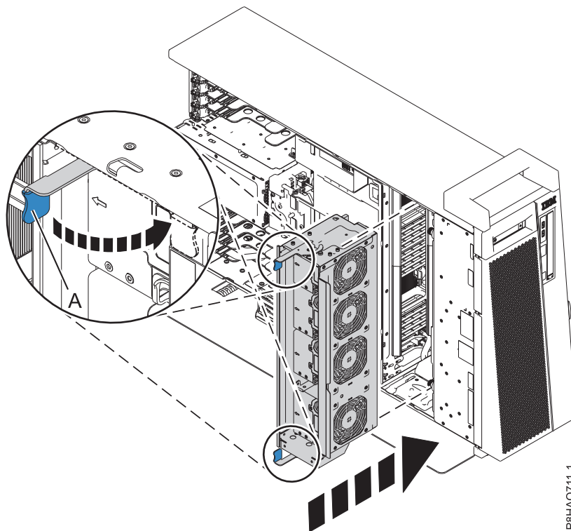
Abbildung 10. Lüfterrahmen austauschen - Standalone-System
