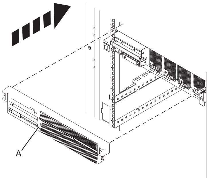
Abbildung 47. Vordere Abdeckung des Systemcontrollers installieren
