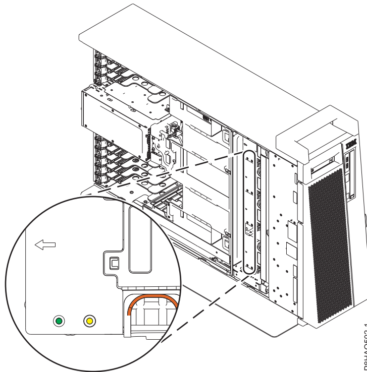
Abbildung 2. Anzeigen am Lüfterrahmen für die AMDs in einem Standalone-System
