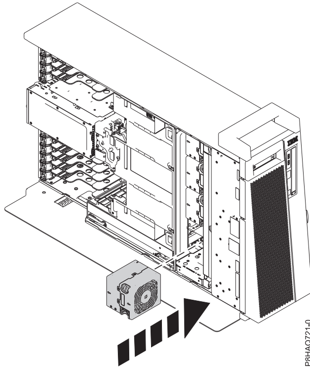
Abbildung 6. Lüfter austauschen - Standalone-System
