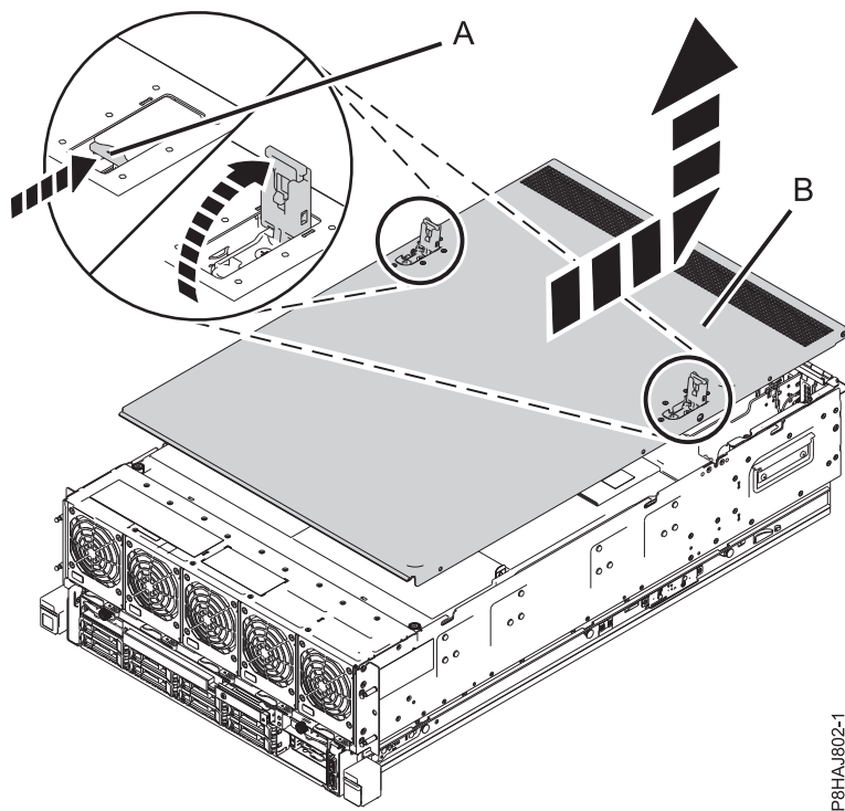
Abbildung 38. Serviceabdeckung ausbauen
