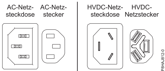
Abbildung 53. AC- und HVDC-Anschlüsse
