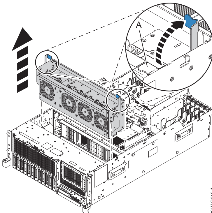
Abbildung 7. Lüfterrahmen ausbauen - Einschubsystem
