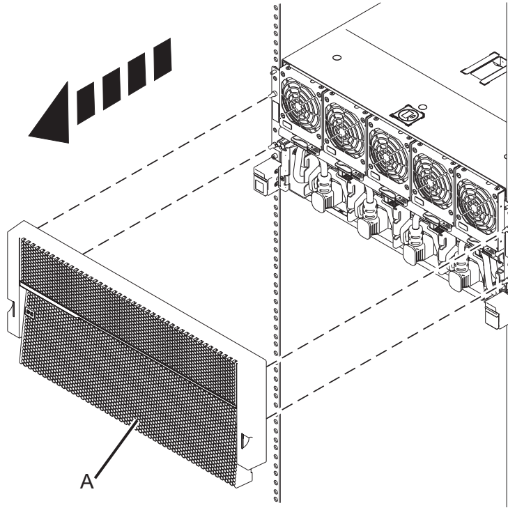
Abbildung 44. Vordere Abdeckung ausbauen
