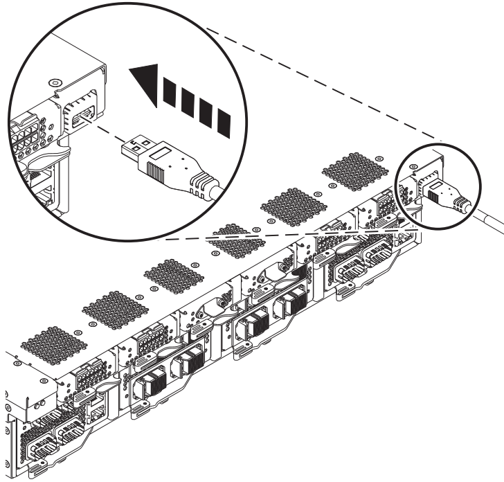
Abbildung 8. Verbinden Sie das USB-Kabel mit dem USB-Anschluss auf der Rückseite des Systemcontrollers vom Typ 9080-MHE, 9080-MME, 9119-MHE oder 9119-MME am Steckplatz P1-C11-T1.
