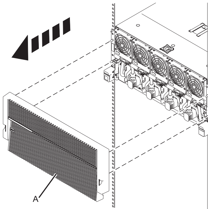
Abbildung 14. Vordere Abdeckung ausbauen
