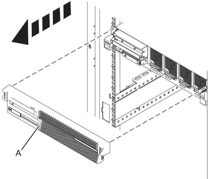
Abbildung 15. Vordere Abdeckung des Systemcontrollers ausbauen
