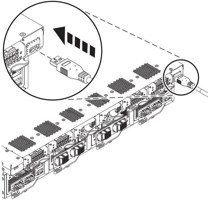
Abbildung 4. Verbinden Sie das USB-Kabel mit dem USB-Anschluss auf der Rückseite des Systemcontrollers vom Typ 9080-MHE, 9080-MME, 9119-MHE oder 9119-MME am Steckplatz P1-C11-T1.
