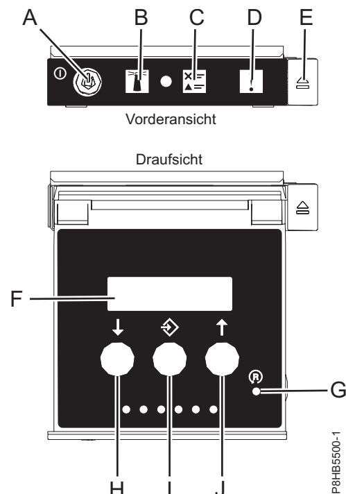
Abbildung 13. Steuerkonsole
