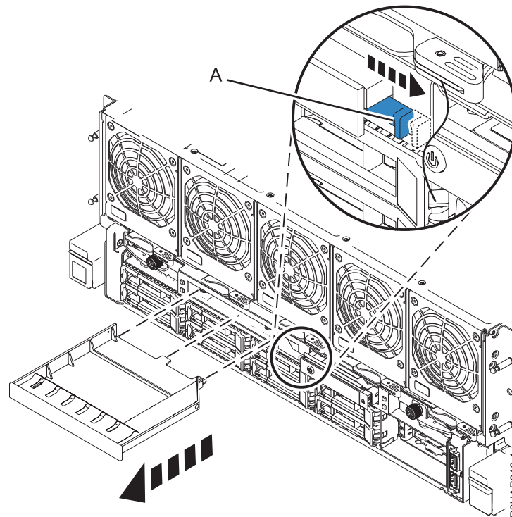
Abbildung 5. Entfernen Sie die Abdeckblende der Einheit für austauschbare Datenträger aus dem System.
