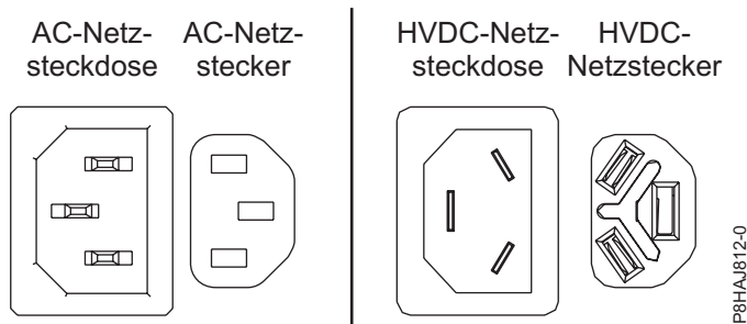
Abbildung 26. AC- und HVDC-Anschlüsse
