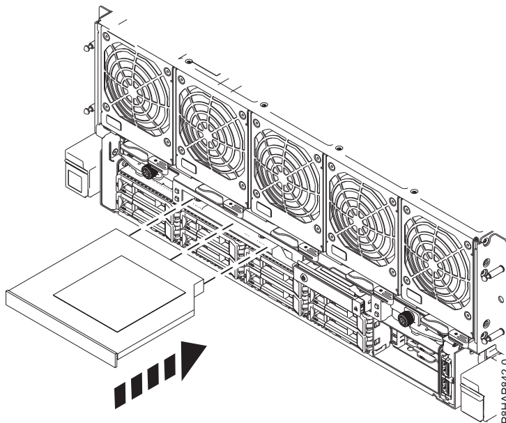
Abbildung 4. DVD-Laufwerk im System installieren
