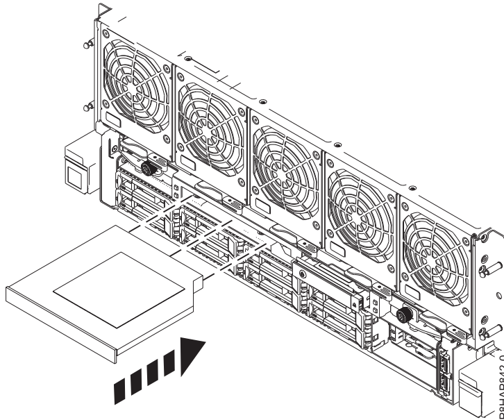
Abbildung 6. DVD-Laufwerk im System installieren
