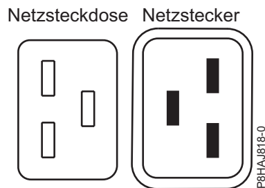
Abbildung 27. Anschlüsse beim System vom Typ 8408-44E
