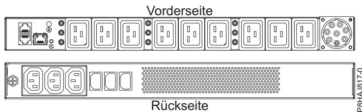
Abbildung 28. PDU beim System vom Typ 8408-44E
