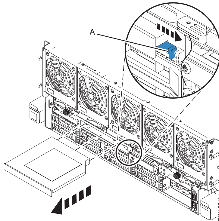
Abbildung 11. DVD-Laufwerk aus dem System ausbauen
