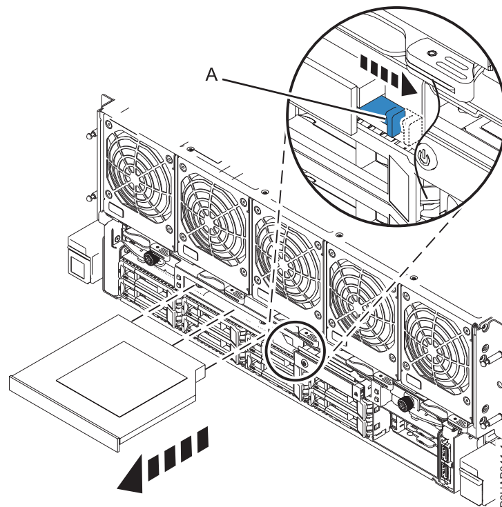
Abbildung 9. DVD-Laufwerk aus dem System ausbauen
