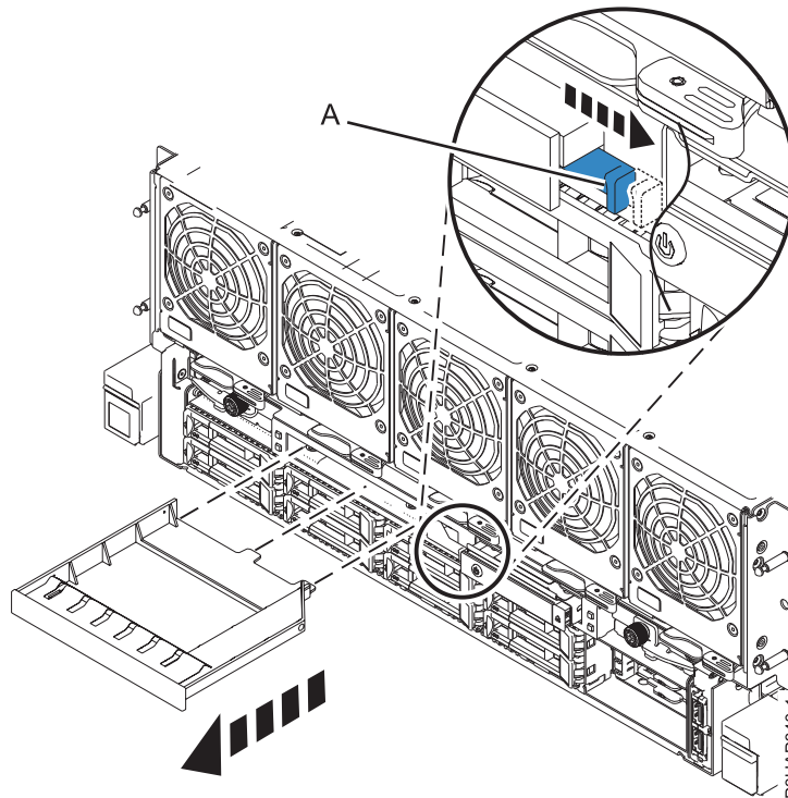
Abbildung 1. Entfernen Sie die Abdeckblende der Einheit für austauschbare Datenträger aus dem System.
