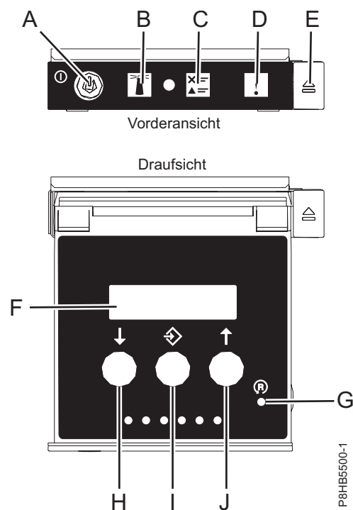
Abbildung 14. Anzeigen der Steuerkonsole
