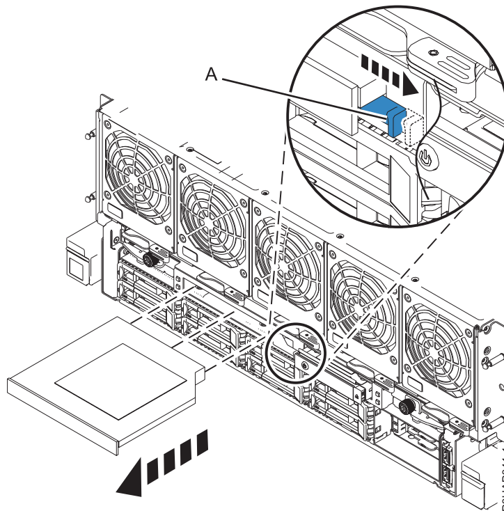
Abbildung 7. DVD-Laufwerk aus dem System ausbauen
