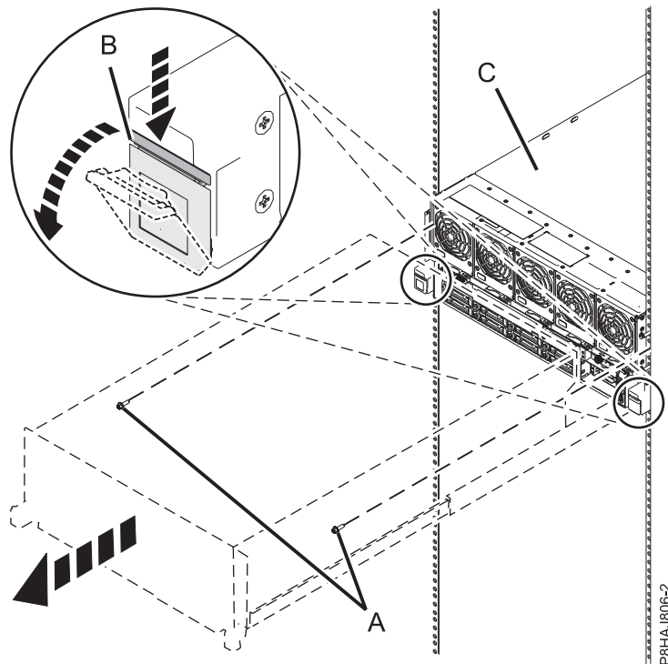
Abbildung 24. System in Serviceposition bringen
