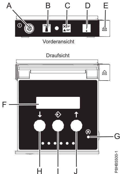
Abbildung 15. Steuerkonsole
