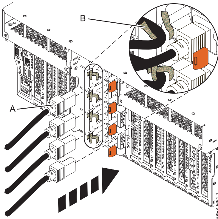
Abbildung 35. Netzkabel an ein System vom Typ 8247-42L, 8286-41A oder 8286-42A anschließen
