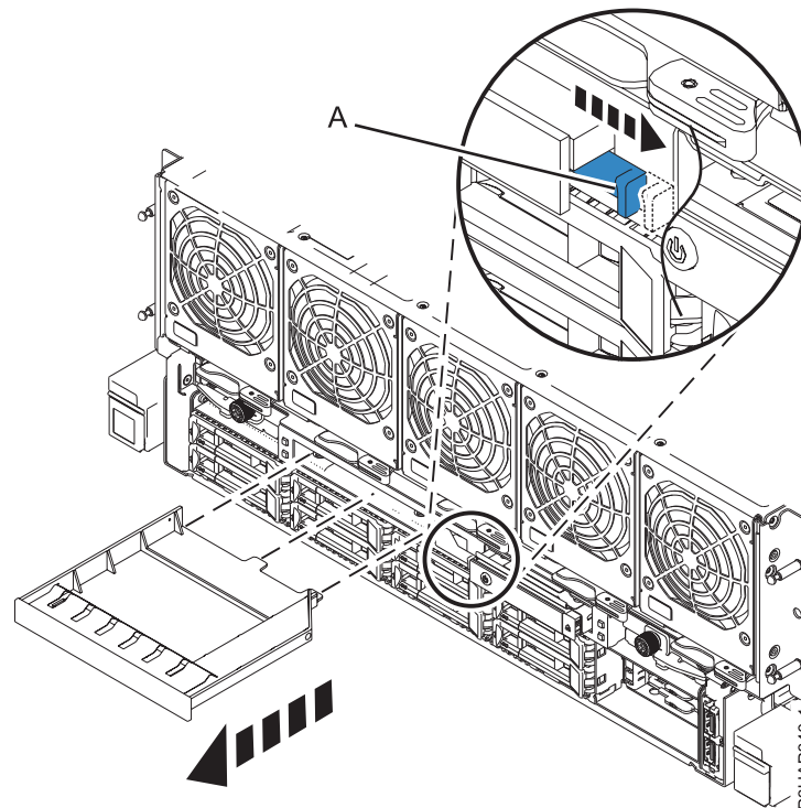
Abbildung 3. Entfernen Sie die Abdeckblende der Einheit für austauschbare Datenträger aus dem System.
