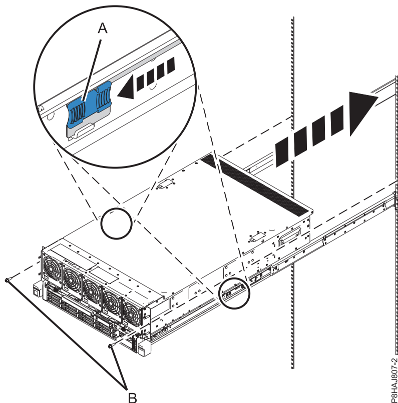
Abbildung 25. System in die Betriebsposition bringen
