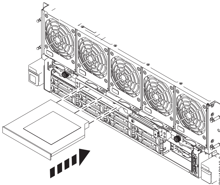
Abbildung 12. DVD-Laufwerk im System installieren
