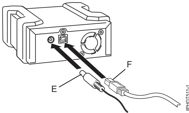
Abbildung 13. USB-Kabel und Netzkabel anschließen
