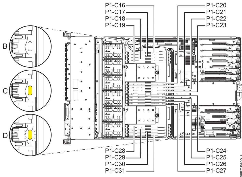
Abbildung 10. Steckreihenfolge der Speichermodule
