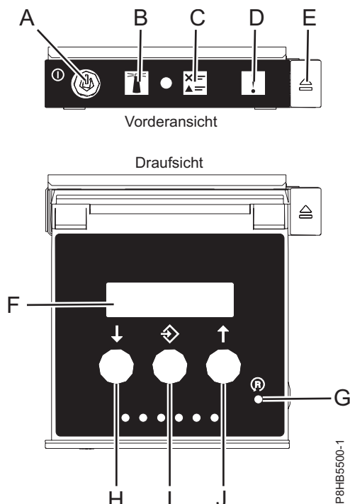
Abbildung 12. Steuerkonsole
