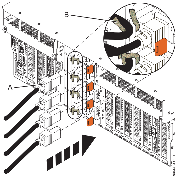
Abbildung 22. Netzkabel bei einem System vom Typ 8247-42L, 8286-41A oder 8286-42A anschließen
