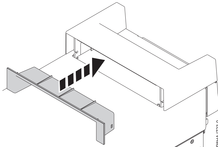
Abbildung 37. Einsetzen des Elements innerhalb der Griffabdeckung bei einem Standalone-System vom Typ 8286-41A
