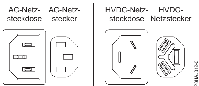
Abbildung 13. AC- und HVDC-Anschlüsse
