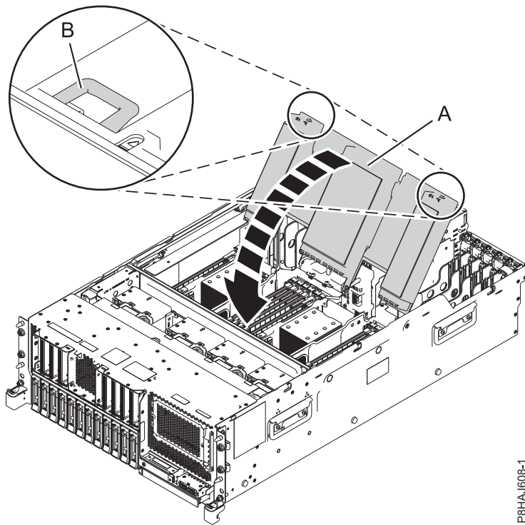
Abbildung 45. Schließen der Luftführung
