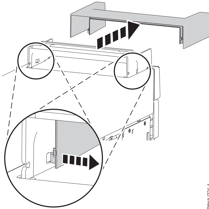
Abbildung 29. Ausbauen der Griffabdeckung bei einem Standalone-System vom Typ 8286-41A
