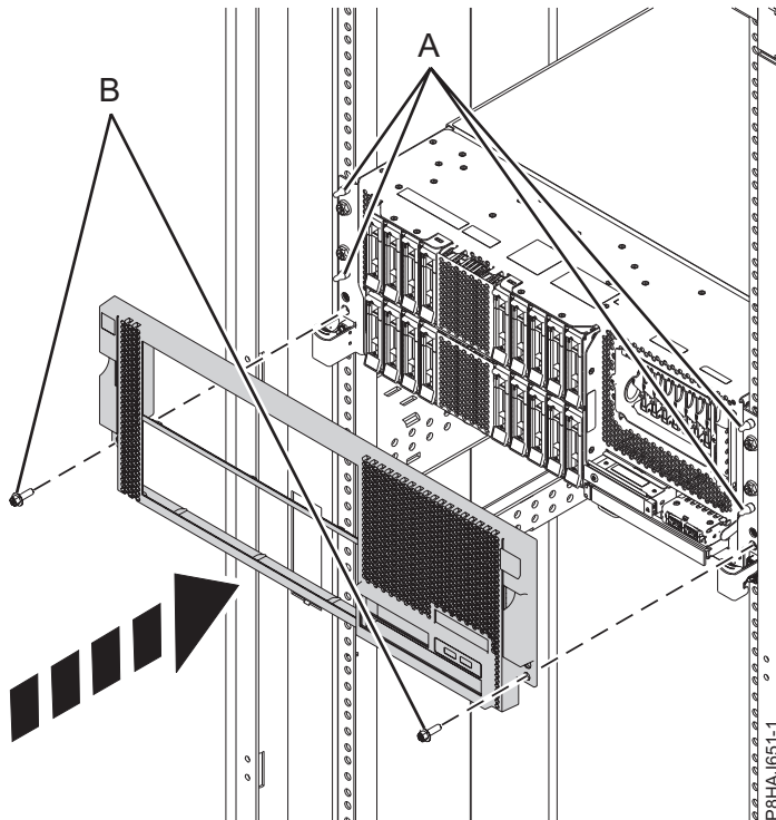
Abbildung 33. Vordere Abdeckung installieren
