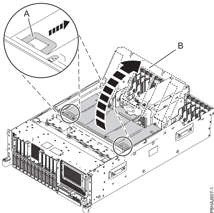
Abbildung 44. Öffnen der Luftführung
