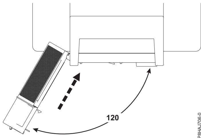
Abbildung 35. Drehen der vorderen Abdeckung
