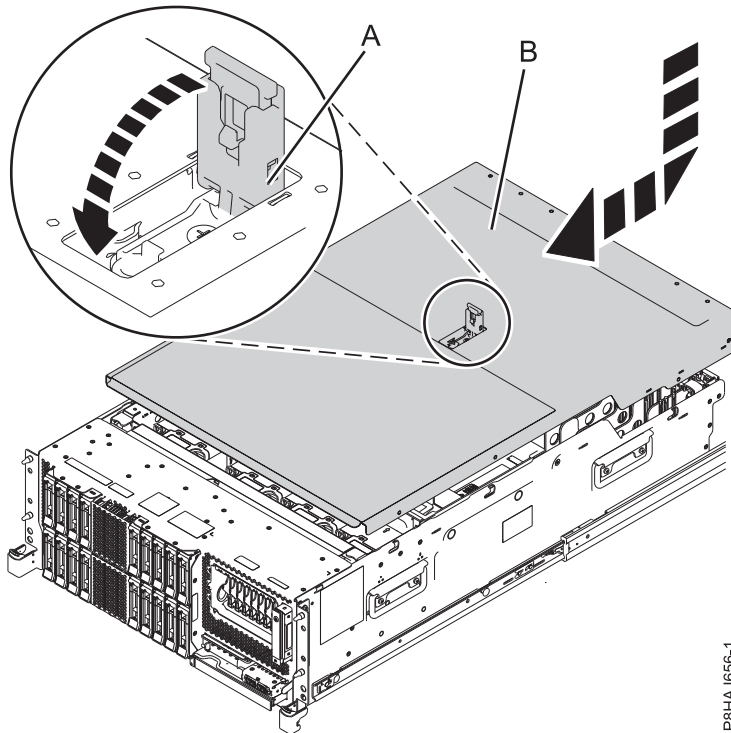
Abbildung 42. Serviceabdeckung installieren
