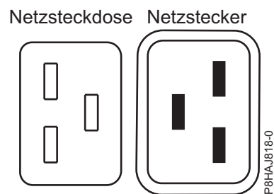
Abbildung 14. Anschlüsse beim System vom Typ 8408-44E
