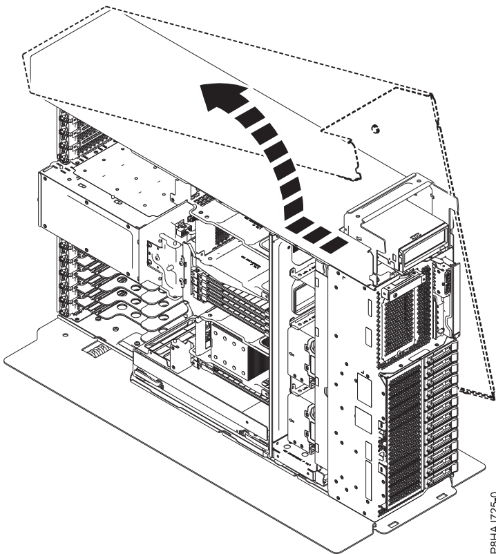
Abbildung 31. Ausbauen der Seitenabdeckung bei einem Standalone-System vom Typ 8286-41A
