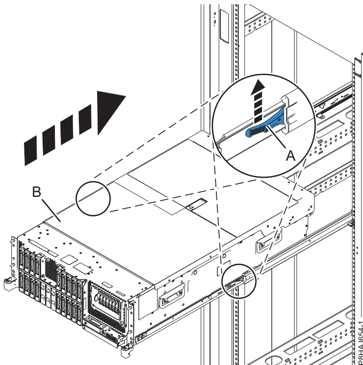
Abbildung 50. System in die Betriebsposition bringen
