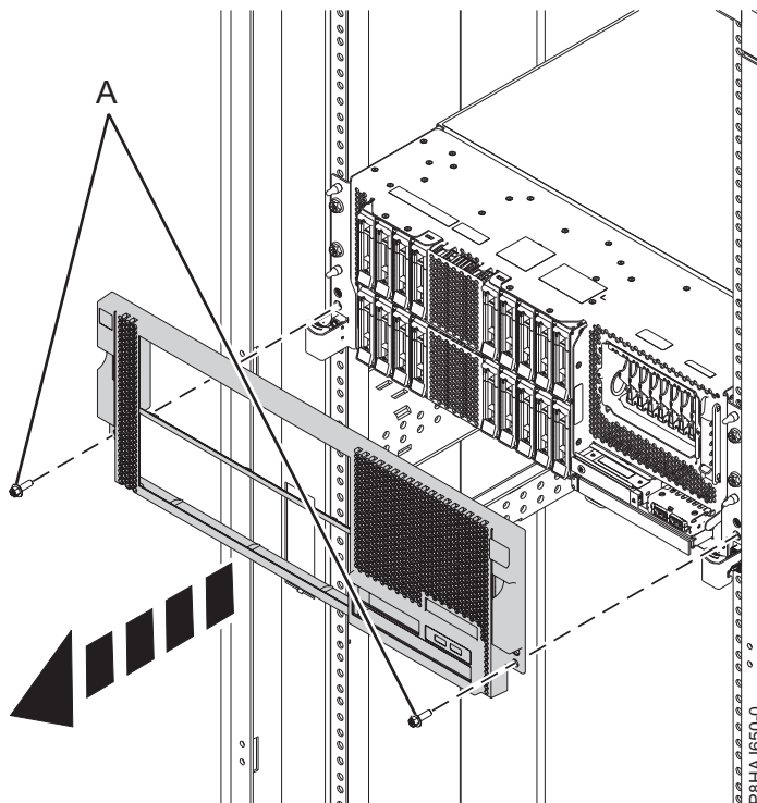
Abbildung 26. Vordere Abdeckung ausbauen
