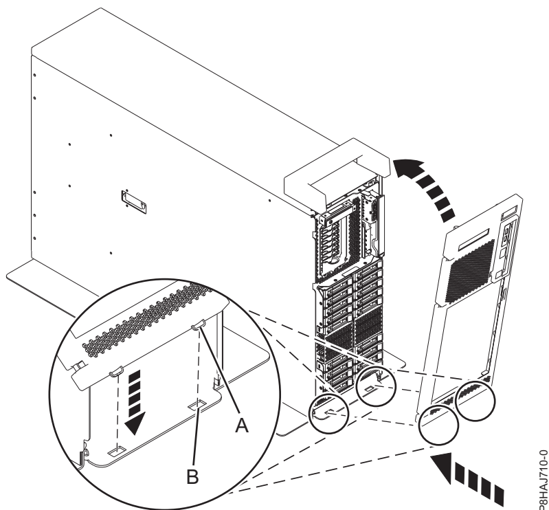
Abbildung 34. Vordere Abdeckung installieren
