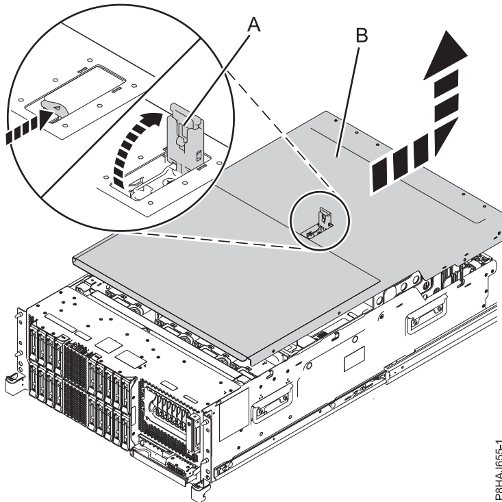
Abbildung 40. Serviceabdeckung ausbauen
