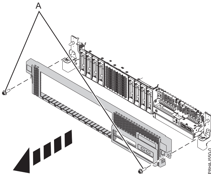
Abbildung 25. Vordere Abdeckung ausbauen
