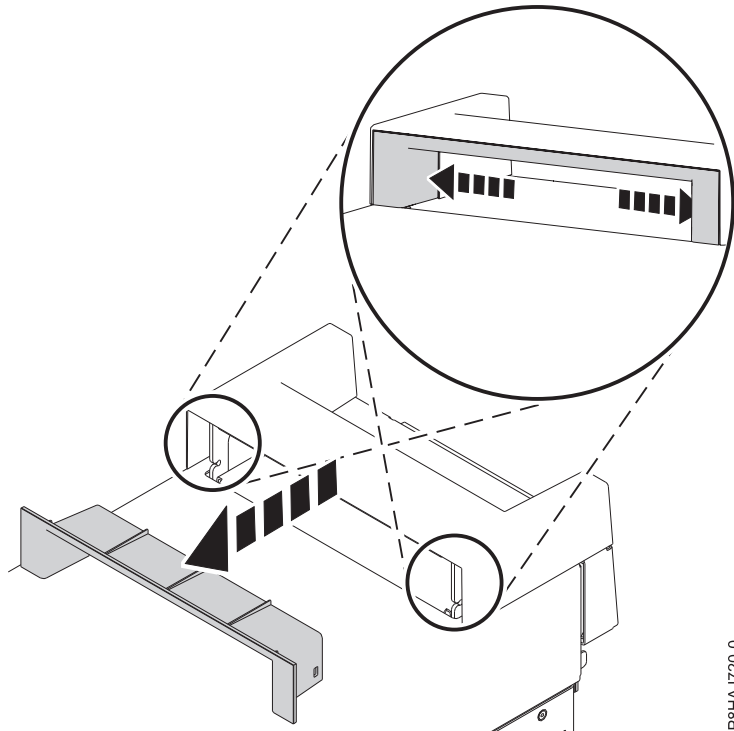
Abbildung 28. Entfernen des Elements innerhalb der Griffabdeckung bei einem Standalone-System vom Typ 8286-41A
