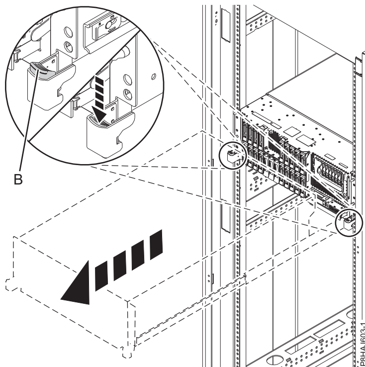
Abbildung 49. Seitliche Verriegelungen entriegeln
