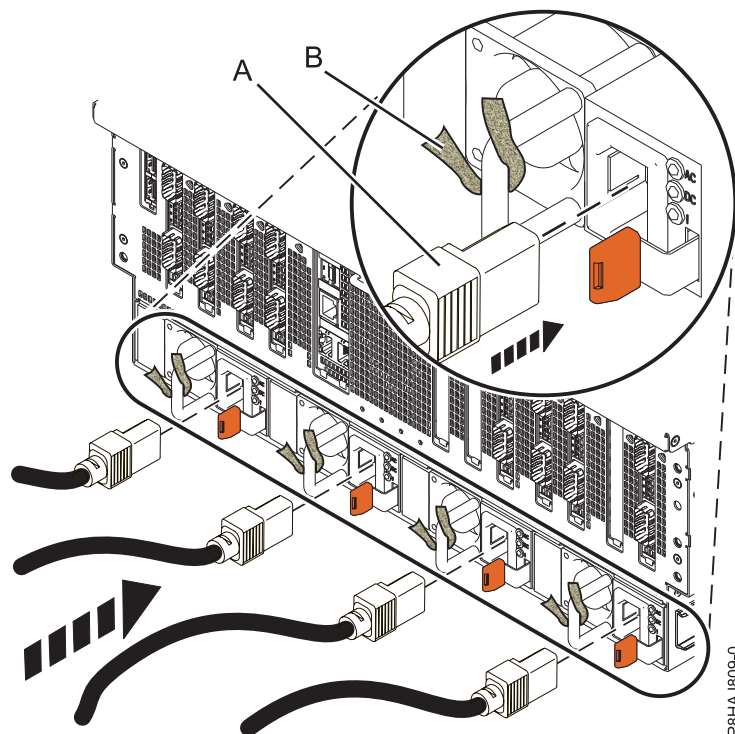
Abbildung 24. Netzkabel bei einem System vom Typ 8408-44E oder 8408-E8E anschließen
