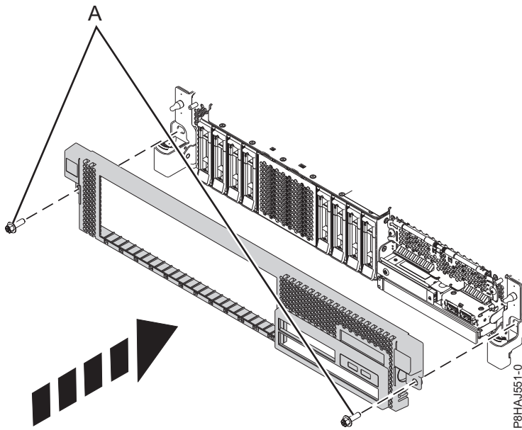
Abbildung 32. Vordere Abdeckung installieren
