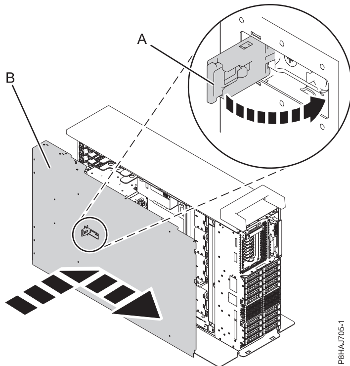
Abbildung 43. Serviceabdeckung installieren
