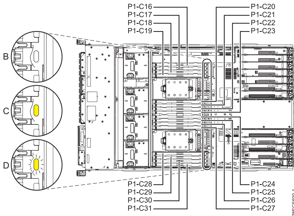
Abbildung 1. Positionen der Speichermodule und Serviceindikatoren im System vom Typ 8247-42L, 8286-41A oder 8286-42A
