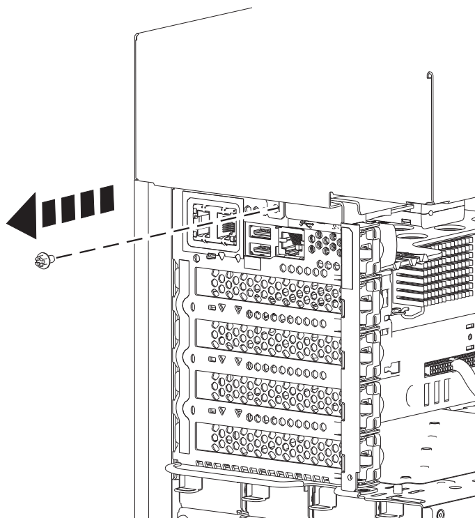
Abbildung 30. Entfernen der Schraube der Seitenabdeckung bei einem Standalone-System vom Typ 8286-41A
