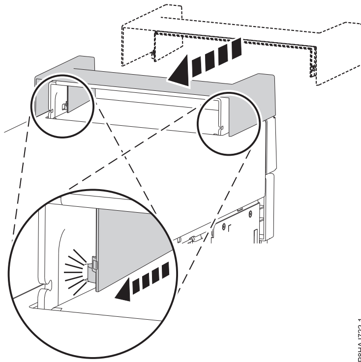
Abbildung 36. Befestigen der Griffabdeckung bei einem Standalone-System vom Typ 8286-41A
