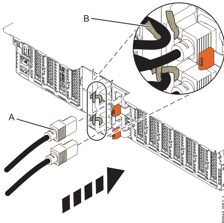
Abbildung 23. Netzkabel bei einem System vom Typ 5148-21L, 5148-22L, 8247-21L, 8247-22L, 8284-21A oder 8284-22A anschließen
