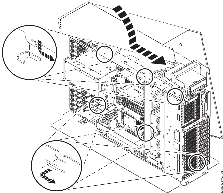
Abbildung 38. Installieren der Seitenabdeckung bei einem Standalone-System vom Typ 8286-41A
