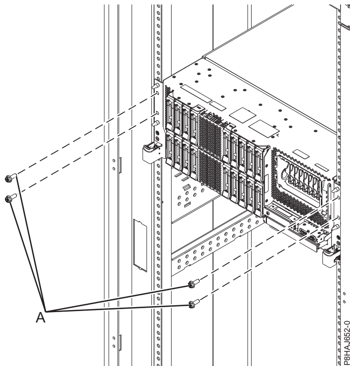
Abbildung 48. Entfernen der vorderen Schrauben
