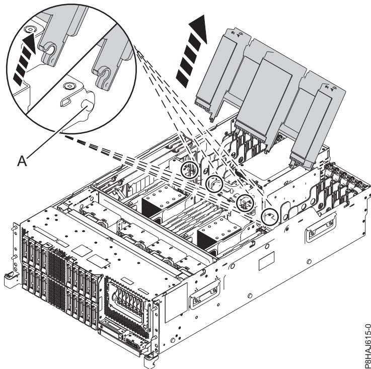
Abbildung 46. Luftführung ausbauen
