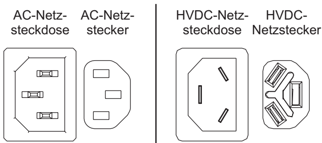
Abbildung 19. AC- und HVDC-Anschlüsse
