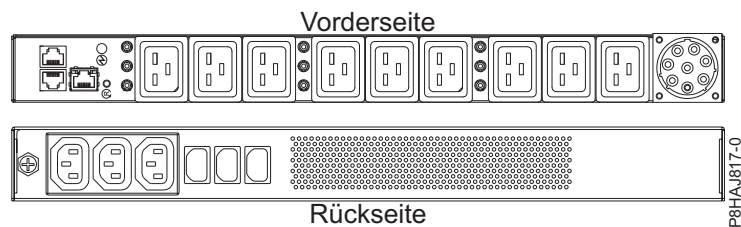
Abbildung 15. PDU beim System vom Typ 8408-44E
