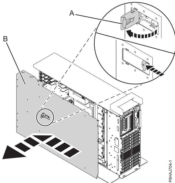
Abbildung 41. Serviceabdeckung ausbauen
