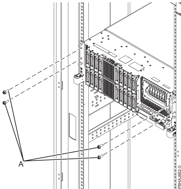
Abbildung 78. Vordere Schrauben entfernen
