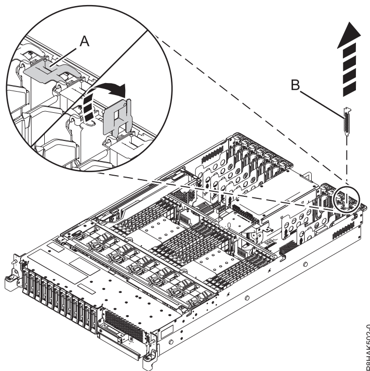
Abbildung 2. Platzhalterelement aus einem PCIe-Adaptersteckplatz in einem System vom Typ 5148-21L, 5148-22L, 8247-21L, 8247-22L, 8284-21A oder 8284-22A ausbauen
