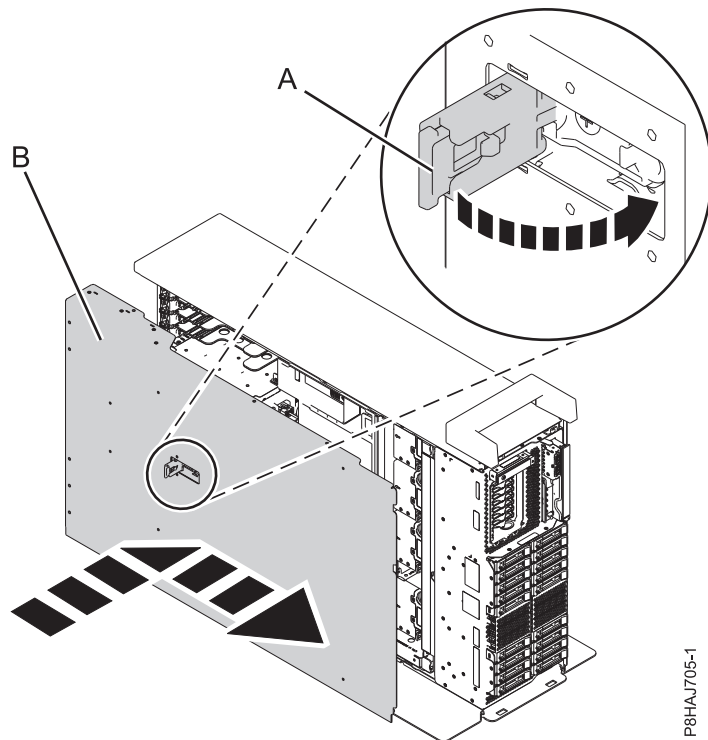
Abbildung 73. Serviceabdeckung installieren
