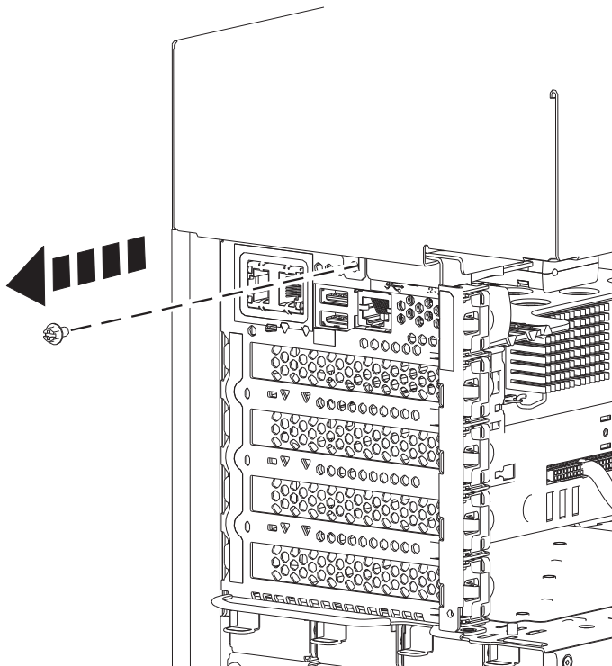
Abbildung 60. Schraube der Seitenabdeckung bei einem eigenständigen System vom Typ 8286-41A entfernen
