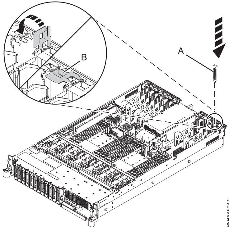
Abbildung 16. Platzhalterelement in einem PCIe-Adaptersteckplatz in einem System vom Typ 5148-21L, 5148-22L, 8247-21L, 8247-22L, 8284-21A oder 8284-22A installieren
