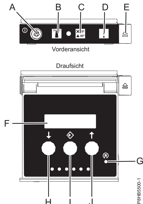
Abbildung 42. Steuerkonsole
