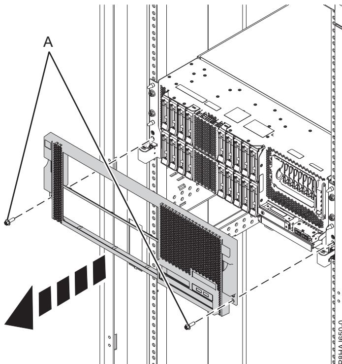
Abbildung 56. Vordere Abdeckung ausbauen
