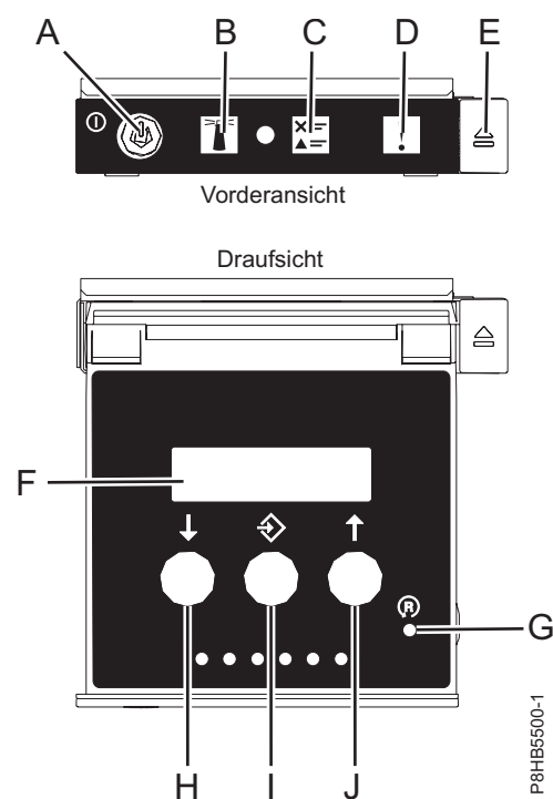
Abbildung 41. LEDs der Steuerkonsole
