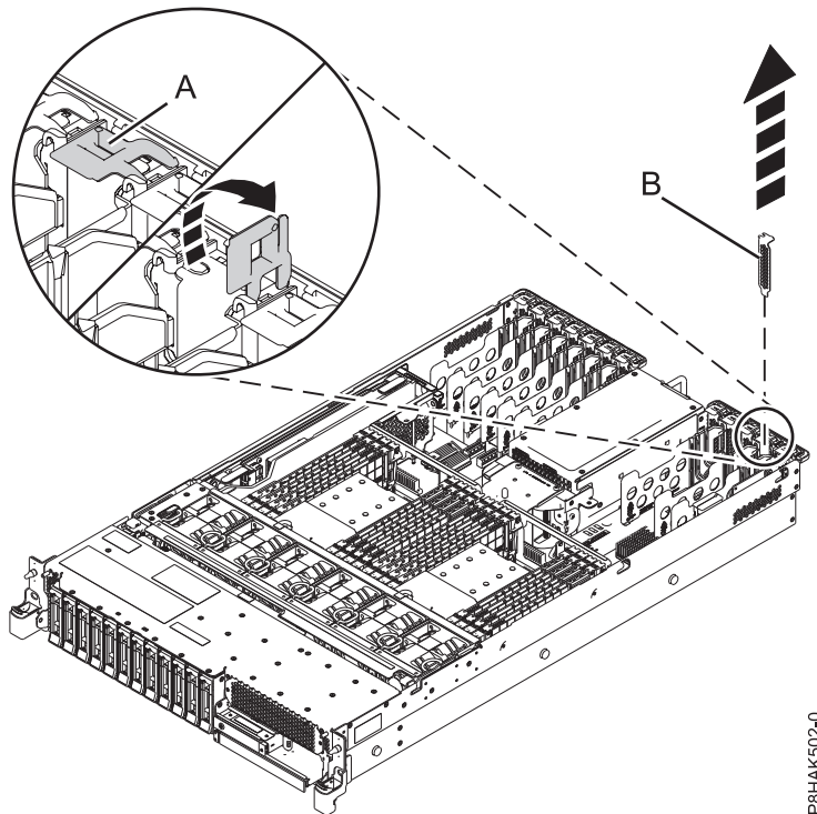
Abbildung 28. Platzhalterelement aus einem PCIe-Adaptersteckplatz in einem System vom Typ 5148-21L, 5148-22L, 8247-21L, 8247-22L, 8284-21A oder 8284-22A ausbauen
