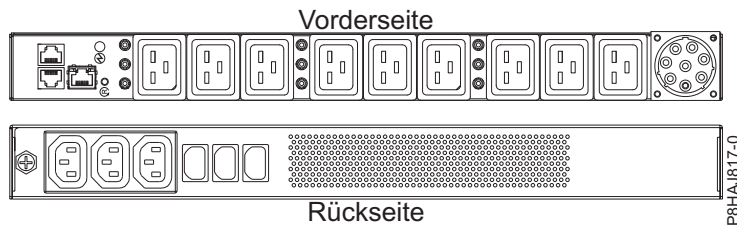
Abbildung 45. PDU beim System vom Typ 8408-44E
