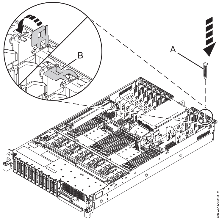
Abbildung 27. Platzhalterelement in einem PCIe-Adaptersteckplatz in einem System vom Typ 5148-21L, 5148-22L, 8247-21L, 8247-22L, 8284-21A oder 8284-22A installieren
