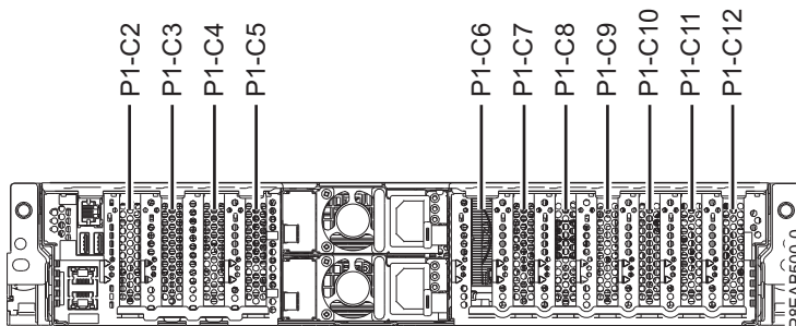
Abbildung 1. Positionen der PCIe-Adaptersteckplätze in einem System vom Typ 5148-21L, 5148-22L, 8247-21L, 8247-22L, 8284-21A oder 8284-22A
