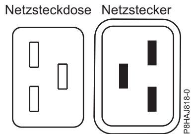
Abbildung 50. Anschlüsse beim System vom Typ 8408-44E
