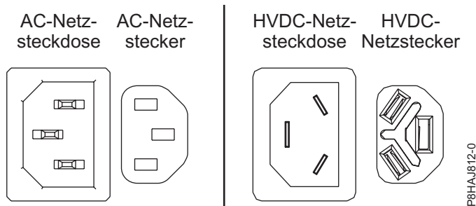
Abbildung 43. AC- und HVDC-Anschlüsse
