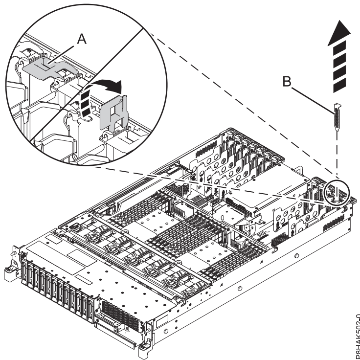
Abbildung 8. Platzhalterelement aus einem PCIe-Adaptersteckplatz in einem System vom Typ 5148-21L, 5148-22L, 8247-21L, 8247-22L, 8284-21A oder 8284-22A ausbauen
