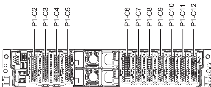
Abbildung 7. Positionen der PCIe-Adaptersteckplätze in einem System vom Typ 5148-21L, 5148-22L, 8247-21L, 8247-22L, 8284-21A oder 8284-22A
