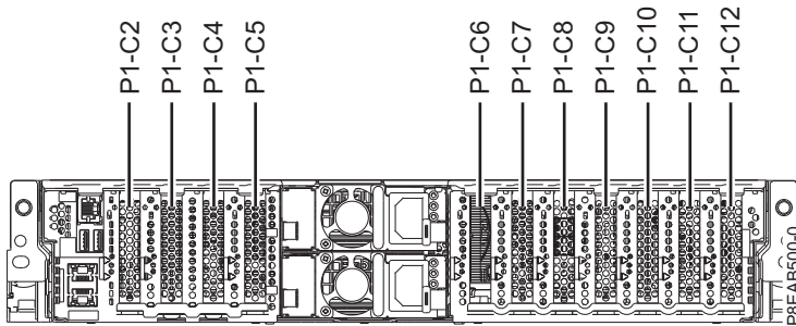
Abbildung 10. Positionen der PCIe-Adaptersteckplätze in einem System vom Typ 5148-21L, 5148-22L, 8247-21L, 8247-22L, 8284-21A oder 8284-22A
