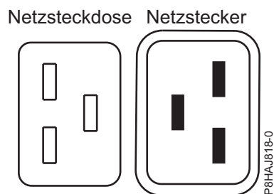
Abbildung 44. Anschlüsse beim System vom Typ 8408-44E
