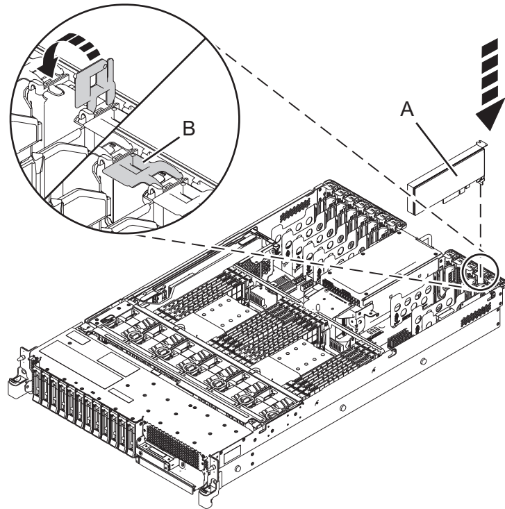
Abbildung 22. PCIe-Adapter im System vom Typ 5148-21L, 5148-22L, 8247-21L, 8247-22L, 8284-21A oder 8284-22A installieren oder austauschen
