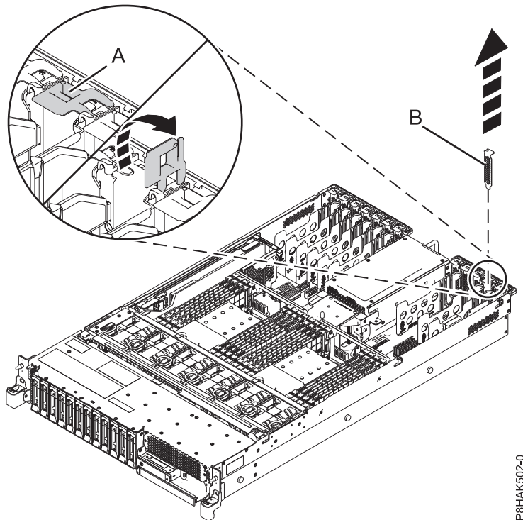
Abbildung 11. Platzhalterelement aus einem PCIe-Adaptersteckplatz in einem System vom Typ 5148-21L, 5148-22L, 8247-21L, 8247-22L, 8284-21A oder 8284-22A ausbauen
