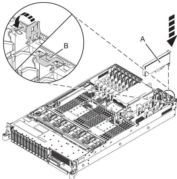
Abbildung 3. PCIe-Adapter im System vom Typ 5148-21L, 5148-22L, 8247-21L, 8247-22L, 8284-21A oder 8284-22A installieren oder austauschen
