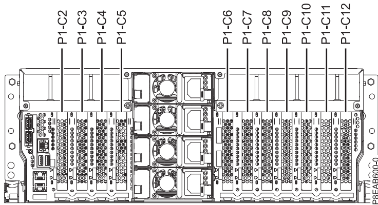
Abbildung 17. Positionen der PCIe-Adaptersteckplätze in einem Einschubsystem
