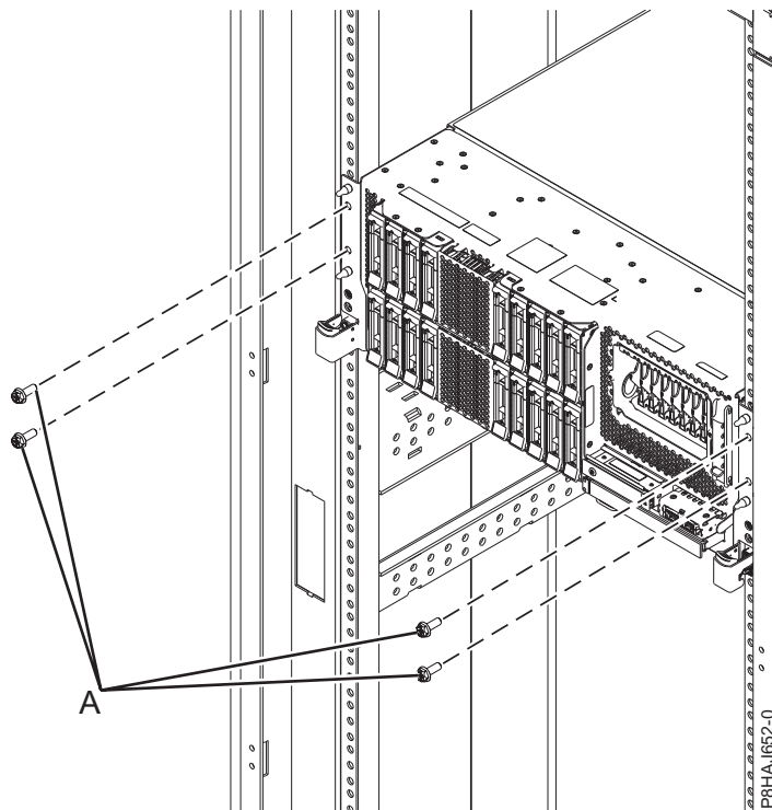
Abbildung 118. Vordere Schrauben entfernen
