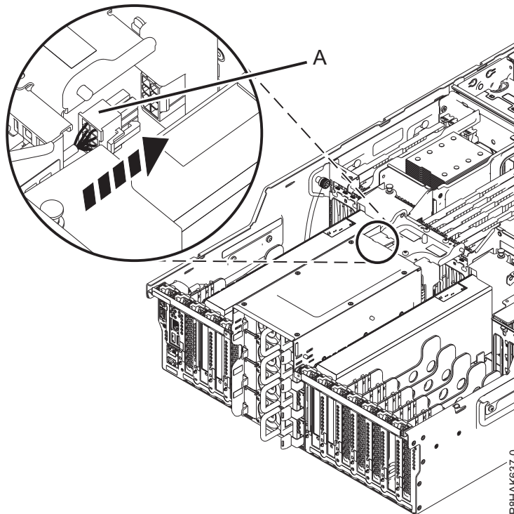
Abbildung 6. Netzkabel für den PCIe-Adapter (GPU) im System vom Typ 8247-42L anschließen
