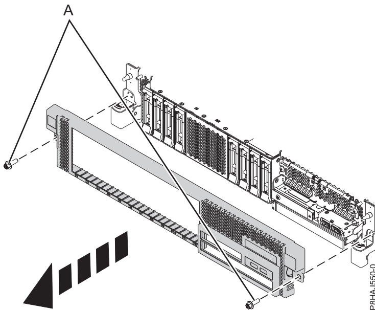
Abbildung 95. Vordere Abdeckung ausbauen
