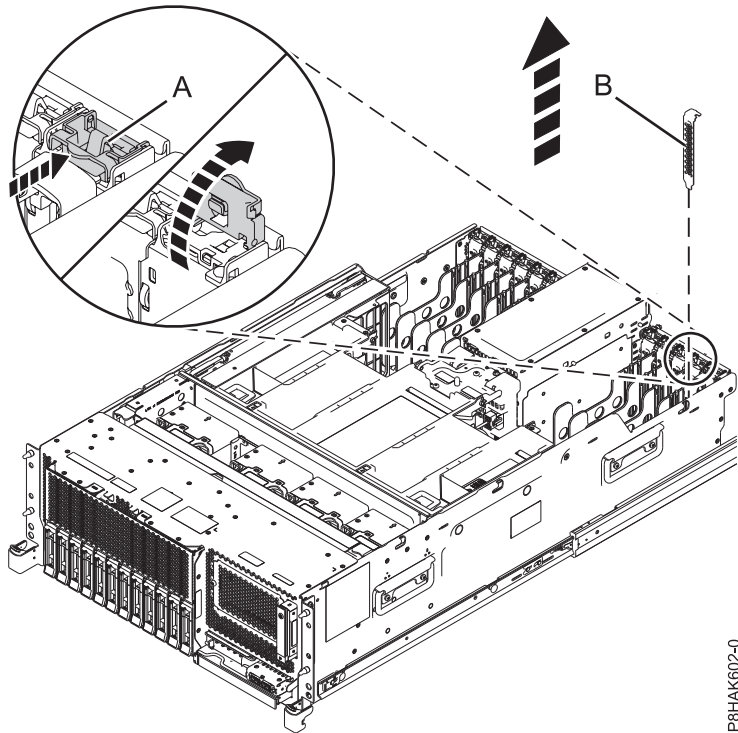
Abbildung 3. Platzhalterelement aus einem PCIe-Adaptersteckplatz in einem Einschubsystem ausbauen
