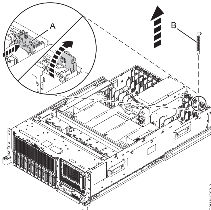
Abbildung 13. Platzhalterelement aus einem PCIe-Adaptersteckplatz in einem Einschubsystem ausbauen
