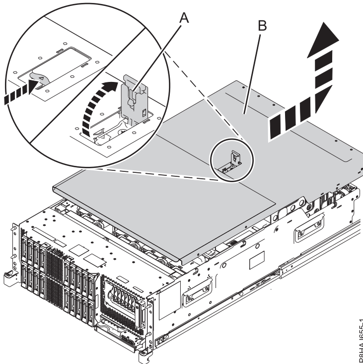
Abbildung 110. Serviceabdeckung ausbauen
