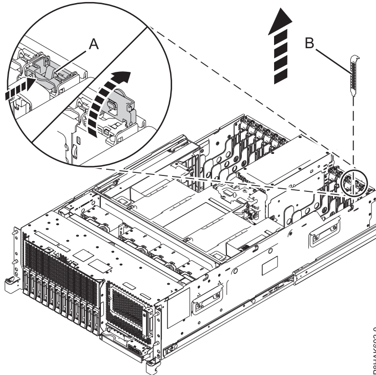
Abbildung 25. Platzhalterelement aus einem PCIe-Adaptersteckplatz in einem Einschubsystem ausbauen
