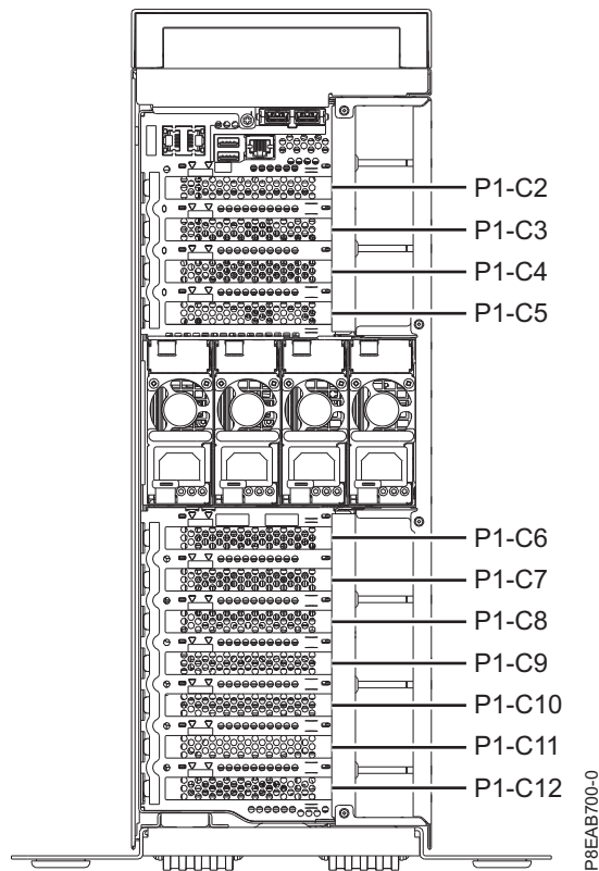
Abbildung 2. Positionen der PCIe-Adaptersteckplätze in einem eigenständiges System vom Typ 8286-41A
