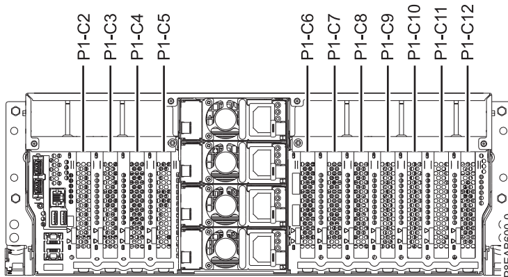
Abbildung 11. Positionen der PCIe-Adaptersteckplätze in einem Einschubsystem
