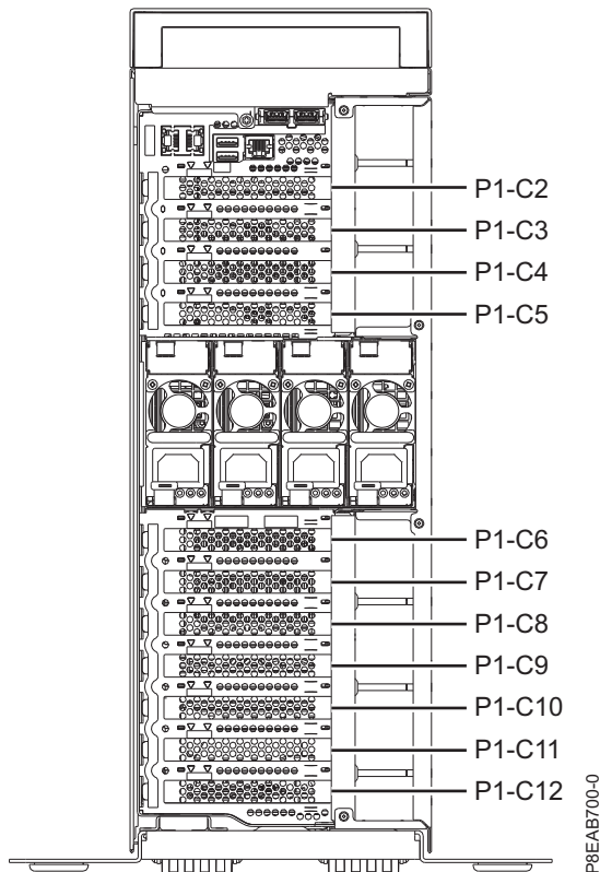
Abbildung 12. Positionen der PCIe-Adaptersteckplätze in einem eigenständiges System vom Typ 8286-41A
