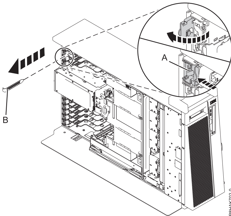
Abbildung 4. Platzhalterelement aus einem PCIe-Adaptersteckplatz in einem eigenständiges System vom Typ 8286-41A ausbauen
