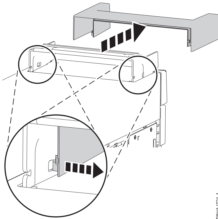
Abbildung 99. Griffabdeckung bei einem eigenständigen System vom Typ 8286-41A ausbauen
