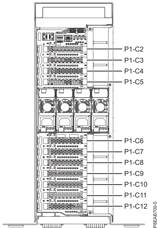
Abbildung 24. Positionen der PCIe-Adaptersteckplätze in einem eigenständiges System vom Typ 8286-41A
