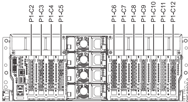
Abbildung 23. Positionen der PCIe-Adaptersteckplätze in einem Einschubsystem
