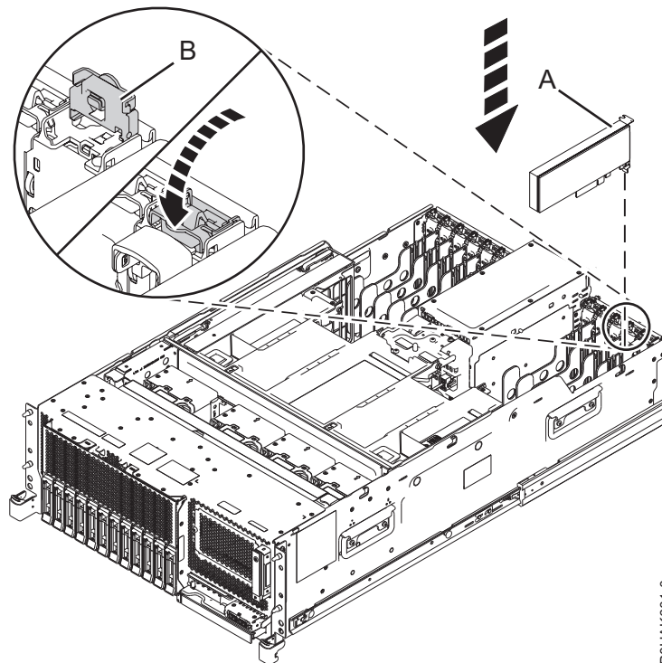
Abbildung 74. PCIe-Adapter in einem Einschubsystem installieren oder austauschen
