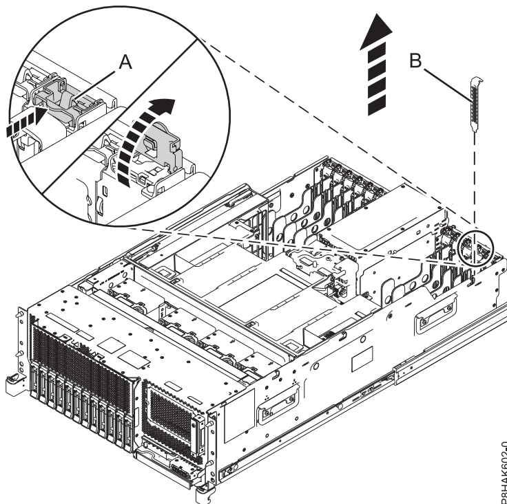
Abbildung 19. Platzhalterelement aus einem PCIe-Adaptersteckplatz in einem Einschubsystem ausbauen
