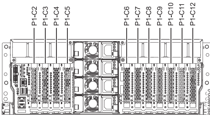
Abbildung 1. Positionen der PCIe-Adaptersteckplätze in einem Einschubsystem
