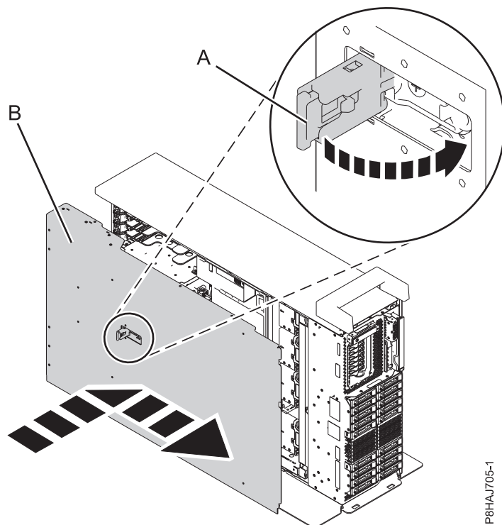
Abbildung 113. Serviceabdeckung installieren
