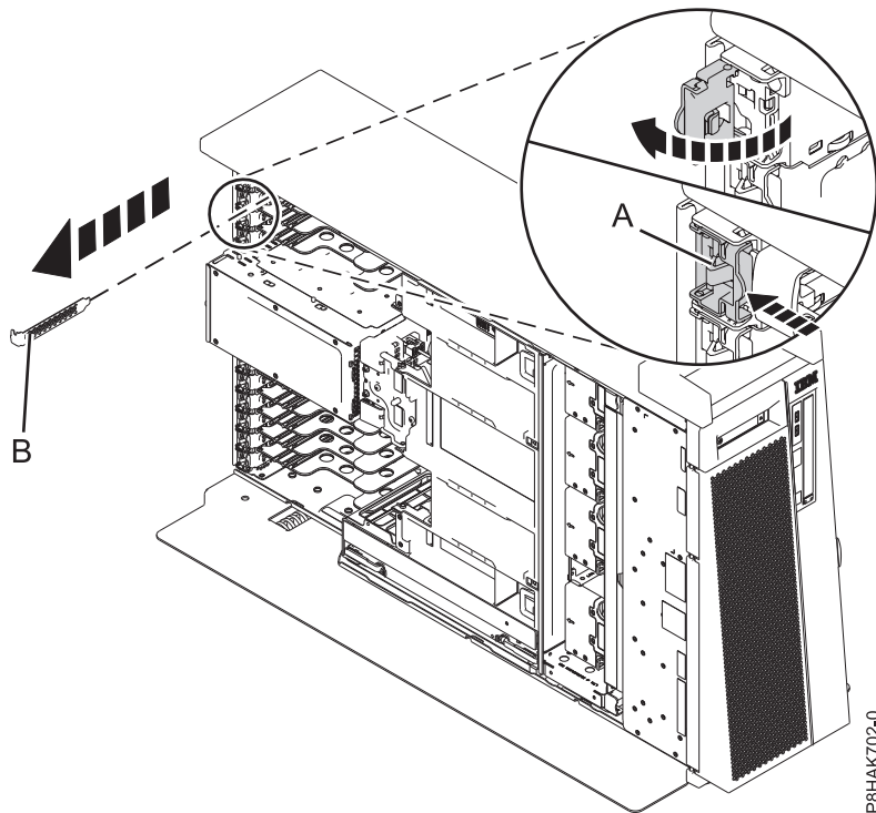
Abbildung 14. Platzhalterelement aus einem PCIe-Adaptersteckplatz in einem eigenständiges System vom Typ 8286-41A ausbauen
