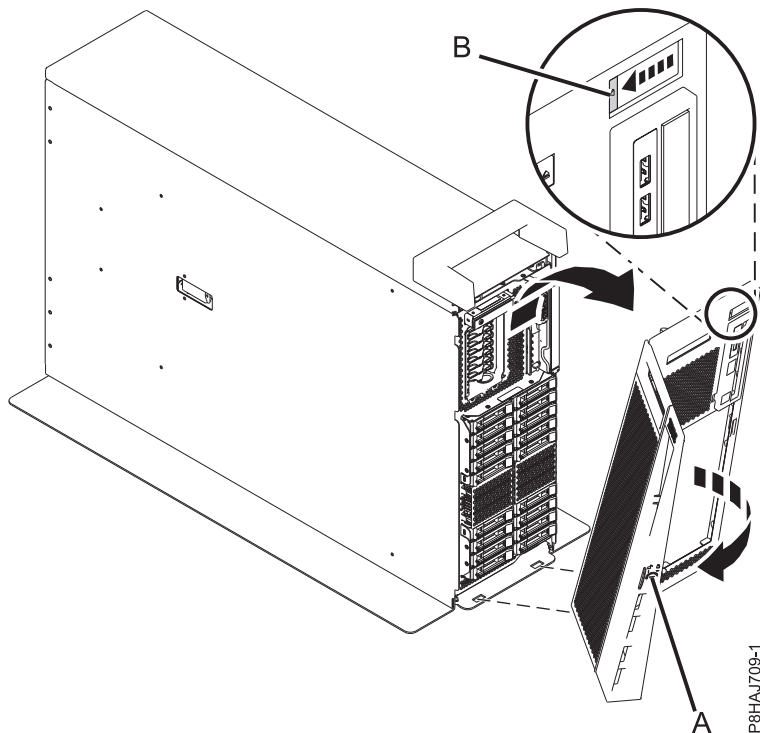
Abbildung 97. Vordere Abdeckung ausbauen
