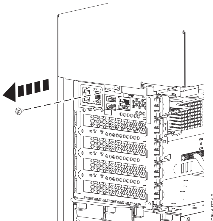
Abbildung 100. Schraube der Seitenabdeckung bei einem eigenständigen System vom Typ 8286-41A entfernen
