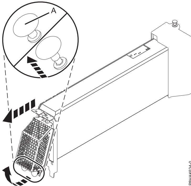
Abbildung 40. Schutzabdeckung aus dem GPU-Adapter ausbauen
