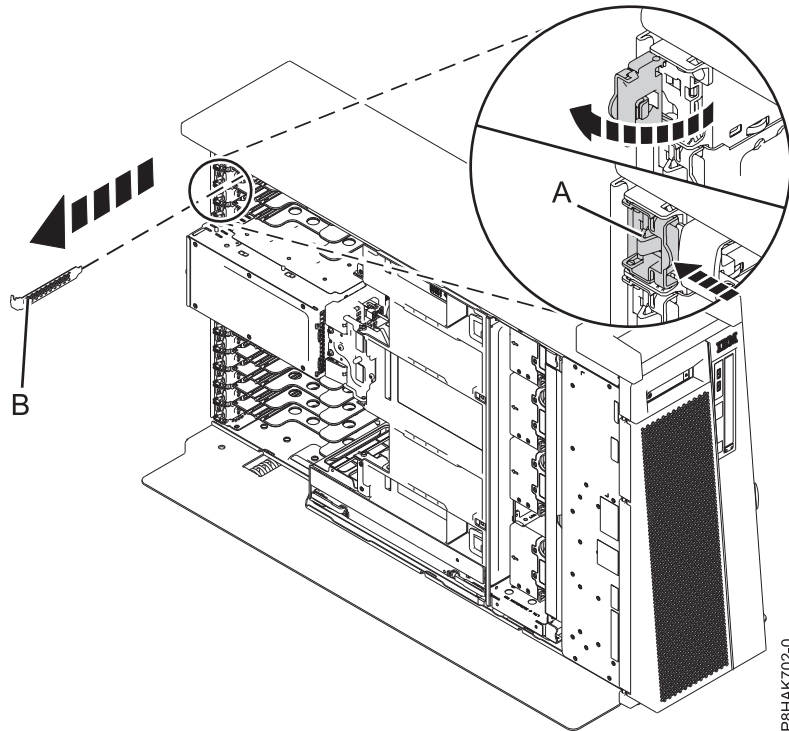
Abbildung 20. Platzhalterelement aus einem PCIe-Adaptersteckplatz in einem eigenständiges System vom Typ 8286-41A ausbauen
