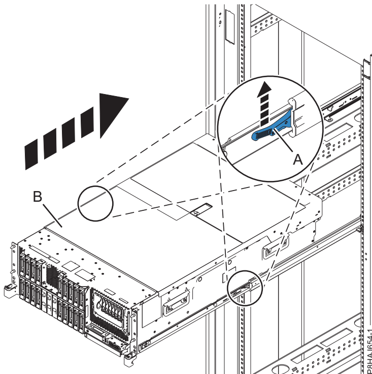
Abbildung 120. System in die Betriebsposition bringen
