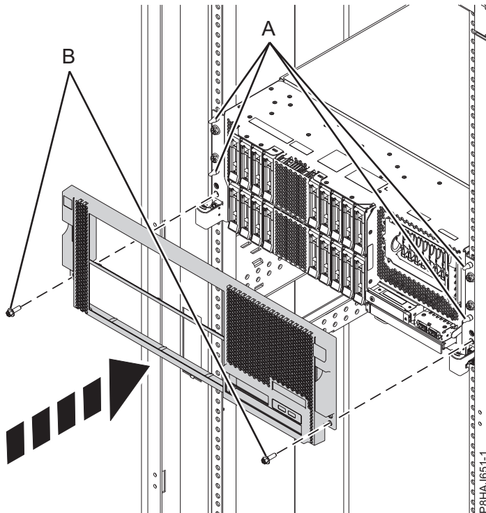
Abbildung 103. Vordere Abdeckung installieren
