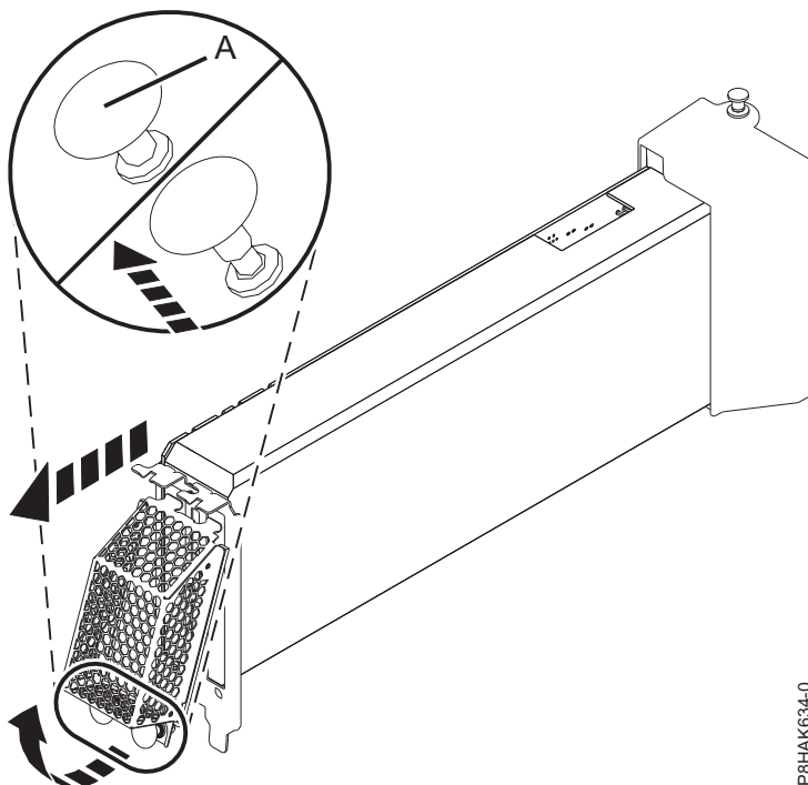
Abbildung 5. Schutzabdeckung aus dem GPU-Adapter ausbauen
