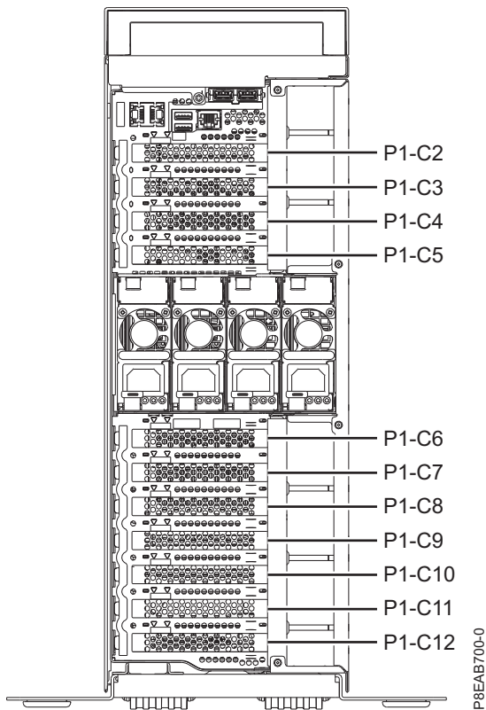
Abbildung 18. Positionen der PCIe-Adaptersteckplätze in einem eigenständiges System vom Typ 8286-41A
