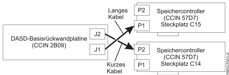
Abbildung 8. SAS-Kabel in einer Konfiguration mit unterteilter Festplatte wieder anschließen
