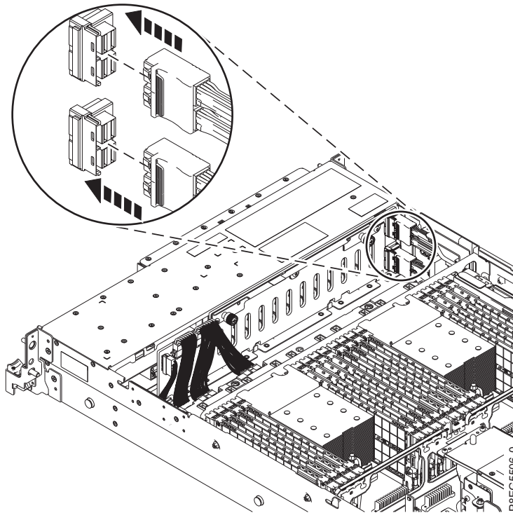
Abbildung 7. Vordere SAS-Kabel wieder an der Rückwandplatine des Plattenlaufwerks anschließen
