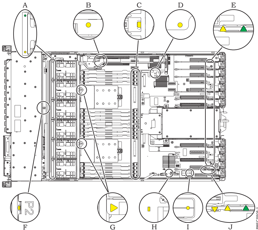
Abbildung 9. Serviceanzeigen
