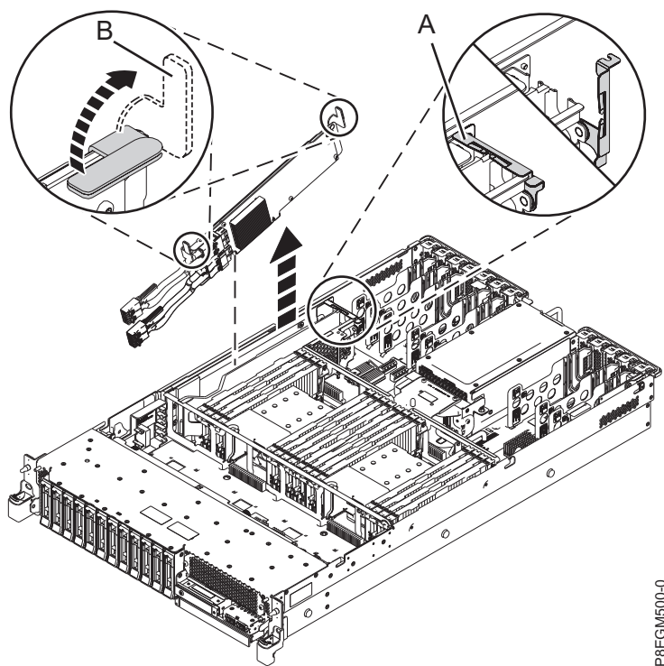
Abbildung 12. Internen SAS-RAID-Adapter ausbauen
