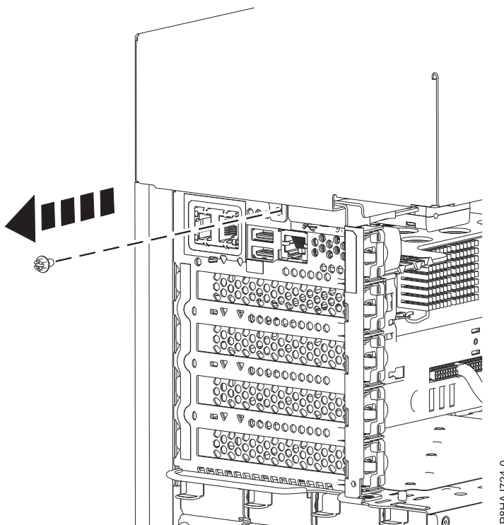
Abbildung 25. Entfernen der Schraube von der Seitenabdeckung bei einem Standalone-System vom Typ 8286-41A
