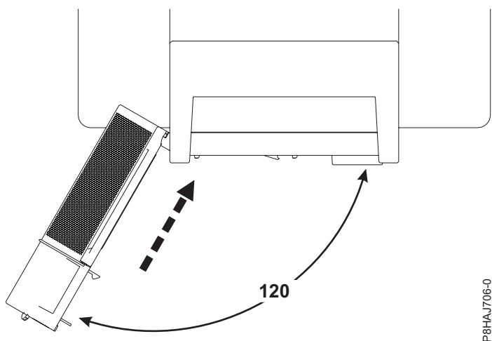
Abbildung 30. Drehen der vorderen Abdeckung
