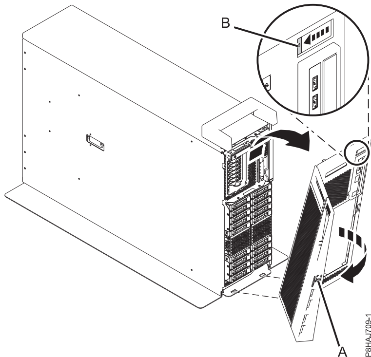
Abbildung 22. Vordere Abdeckung ausbauen
