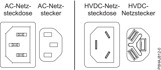
Abbildung 46. AC- und HVDC-Anschlüsse
