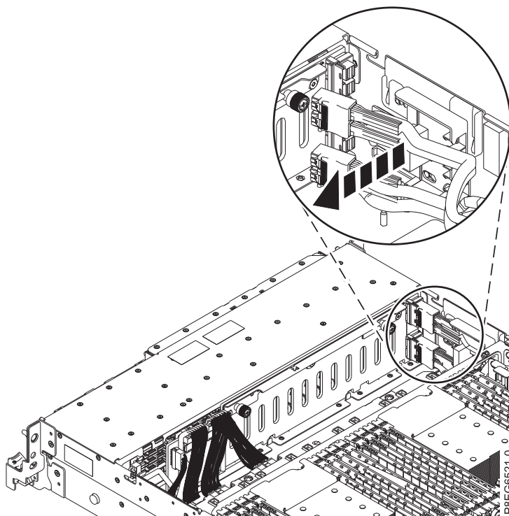
Abbildung 2. Vordere SAS-Kabel aus dem Führungsblock entfernen
