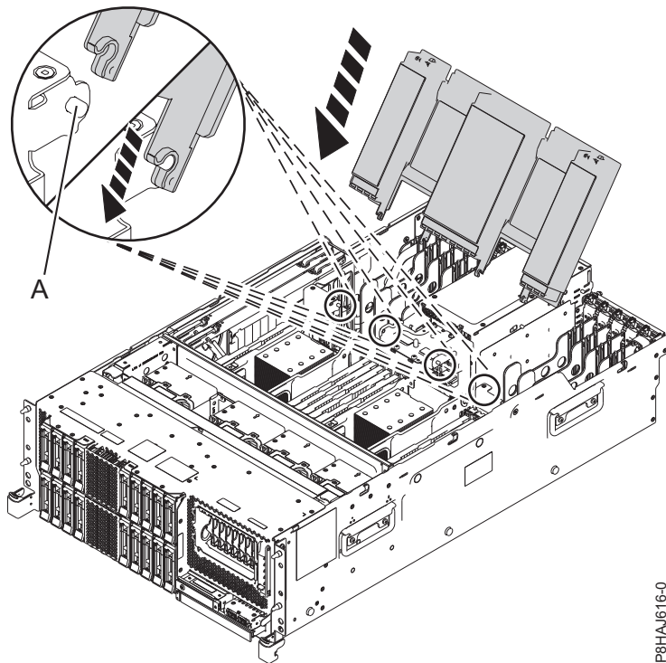
Abbildung 42. Luftführung installieren
