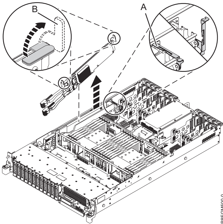
Abbildung 3. Internen SAS-RAID-Adapter in Steckplatz P1-C14 ausbauen
