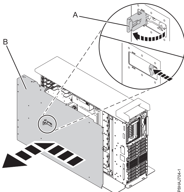
Abbildung 36. Serviceabdeckung ausbauen
