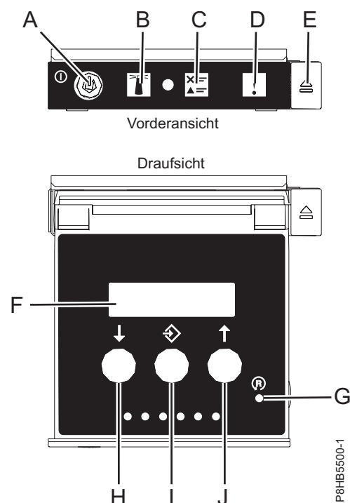
Abbildung 18. LEDs der Steuerkonsole
