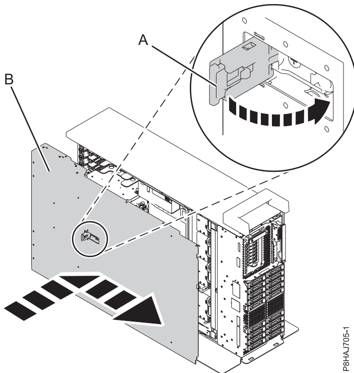
Abbildung 38. Serviceabdeckung installieren
