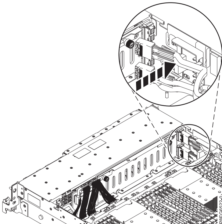
Abbildung 6. Vordere SAS-Kabel verlegen
