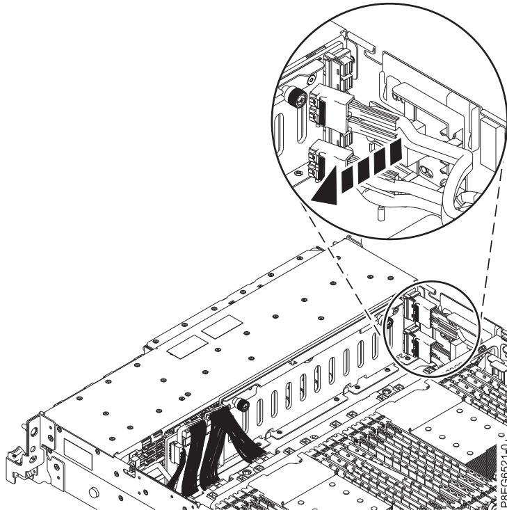
Abbildung 11. Vorderes SAS-Kabel aus dem Führungsblock entfernen
