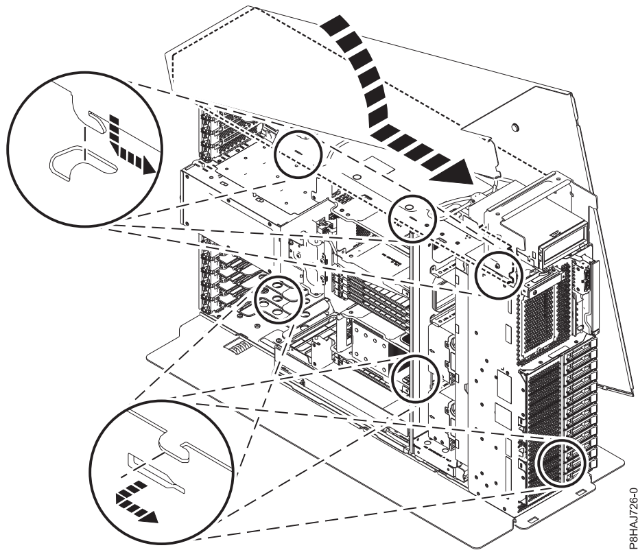
Abbildung 33. Installieren der Seitenabdeckung bei einem Standalone-System vom Typ 8286-41A
