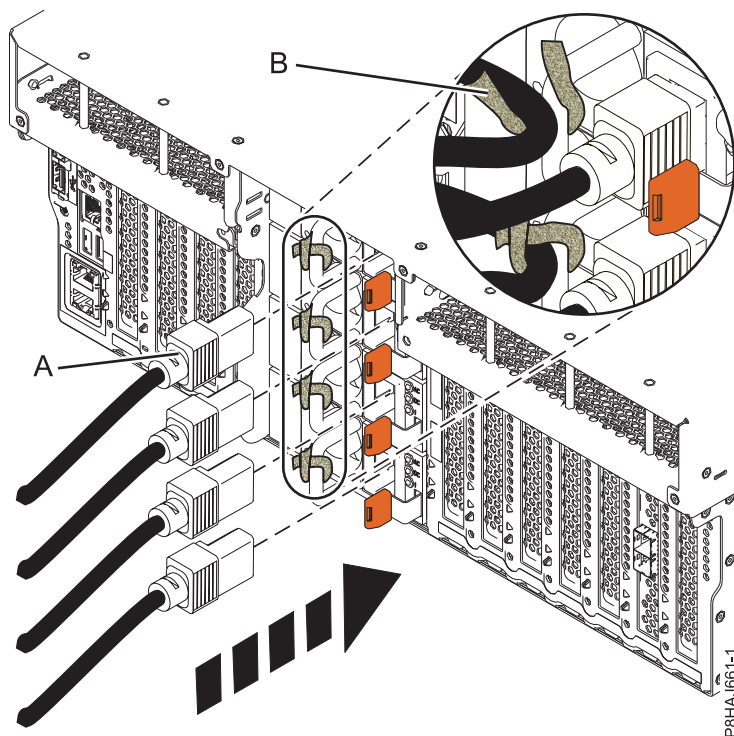
Abbildung 55. Netzkabel anschließen - System vom Typ 8247-42L, 8286-41A oder 8286-42A
