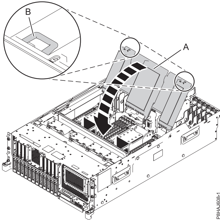
Abbildung 40. Schließen der Luftführung
