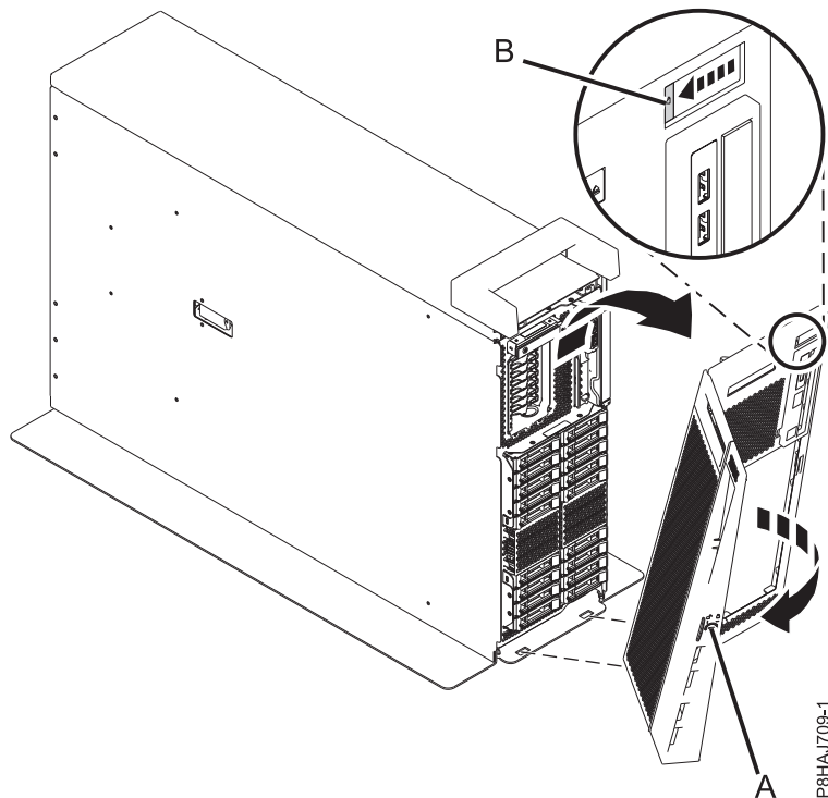
Abbildung 9. Vordere Abdeckung ausbauen
