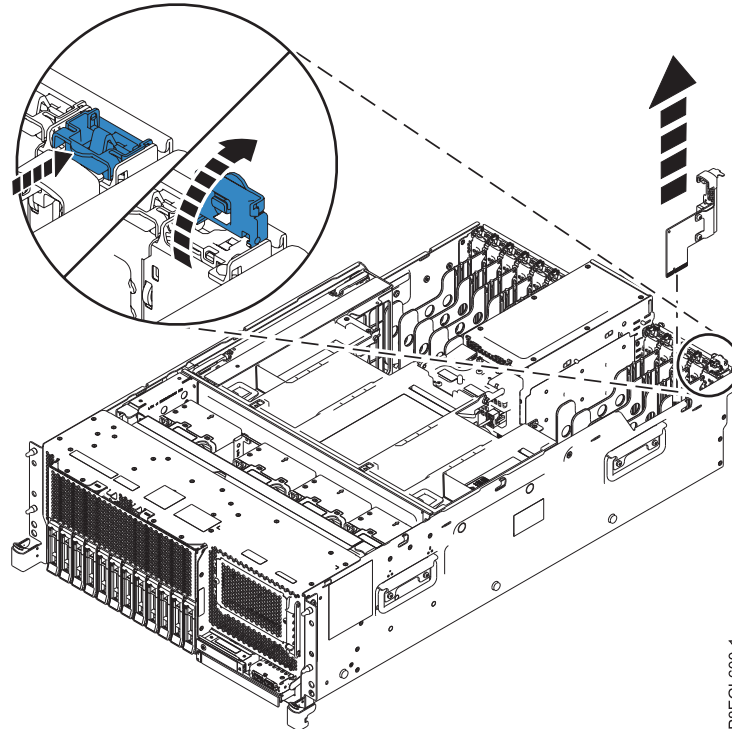
Abbildung 1. Ausbauen der System-E/A-Karte aus einem Einschubsystem
