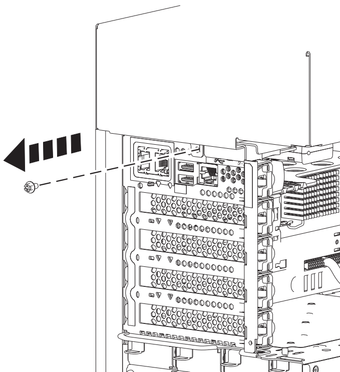
Abbildung 12. Entfernen der Schraube von der Seitenabdeckung bei einem Standalone-System vom Typ 8286-41A
