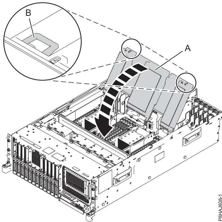
Abbildung 27. Schließen der Luftführung
