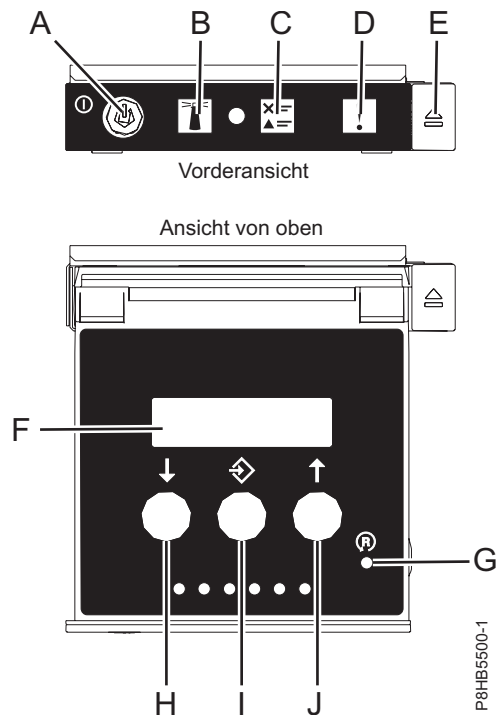
Abbildung 6. Steuerkonsole
