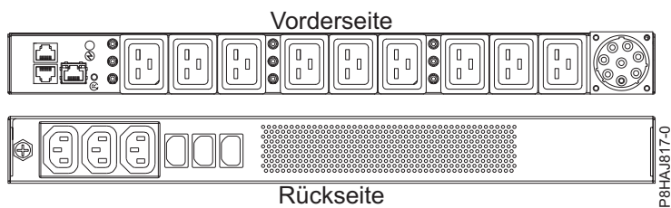
Abbildung 33. PDU beim System vom Typ 8408-44E
