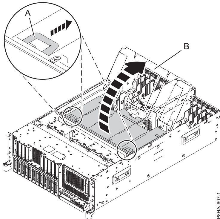
Abbildung 24. Öffnen der Luftführung
