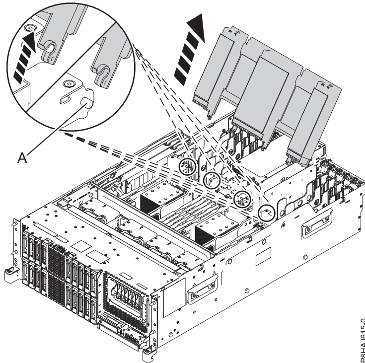
Abbildung 26. Luftführung ausbauen
