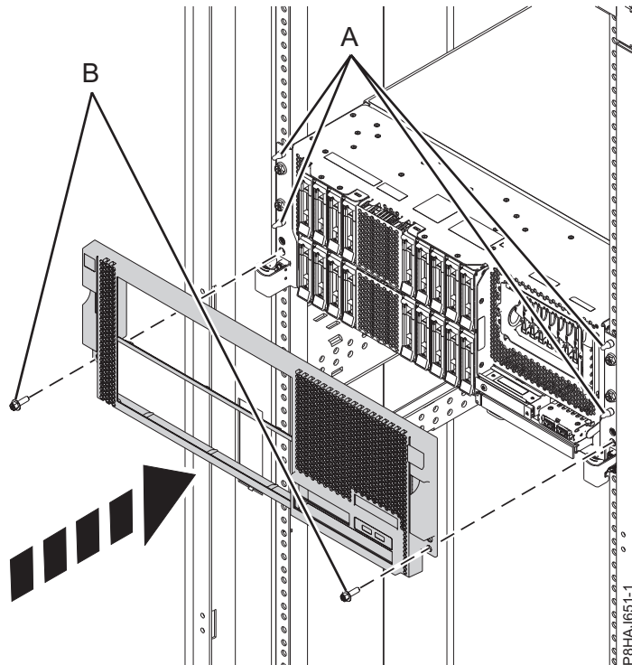
Abbildung 13. Vordere Abdeckung installieren
