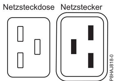
Abbildung 32. Anschlüsse beim System vom Typ 8408-44E
