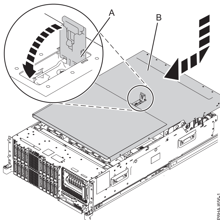
Abbildung 24. Serviceabdeckung installieren
