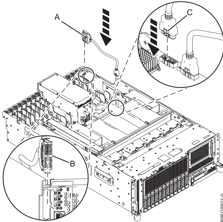
Abbildung 3. Hinteres USB-Kabel austauschen
