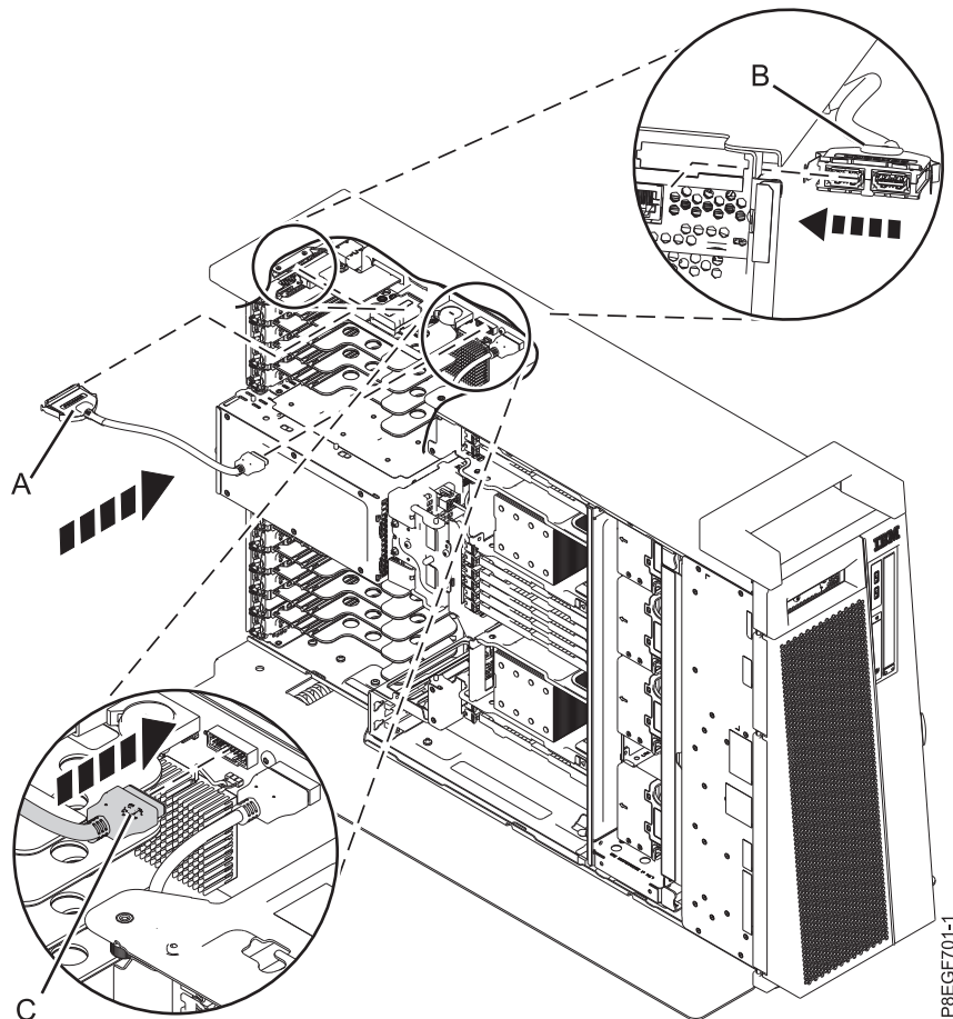
Abbildung 4. Hinteres USB-Kabel bei der Standalone-Version des Systems vom Typ 8286-41A austauschen
