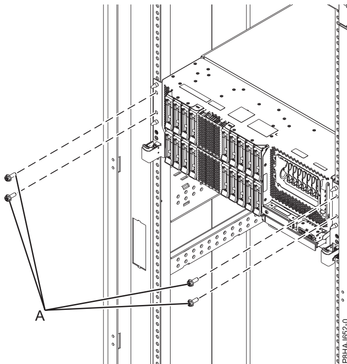
Abbildung 30. Vordere Schrauben entfernen
