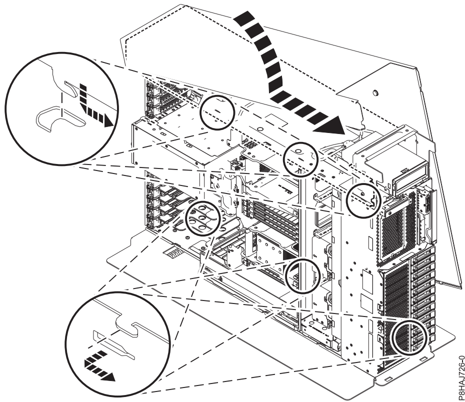
Abbildung 20. Seitenabdeckung bei einem eigenständigen System vom Typ 8286-41A installieren
