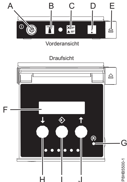
Abbildung 6. Steuerkonsole
