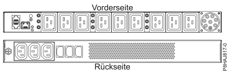
Abbildung 35. Stromversorgungseinheit für das System vom Typ 8408-44E
