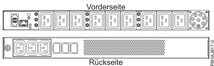
Abbildung 41. Stromversorgungseinheit für das System vom Typ 8408-44E
