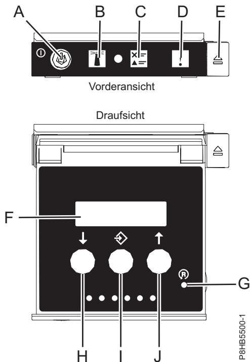
Abbildung 13. Steuerkonsole
