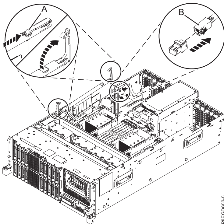
Abbildung 4. Hinteres SAS-Kabel in Steckplatz P1-C14 entfernen
