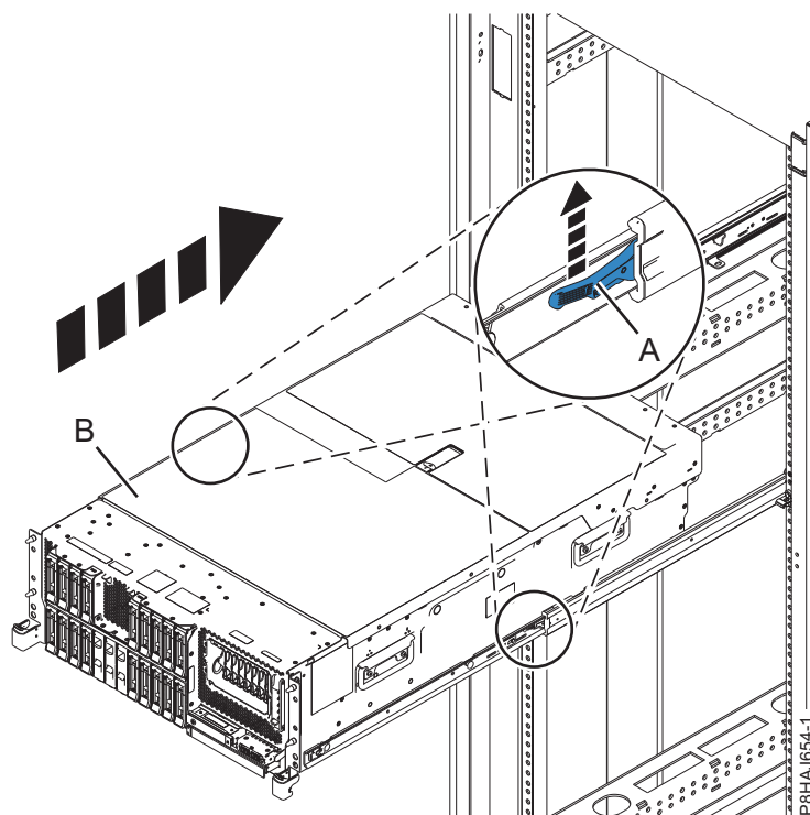
Abbildung 39. System in die Betriebsposition bringen
