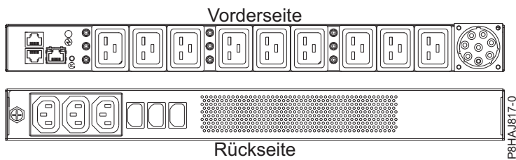
Abbildung 48. PDU beim System vom Typ 8408-44E
