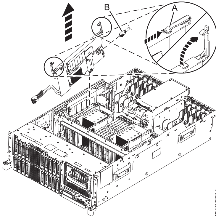
Abbildung 3. Internen SAS-RAID-Adapter in Steckplatz P1-C15 entfernen
