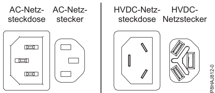
Abbildung 40. AC- und HVDC-Anschlüsse
