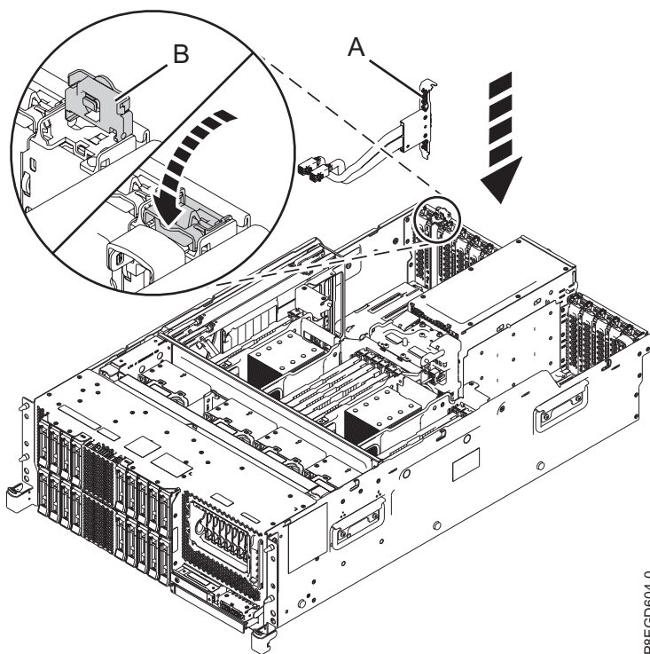
Abbildung 6. Hinteres SAS-Kabel installieren
