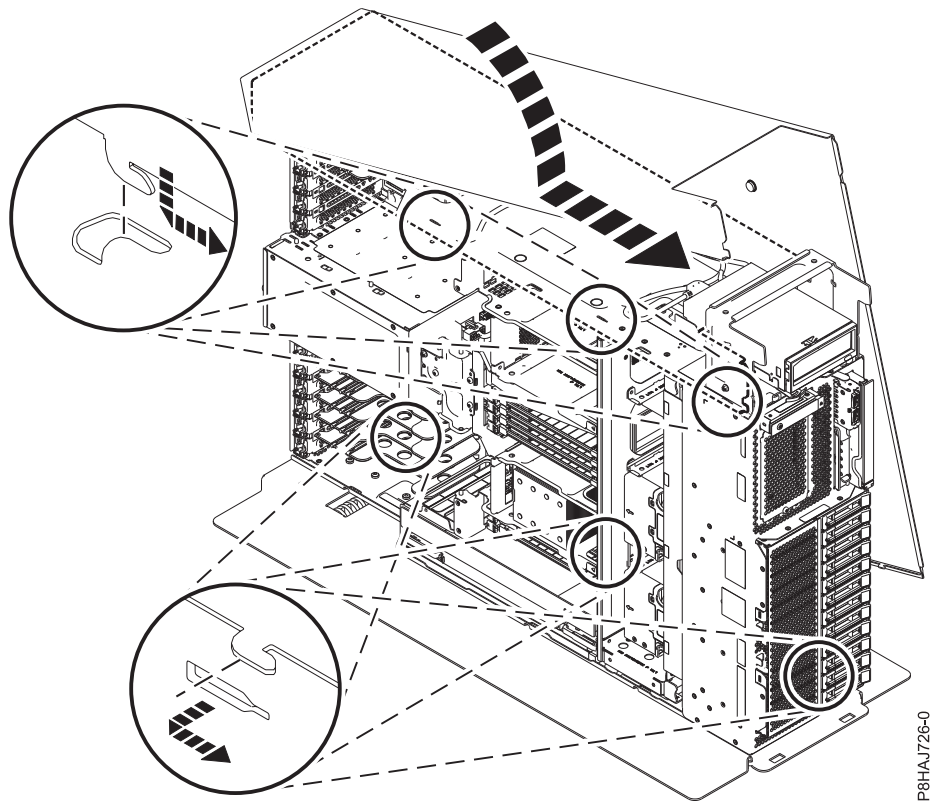
Abbildung 27. Seitenabdeckung bei einem eigenständigen System vom Typ 8286-41A installieren
