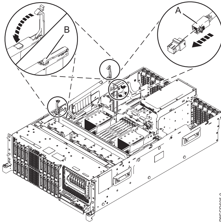
Abbildung 7. Hinteres SAS-Kabel in Steckplatz P1-C14 austauschen
