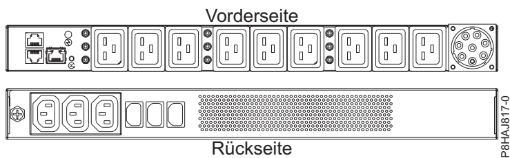
Abbildung 42. PDU beim System vom Typ 8408-44E
