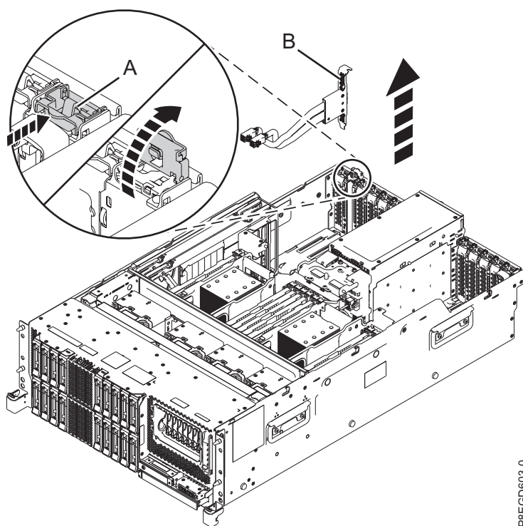
Abbildung 5. Hinteres SAS-Kabel entfernen
