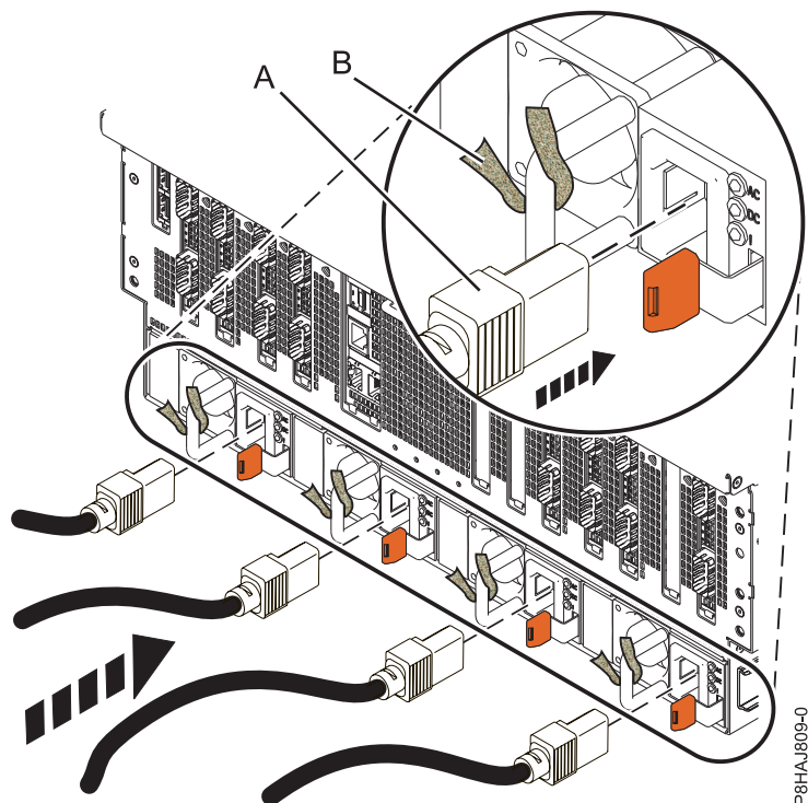
Abbildung 51. Netzkabel anschließen - System vom Typ 8408-44E oder 8408-E8E
