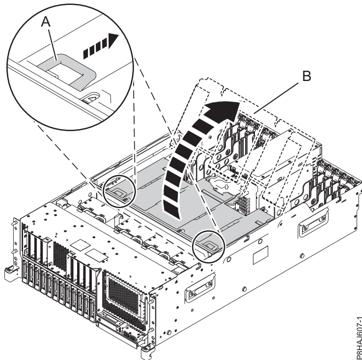
Abbildung 33. Öffnen der Luftführung
