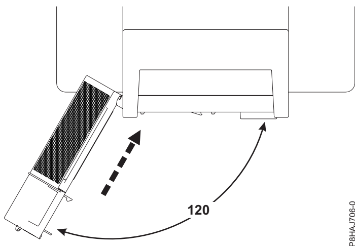
Abbildung 24. Vordere Abdeckung drehen
