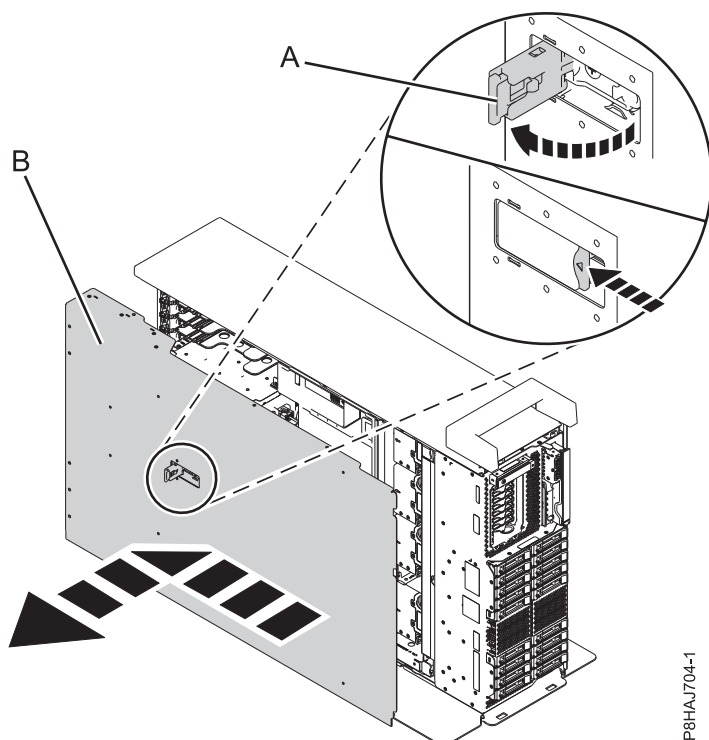
Abbildung 30. Serviceabdeckung ausbauen
