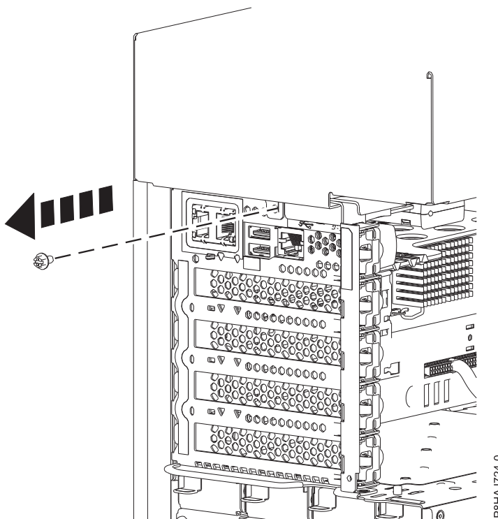
Abbildung 19. Schraube bei einem eigenständigen System vom Typ 8286-41A von der Seitenabdeckung entfernen
