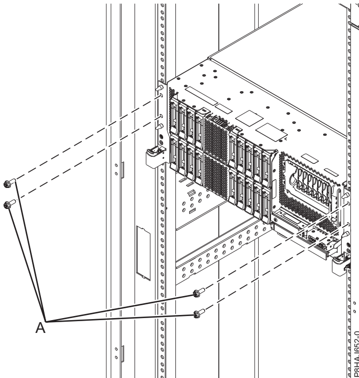
Abbildung 37. Vordere Schrauben entfernen
