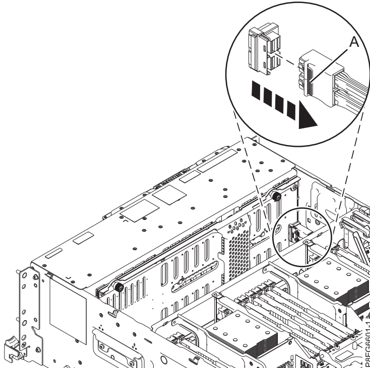
Abbildung 2. SAS-Kabel von der Rückwandplatine des Plattenlaufwerks abziehen
