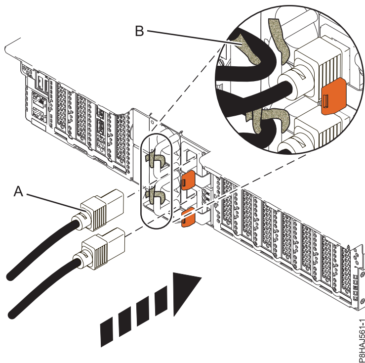
Abbildung 50. Netzkabel anschließen - System vom Typ 5148-21L, 5148-22L, 8247-21L, 8247-22L, 8284-21A oder 8284-22A
