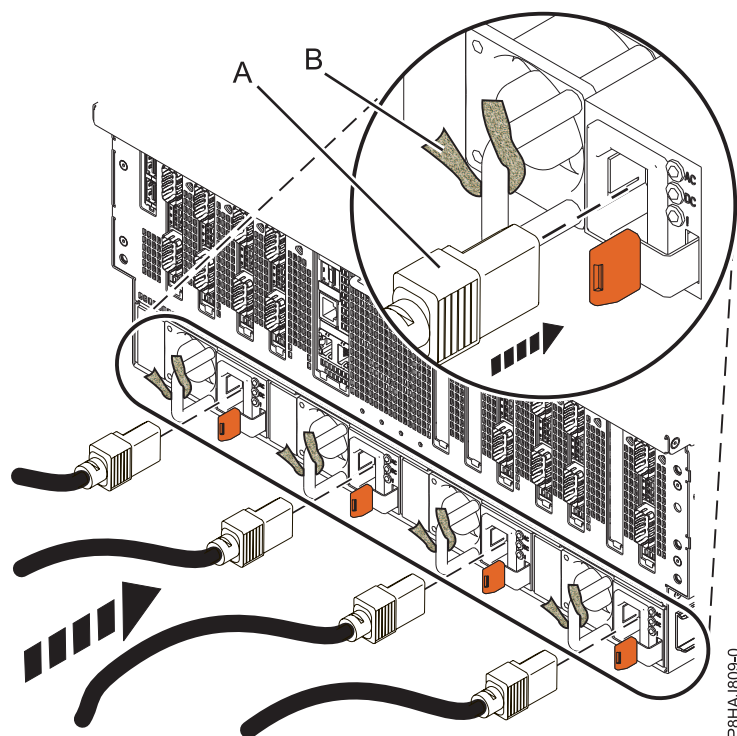
Abbildung 49. Netzkabel an ein System vom Typ 8408-44E oder 8408-E8E anschließen
