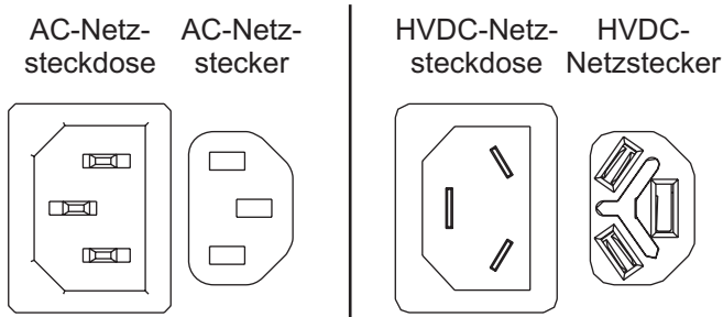
Abbildung 44. AC- und HVDC-Anschlüsse
