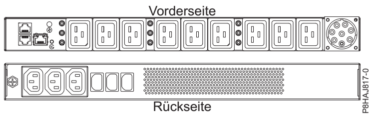
Abbildung 46. PDU beim System vom Typ 8408-44E
