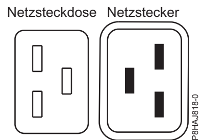
Abbildung 39. Anschlüsse beim System vom Typ 8408-44E
