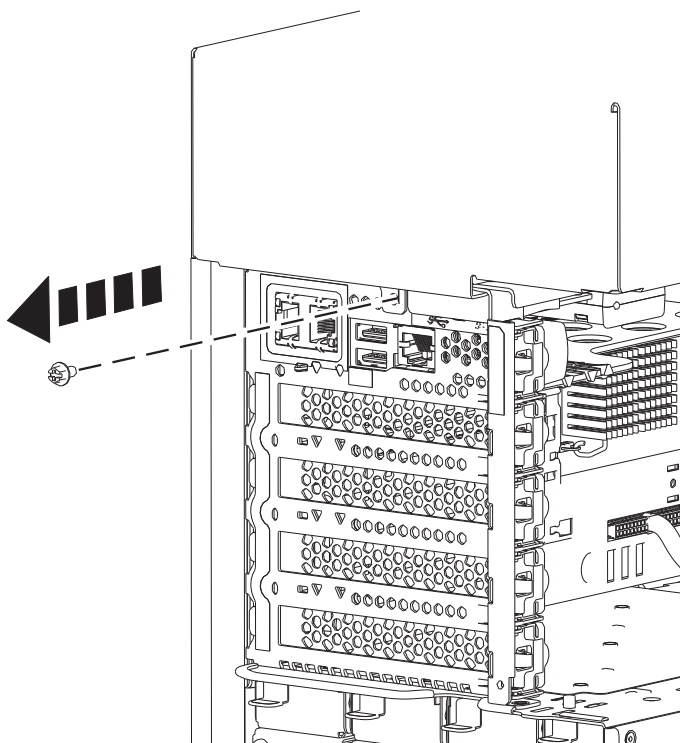
Abbildung 17. Schraube bei einem eigenständigen System vom Typ 8286-41A von der Seitenabdeckung entfernen
