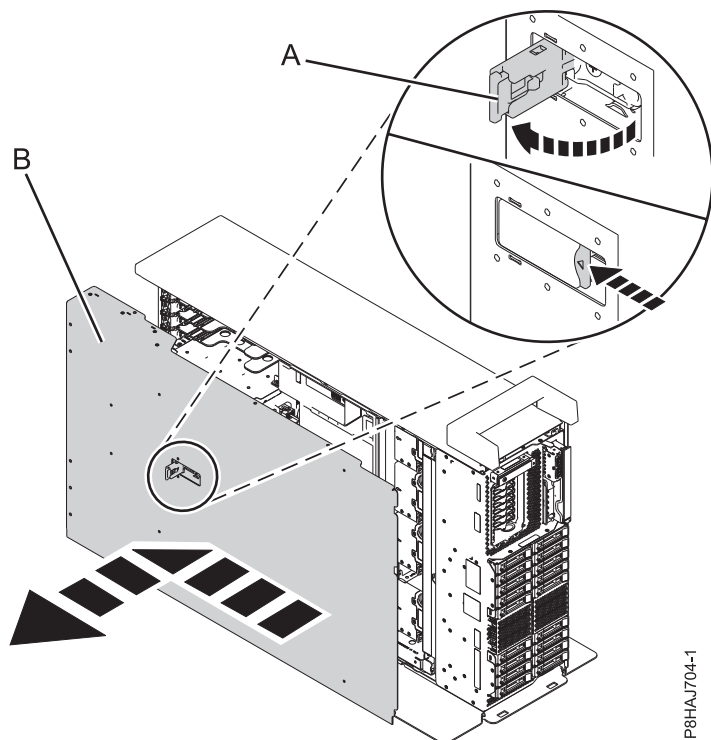
Abbildung 28. Serviceabdeckung ausbauen
