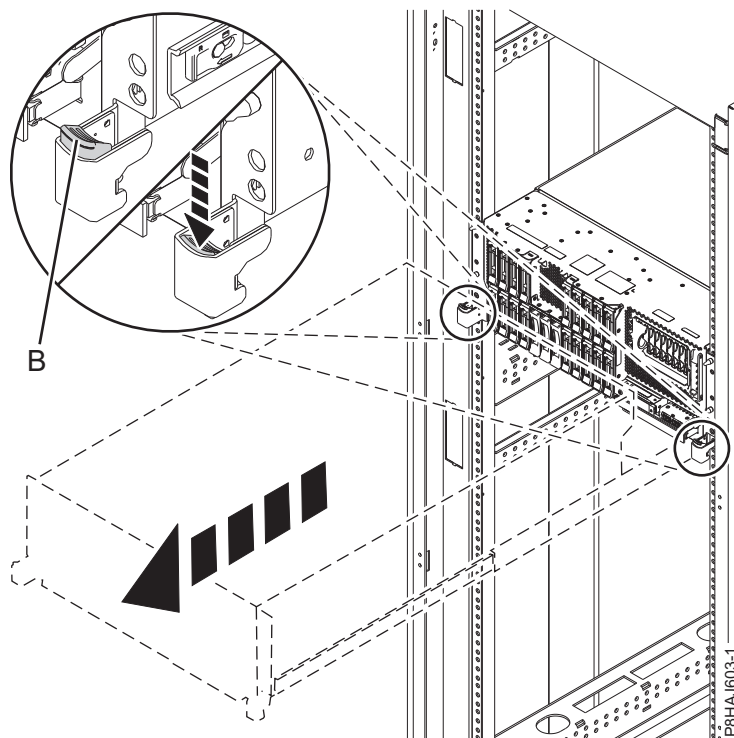
Abbildung 36. Seitliche Verriegelungen entriegeln
