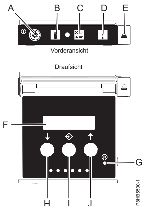
Abbildung 10. LEDs der Steuerkonsole
