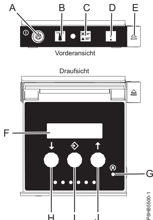
Abbildung 11. Steuerkonsole
