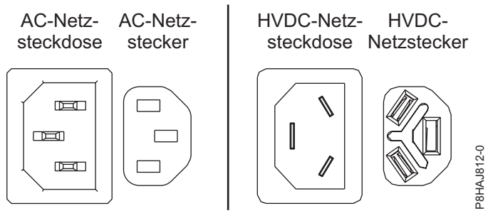
Abbildung 38. AC- und HVDC-Anschlüsse
