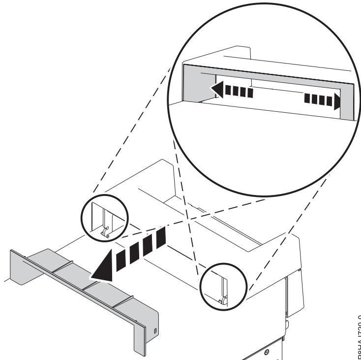
Abbildung 15. Element innerhalb der Griffabdeckung bei einem eigenständigen System vom Typ 8286-41A entfernen
