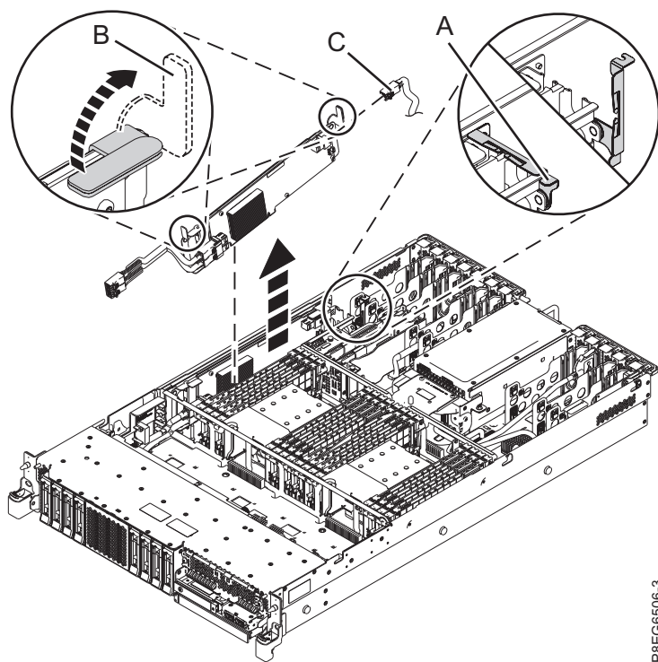
Abbildung 3. SAS-RAID-Adapter ausbauen
