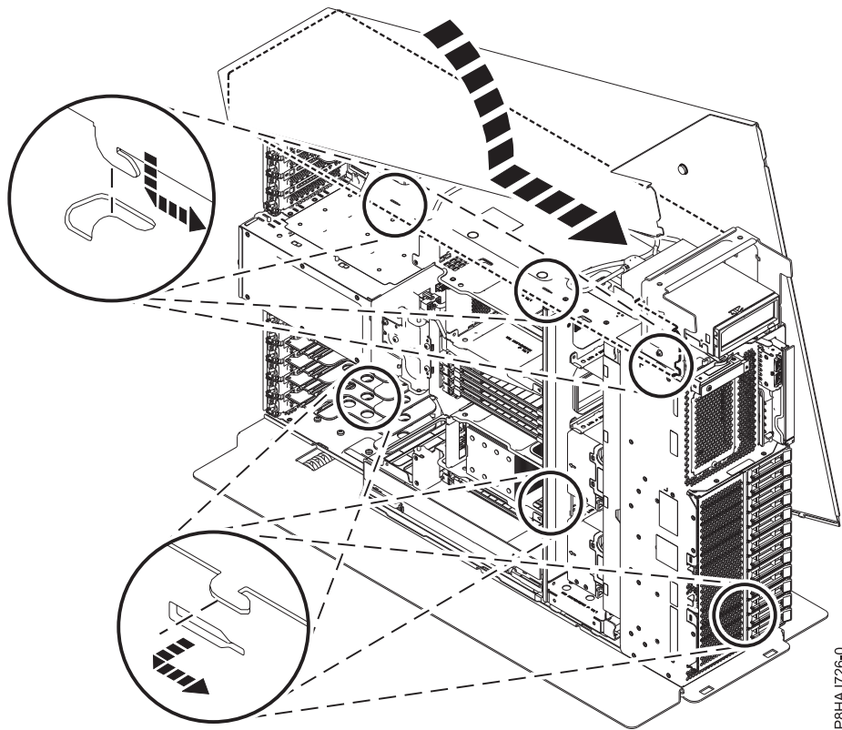
Abbildung 25. Seitenabdeckung bei einem eigenständigen System vom Typ 8286-41A installieren
