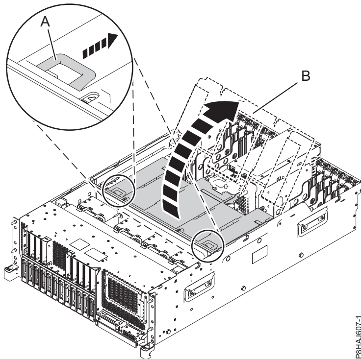
Abbildung 31. Öffnen der Luftführung
