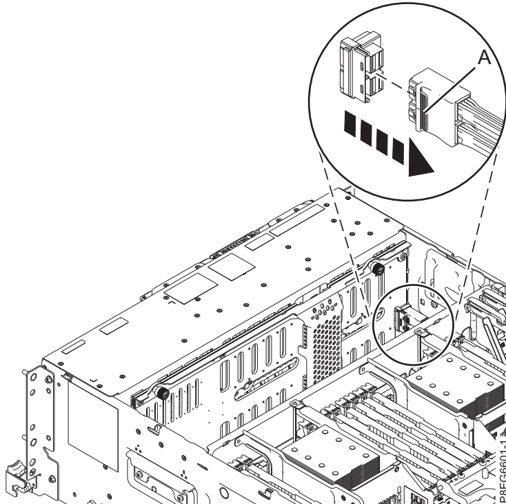
Abbildung 2. SAS-Kabel herausziehen
