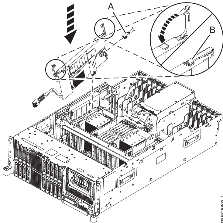
Abbildung 4. Internen SAS-RAID-Adapter austauschen
