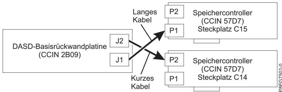
Abbildung 6. SAS-Kabel in einer Konfiguration mit unterteilter Festplatte wieder anschließen
