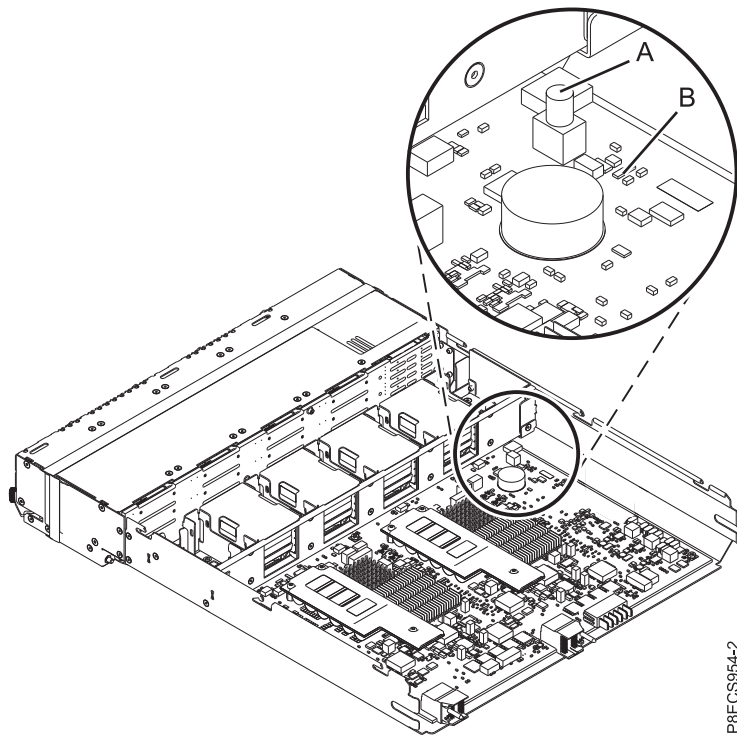
Abbildung 10. Kennzeichnungs-LED aktivieren
