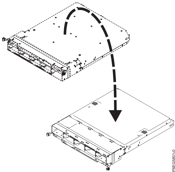
Abbildung 8. RAID-Baugruppe umdrehen
