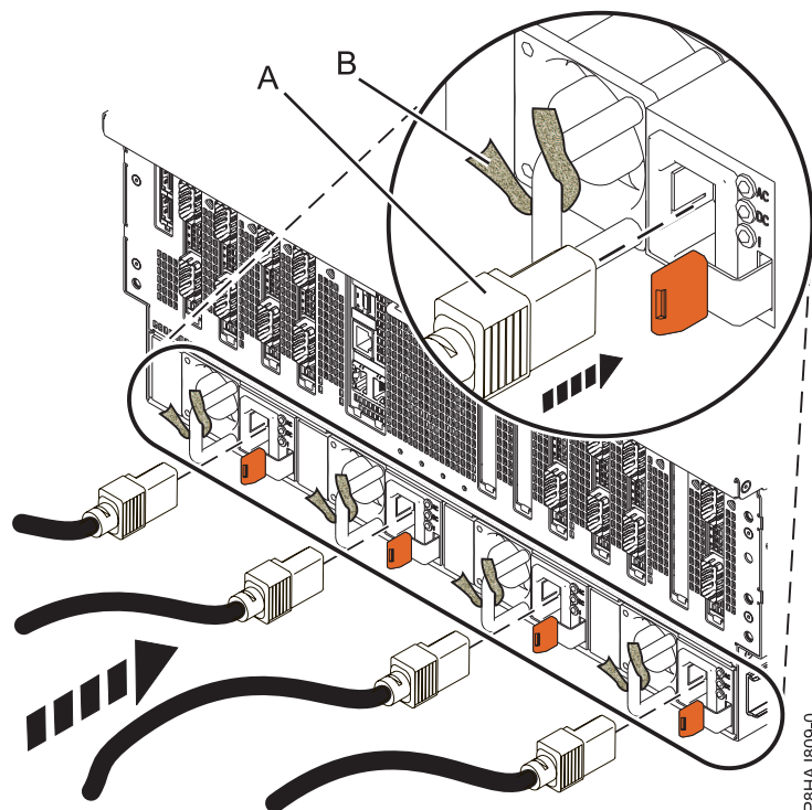
Abbildung 36. Netzkabel an ein System vom Typ 8408-44E oder 8408-E8E anschließen
