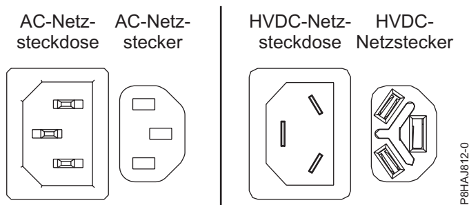
Abbildung 25. AC- und HVDC-Anschlüsse
