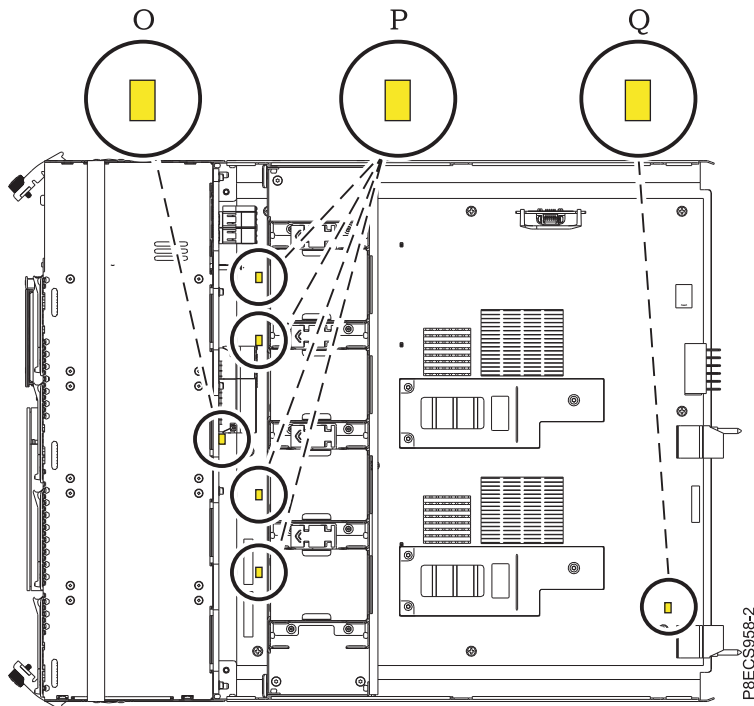
Abbildung 11. Serviceanzeigen-LEDs
