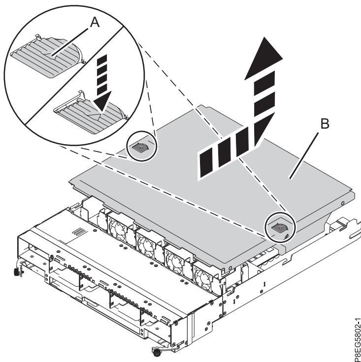
Abbildung 9. Abdeckung der RAID-Baugruppe ausbauen
