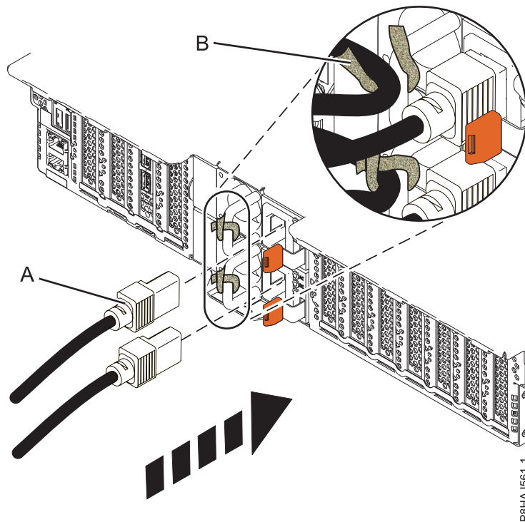
Abbildung 35. Netzkabel an ein System vom Typ 5148-21L, 5148-22L, 8247-21L, 8247-22L, 8284-21A oder 8284-22A anschließen
