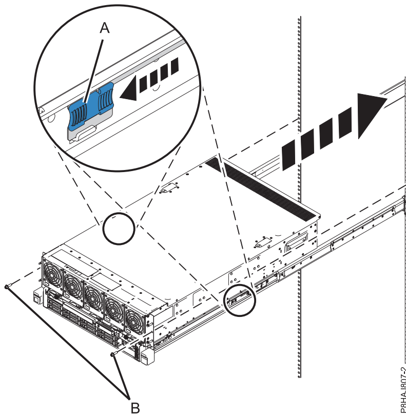
Abbildung 46. System in die Betriebsposition bringen
