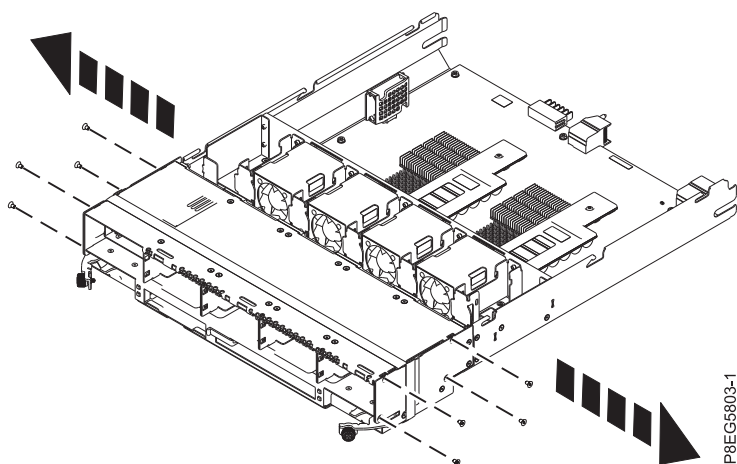
Abbildung 12. Schrauben an der RAID-Baugruppe entfernen
