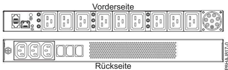
Abbildung 27. PDU beim System vom Typ 8408-44E
