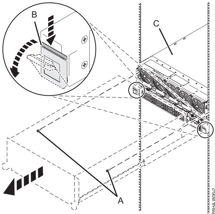
Abbildung 45. System in Serviceposition bringen
