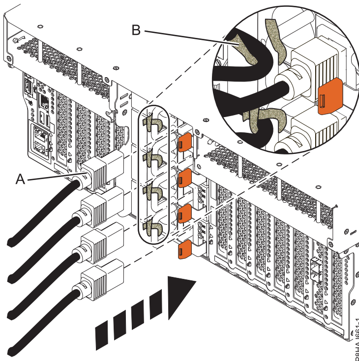
Abbildung 59. Netzkabel an ein System vom Typ 8247-42L, 8286-41A oder 8286-42A anschließen
