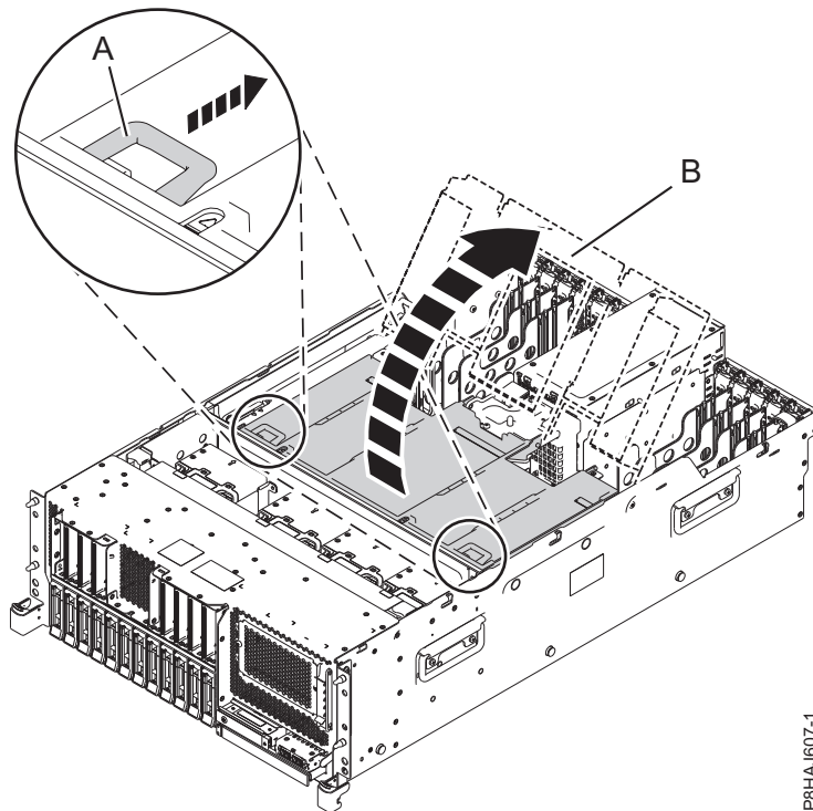
Abbildung 43. Öffnen der Luftführung
