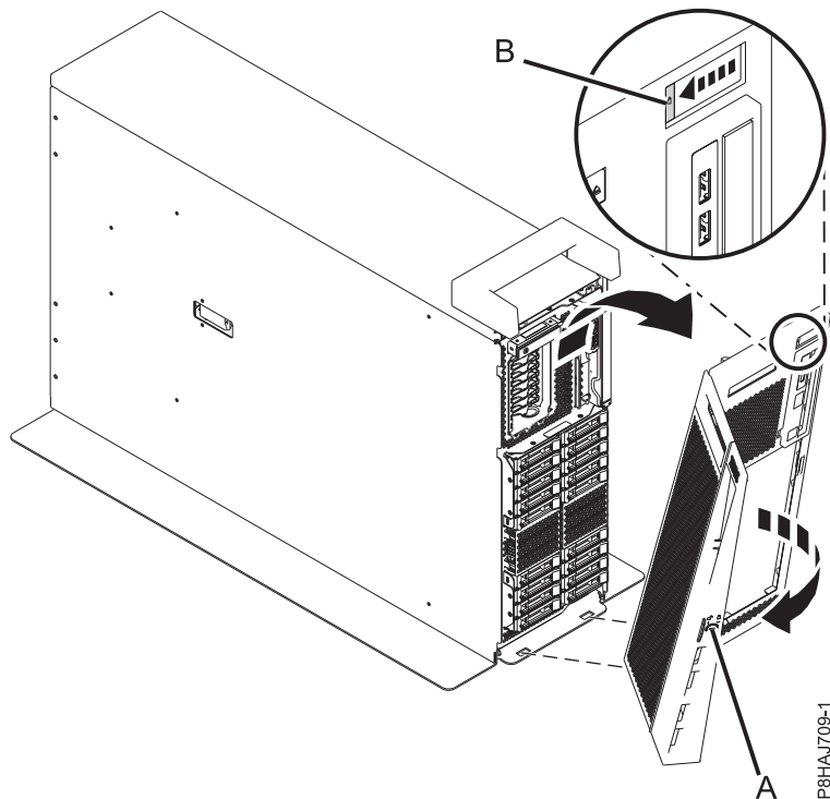
Abbildung 26. Vordere Abdeckung ausbauen
