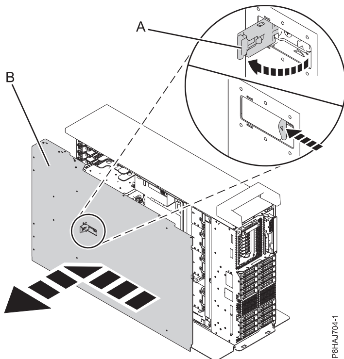
Abbildung 40. Serviceabdeckung ausbauen
