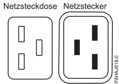
Abbildung 57. Anschlüsse beim System vom Typ 8408-44E
