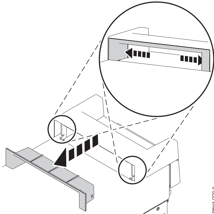
Abbildung 27. Entfernen des Elements innerhalb der Griffabdeckung bei einem Standalone-System vom Typ 8286-41A
