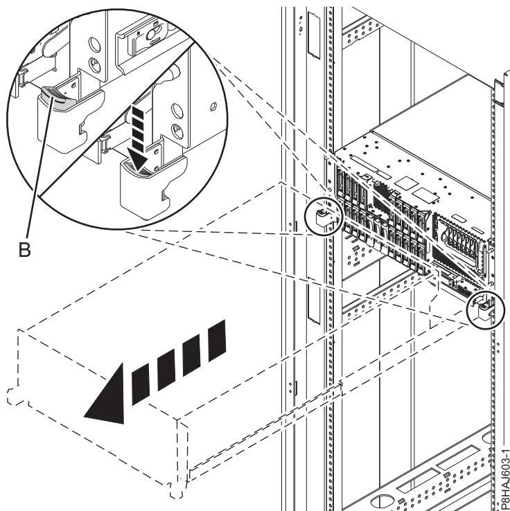
Abbildung 48. Seitliche Verriegelungen entriegeln
