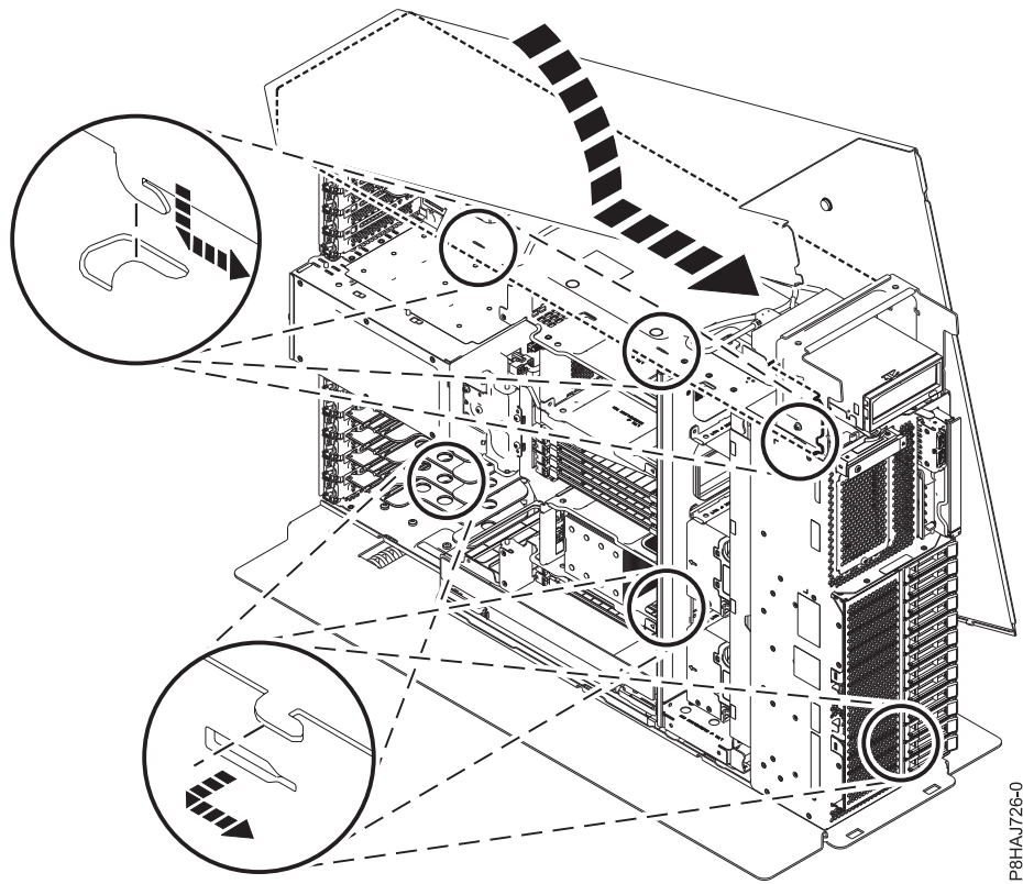
Abbildung 37. Installieren der Seitenabdeckung bei einem Standalone-System vom Typ 8286-41A
