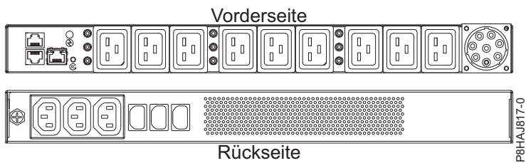
Abbildung 58. PDU beim System vom Typ 8408-44E
