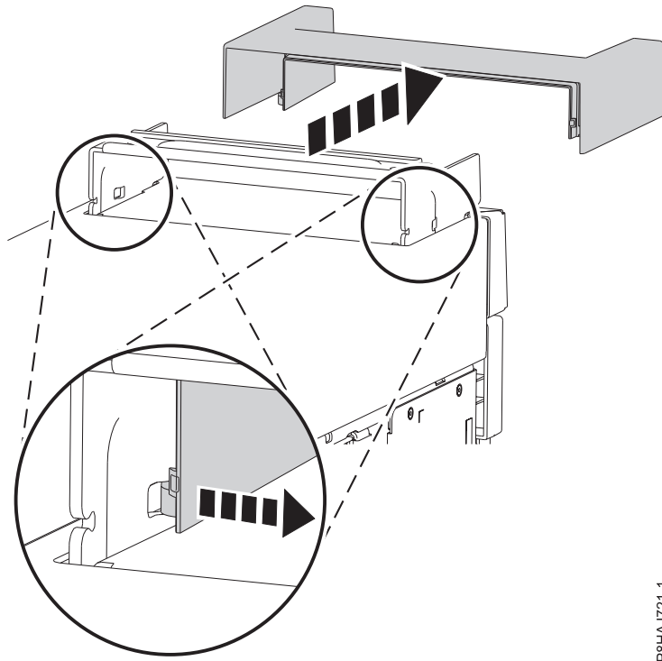
Abbildung 28. Ausbauen der Griffabdeckung bei einem Standalone-System vom Typ 8286-41A
