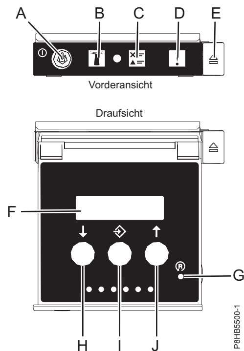
Abbildung 22. LEDs der Steuerkonsole
