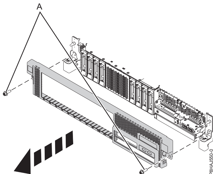
Abbildung 24. Vordere Abdeckung ausbauen
