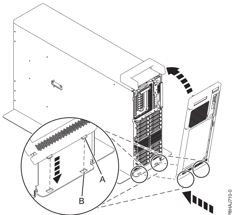
Abbildung 33. Vordere Abdeckung installieren
