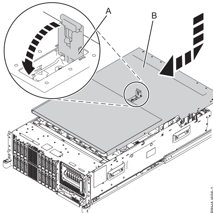
Abbildung 41. Serviceabdeckung installieren
