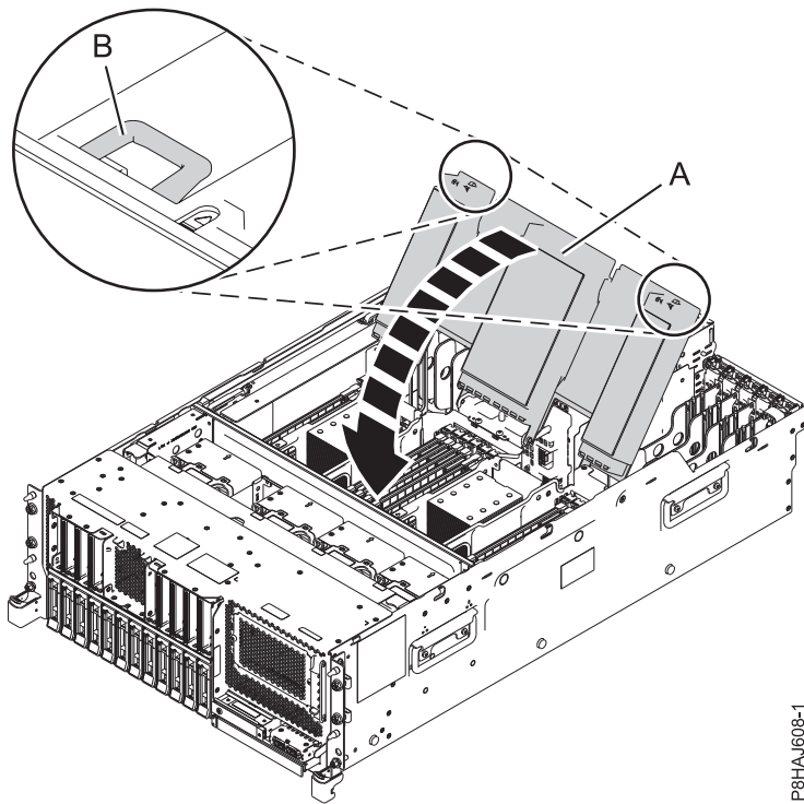
Abbildung 44. Schließen der Luftführung
