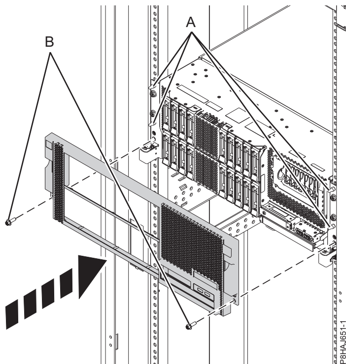
Abbildung 32. Vordere Abdeckung installieren
