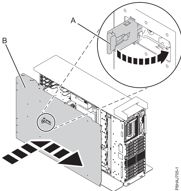
Abbildung 42. Serviceabdeckung installieren
