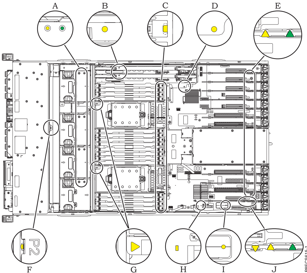
Abbildung 12. Serviceanzeigen
