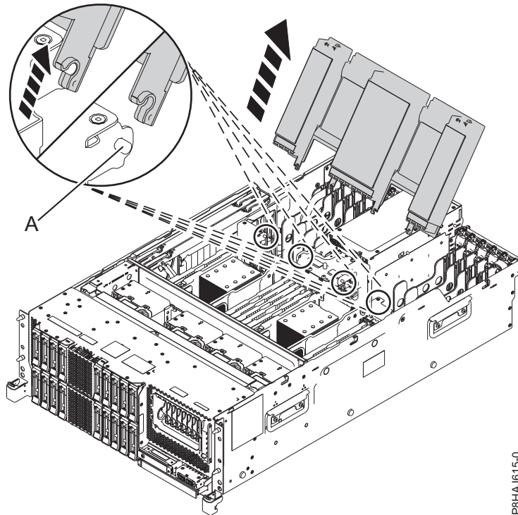
Abbildung 45. Luftführung ausbauen
