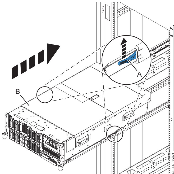
Abbildung 49. System in die Betriebsposition bringen
