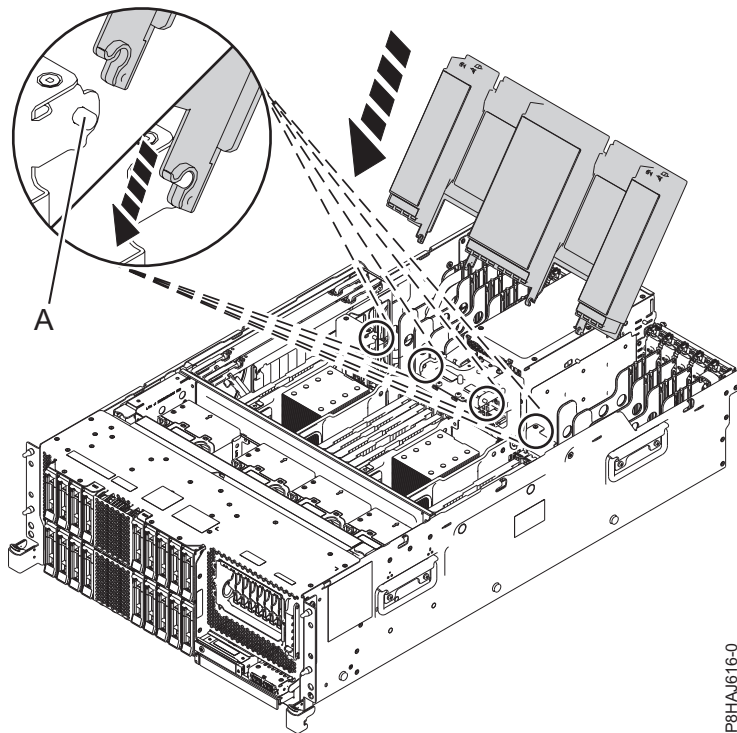
Abbildung 46. Luftführung installieren
