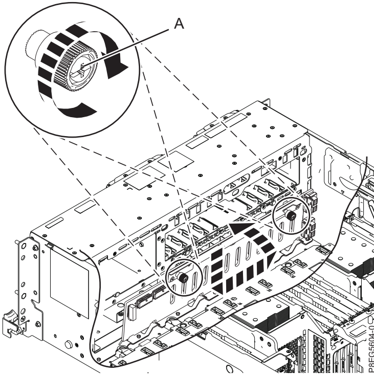
Abbildung 6. Plattenlaufwerksrückwandplatine wiedereinbauen
