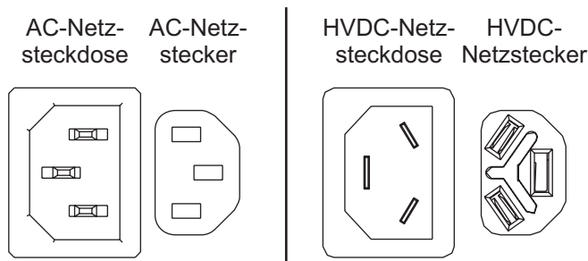
Abbildung 56. AC- und HVDC-Anschlüsse
