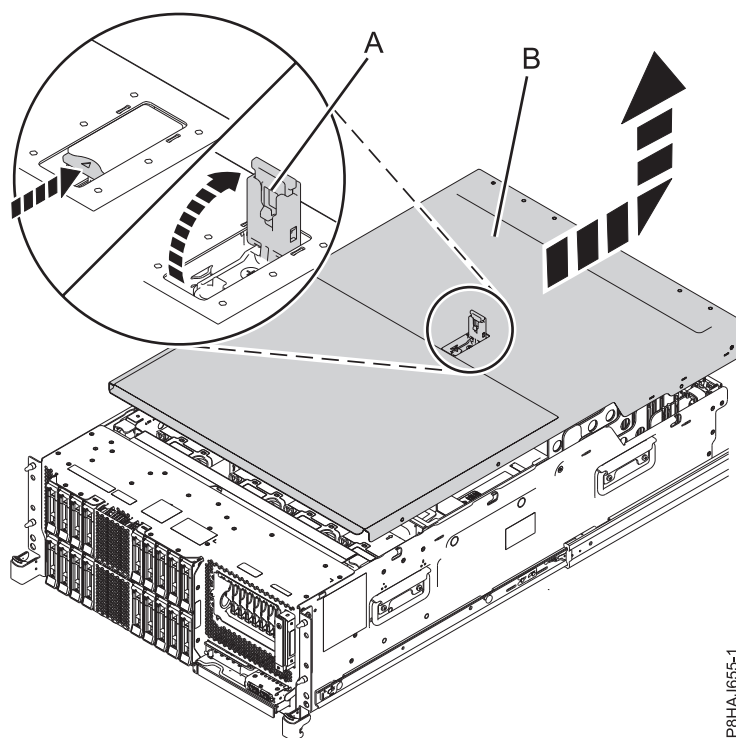
Abbildung 39. Serviceabdeckung ausbauen
