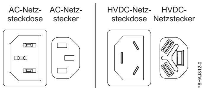
Abbildung 50. AC- und HVDC-Anschlüsse
