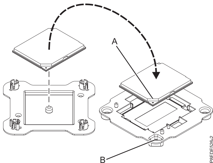
Abbildung 45. Platzieren des Systemprozessormoduls in der Verpackung
