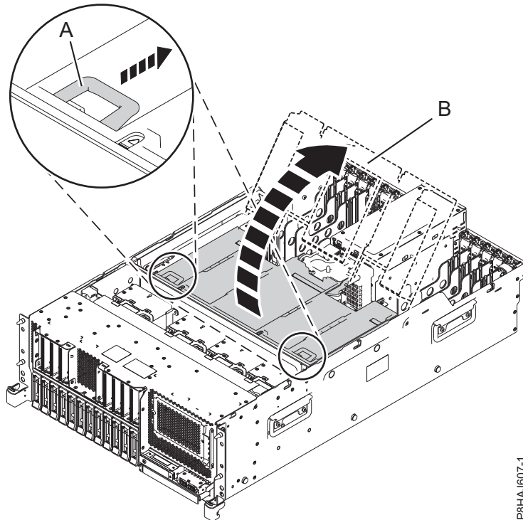
Abbildung 67. Öffnen der Luftführung
