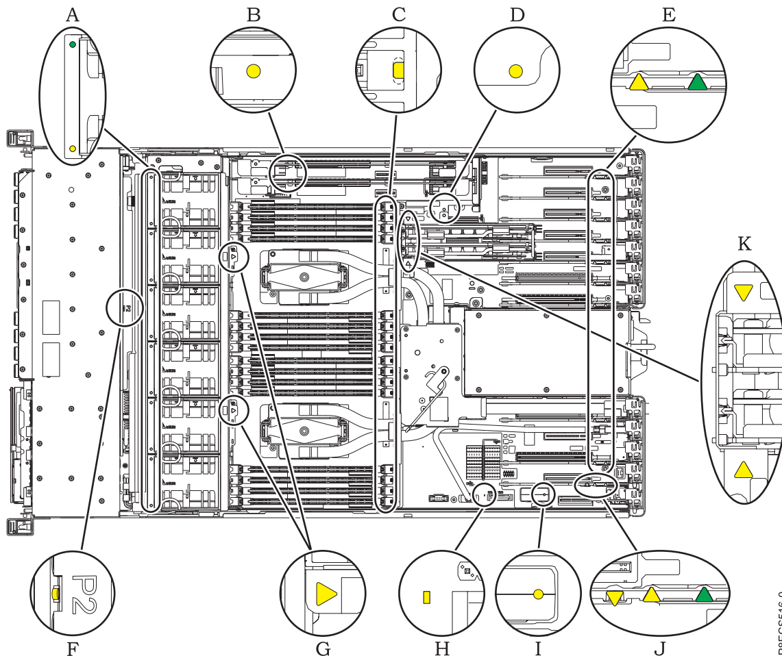
Abbildung 22. Serviceanzeigen-LEDs
