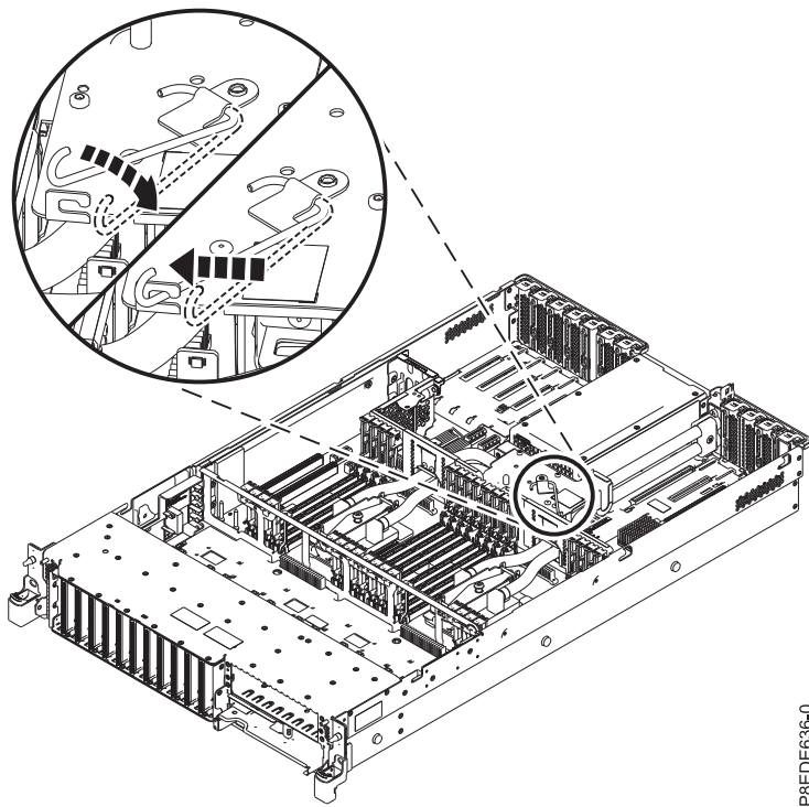
Abbildung 43. Servicehaken an die verriegelte Position zurückdrehen
