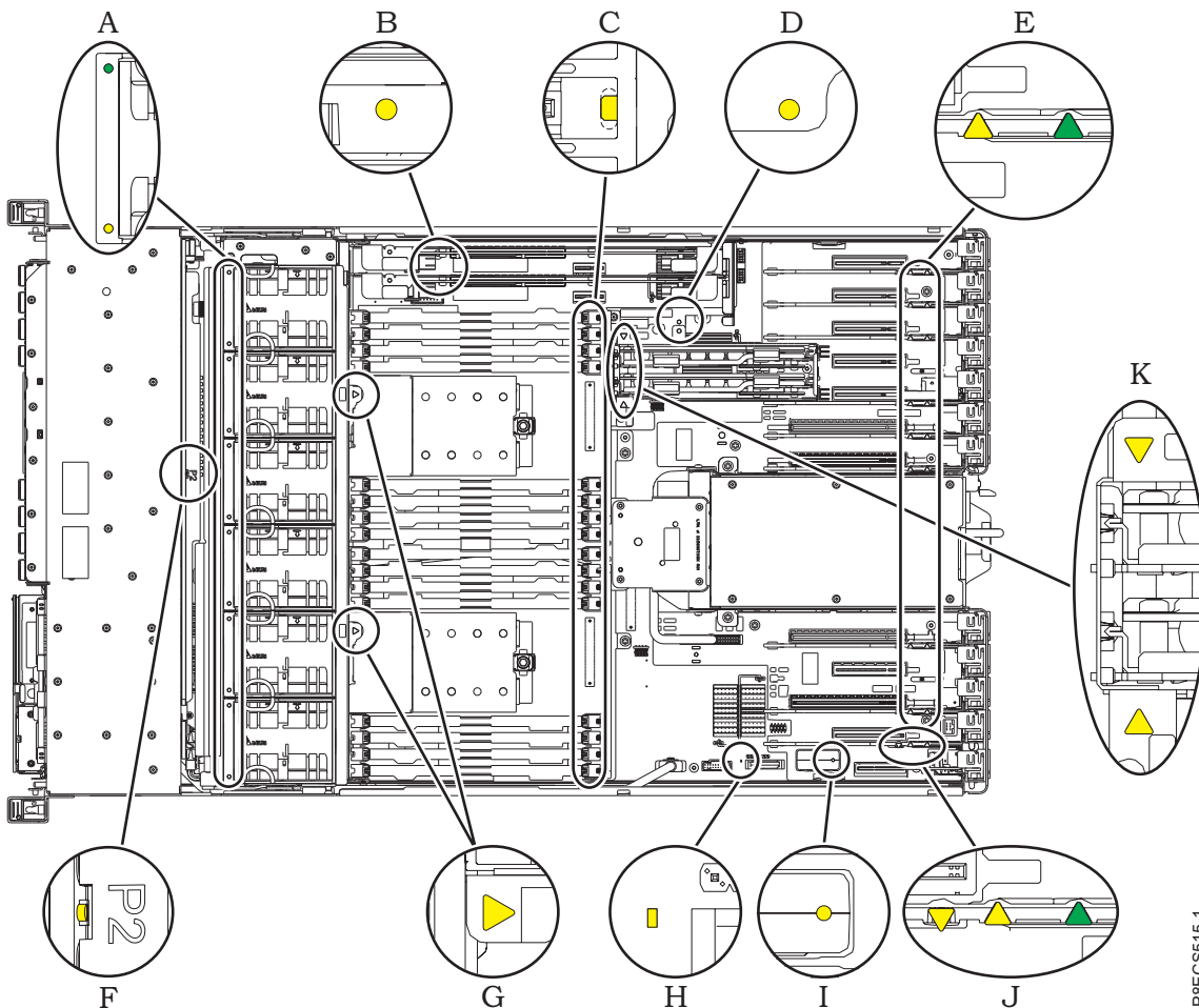
Abbildung 1. Serviceanzeigen
