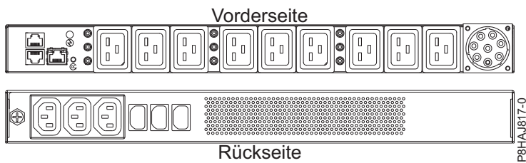
Abbildung 82. PDU beim System vom Typ 8408-44E
