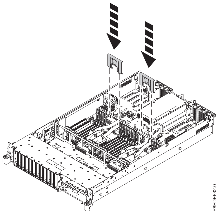
Abbildung 44. Trennwände an den korrekten Positionen absenken
