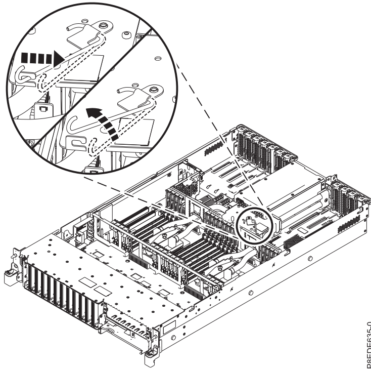
Abbildung 25. Servicehaken entriegeln
