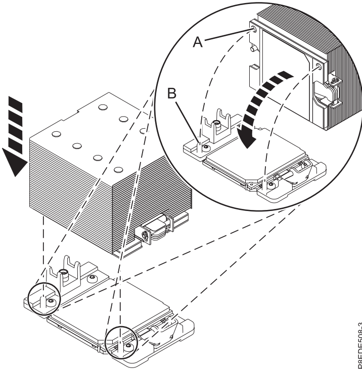
Abbildung 18. Installieren des Kühlblechs
