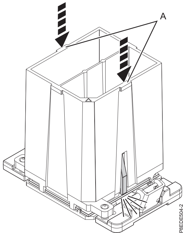
Abbildung 7. Systemprozessormodul im Werkzeug einrasten lassen
