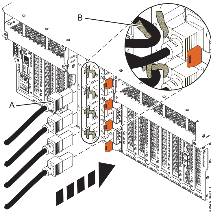
Abbildung 83. Netzkabel an ein System vom Typ 8247-42L, 8286-41A oder 8286-42A anschließen
