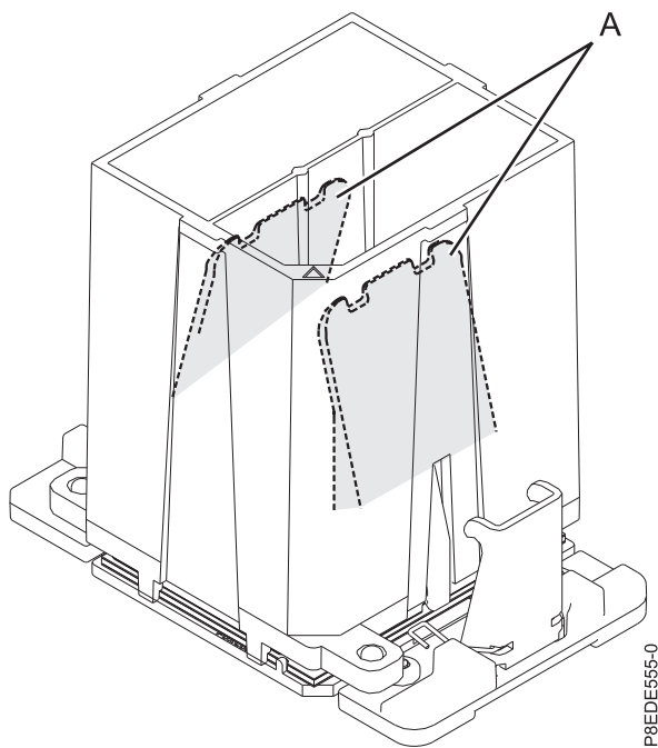
Abbildung 38. Werkzeug vom Systemprozessormodul trennen
