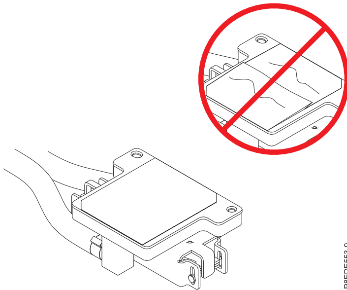
Abbildung 39. Material der Thermoschicht (Thermal Interface Material, TIM) überprüfen
