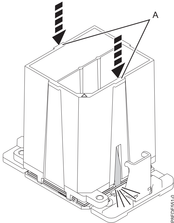
Abbildung 30. Systemprozessormodul im Werkzeug einrasten lassen
