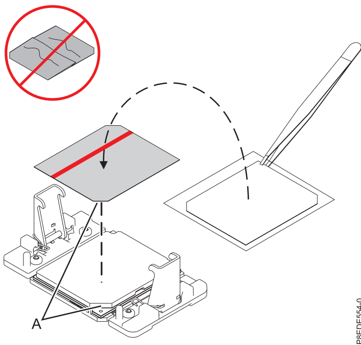
Abbildung 40. Material der Thermoschicht (Thermal Interface Material, TIM) austauschen
