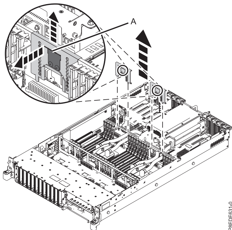
Abbildung 24. Trennwand entfernen
