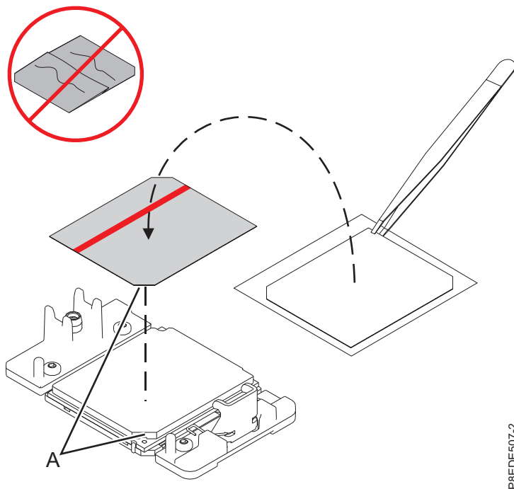
Abbildung 17. Installieren des TIM auf der Prozessorabdeckung
