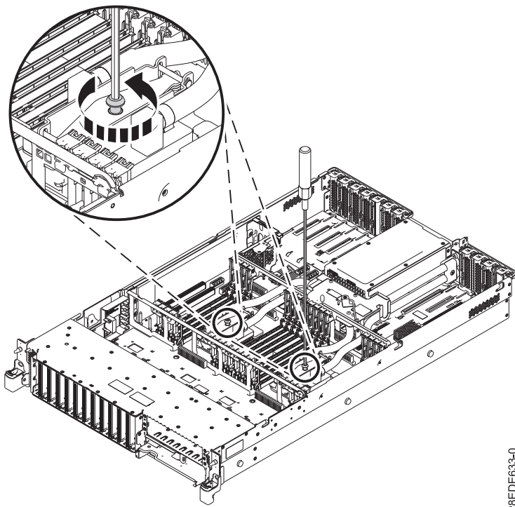
Abbildung 26. Halteschraube an der gekühlten Platte lösen
