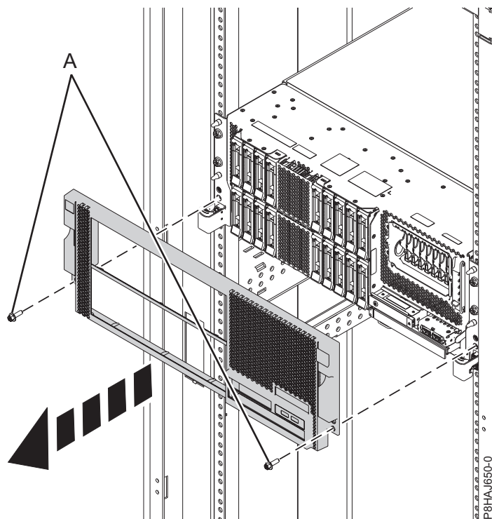
Abbildung 23. Vordere Abdeckung ausbauen
