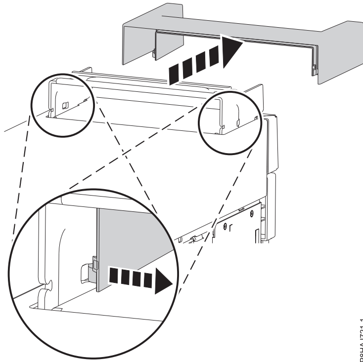
Abbildung 26. Ausbauen der Griffabdeckung bei einem Standalone-System vom Typ 8286-41A
