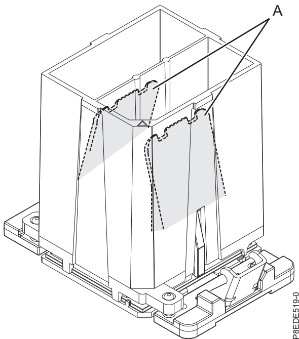
Abbildung 14. Trennen des Werkzeugs vom Systemprozessormodul
