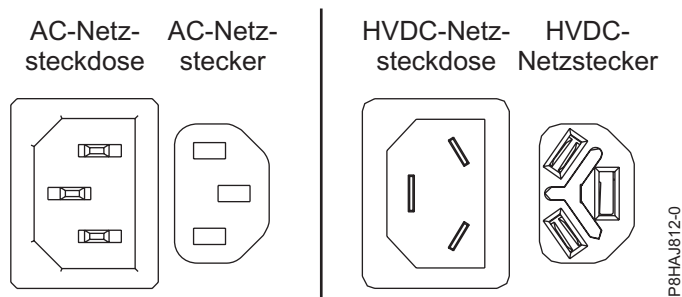
Abbildung 48. AC- und HVDC-Anschlüsse
