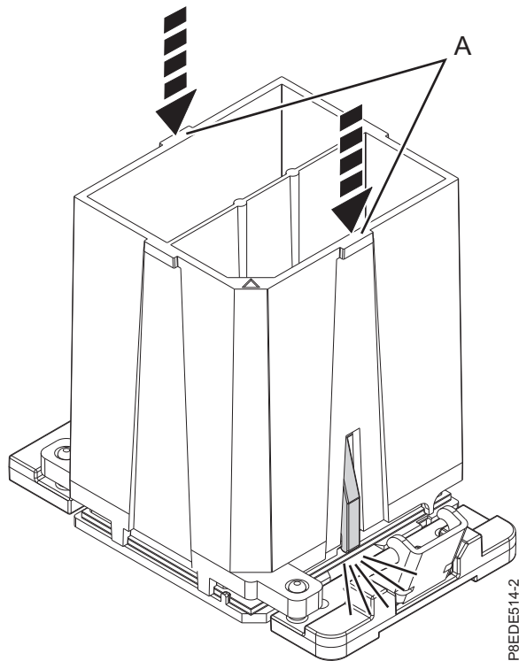
Abbildung 6. Systemprozessormodul im Werkzeug einrasten lassen
