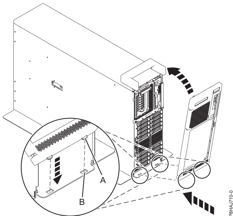
Abbildung 31. Vordere Abdeckung installieren
