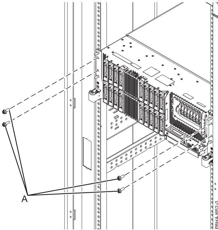
Abbildung 45. Entfernen der vorderen Schrauben
