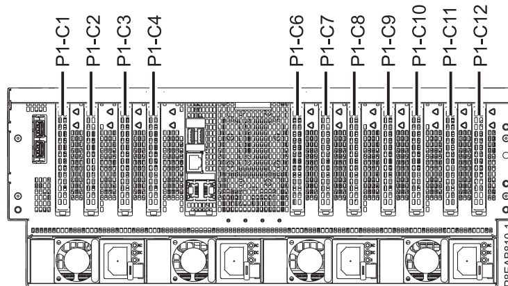
Abbildung 1. Rückansicht eines Systems vom Typ 8408-44E oder 8408-E8E mit Positionscodes der PCIe-Steckplätze
