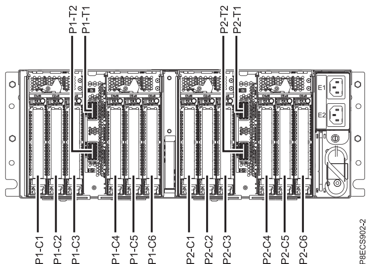
Abbildung 2. Rückansicht des Einschubs für PCIe3-Erweiterungen mit Positionscodes der PCIe-Steckplätze
