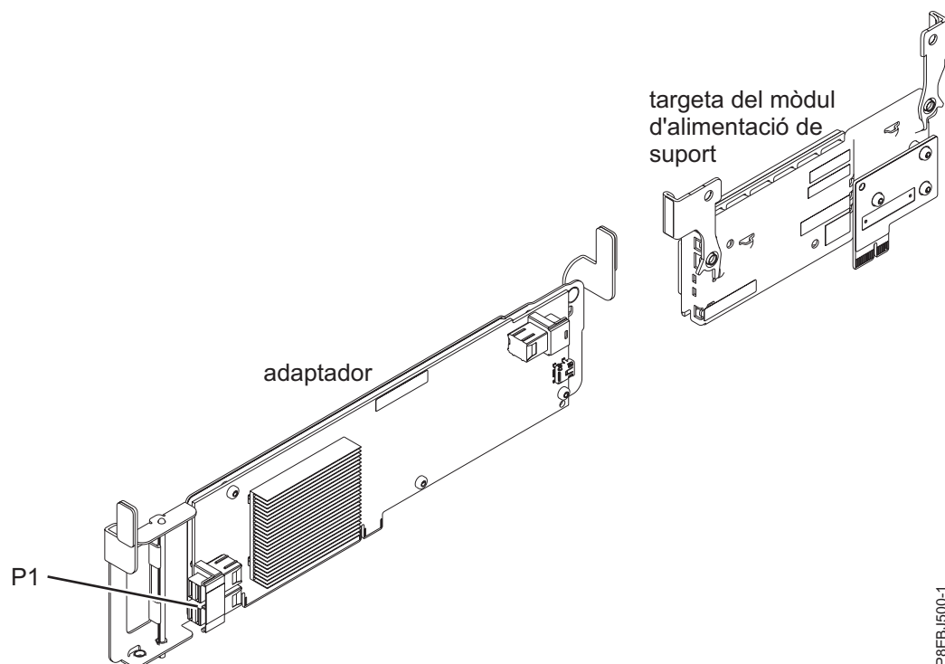
Figura 55. adaptador intern SAS RAID PCIe3 x8 de memòria cau de 6Gb
