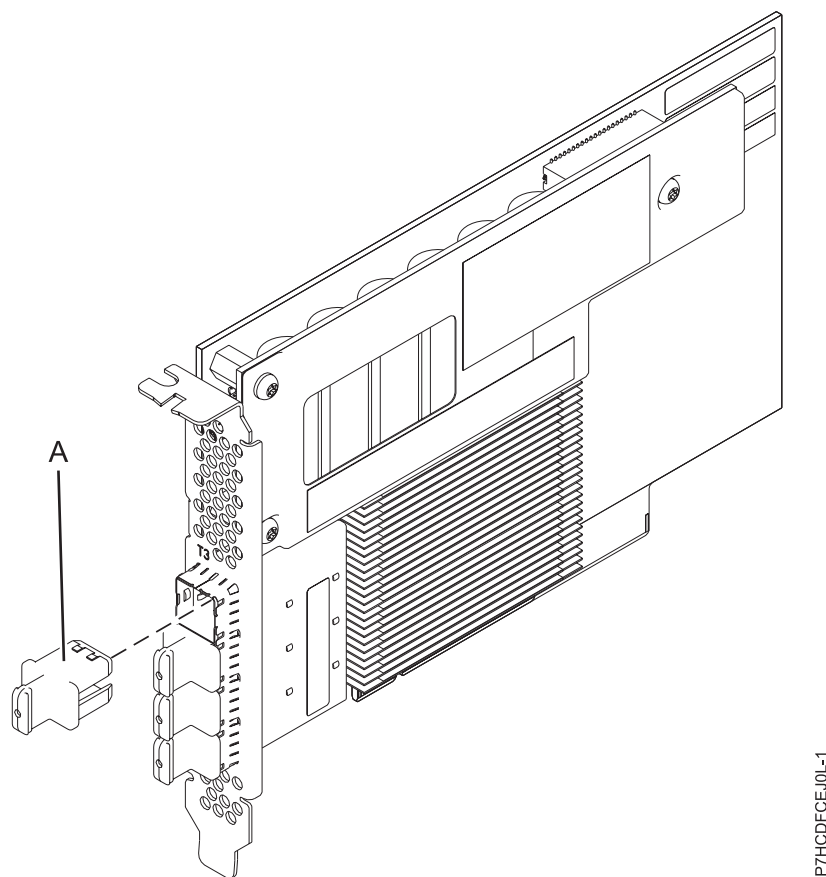
Figura 14. Adaptador SAS RAID PCIe3 amb 12 GB memòria cau i 6 Gb
