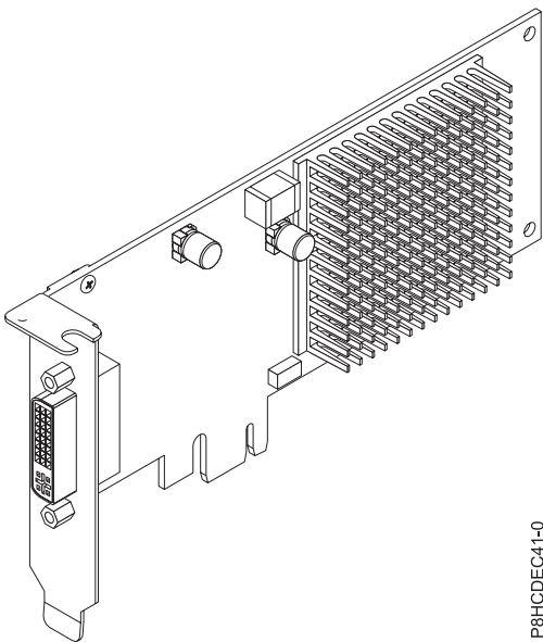
Figura 13. adaptador de gràfics PCIe2 LP 3D
