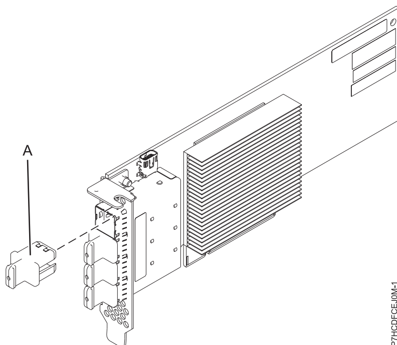
Figura 16. Adaptador de ports PCIe3 LP 4 x8 SAS
