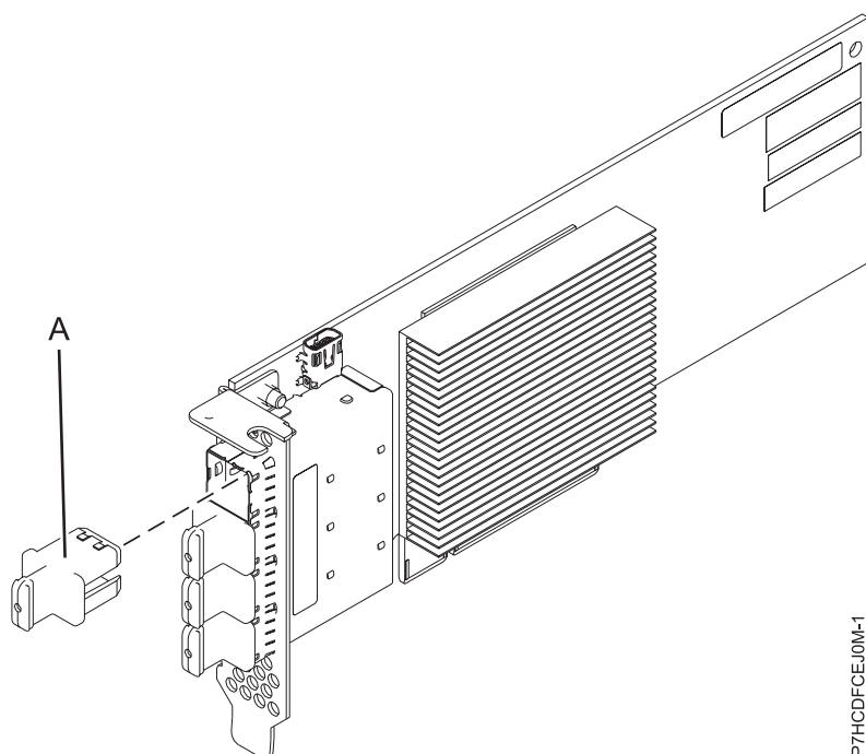
Figura 18. Adaptador de ports PCIe3 LP 4 x8 SAS
