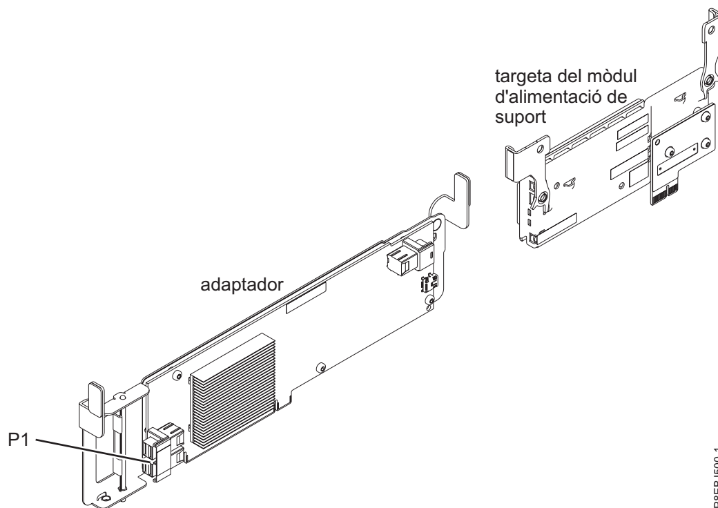
Figura 56. adaptador intern SAS RAID PCIe3 x8 de memòria cau de 6Gb
