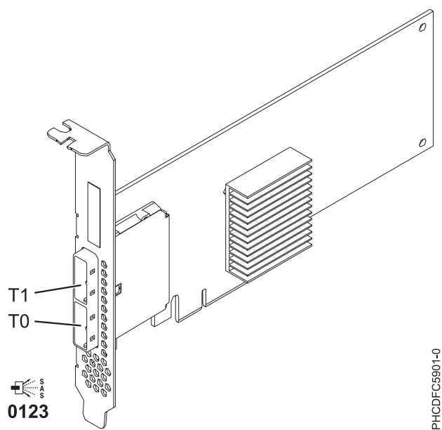
Figura 49. Adaptador SAS PCIe Dual - x4
