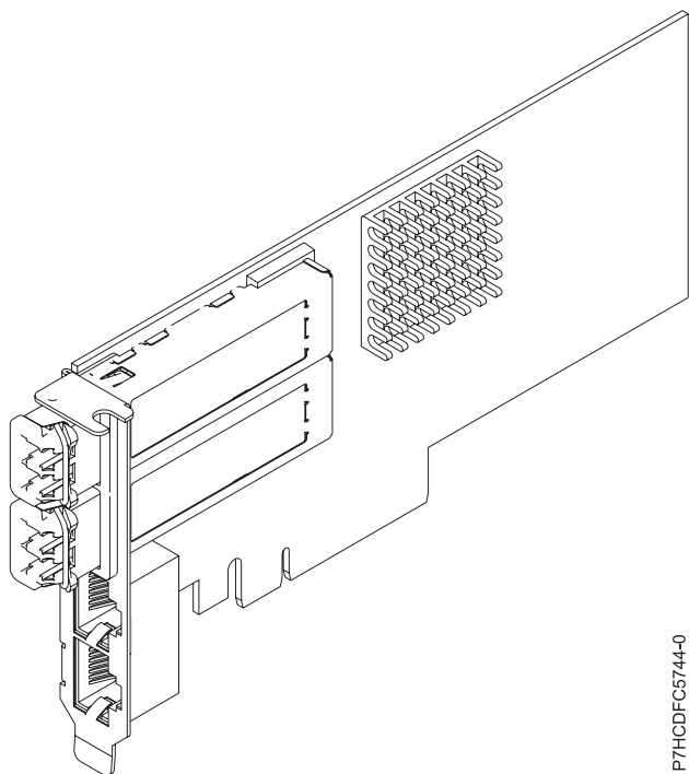
Figura 23. adaptador PCIe2 LP 2x10GbE SR 2x1GbE UTP
