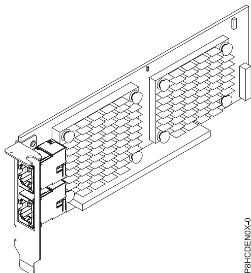
Figura 44. Adaptador FC EN0X
