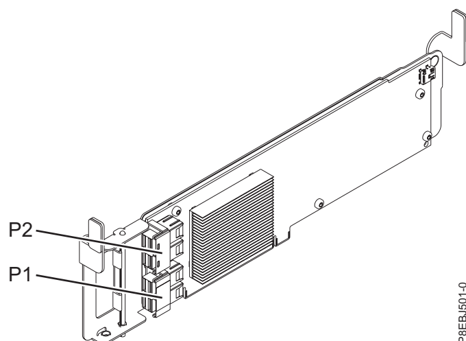
Figura 54. adaptador intern SAS RAID PCIe3 x8 de 6Gb
