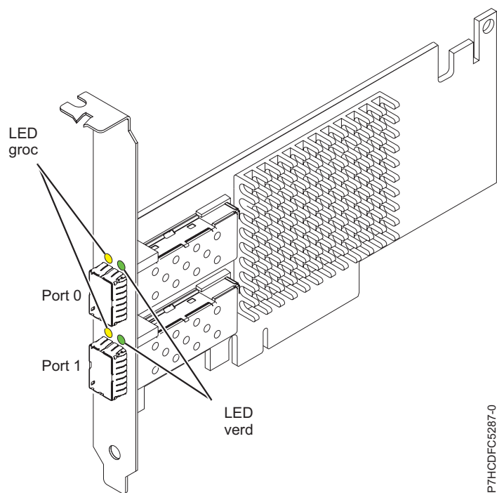
Figura 25. Adaptador SR PCIe2 LP de 2 ports i 10GbE
