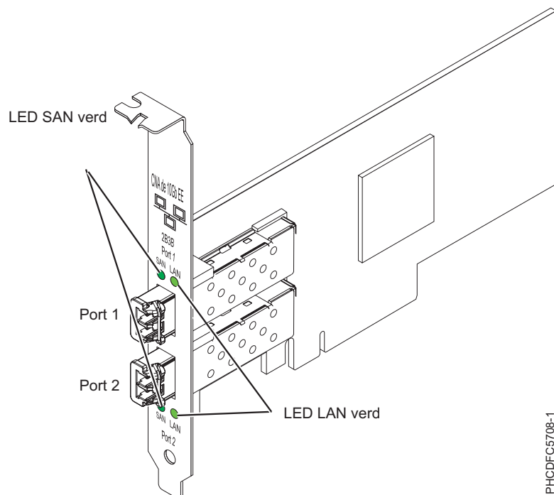
Figura 20. Adaptador de dos ports FCoE PCIe de 10 Gb
