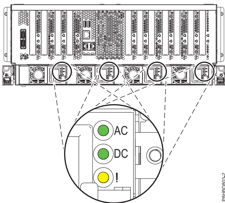
Figura 1. Ubicació de les fonts d'alimentació i dels LED al sistema 8408-44E o 8408-E8E
