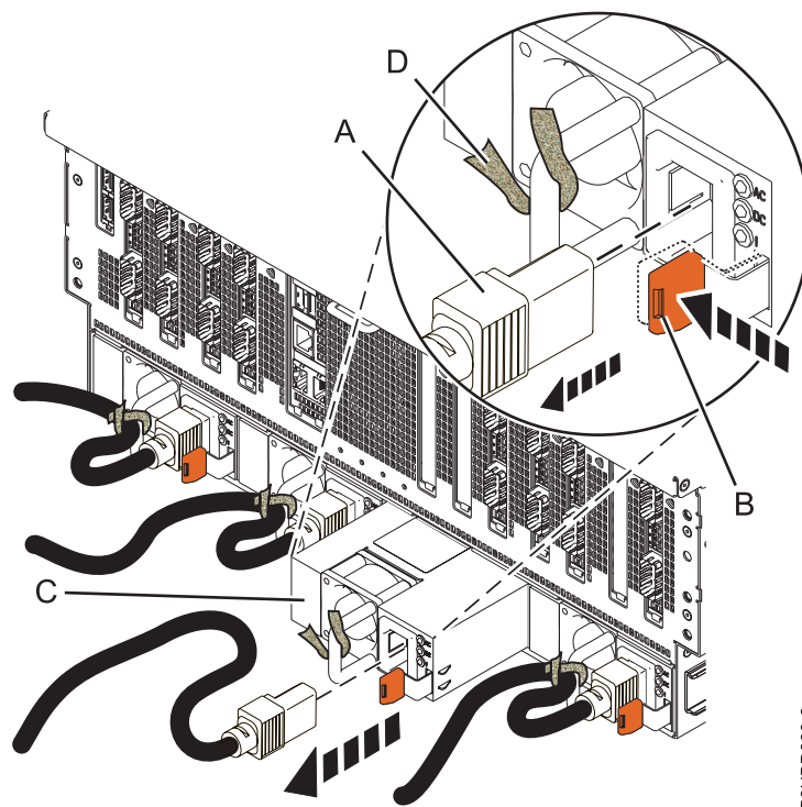
Figura 4. Extracció d'una font d'alimentació del sistema 8408-E8E
