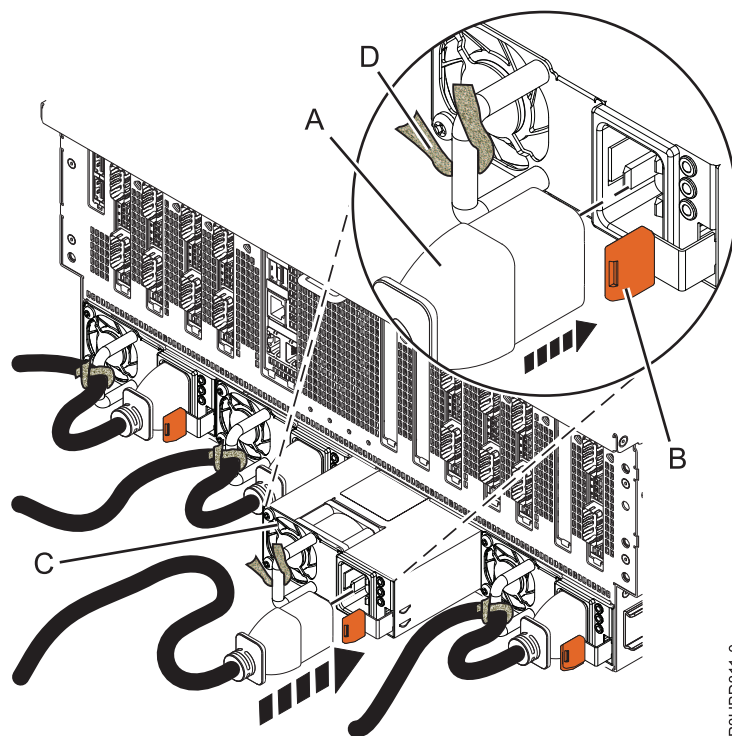
Figura 5. Substitució d'una font d'alimentació al sistema 8408-44E
