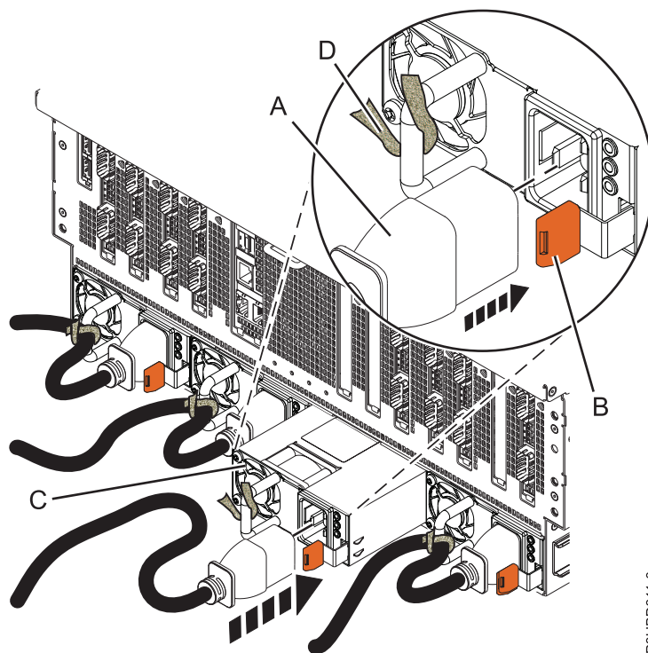
Figura 12. Substitució d'una font d'alimentació al sistema 8408-44E
