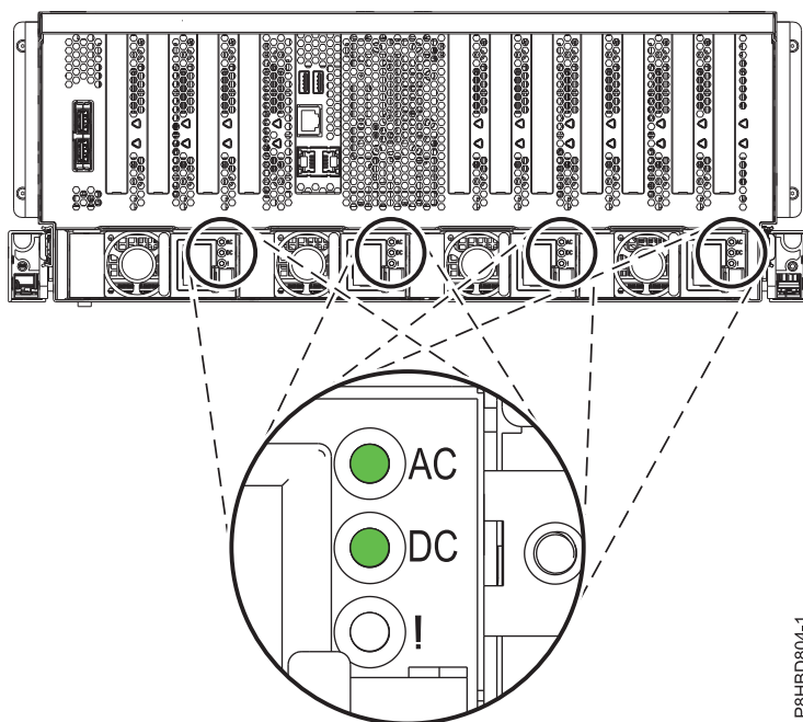
Figura 7. LED d'una font d'alimentació en funcionament
