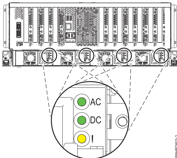
Figura 8. Ubicació de les fonts d'alimentació i dels LED en un sistema 8408-44E o 8408-E8E
