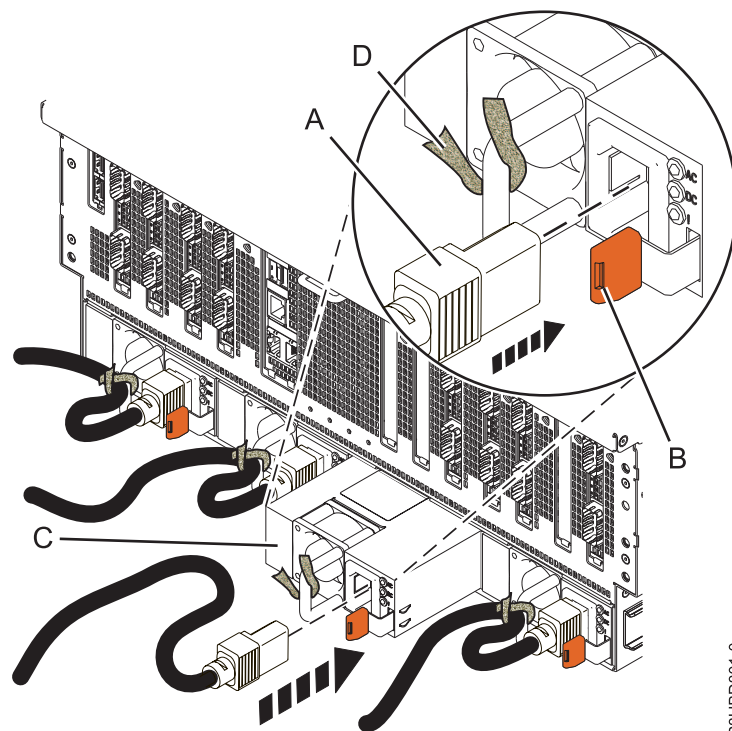
Figura 6. Substitució d'una font d'alimentació al sistema 8408-E8E
