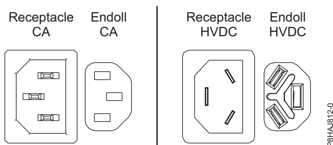
Figura 23. Connectors de CA i d'HVDC
