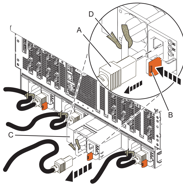
Figura 11. Extracció d'una font d'alimentació del sistema 8408-E8E
