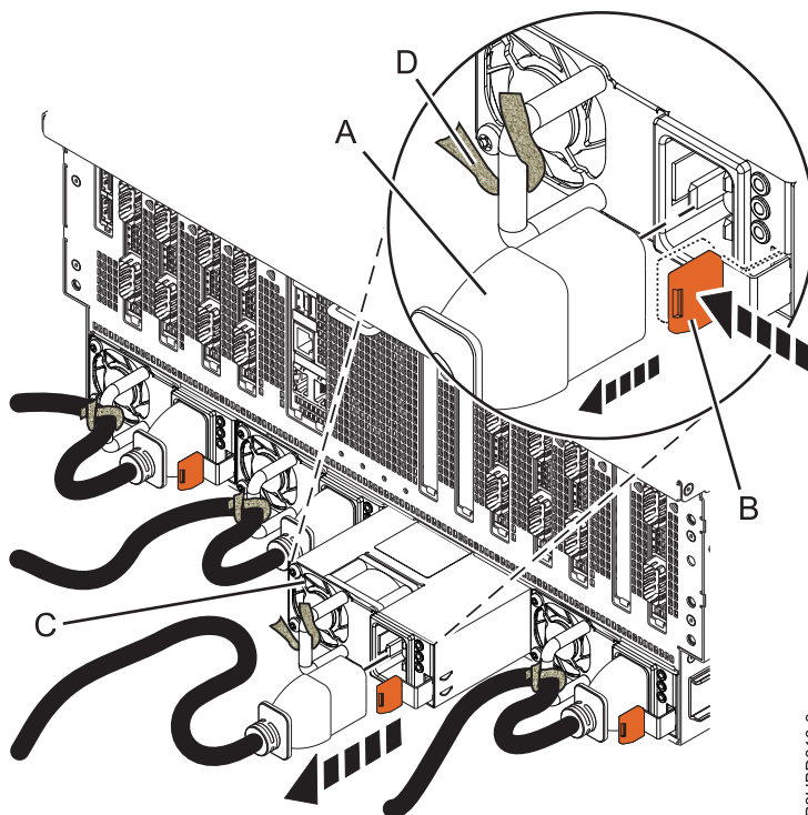
Figura 10. Extracció d'una font d'alimentació del sistema 8408-44E
