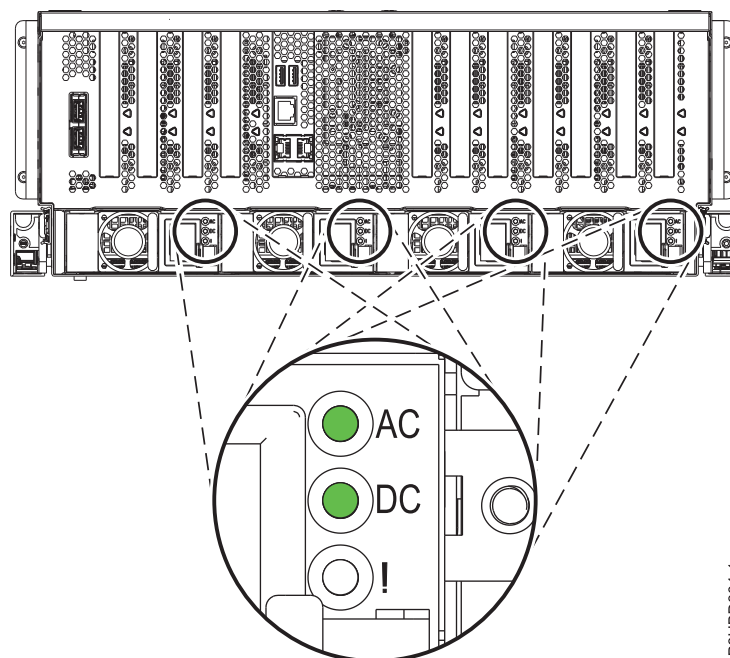
Figura 14. LED d'una font d'alimentació en funcionament
