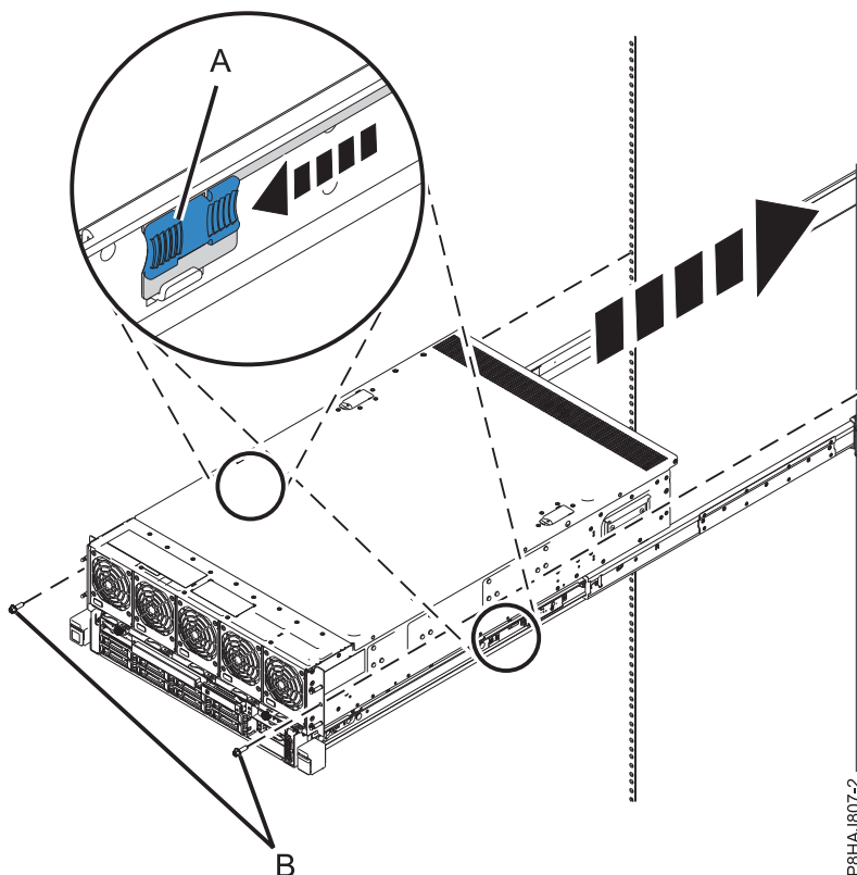
Figura 38. Col·locació del sistema en posició operativa
