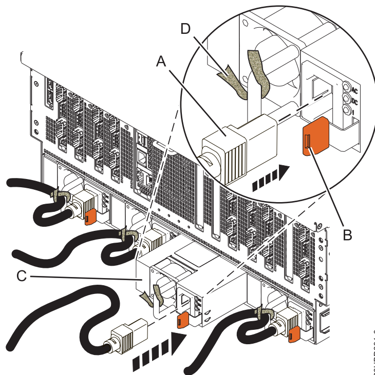
Figura 13. Substitució d'una font d'alimentació al sistema 8408-E8E
