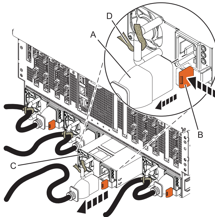
Figura 3. Extracció d'una font d'alimentació del sistema 8408-44E
