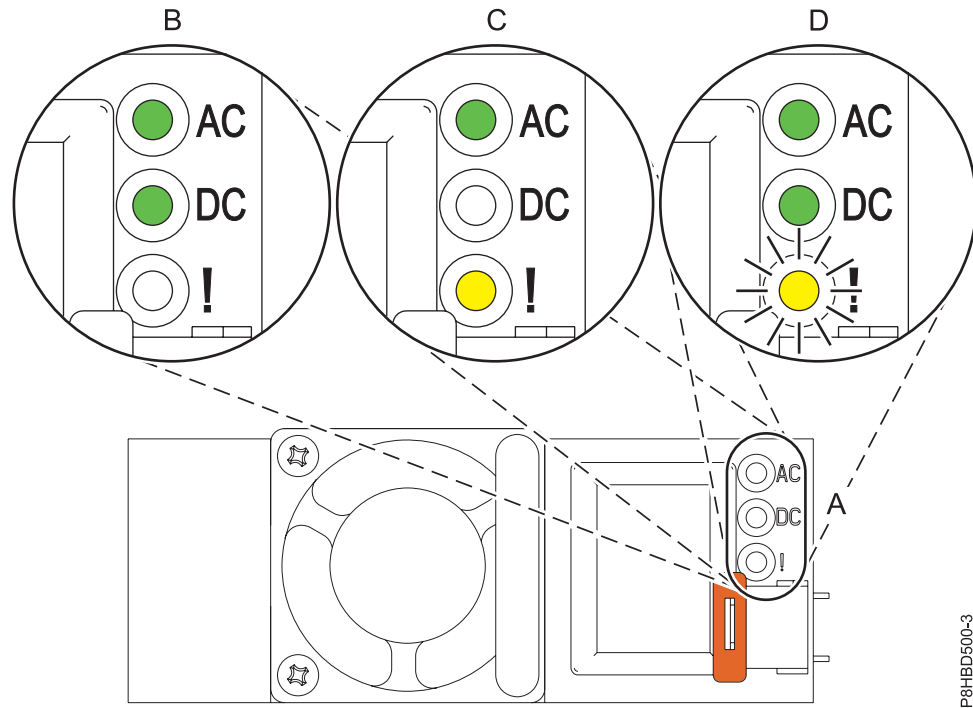
Figura 2. LED d'una font d'alimentació en funcionament i d'una que falla
