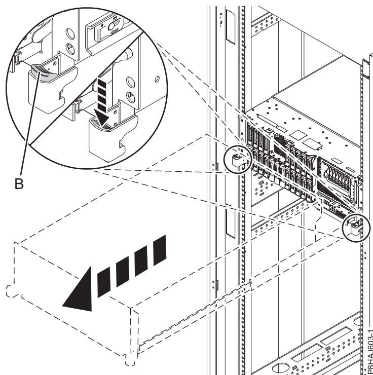
Figura 51. Alliberament dels pestells laterals
