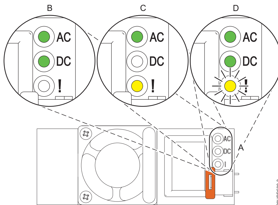
Figura 12. LED d'una font d'alimentació en funcionament i d'una que falla
