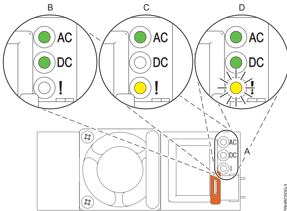
Figura 3. LED d'una font d'alimentació en funcionament i d'una que falla
