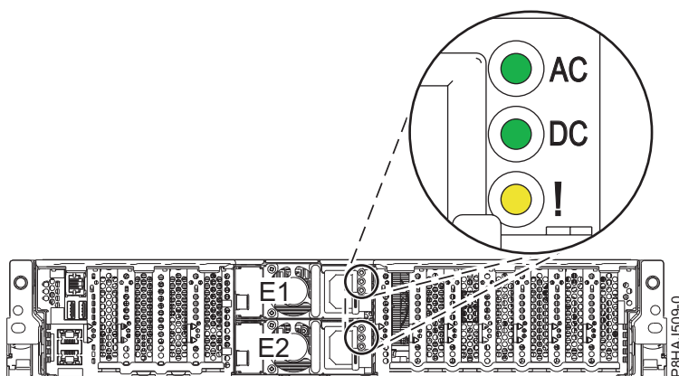
Figura 7. Ubicació de les fonts d'alimentació i dels LED del sistema
