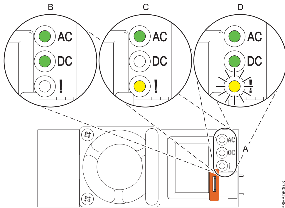
Figura 6. LED d'una font d'alimentació en funcionament i d'una que falla
