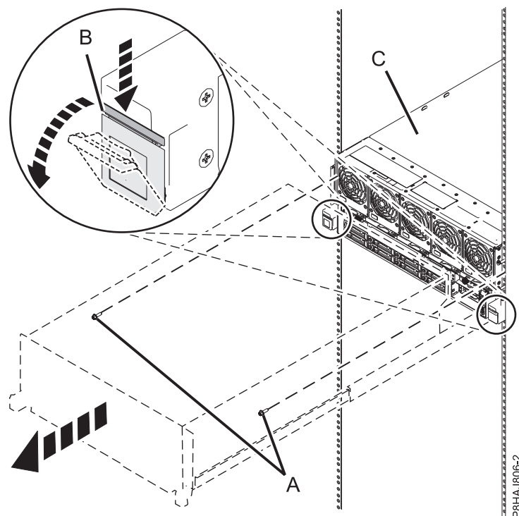
Figura 16. Col·locació del sistema en posició de servei
