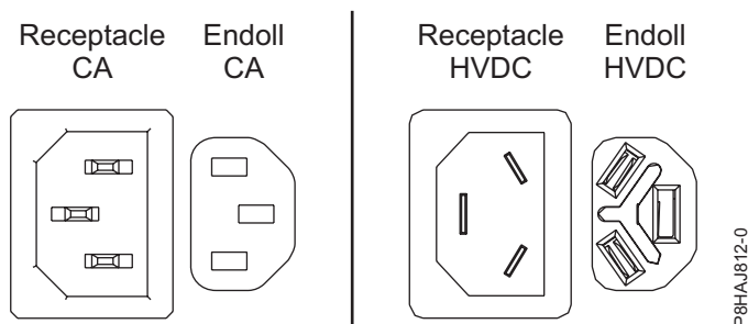
Figura 24. Connectors de CA i d'HVDC
