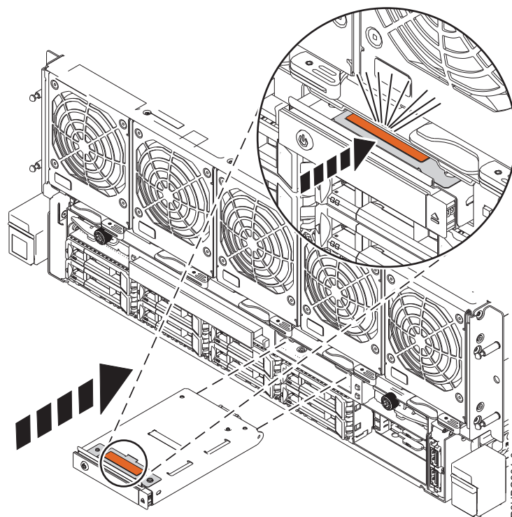
Figura 5. Substitució del tauler de control al sistema 8408-44E o 8408-E8E
