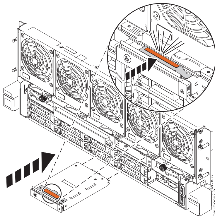
Figura 2. Substitució del tauler de control al sistema 8408-44E o 8408-E8E
