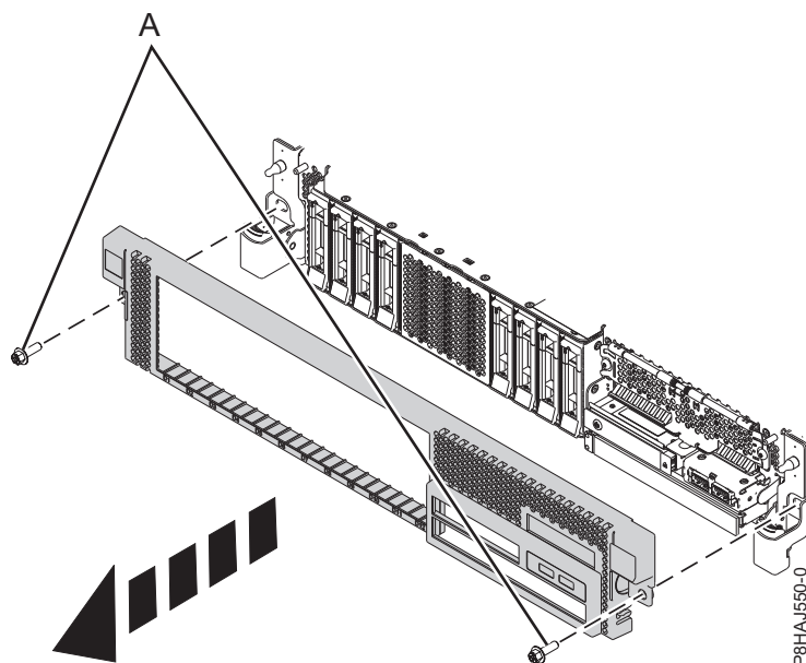
Figura 8. Extracció de la coberta frontal
