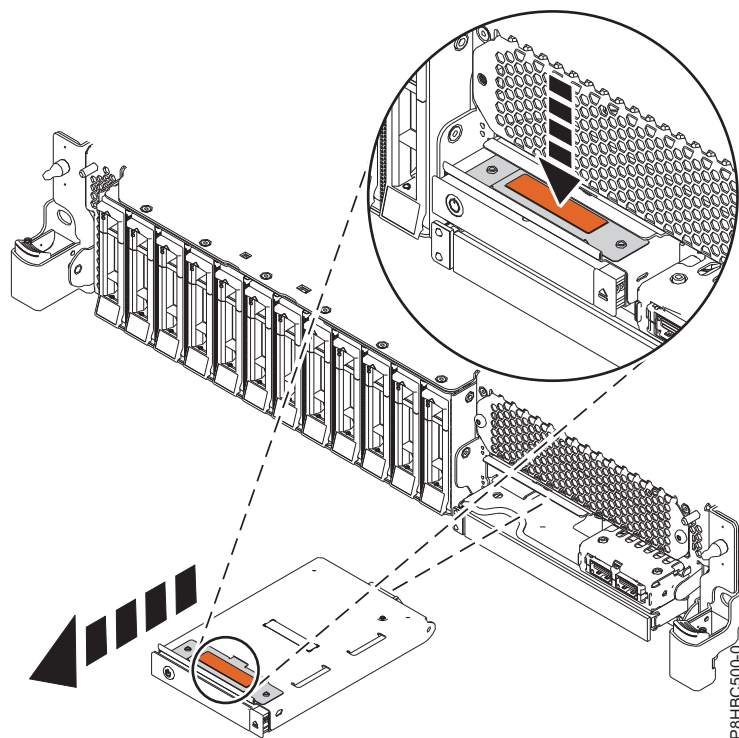
Figura 1. Extracció del tauler de control
