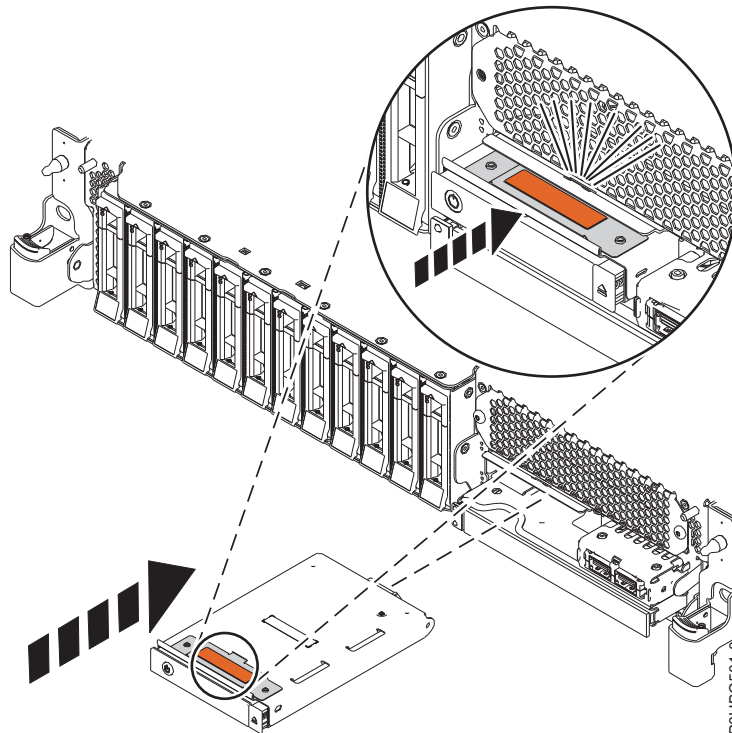
Figura 5. Substitució del tauler de control
