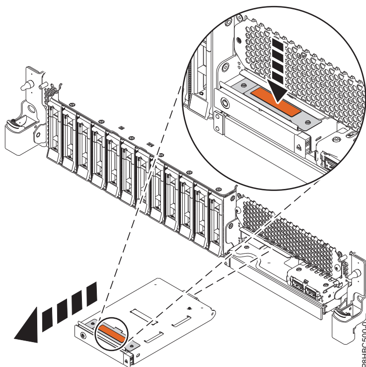
Figura 4. Extracció del tauler de control
