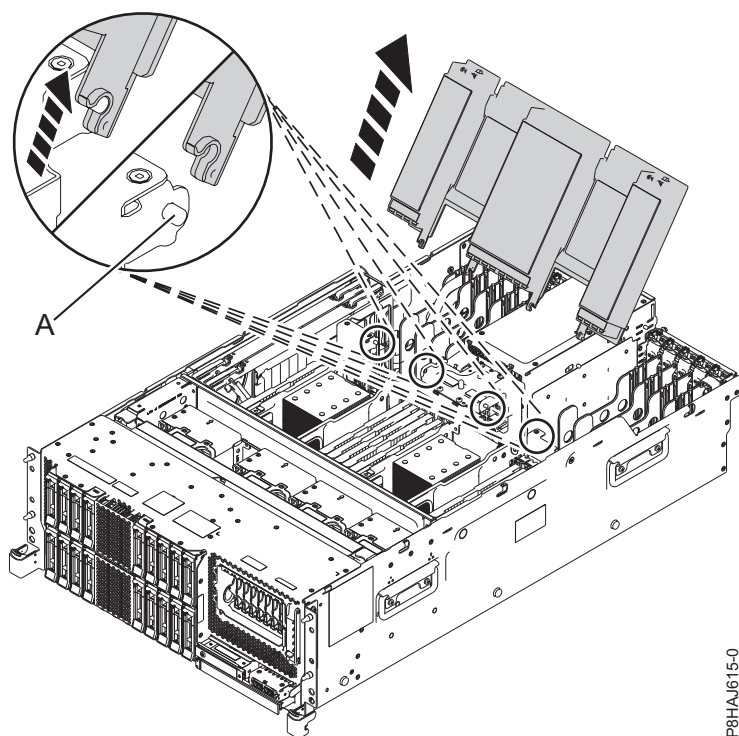
Figura 29. Extracció del deflector d'aire
