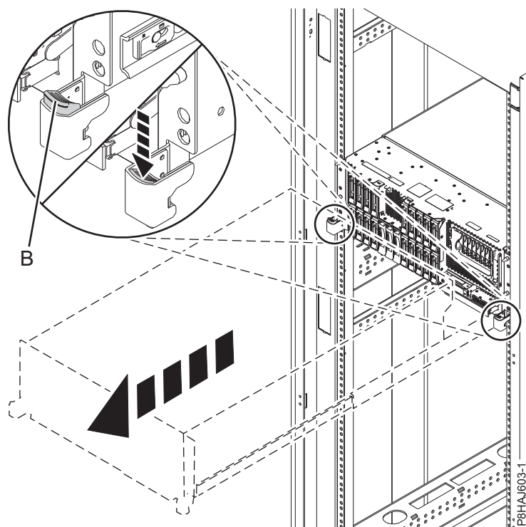
Figura 32. Alliberament dels pestells laterals
