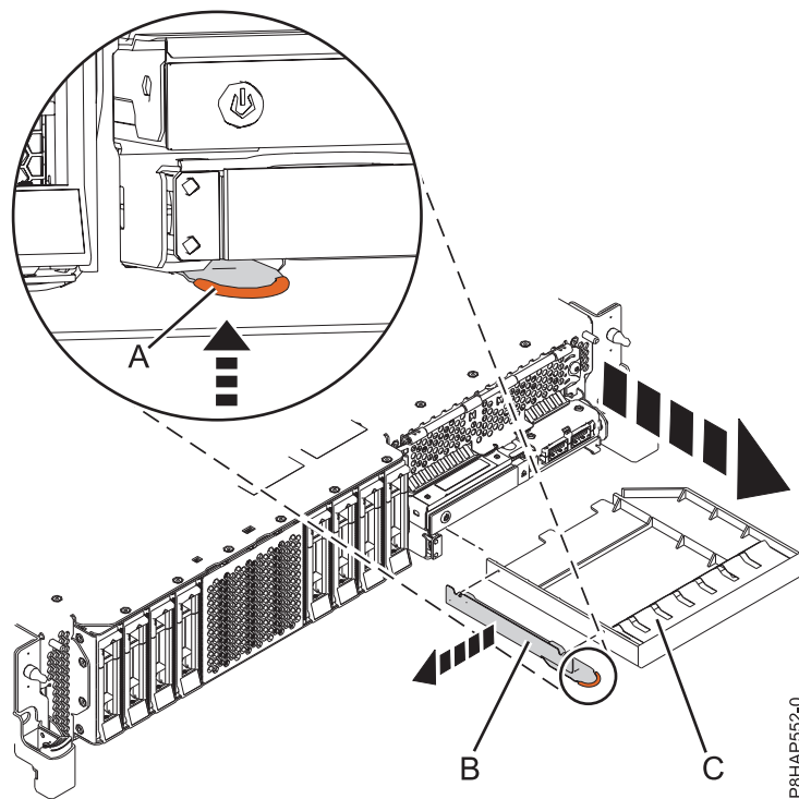
Figura 9. Extracció del sistema de la placa de rebliment del dispositiu de suport d'emmagatzematge i de la peça de subjecció
