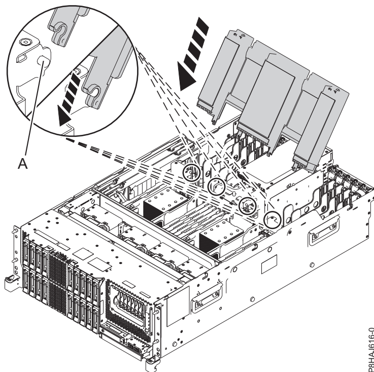
Figura 95. Substitució del deflector d'aire
