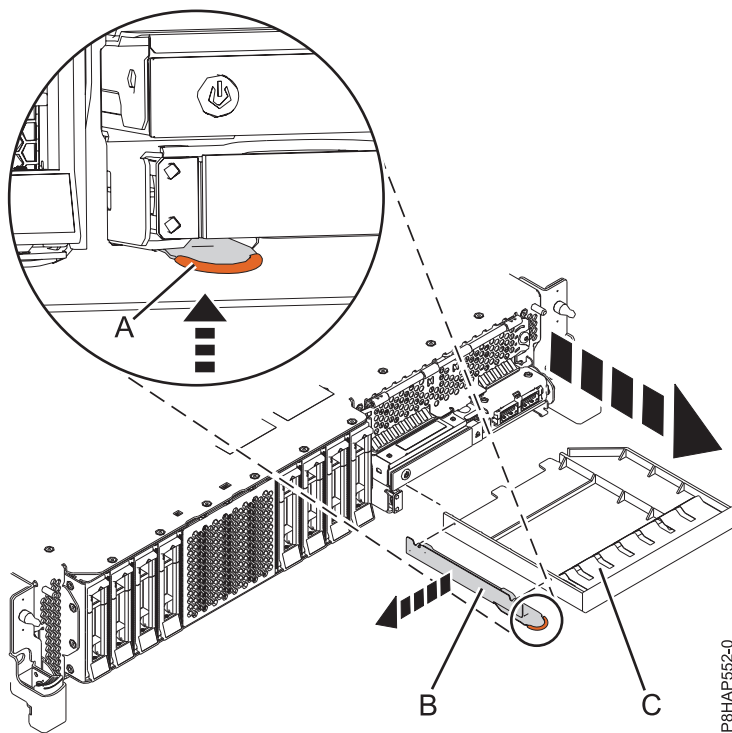
Figura 19. Extracció del sistema de la placa de reblliment del dispositiu de suport d'emmagatzematge i de la peça de subjecció
