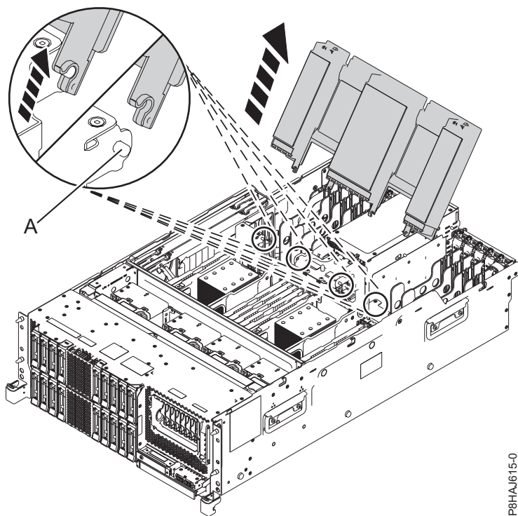
Figura 94. Extracció del deflector d'aire
