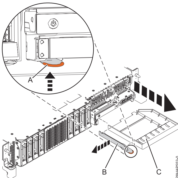
Figura 42. Extracció del sistema de la placa de reblliment del dispositiu de suport d'emmagatzematge i de la peça de subjecció
