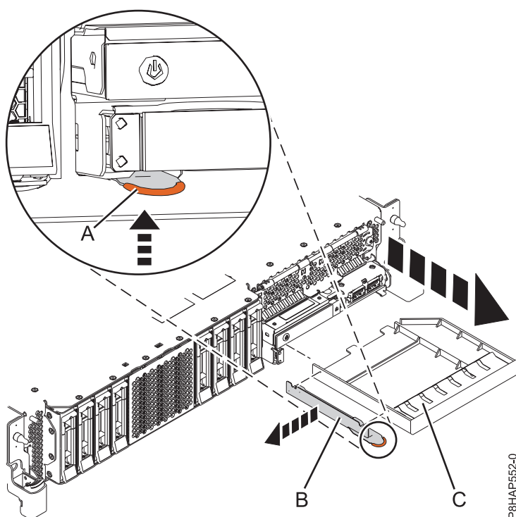
Figura 56. Extracció del sistema de la placa de reblliment del dispositiu de suport d'emmagatzematge i de la peça de subjecció
