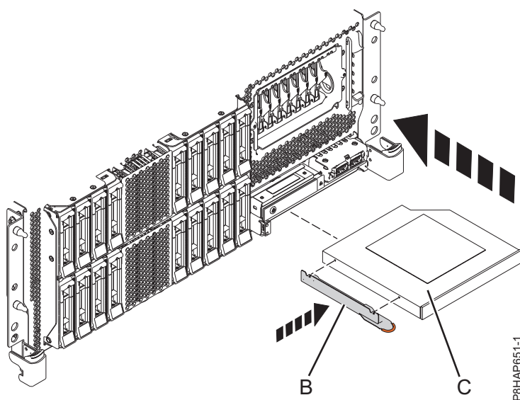
Figura 58. Substitució d'un dispositiu de suport d'emmagatzematge extraplà en un sistema 8247-42L, 8286-41A o 8286-42A muntat en bastidor
