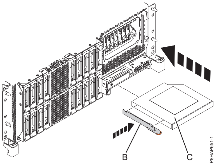
Figura 28. Substitució d'un dispositiu de suport d'emmagatzematge extraplà en un sistema 8247-42L, 8286-41A o 8286-42A muntat en bastidor
