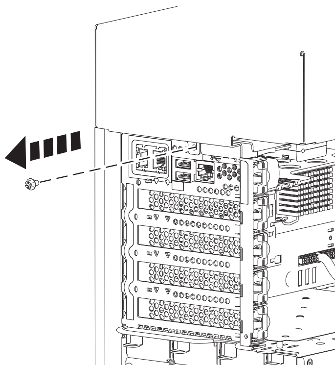
Figura 78. Extracció del cargol de la coberta lateral model 8286-41A
