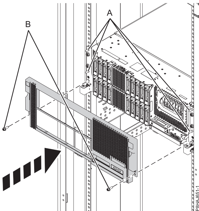
Figura 81. Instal·lació de la coberta frontal
