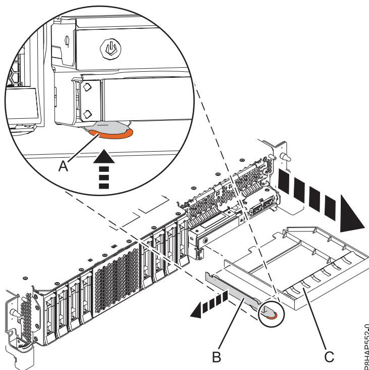
Figura 26. Extracció del sistema de la placa de reblliment del dispositiu de suport d'emmagatzematge i de la peça de subjecció
