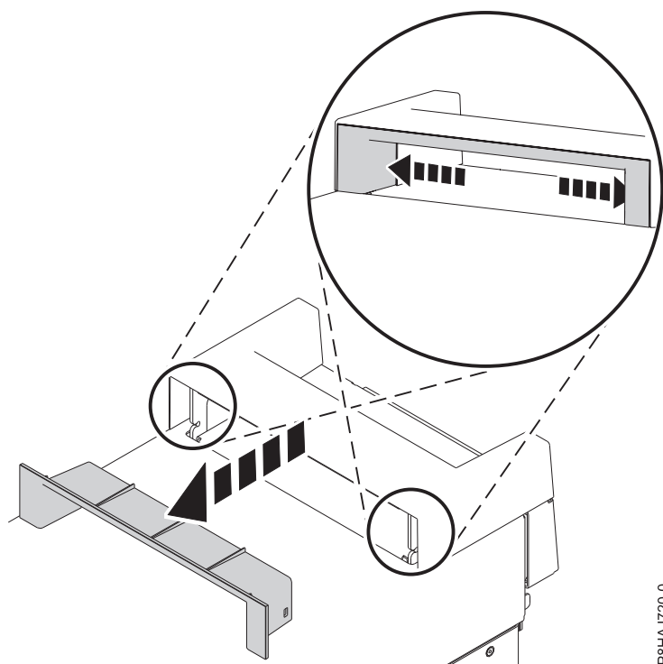
Figura 76. Extracció de la peça de la tapa de nansa d'un sistema autònom 8286-41A
