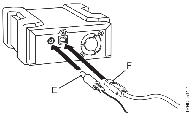
Figura 60. Connexió dels cables USB i d'alimentació
