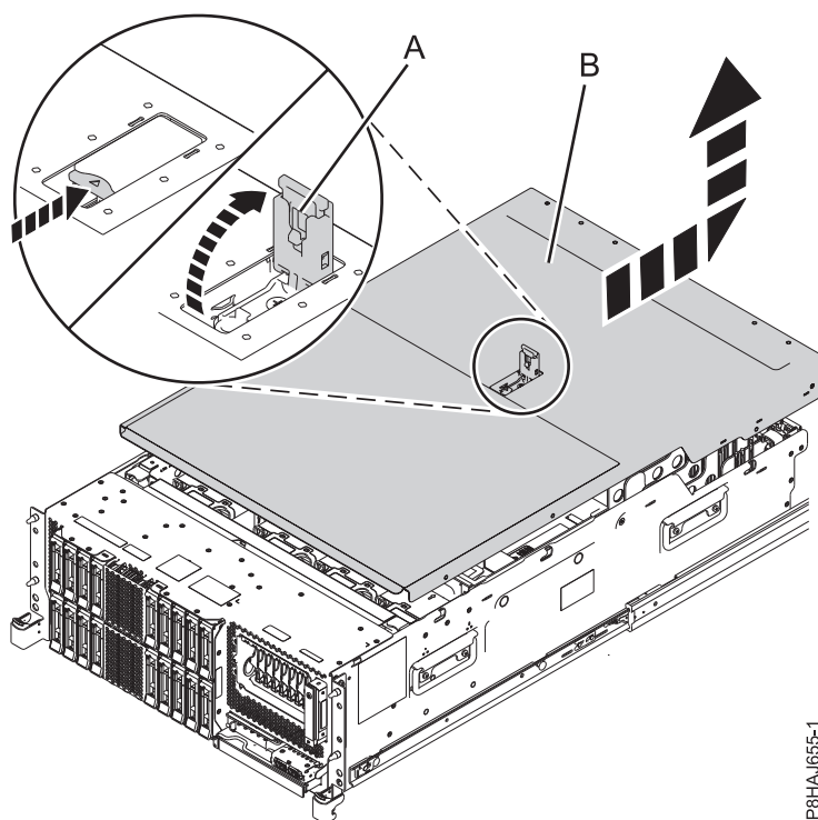
Figura 88. Extracció de la coberta d'accés de servei
