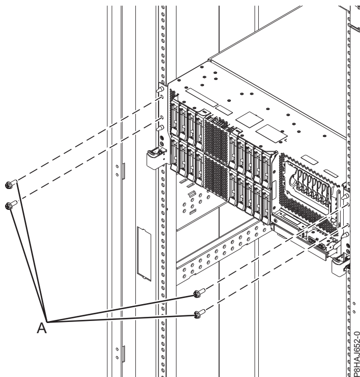
Figura 96. Extracció dels cargols frontals
