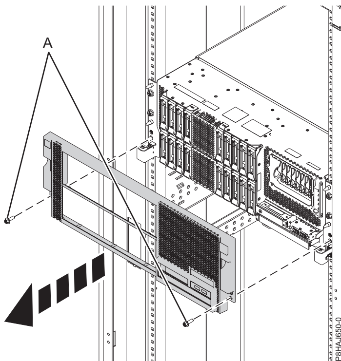
Figura 74. Extracció de la coberta frontal
