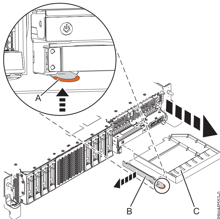
Figura 1. Extracció del sistema de reblliment del dispositiu de suport d'emmagatzematge i de la peça de subjectió
