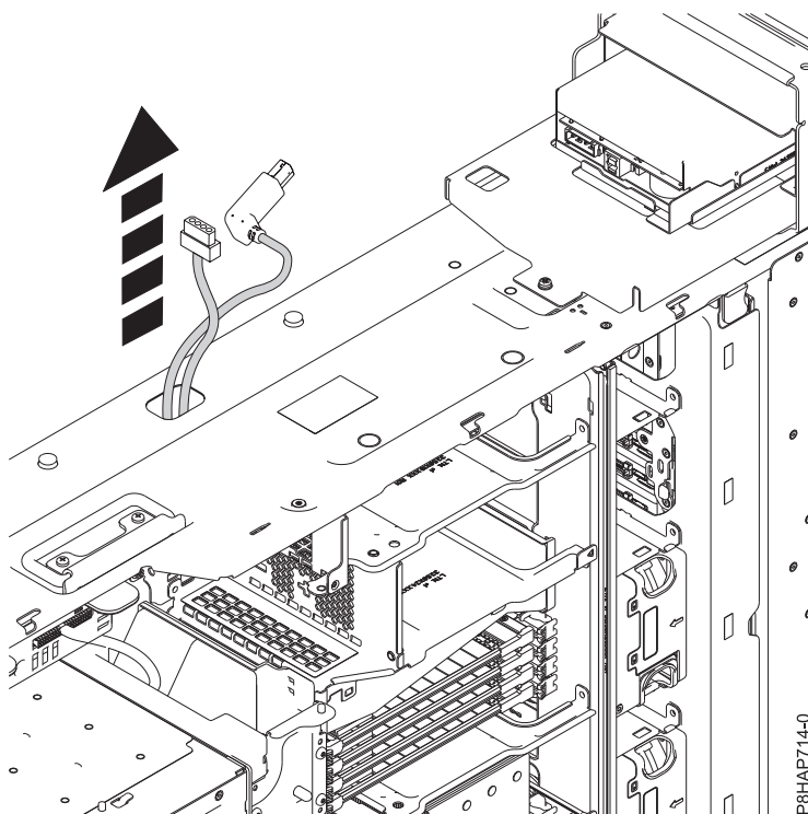
Figura 69. Com fer passar els cables USB i d'alimentació de l'estació d'acoblament RDX interna (FC EUA3)
