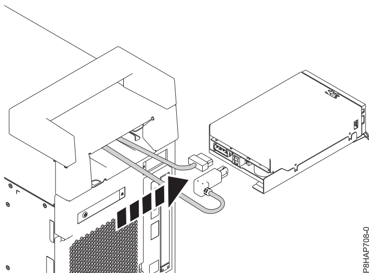
Figura 63. Connexió dels cables USB i d'alimentació de l'estació d'acoblament RDX interna (FC EUA3)
