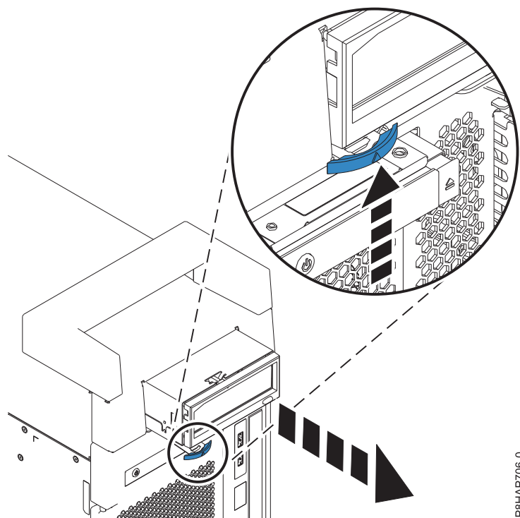
Figura 61. Extracció d'una estació d'acoblament RDX interna
