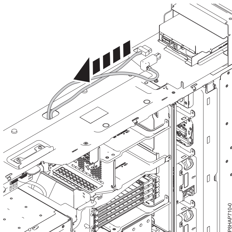
Figura 65. Desconnexió dels cables USB i d'alimentació de l'estació d'acoblament RDX interna (FC EUA3)
