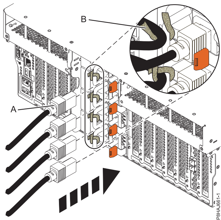
Figura 108. Connexió dels cables d'alimentació a un sistema 8247-42L, 8286-41A o 8286-42A
