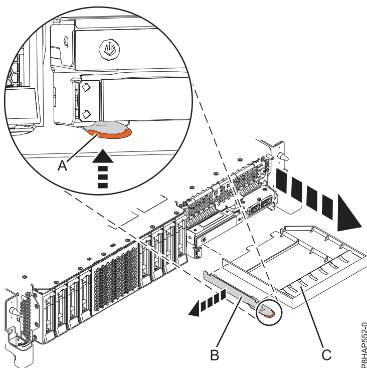
Figura 49. Extracció del sistema de la placa de reblliment del dispositiu de suport d'emmagatzematge i de la peça de subjecció
