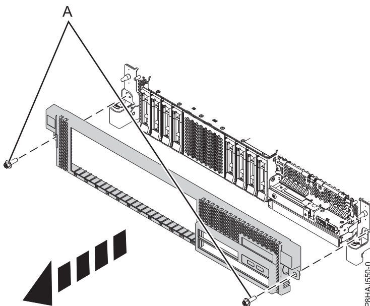
Figura 73. Extracció de la coberta frontal
