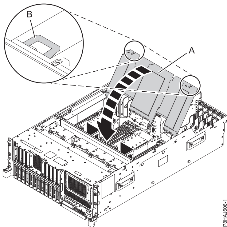
Figura 93. Tancament del deflector d'aire
