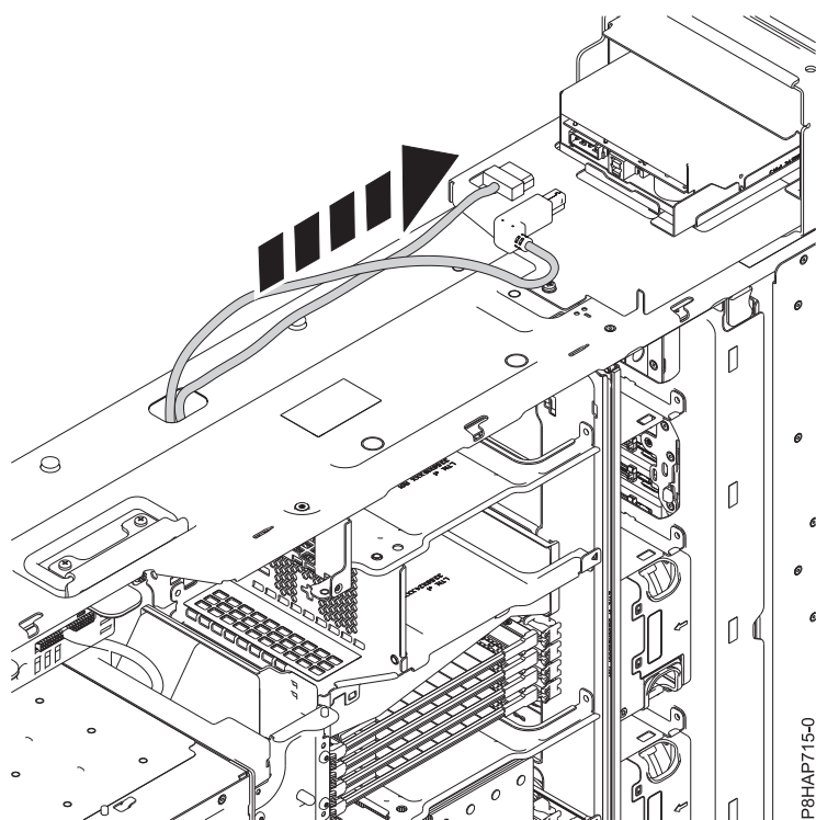
Figura 70. Connexió dels cables USB i d'alimentació a la part posterior de l'estació d'acoblament RDX interna (FC EUA3)
