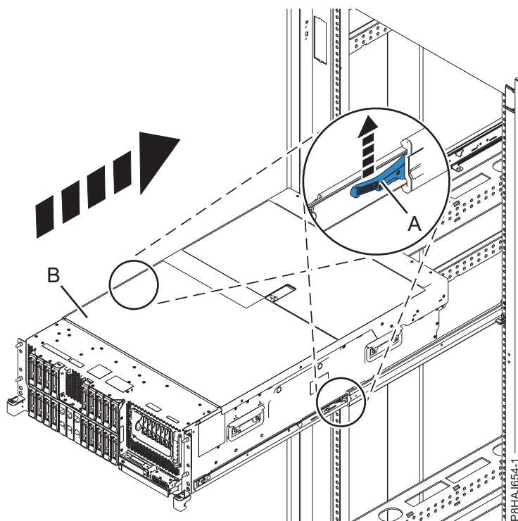
Figura 98. Col·locació del sistema en posició operativa
