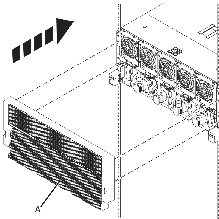
Figura 16. Instal·lació de la coberta frontal
