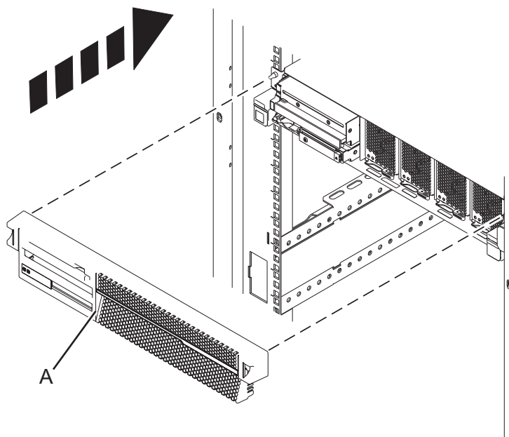
Figura 17. Instal·lació de la coberta frontal de la unitat de control del sistema
