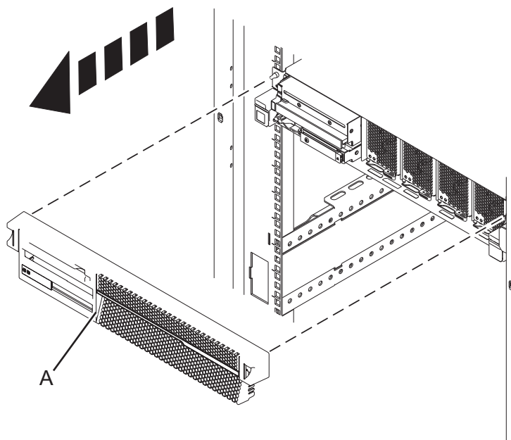
Figura 15. Extracció de la coberta frontal de la unitat de control del sistema
