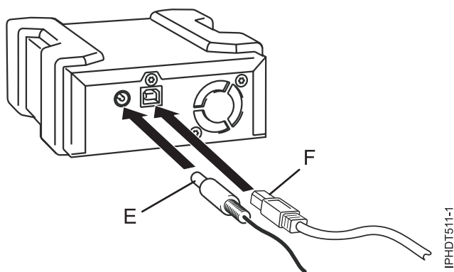
Figura 11. Connexió dels cables USB i d'alimentació
