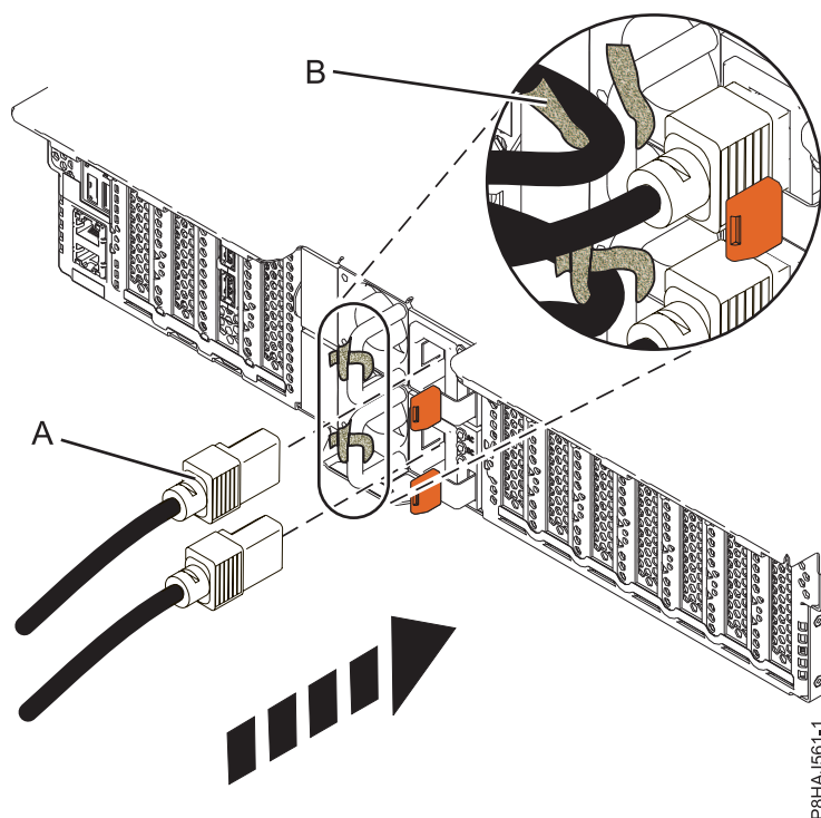
Figura 36. Connexió dels cables d'alimentació a un sistema 5148-21L, 5148-22L, 8247-21L, 8247-22L, 8284-21A, o 8284-22A
