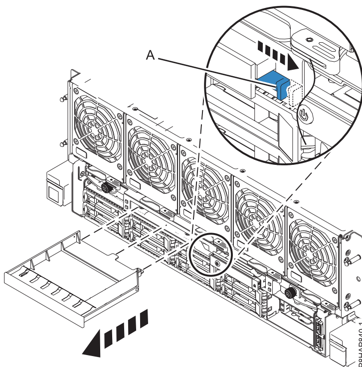
Figura 1. Extracció del sistema del panell de reblliment del dispositiu de suport d'emmagatzematge.
