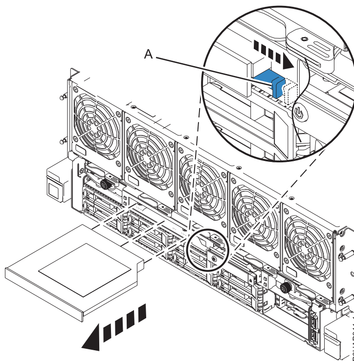
Figura 11. Extracció de la unitat de DVD del sistema
