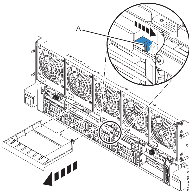
Figura 5. Extracció del sistema del panell de reblliment del dispositiu de suport d'emmagatzematge.
