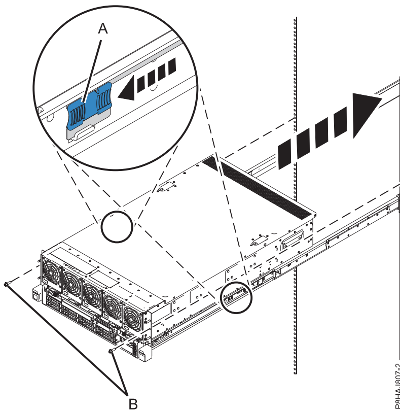
Figura 25. Col·locació del sistema en posició operativa
