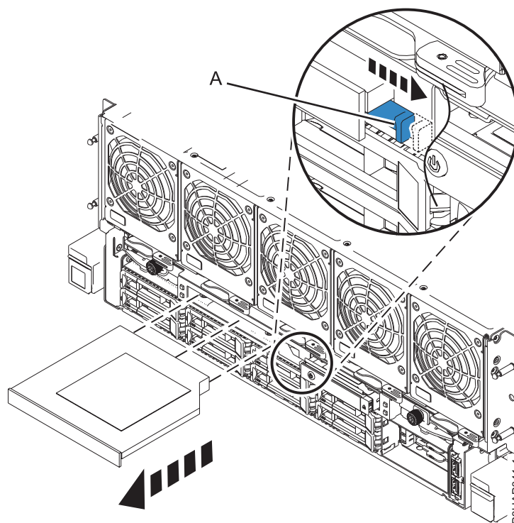
Figura 7. Extracció de la unitat de DVD del sistema
