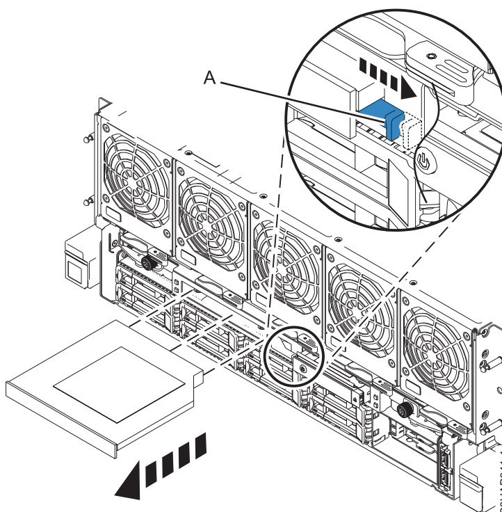
Figura 9. Extracció de la unitat de DVD del sistema
