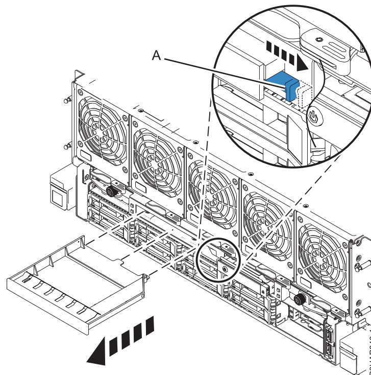
Figura 3. Extracció del sistema del panell de reblliment del dispositiu de suport d'emmagatzematge.
