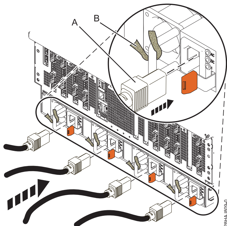
Figura 37. Connexió dels cables d'alimentació a un sistema 8408-44E o 8408-E8E
