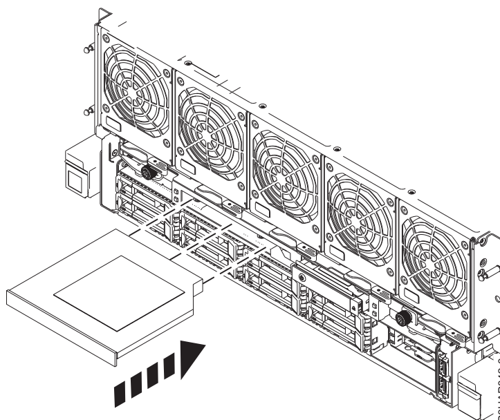
Figura 12. Instal·lació de la unitat de DVD al sistema
