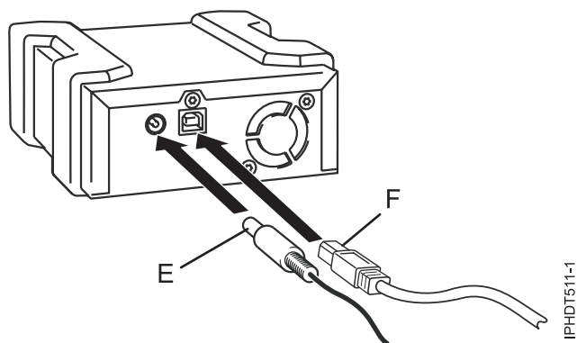
Figura 13. Connexió dels cables USB i d'alimentació
