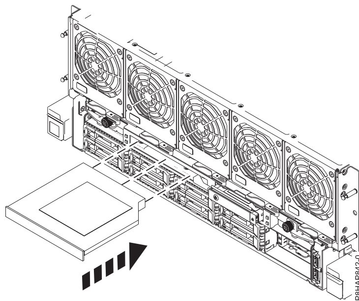
Figura 2. Instal·lació de la unitat de DVD al sistema
