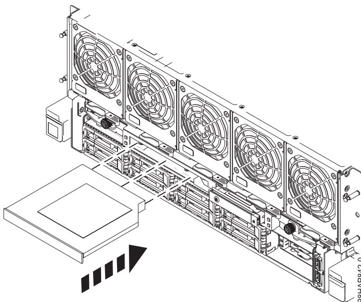
Figura 4. Instal·lació de la unitat de DVD al sistema
