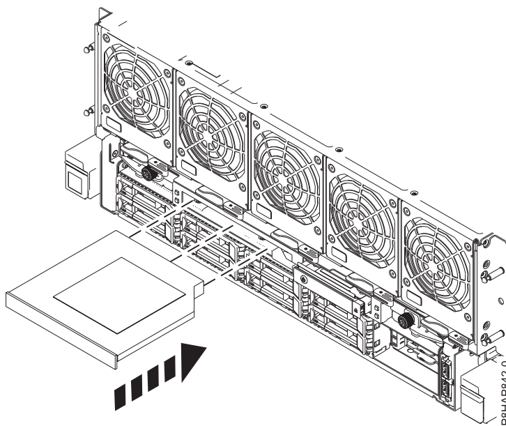
Figura 8. Instal·lació de la unitat de DVD al sistema
