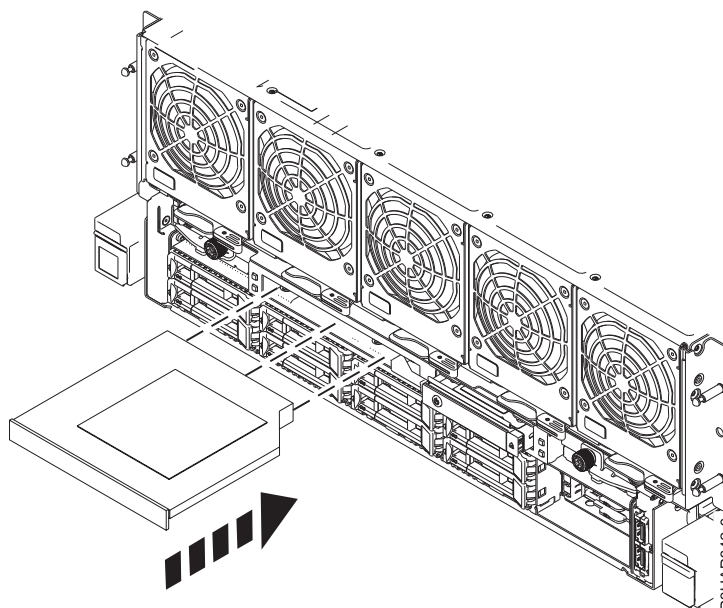
Figura 6. Instal·lació de la unitat de DVD al sistema
