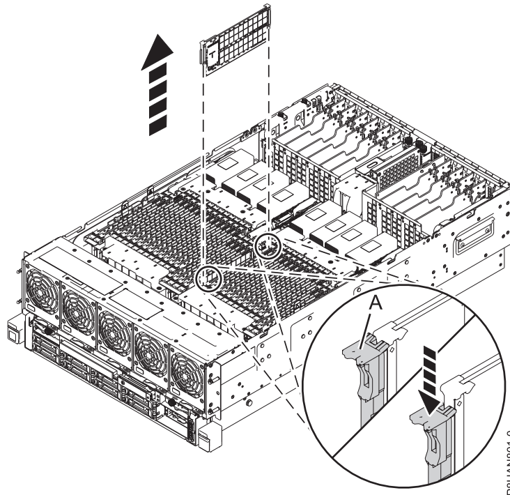
Figura 10. Extracció d'una targeta de memòria del sistema.
