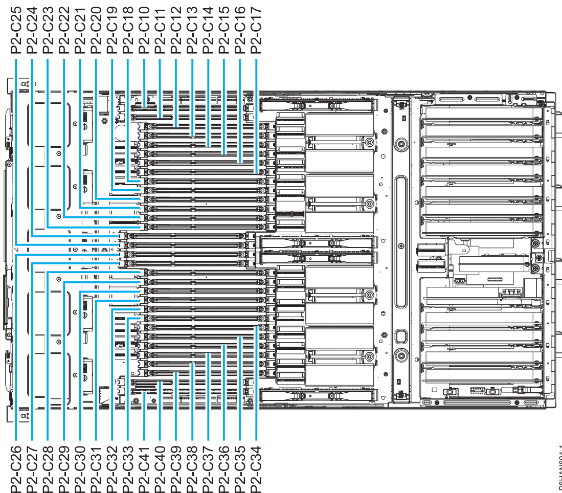
Figura 12. Ubicacions de memòria al sistema 8408-44E o 8408-E8E
