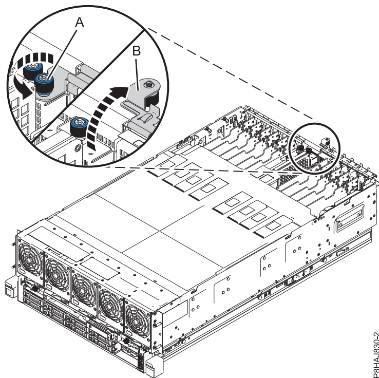
Figura 33. Obertura del pestell d'E/S
