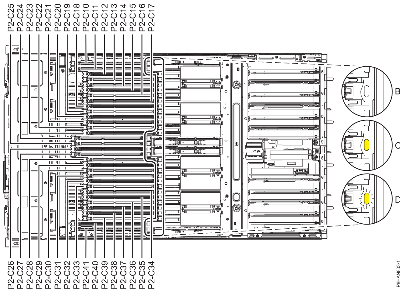
Figura 9. Ubicació de les ranures de memòria i dels LED
