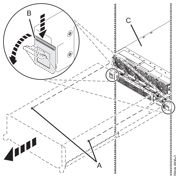
Figura 35. Col·locació del sistema en posició de servei
