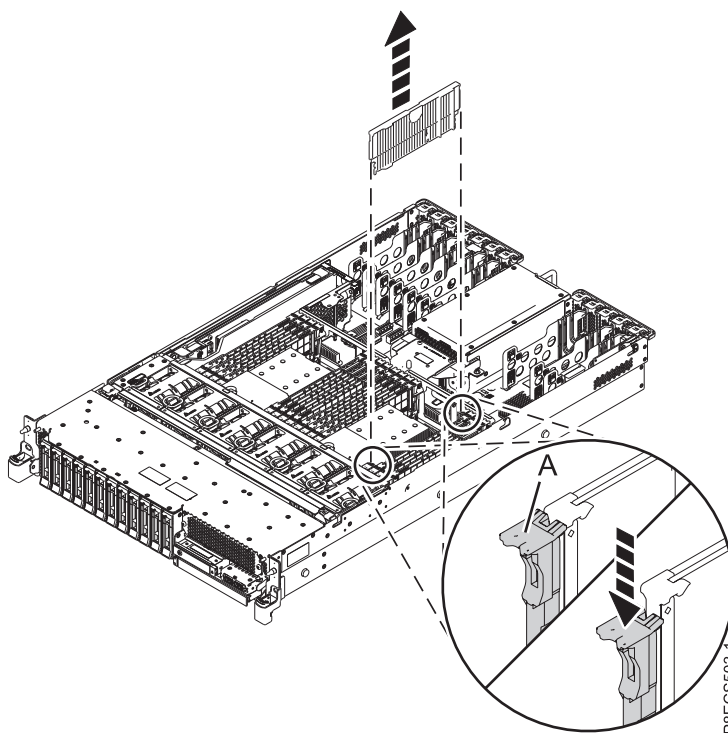
Figura 7. Extracció del panell de rebliment d'un mòdul de memòria de la ranura del mòdul de memòria en un sistema 5148-21L, 5148-22L, 8247-21L, 8247-22L, 8284-21A, o 8284-22A
