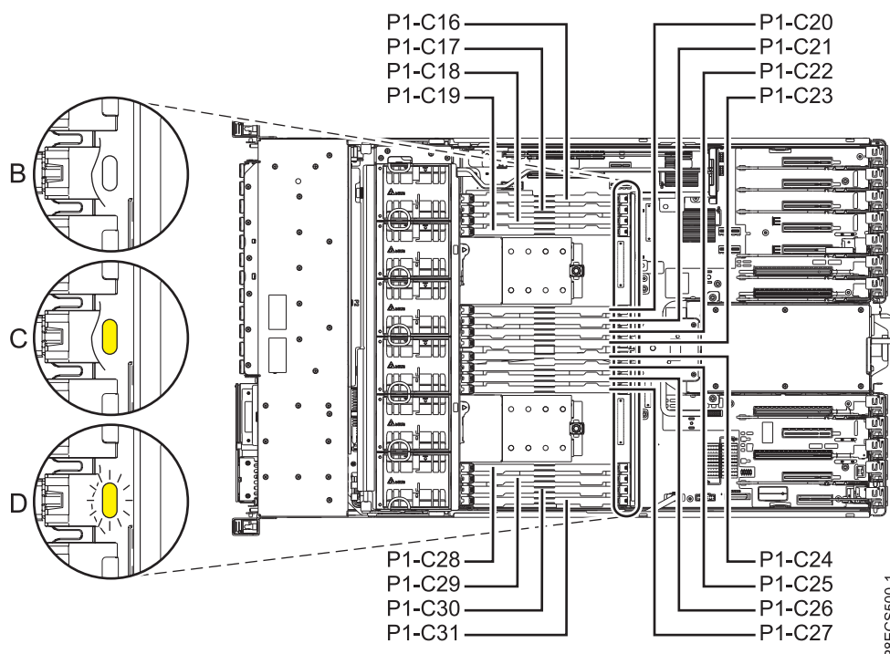
Figura 1. Ubicacions dels mòduls de memòria i dels indicadors de servei del sistema 5148-21L, 5148-22L, 8247-21L, 8247-22L, 8284-21A, o 8284-22A
