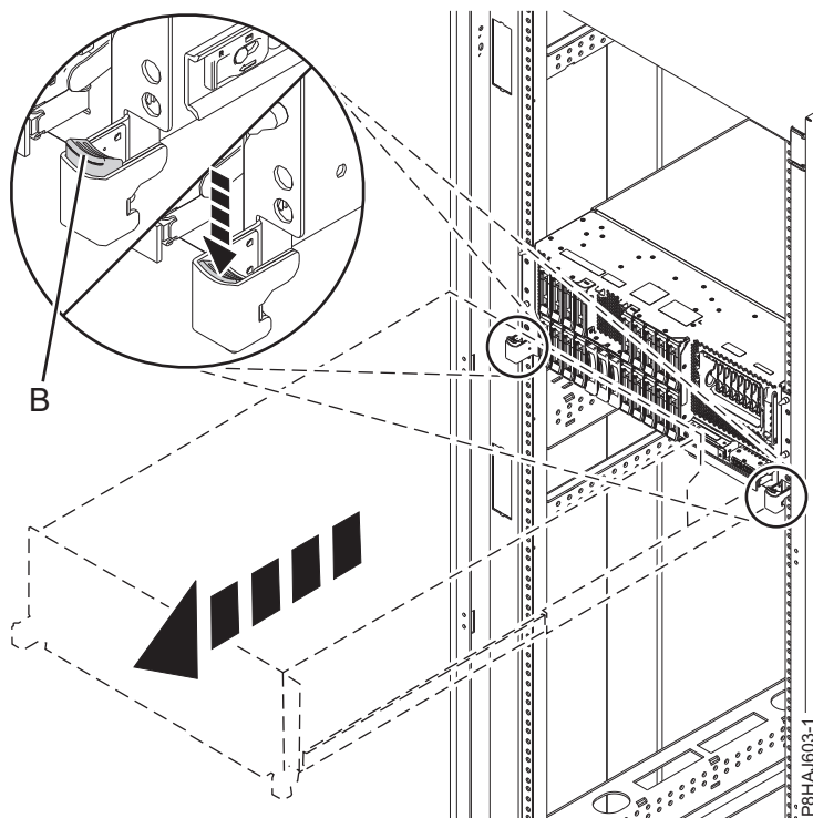
Figura 49. Alliberament dels pestells laterals
