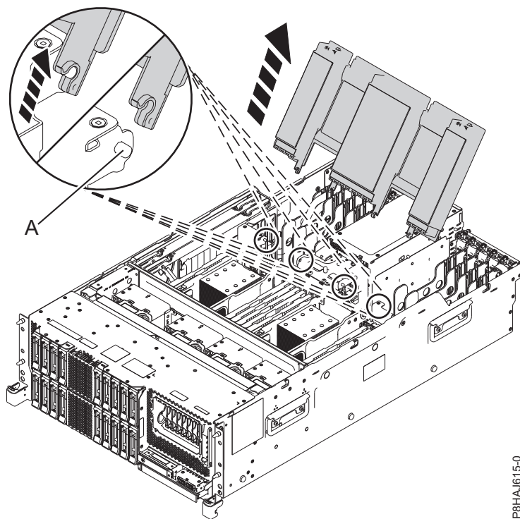
Figura 46. Extracció del deflector d'aire
