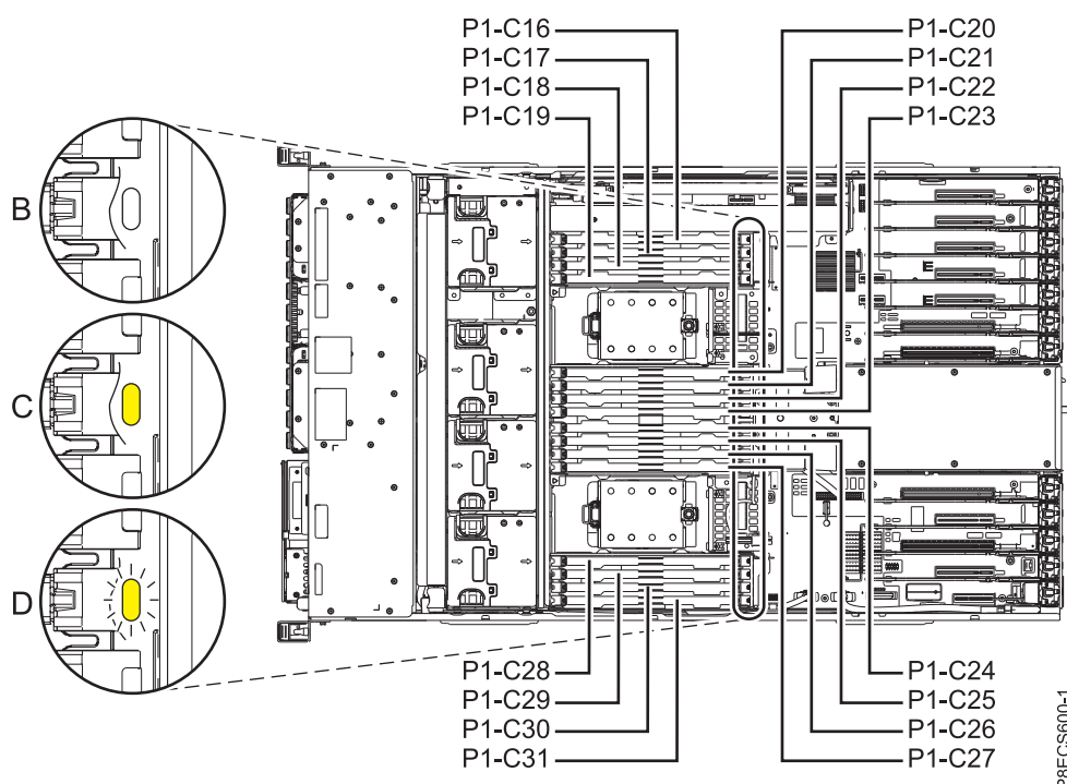
Figura 1. Ubicacions dels mòduls de memòria i dels indicadors de servei del sistema 8247-42L, 8286-41A o 8286-42A
