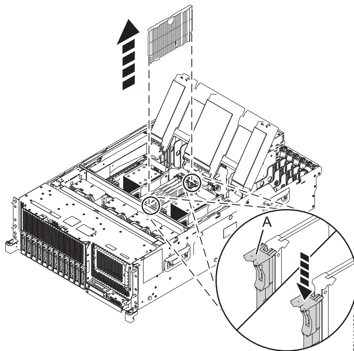
Figura 7. Extracció del panell de rebliment d'un mòdul de memòria de la ranura del mòdul de memòria en un sistema 8247-42L, 8286-41A o 8286-42A
