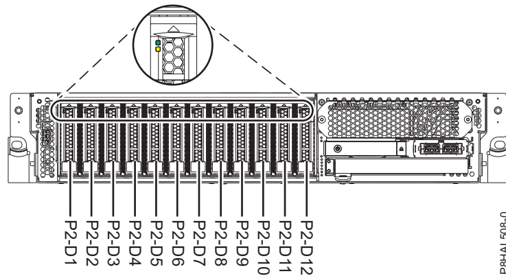
Figura 58. Ubicacions de la unitat de disc i dels indicadors de servei per a un sistema funció bàsica
