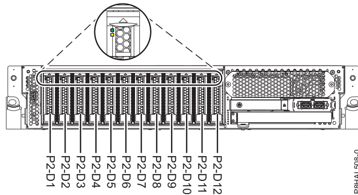
Figura 48. Ubicacions de la unitat de disc i dels indicadors de servei per a un sistema funció bàsica
