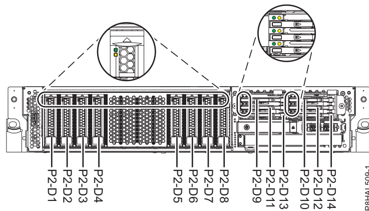
Figura 49. Ubicacions de la unitat de disc, de la unitat d'estat sòlid i dels indicadors de servei per a un sistema de funció expandida
