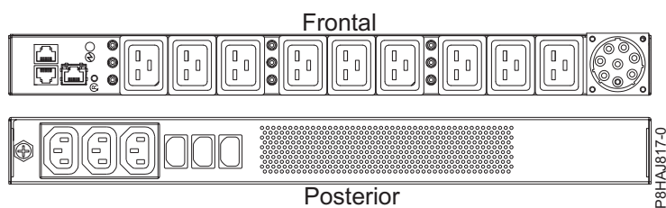
Figura 125. PDU per al sistema 8408-44E
