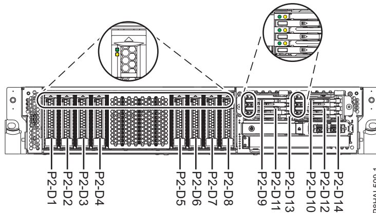
Figura 29. Ubicacions de la unitat de disc, de la unitat d'estat sòlid i dels indicadors de servei per a un sistema de funció estesa
