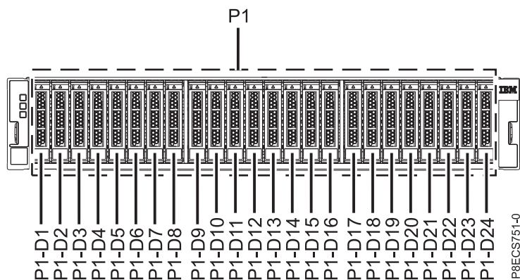
Figura 110. Vista frontal de l'allotjament d'emmagatzematge ESLS que mostra les ubicacions de les unitats de disc
