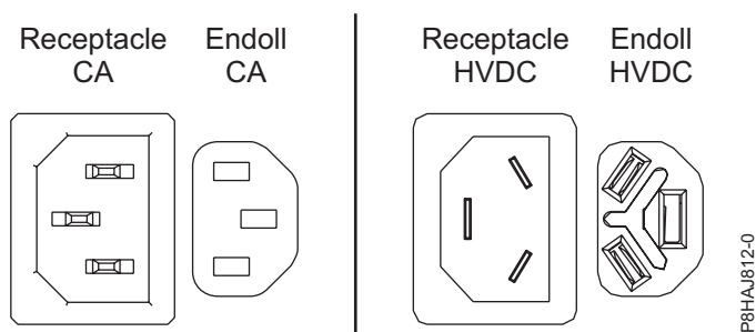
Figura 123. Connectors de CA i d'HVDC
