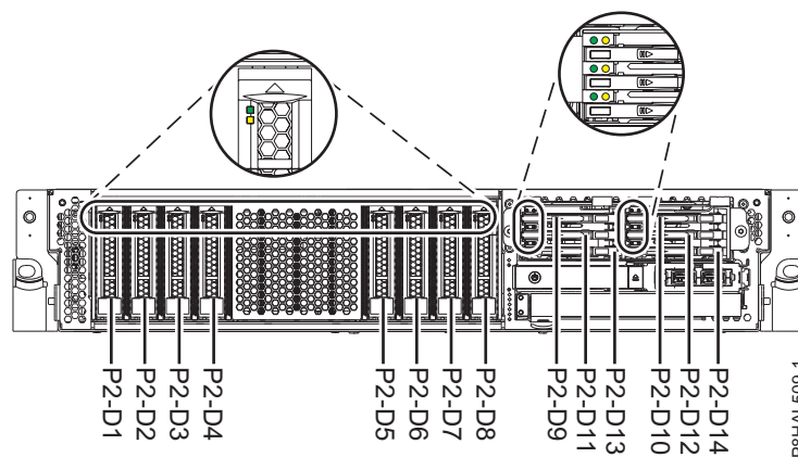
Figura 105. Ubicacions de les unitats de disc, unitats d'estat sòlid i indicadors de servei en un sistema 5148-21L, 5148-22L, 8247-21L, 8247-22L, 8284-21A, o 8284-22A de funció expandida
