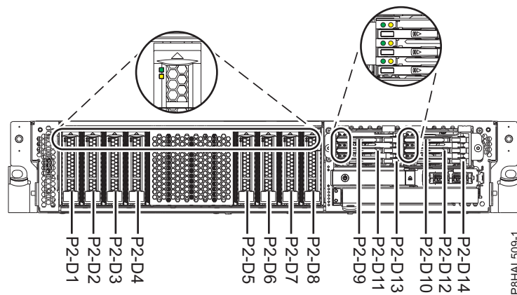
Figura 59. Ubicacions de la unitat de disc, de la unitat d'estat sòlid i dels indicadors de servei per a un sistema de funció expandida
