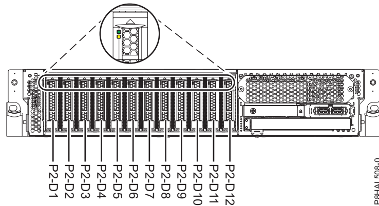
Figura 82. Ubicacions de la unitat de disc i dels indicadors de servei per a un sistema funció bàsica
