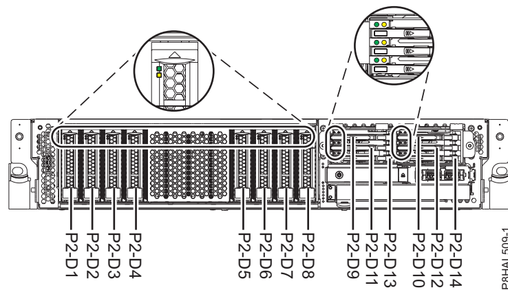
Figura 83. Ubicacions de la unitat de disc, de la unitat d'estat sòlid i dels indicadors de servei per a un sistema de funció expandida
