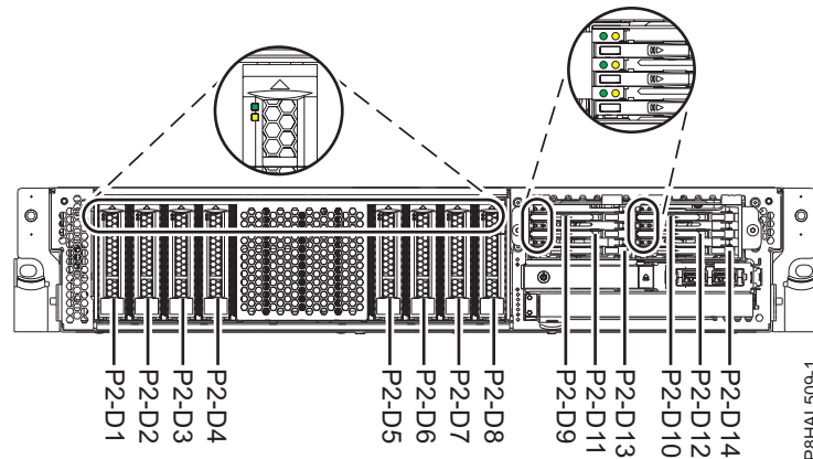
Figura 39. Ubicacions de la unitat de disc, de la unitat d'estat sòlid i dels indicadors de servei per a un sistema de funció estesa
