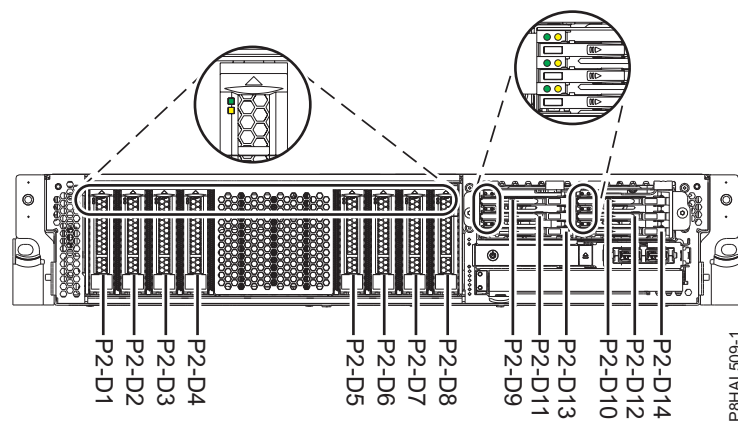
Figura 11. Ubicacions de la unitat de disc, de la unitat d'estat sòlid i dels indicadors de servei per a un sistema de funció estesa
