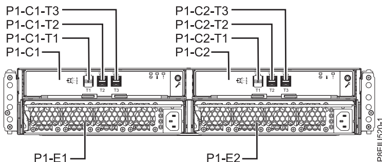
Figura 111. Vista posterior de l'allotjament
