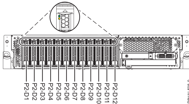
Figura 104. Ubicacions de les unitats de disc i dels indicadors de servei en un sistema 5148-21L, 5148-22L, 8247-21L, 8247-22L, 8284-21A, o 8284-22A de funció bàsica
