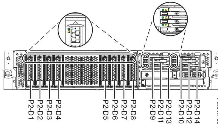
Figura 6. Ubicacions de la unitat de disc, de la unitat d'estat sòlid i dels indicadors de servei per a un sistema de funció expandida
