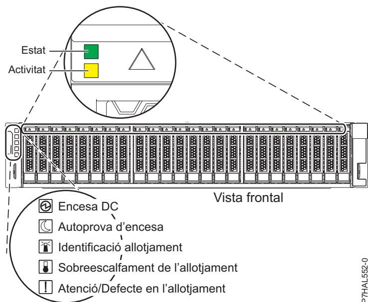
Figura 108. Vista frontal de l'allotjament d'unitats de disc 5887 que mostra els indicadors de servei
