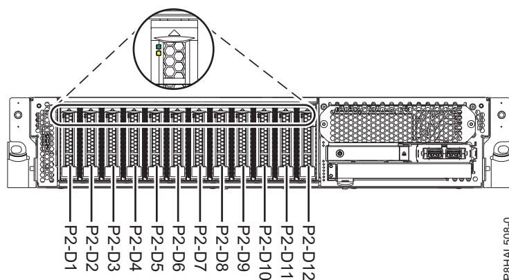
Figura 70. Ubicacions de la unitat de disc i dels indicadors de servei per a un sistema funció bàsica
