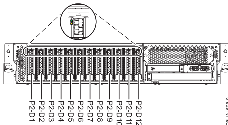
Figura 38. Ubicacions de la unitat de disc i dels indicadors de servei per a un sistema funció bàsica
