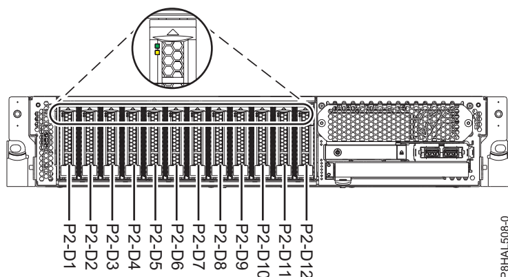
Figura 1. Ubicacions de la unitat de disc i dels indicadors de servei per a un sistema funció bàsica
