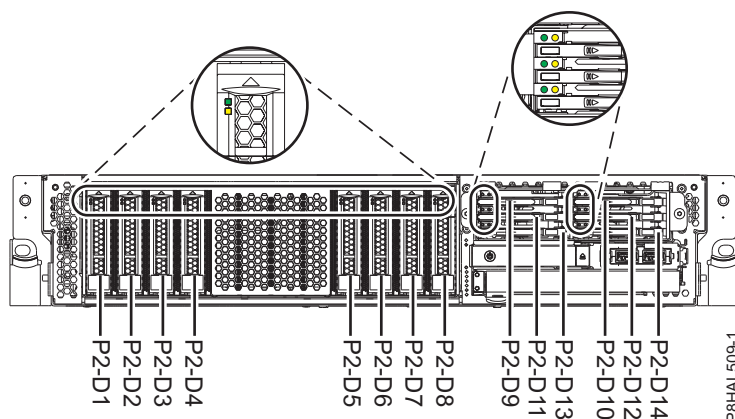
Figura 71. Ubicacions de la unitat de disc, de la unitat d'estat sòlid i dels indicadors de servei per a un sistema de funció expandida
