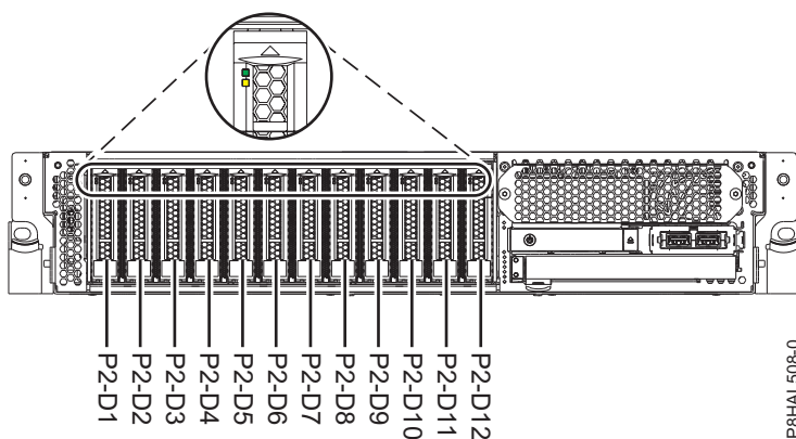
Figura 10. Ubicacions de la unitat de disc i dels indicadors de servei per a un sistema funció bàsica
