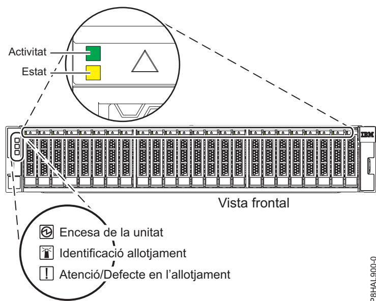
Figura 112. Vista frontal de l'allotjament que mostra els indicadors de servei
