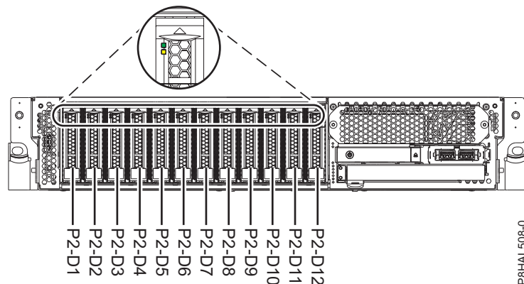
Figura 18. Ubicacions de la unitat de disc i dels indicadors de servei per a un sistema funció bàsica
