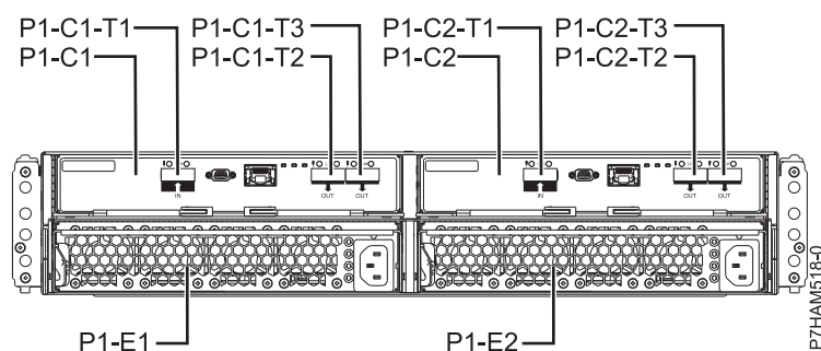
Figura 107. Vista posterior de l'allotjament d'unitats de disc 5887
