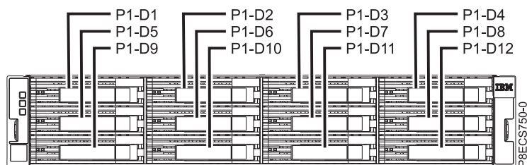
Figura 109. Vista frontal de l'allotjament d'emmagatzematge ESLL que mostra les ubicacions de les unitats de disc
