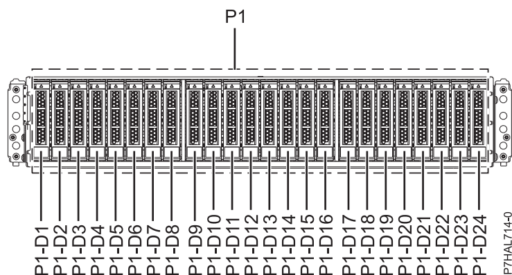
Figura 106. Vista frontal del model allotjament d'unitats de disc 5887 que mostra les ubicacions de les unitats de disc
