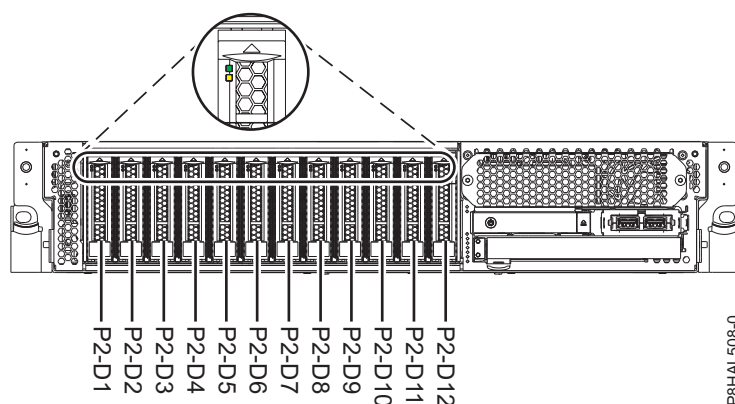
Figura 28. Ubicacions de la unitat de disc i dels indicadors de servei per a un sistema funció bàsica
