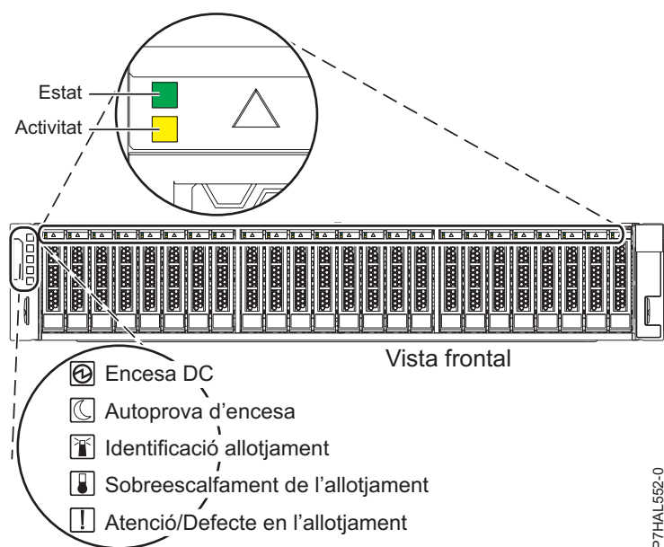
Figura 28. Vista frontal de l'allotjament d'unitats de disc 5887 que mostra els indicadors de servei
