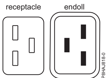
Figura 78. Connectors per al sistema 8408-44E
