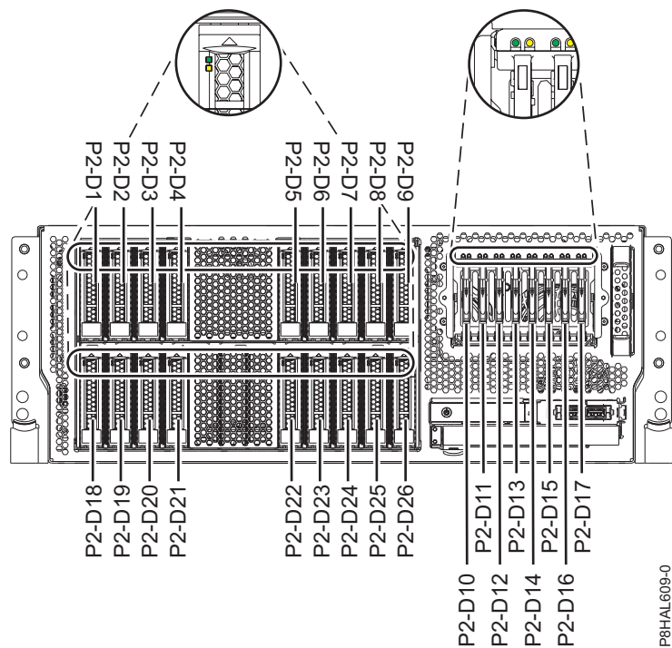
Figura 60. Ubicacions d'unitat de disc, unitat d'estat sòlid i indicadors de servei en un sistema de funció expandida 8286-41A o 8286-42A muntat en bastidor
