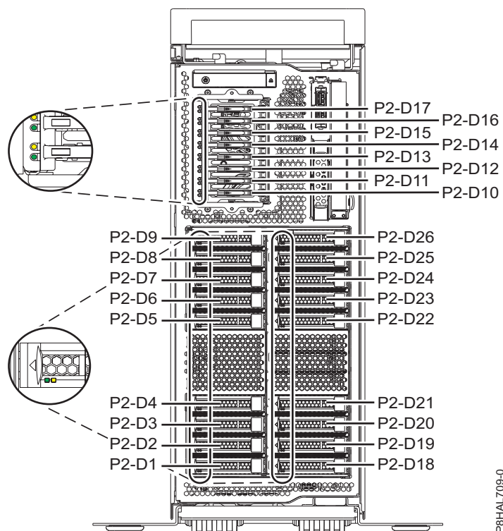
Figura 62. Ubicacions d'unitat de disc, unitat d'estat sòlid i indicador de servei en un sistema de funció expandida 8286-41A autònom
