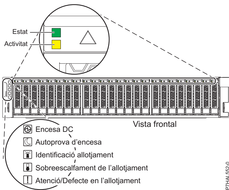
Figura 7. Vista frontal de l'allotjament d'unitats de disc 5887 que mostra els indicadors de servei
