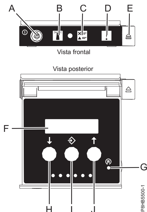
Figura 70. Tauler de control
