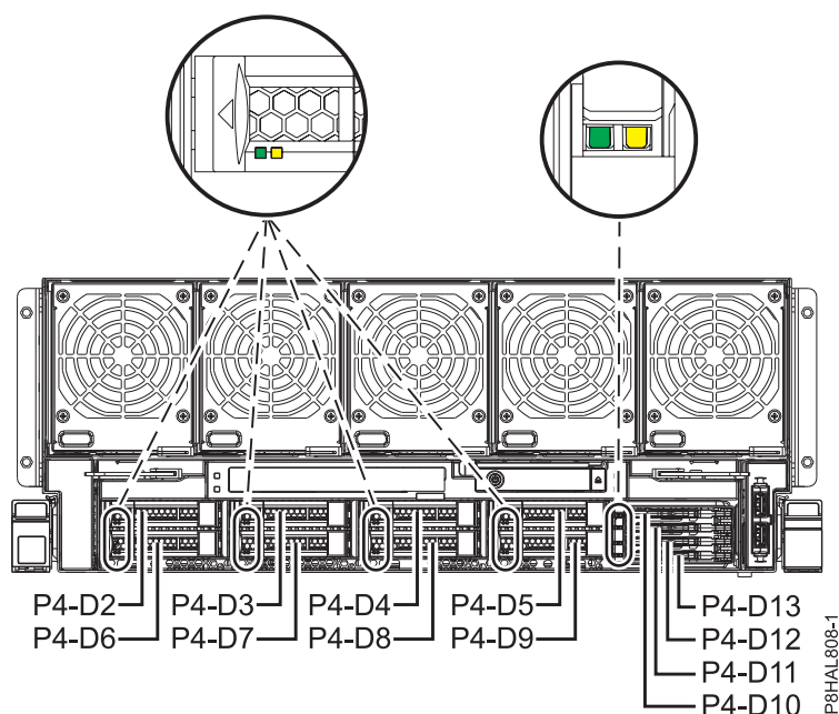
Figura 63. Ubicacions de les unitats de disc i les SSD i indicadors de servei per a un sistema 8408-44E o 8408-E8E
