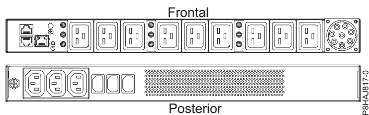
Figura 79. PDU per al sistema 8408-44E
