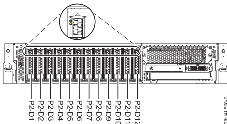
Figura 57. Ubicacions de les unitats de disc i dels indicadors de servei en un sistema 5148-21L, 5148-22L, 8247-21L, 8247-22L, 8284-21A, o 8284-22A de funció bàsica
