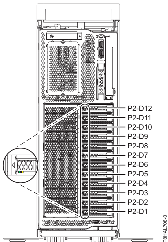
Figura 61. Ubicacions d'unitat de disc, unitat d'estat sòlid i indicador de servei en un sistema de funció bàsica 8286-41A autònom
