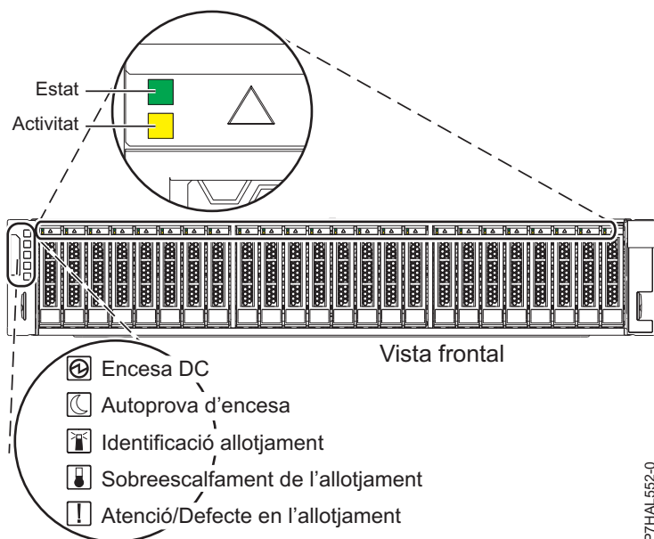
Figura 11. Vista frontal de l'allotjament d'unitats de disc 5887 que mostra els indicadors de servei
