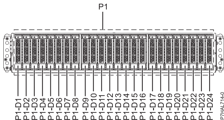
Figura 64. Vista frontal del model allotjament d'unitats de disc 5887 que mostra les ubicacions de les unitats de disc
