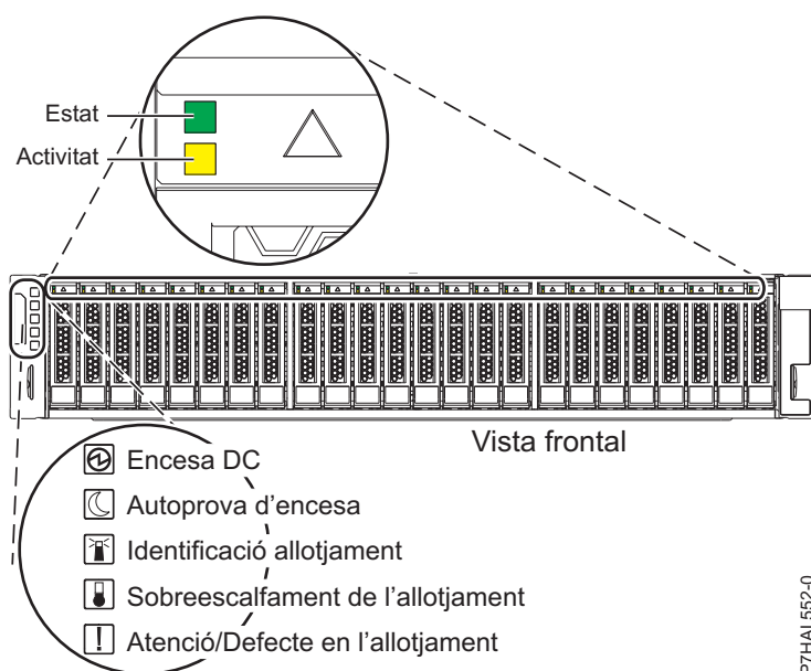
Figura 66. Vista frontal de l'al·lotjament d'unitats de disc 5887 que mostra els indicadors de servei
