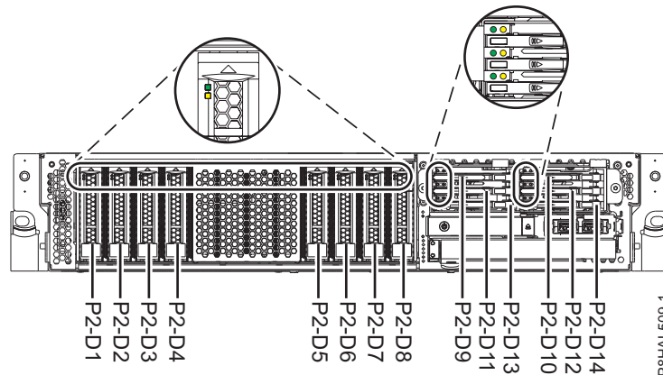
Figura 58. Ubicacions de les unitats de disc, unitats d'estat sòlid i indicadors de servei en un sistema 5148-21L, 5148-22L, 8247-21L, 8247-22L, 8284-21A, o 8284-22A de funció expandida
