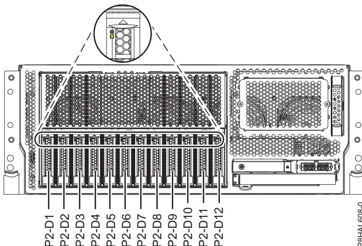
Figura 59. Ubicacions d'unitat de disc, unitat d'estat sòlid i indicadors de servei en un sistema de funció bàsica 8247-42L, 8286-41A o 8286-42A muntat en bastidor
