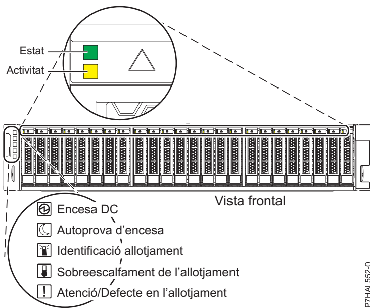
Figura 47. Vista frontal de l'allotjament d'unitats de disc 5887 que mostra els indicadors de servei
