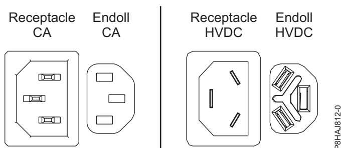
Figura 77. Connectors de CA i d'HVDC
