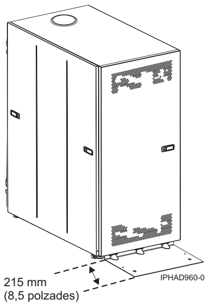
Figura 25. Model 0555 i 7014-S25 amb peu estabilitzador
