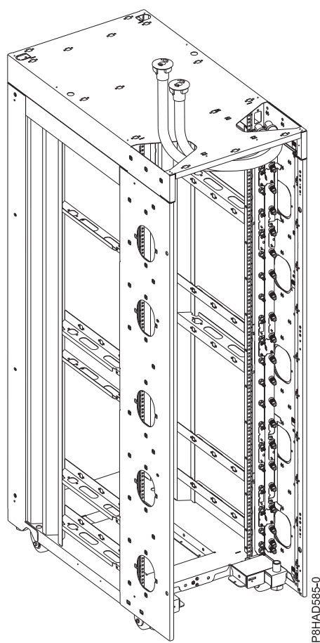
Figura 58. Bastidor i col·lector amb tubs de subministrament i retorn existent a la part superior del bastidor
