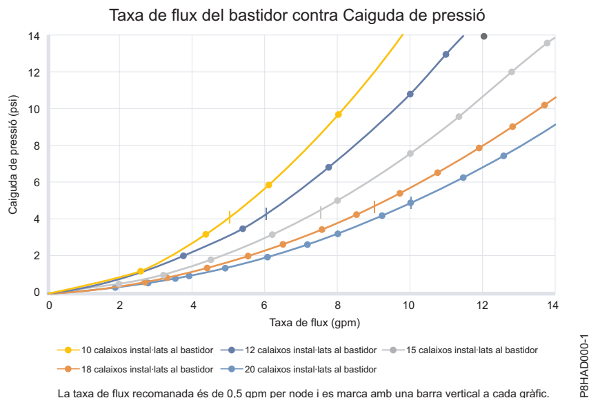
Figura 4. Taxa de flux contra caiguda de pressió (unitats mètriques)
