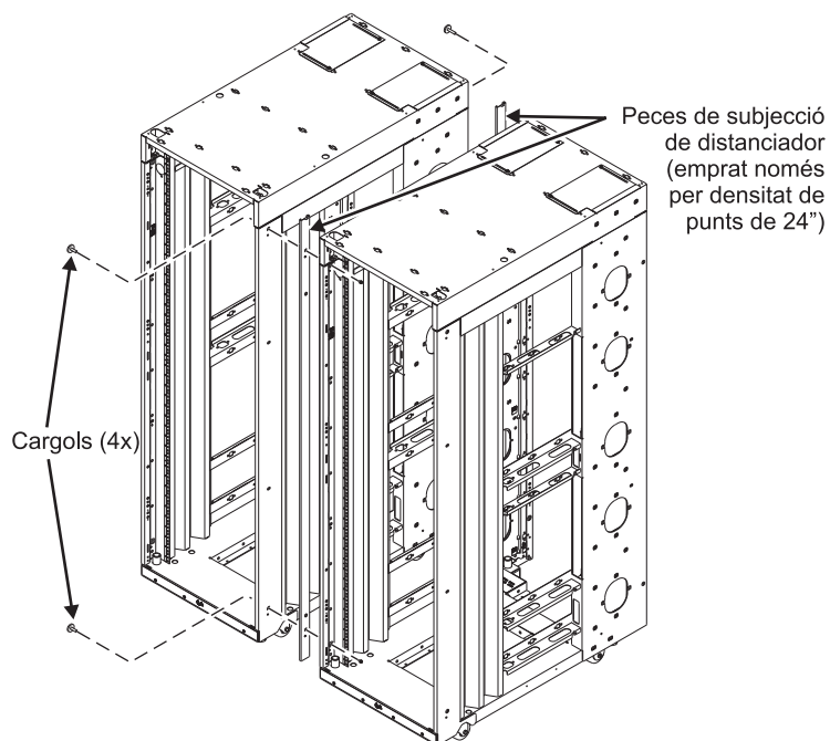
Figura 54. Connexió de diversos bastidors
