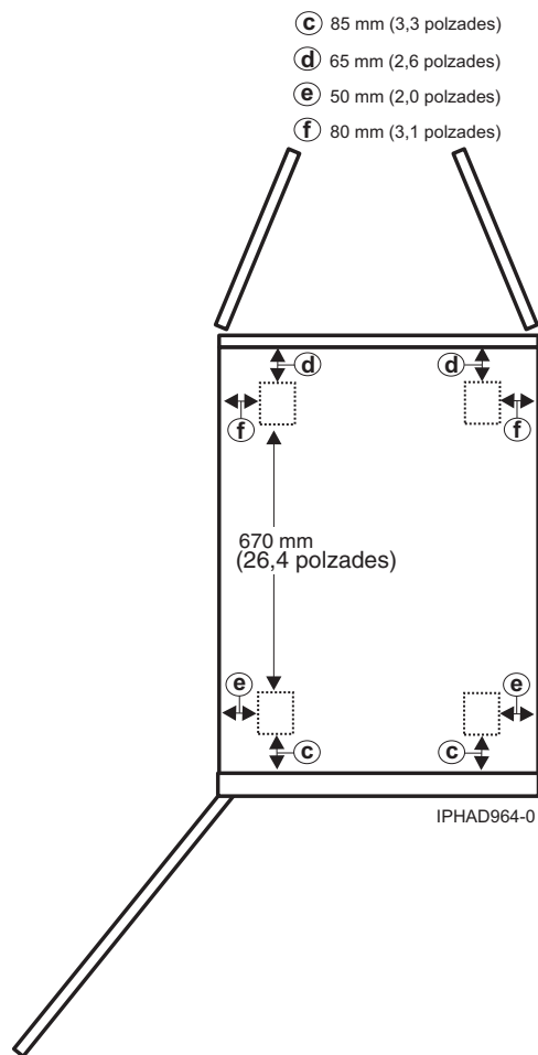
Figura 27. Ubicacions de les rodes giratòries del model 0555 i 7014-S25
