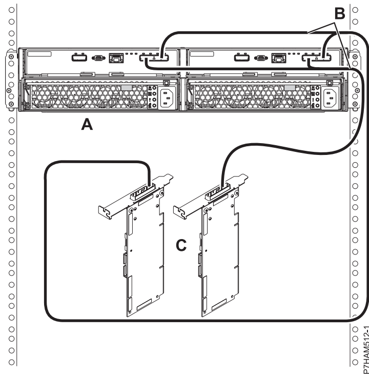
Figura 102. Connexió de mode 1 d'un allotjament 5887 utilitzant cables YO a adaptadors SAS duals
