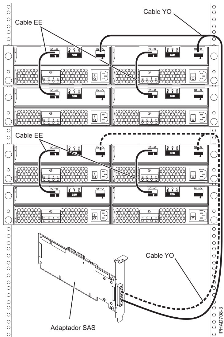
Figura 81. Un adaptador SAS a quatre calaixos d'expansió de discs
