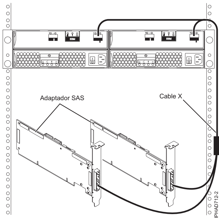
Figura 88. Dos adaptadors SAS RAID a un calaix d'expansió de discs en una configuració HA RAID
