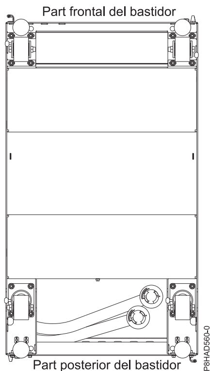
Figura 47. Ubicacions de sortida de tubs de la part inferior (quan es mira des de baix)
