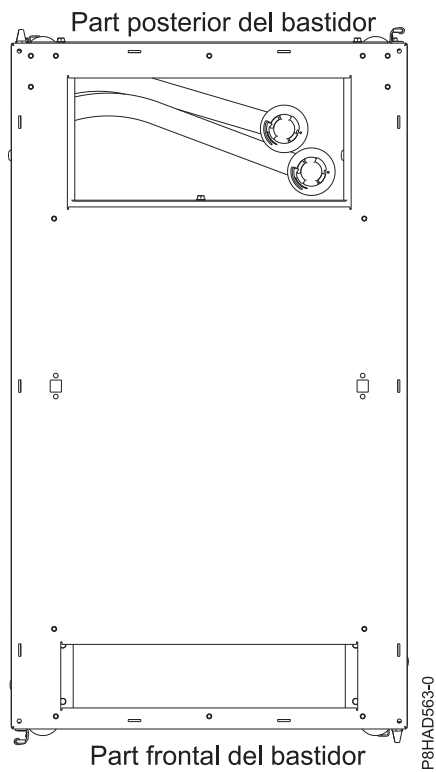
Figura 45. Ubicacions de sortida de tubs de la part superior (quan es mira des de dalt)
