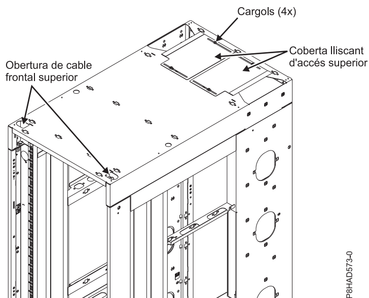
Figura 53. Compartiment superior dels cables
