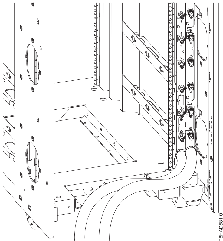
Figura 62. Ubicacions de sortida de tubs de la part inferior
