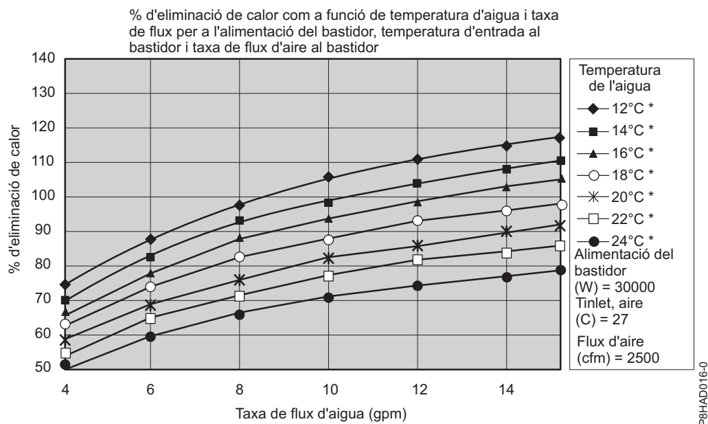
Figura 40. Rendiment habitual de l'intercanviador de calor, 30 kW de càrrega de calor
