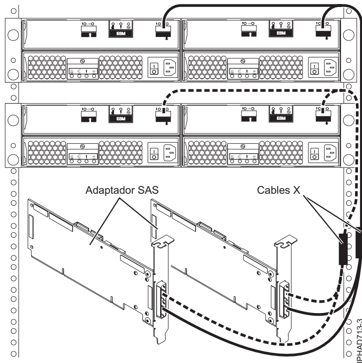
Figura 89. Dos adaptadors SAS RAID a dos calaixos d'expansió de discs en una configuració HA RAID
