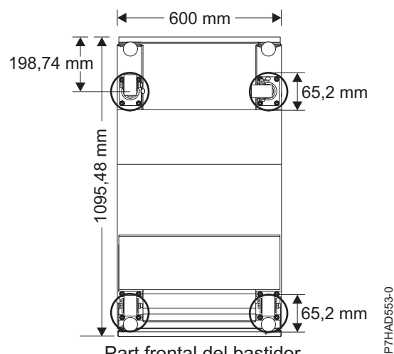
Figura 33. Ubicació de les rodes giratòries
