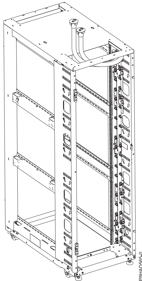
Figura 42. Bastidor i col·lector amb tubs de subministrament i retorn existent a la part superior del bastidor
