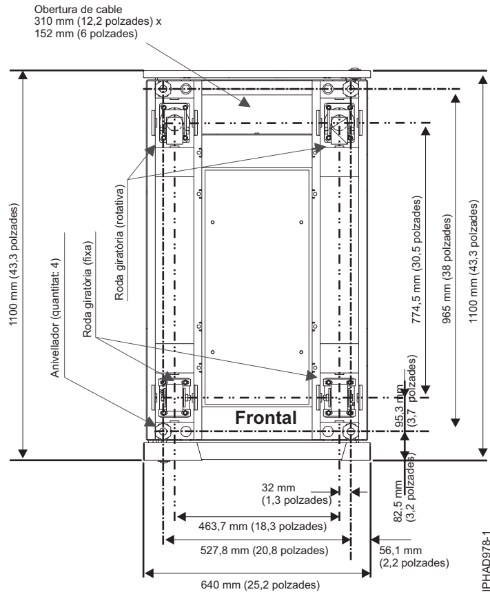
Figura 30. Ubicacions de rodes giratòries i anivelladors
