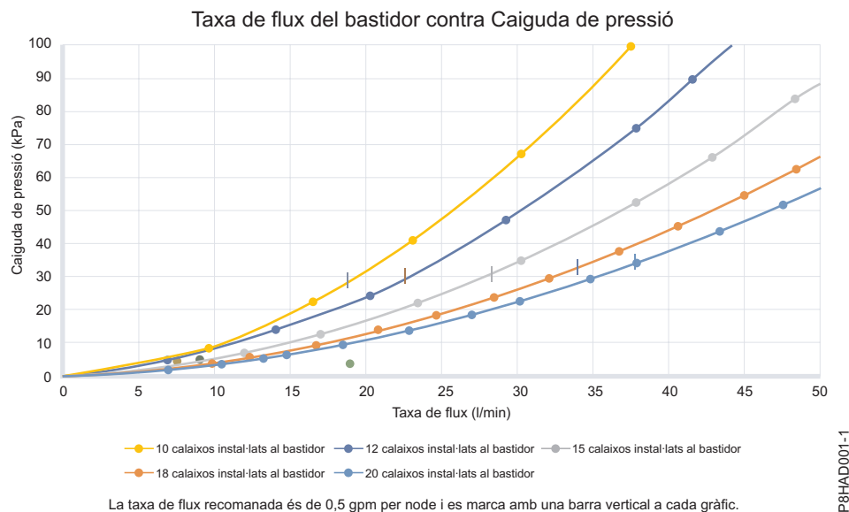
Figura 5. Taxa de flux contra caiguda de pressió (unitats estàndard)
