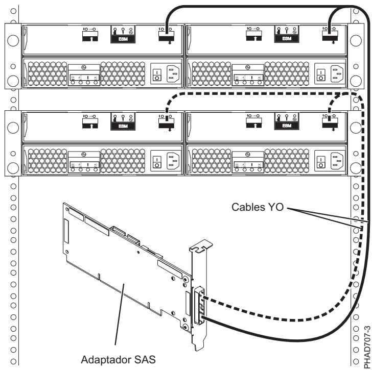
Figura 80. Un adaptador SAS a dos calaixos d'expansió de discs
