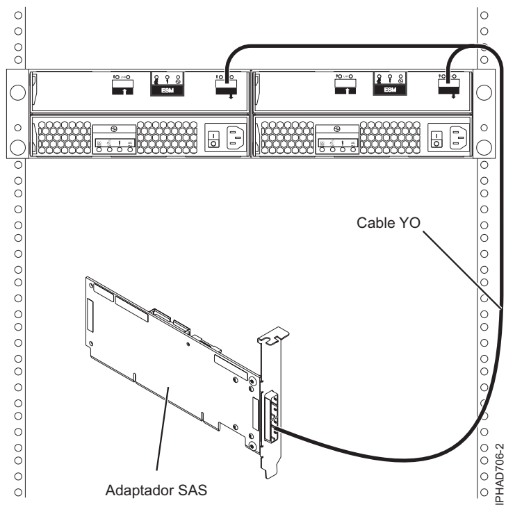
Figura 79. Un adaptador SAS a un calaix d'expansió de discs
