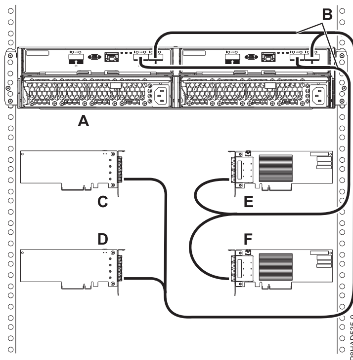
Figura 113. Connexió de mode 4 d'un allotjament 5887 utilitzant cables X a quatre adaptadors PCIe3 SAS únics amb connectors estrets HD.
