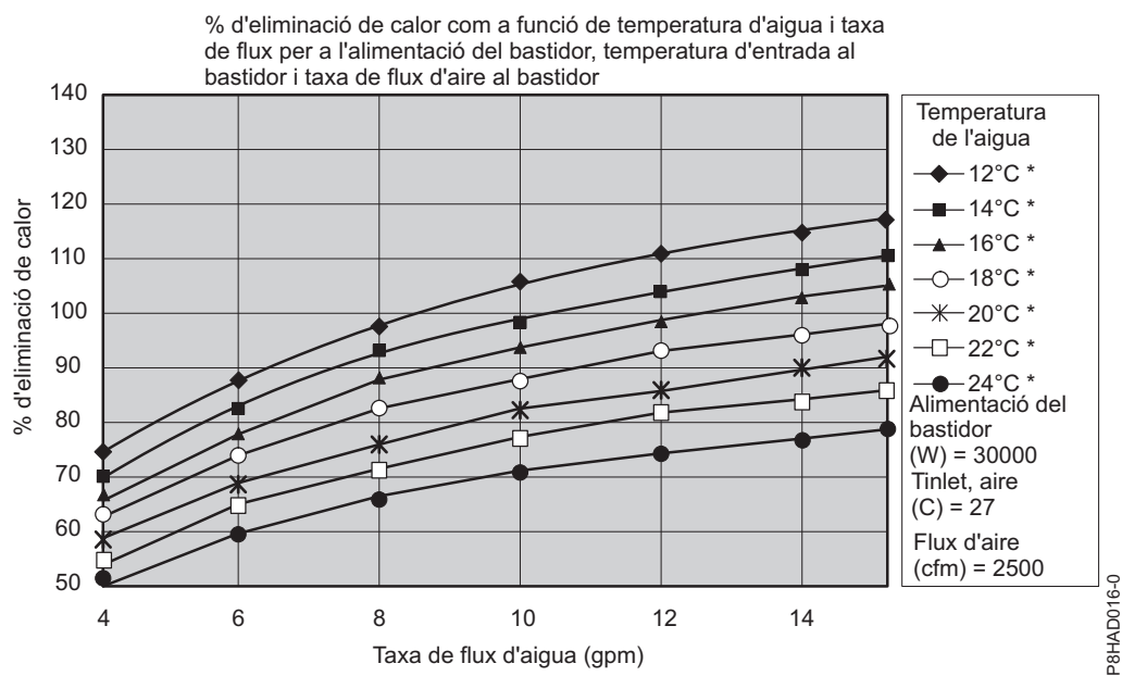
Figura 56. Rendiment habitual de l'intercanviador de calor, 30 kW de càrrega de calor
