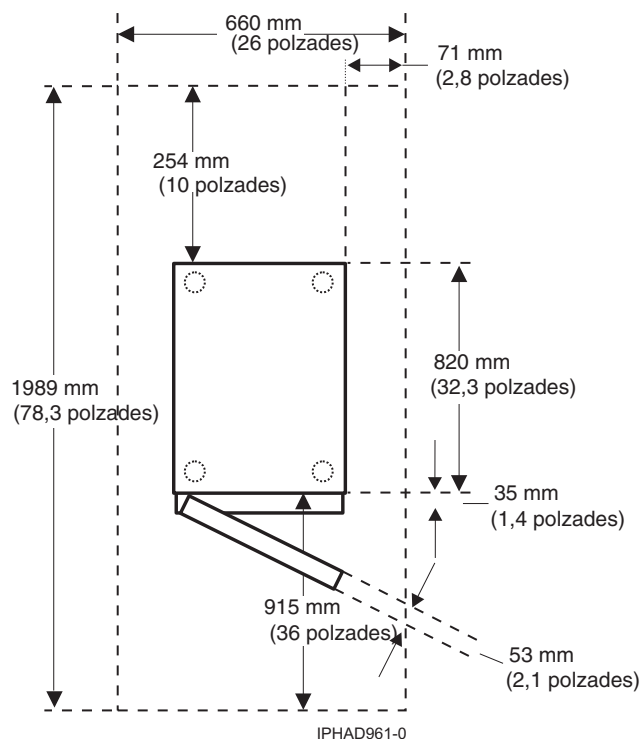
Figura 23. Vista del pla del model 0554 i 7014-S11
