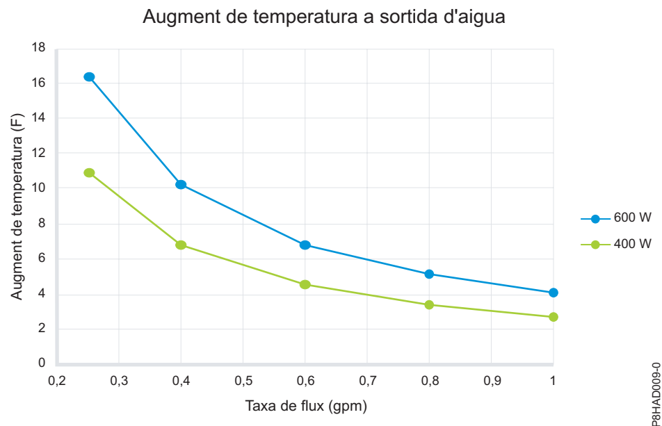
Figura 7. Taxa de flux d'aigua contra subministrament i temperatura (unitats estàndard)
