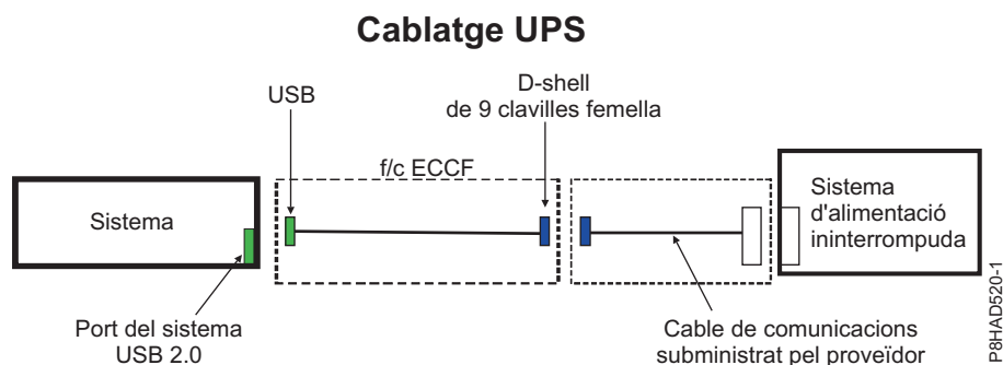
Figura 68. Cablatge UPS per als model 5148-21L, 5148-22L, 8247-21L, 8247-21L, 8247-22L, 8247-42L, 8284-22A, 8286-41A i 8286-42A
