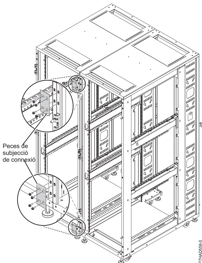
Figura 38. Peces de subjecció de connexió
