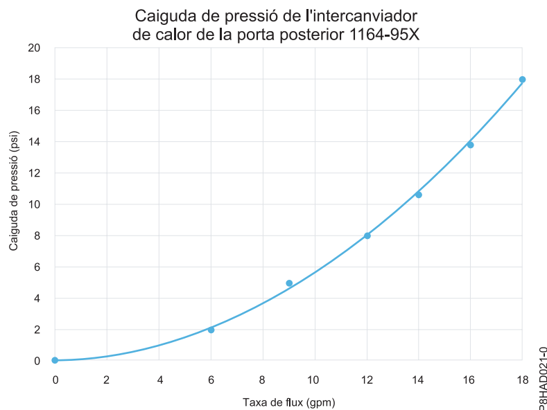
Figura 41. Caiguda de pressió (unitats estàndard)
