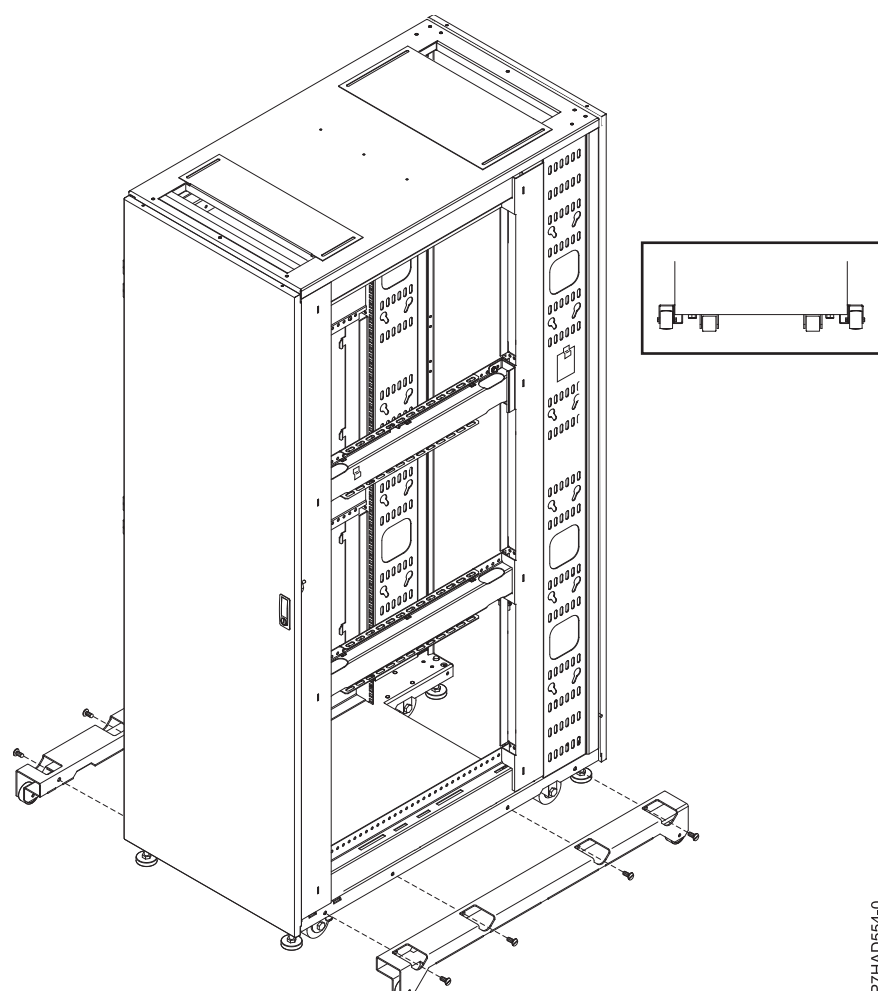
Figura 37. Ubicacions dels estabilitzadors
