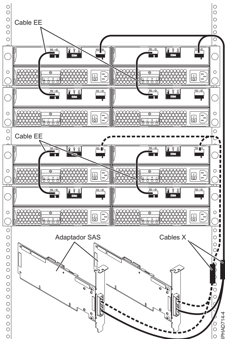
Figura 90. Dos adaptadors SAS RAID a quatre calaixos d'expansió de discs en una configuració HA RAID
