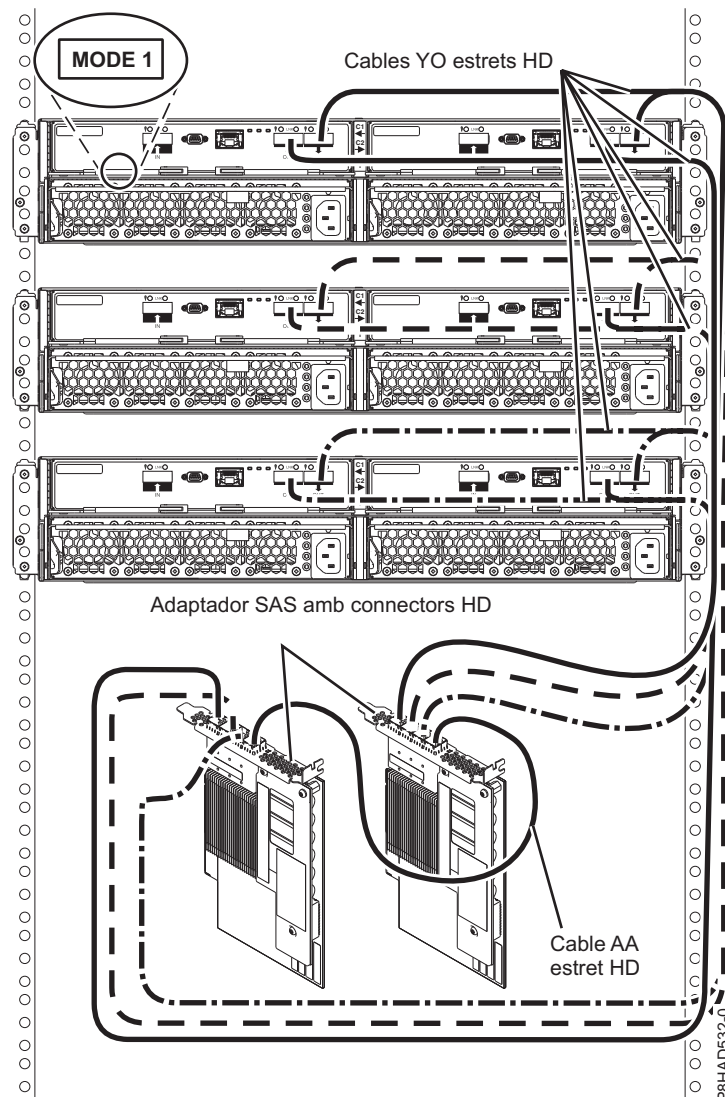
Figura 110. Connexió de mode 1 de tres allotjaments 5887 a dos adaptadors PCIe3 SAS amb connectors estrets HD.
