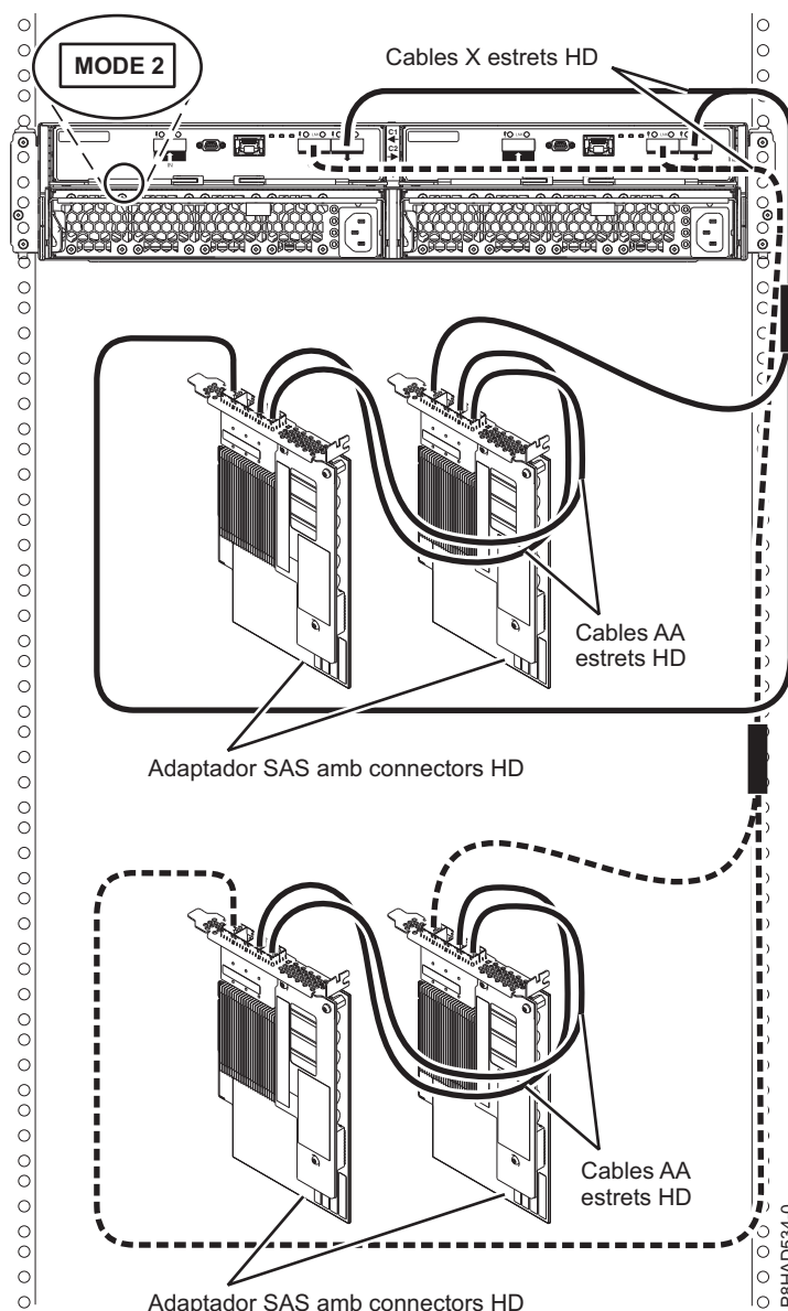
Figura 112. Connexió de mode 2 d'un allotjament 5887 a dos parells d'adaptadors PCIe3 SAS amb connectors estrets HD.
