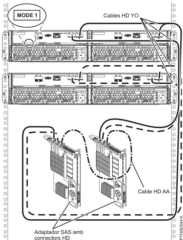
Figura 105. Connexió de mode 1 de dos allotjaments 5887 utilitzant connectors HD a dos adaptadors PCIe2 SAS
