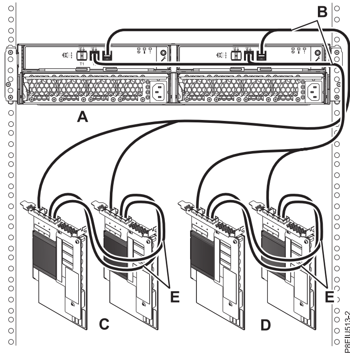
Figura 119. Connexió de mode 2 d'un allotjament d'emmagatzematge ESSL o ESLS utilitzant cables X12 a dos parells d'adaptadors SAS
