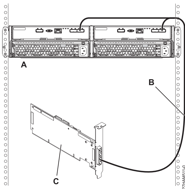
Figura 97. Connexió de mode 1 d'un allotjament 5887 utilitzant un cable YO a un adaptador SAS únic
