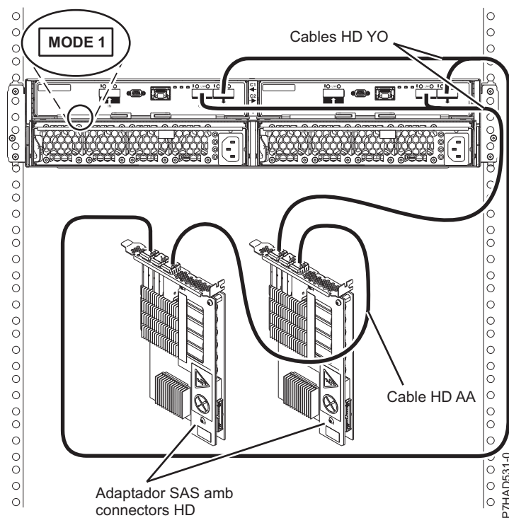
Figura 104. Connexió de mode 1 d'un allotjament 5887 a dos adaptadors PCIe2 SAS amb connectors HD
