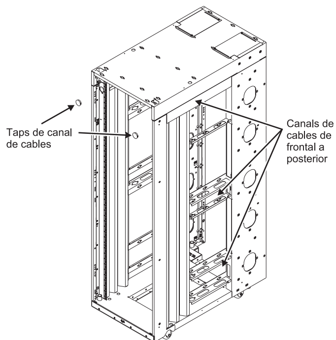
Figura 51. Cablatge al bastidor
