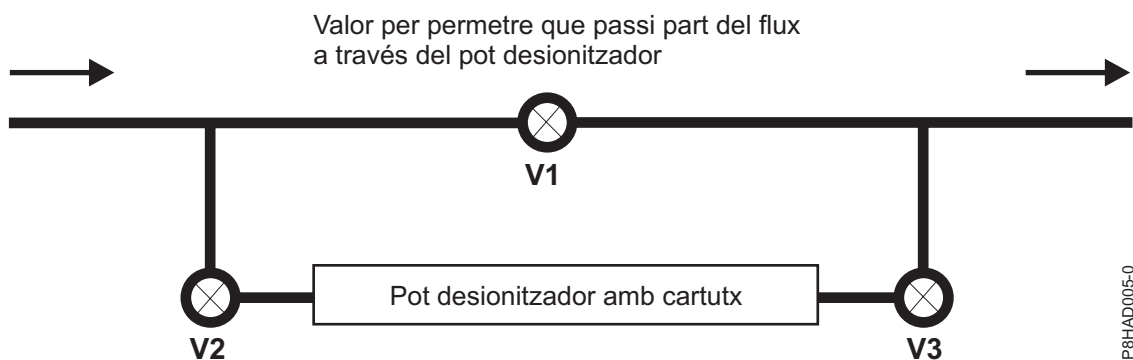
Figura 122. Desionització de l'aigua mitjançant cartutxos de desionització col·locats al bucle de refrigeració
