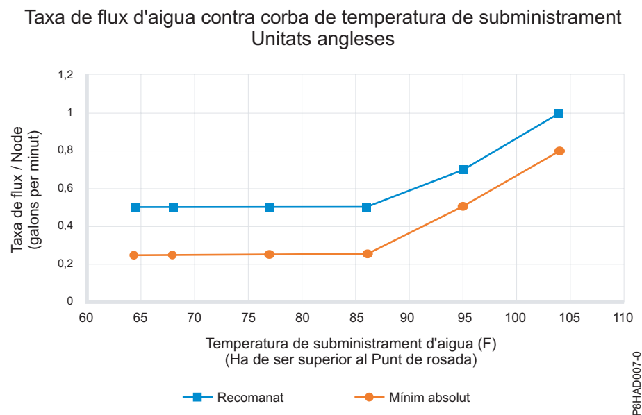
Figura 3. Taxa de flux d'aigua contra subministrament i temperatura (unitats estàndard)
