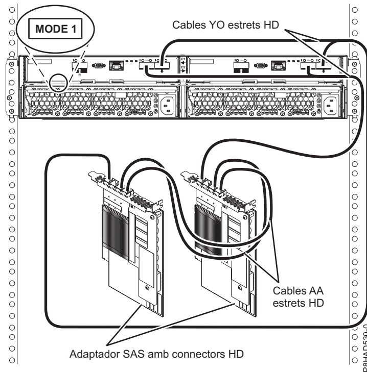
Figura 108. Connexió de mode 1 d'un allotjament 5887 a dos adaptadors PCIe3 SAS amb connectors estrets HD.
