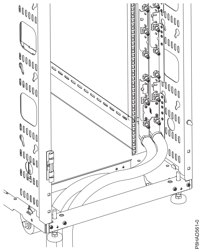
Figura 46. Ubicacions de sortida de tubs de la part inferior
