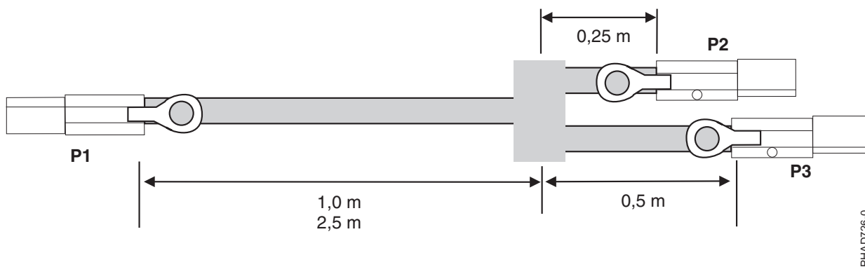
Figura 78. Longituds de cables de conjunt de cable YI SAS extern
