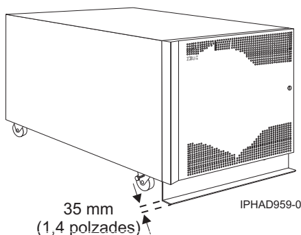
Figura 22. Model 0554 i 7014-S11 amb barra estabilitzadora
