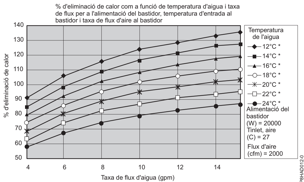
Figura 55. Rendiment habitual de l'intercanviador de calor, 20 kW de càrrega de calor
