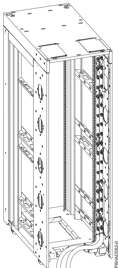
Figura 59. Bastidor i col·lector amb tubs de subministrament i retorn existent a la part inferior del bastidor
