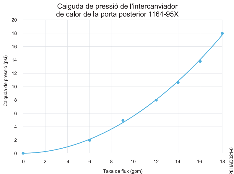
Figura 57. Caiguda de pressió (unitats estàndard)
