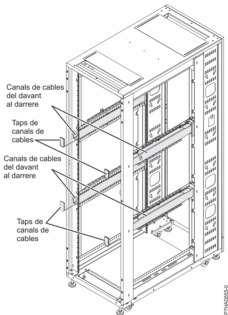
Figura 34. Cablatge al bastidor
