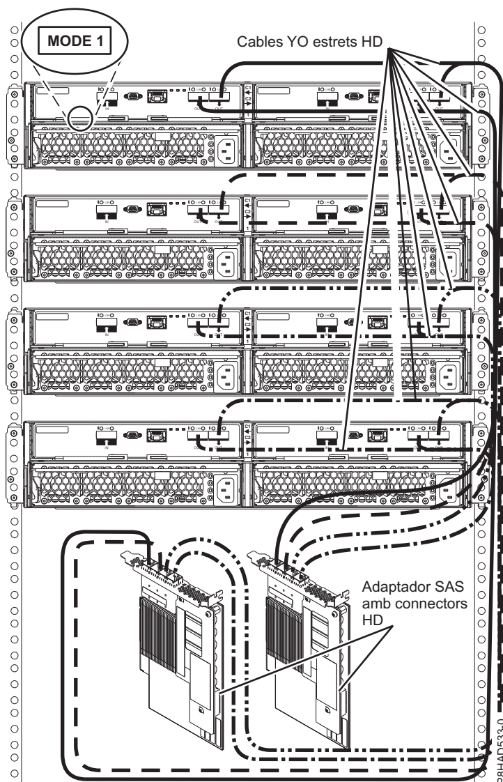
Figura 111. Connexió de mode 1 de quatre allotjaments 5887 a dos adaptadors PCIe3 SAS amb connectors estrets HD.
