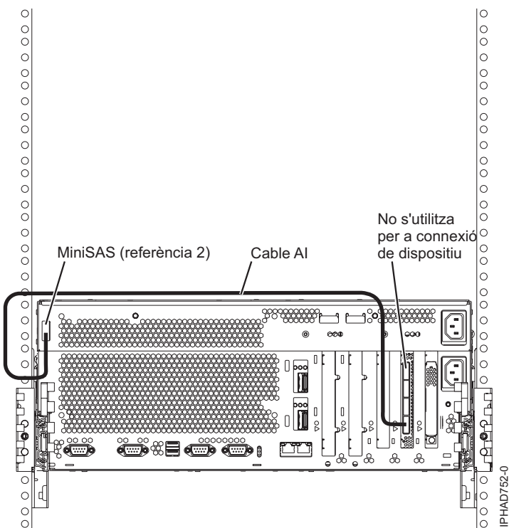
Figura 87. Adaptador FC5904 o FC5908 connectat a calaixos d'expansió de discs
