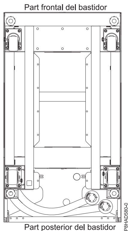
Figura 63. Ubicacions de sortida de tubs de la part inferior (quan es mira des de baix)
