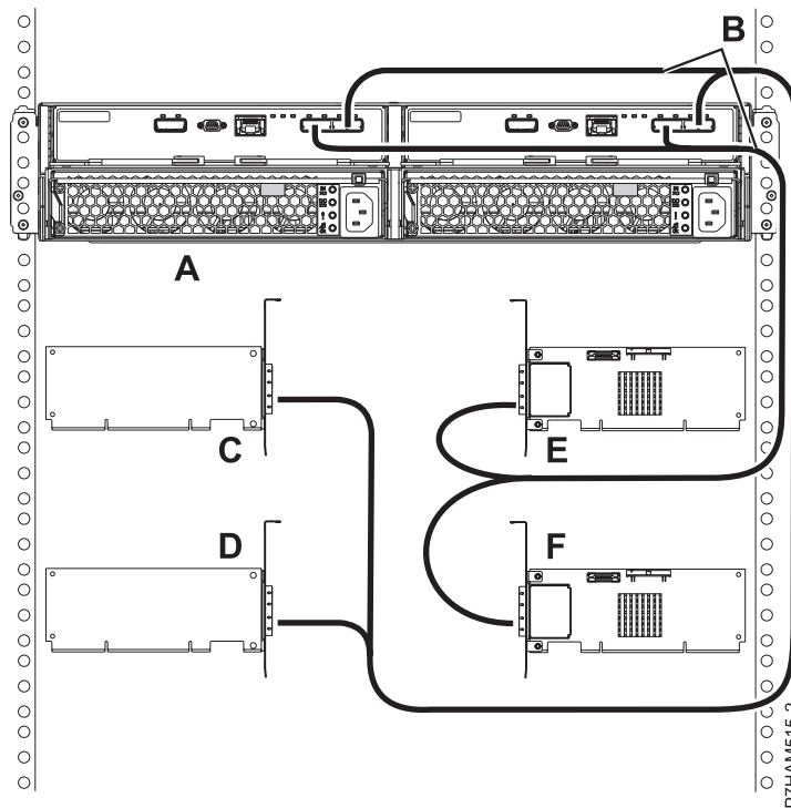
Figura 101. Connexió de mode 4 d'un allotjament 5887 utilitzant cables X a quatre adaptadors SAS únics
