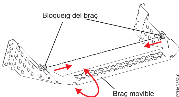
Figura 75. Peça de subjecció portacables
