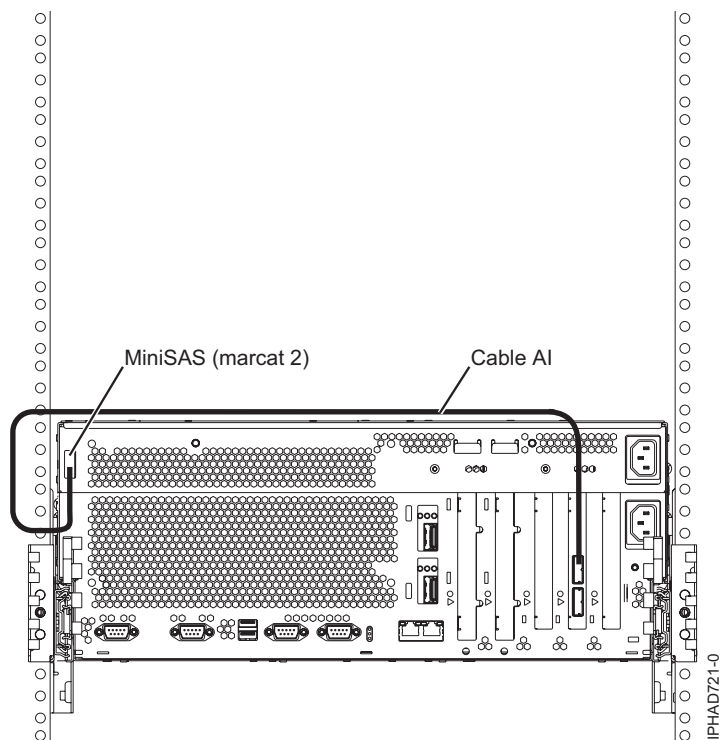
Figura 86. Adaptador SAS a les ranures de disc SAS internes mitjançant el port SAS extern del sistema
