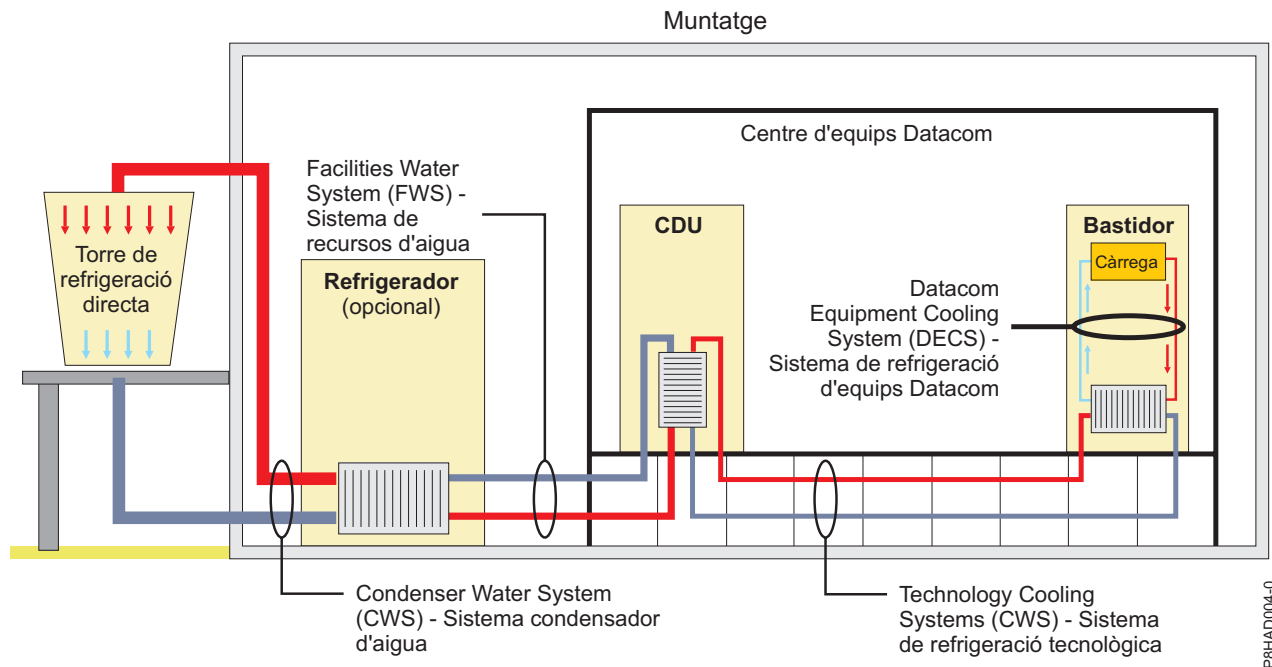
Figura 121. Exemple de sistemes i bucles de refrigeració de líquids en un centre de dades
