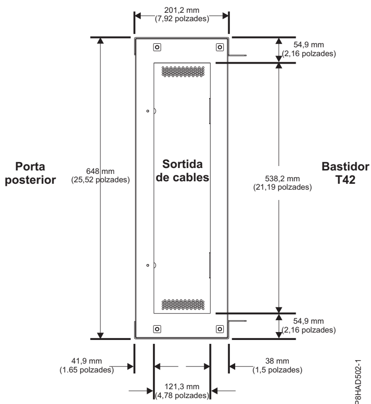
Figura 31. Extensor de bastidor posterior FC ERG0 (vista de dalt a baix)
