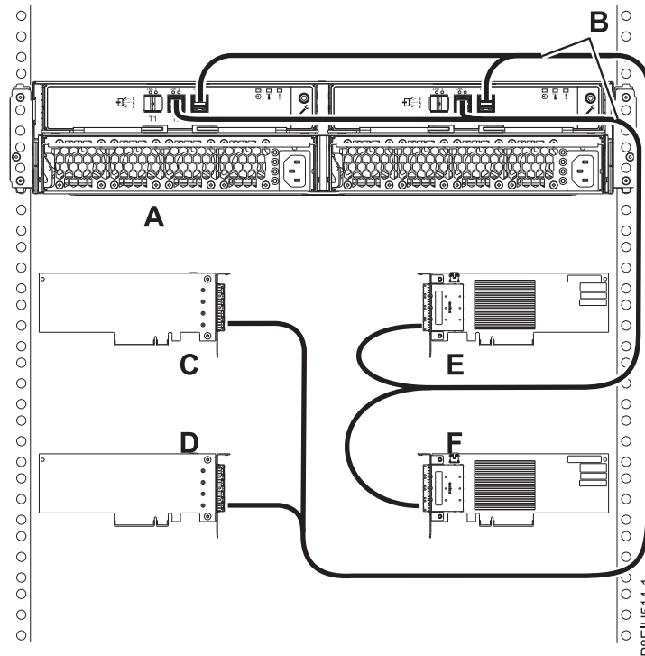
Figura 120. Connexió de mode 4 d'un allotjament d'emmagatzematge ESSL o ESLS utilitzant cables X12 a quatre adaptadors SAS independents
