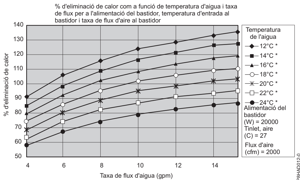
Figura 39. Rendiment habitual de l'intercanviador de calor, 20 kW de càrrega de calor
