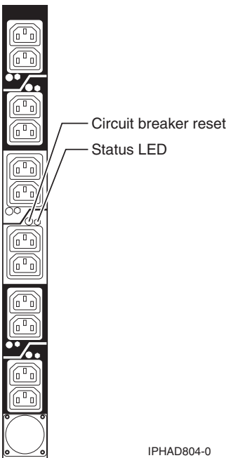
Figura 70. Gràfic de la presa d'alimentació de la PDU
