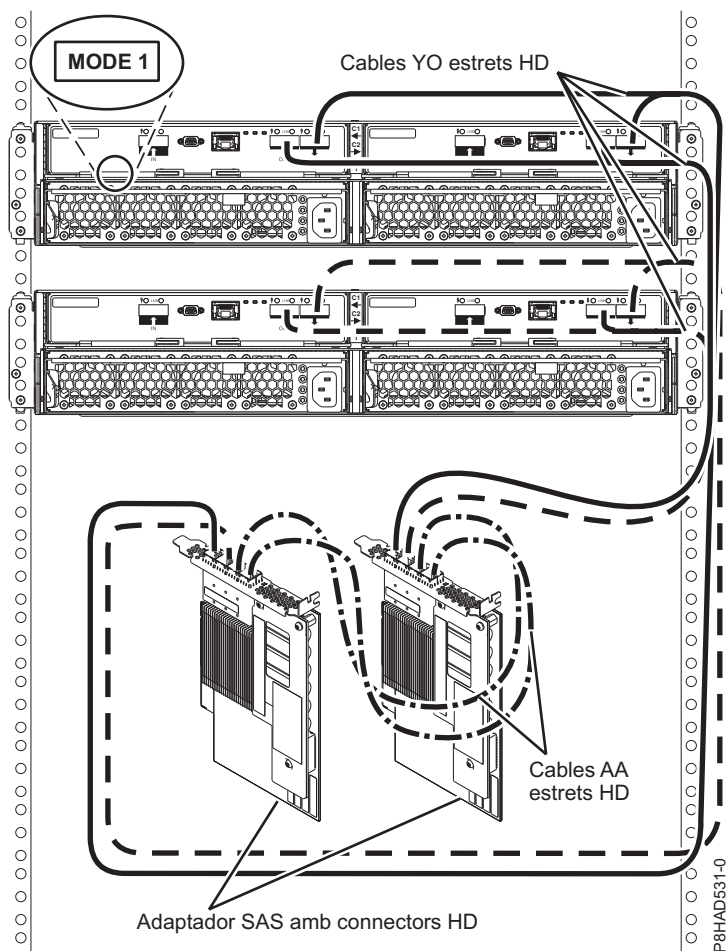
Figura 109. Connexió de mode 1 de dos allotjaments 5887 a dos adaptadors PCIe3 SAS amb connectors estrets HD.
