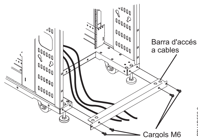
Figura 35. Barra d'accés als cables
