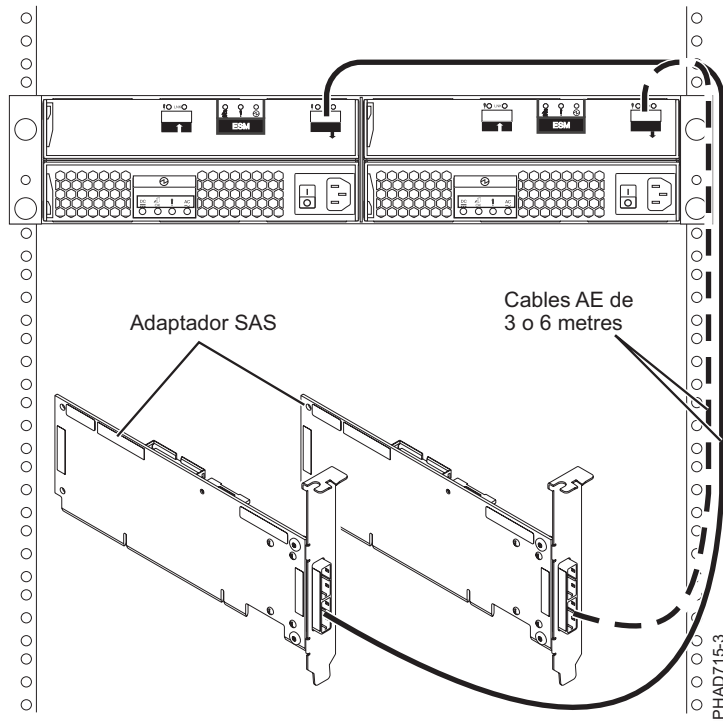
Figura 96. Dos adaptadors SAS RAID a un calaix d'expansió de discos en una configuració HA JBOD
