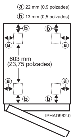
Figura 24. Ubicacions de les rodes giratòries del model 0554 i 7014-S11
