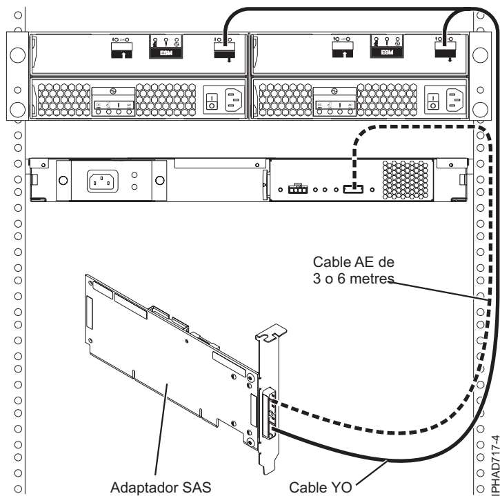
Figura 84. Un adaptador SAS a un calaix d'expansió de discs i a un calaix d'expansió de mitjans
