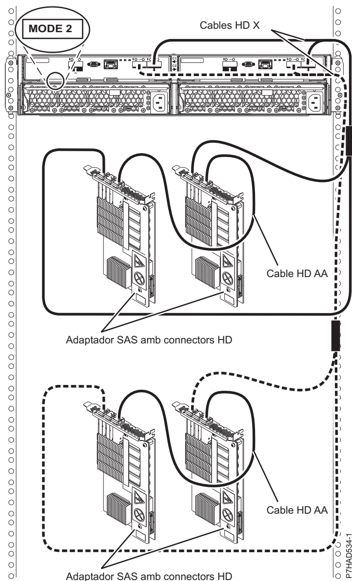
Figura 107. Connexió de mode 2 d'un allotjament 5887 utilitzant connectors HD a dos parells d'adaptadors PCIe2 SAS
