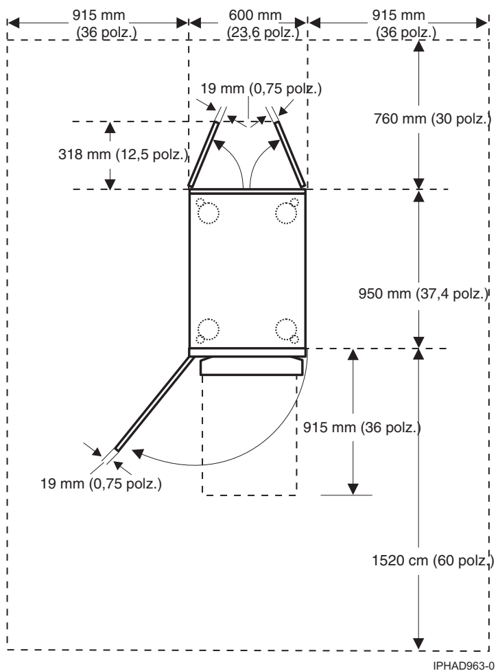
Figura 26. Vista del pla del model 0555 i 7014-S25
