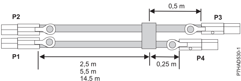
Figura 76. Longituds de cables de conjunt de cable X SAS extern
