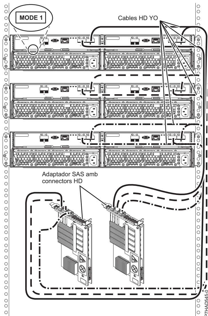
Figura 106. Connexió de mode 1 de tres allotjaments 5887 a dos adaptadors PCIe2 SAS amb connectors HD
