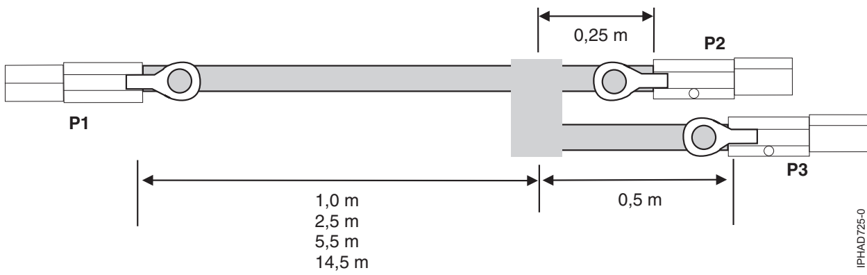
Figura 77. Longituds de cables de conjunt de cable YO SAS extern
