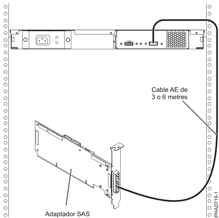
Figura 83. Un adaptador SAS a un calaix d'expansió de mitjans
