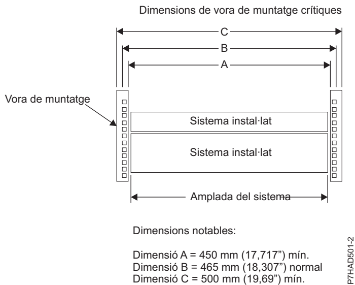
Figura 66. Dimensions de les vores de muntatge de gravetat
