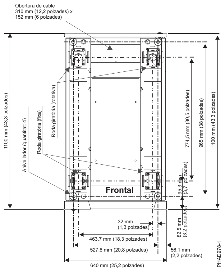
Figura 11. Ubicacions de rodes giratòries i anivelladors
