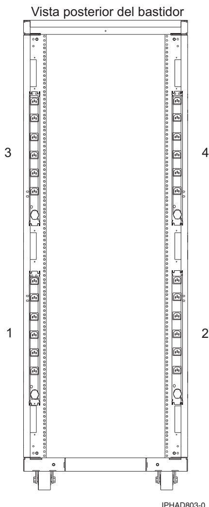
Figura 69. Ubicacions verticals d'unitats de distribució d'alimentació
