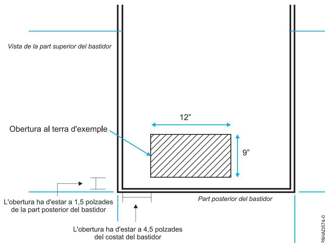
Figura 65. Obertura al terra
