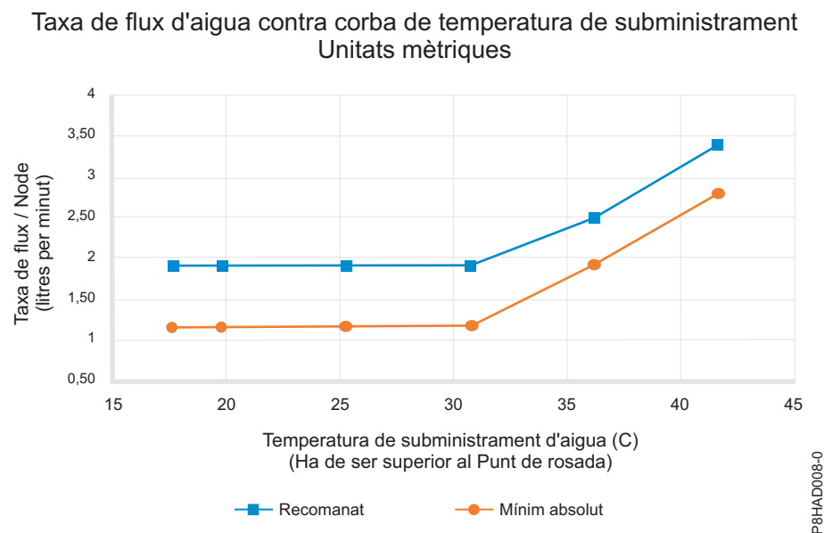
Figura 2. Taxa de flux d'aigua contra subministrament i temperatura (unitats mètriques)
