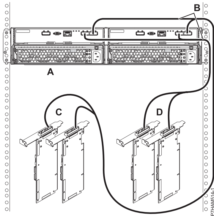
Figura 100. Connexió de mode 2 d'un allotjament 5887 utilitzant cables X a dos parells d'adaptadors SAS
