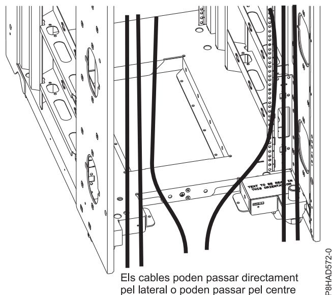
Figura 52. Cablatge per sota del terra
