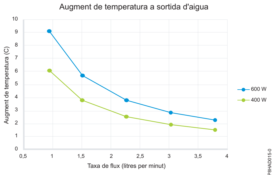
Figura 6. Taxa de flux d'aigua contra subministrament i temperatura (unitats mètriques)
