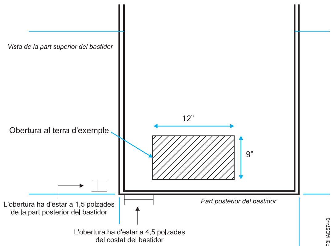
Figura 50. Obertura al terra
