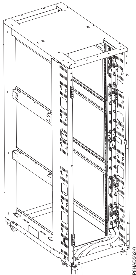
Figura 43. Bastidor i col·lector amb tubs de subministrament i retorn existent a la part inferior del bastidor
