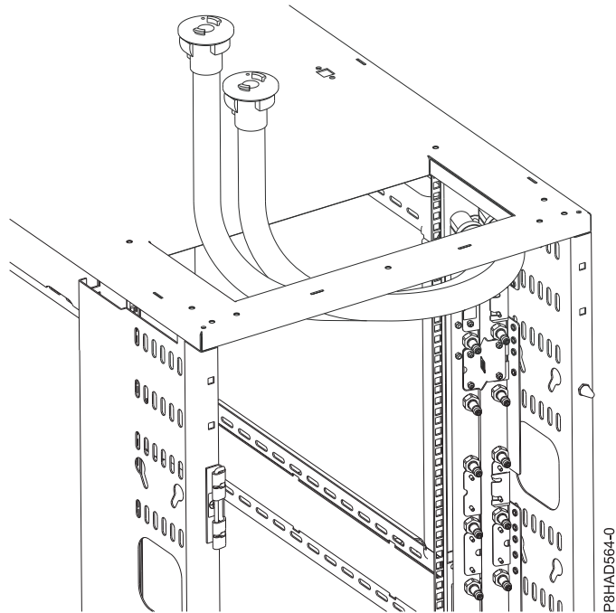
Figura 44. Ubicacions de sortida de tubs de la part superior
