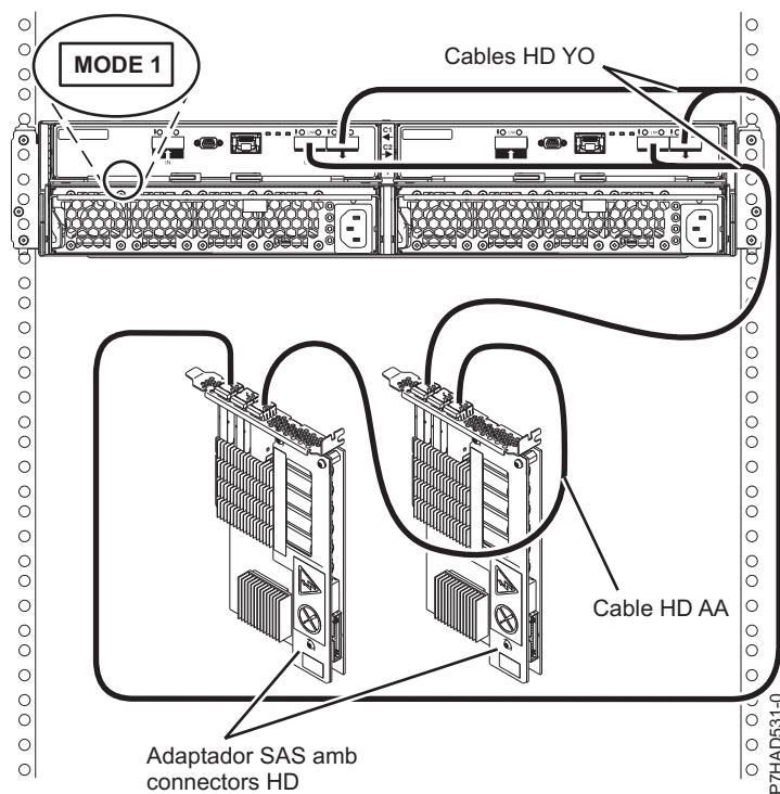
Figura 81. Connexió de mode 1 d'un allotjament 5887 a dos adaptadors PCIe2 SAS amb connectors HD
