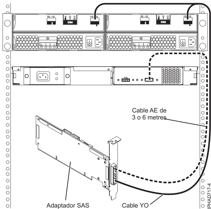
Figura 61. Un adaptador SAS a un calaix d'expansió de discs i a un calaix d'expansió de mitjans
