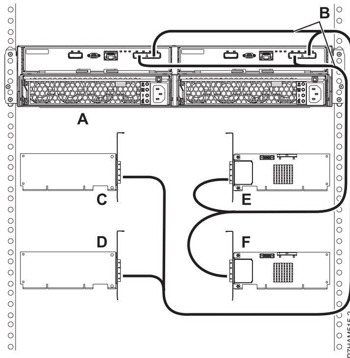
Figura 78. Connexió de mode 4 d'un allotjament 5887 utilitzant cables X a quatre adaptadors SAS únics
