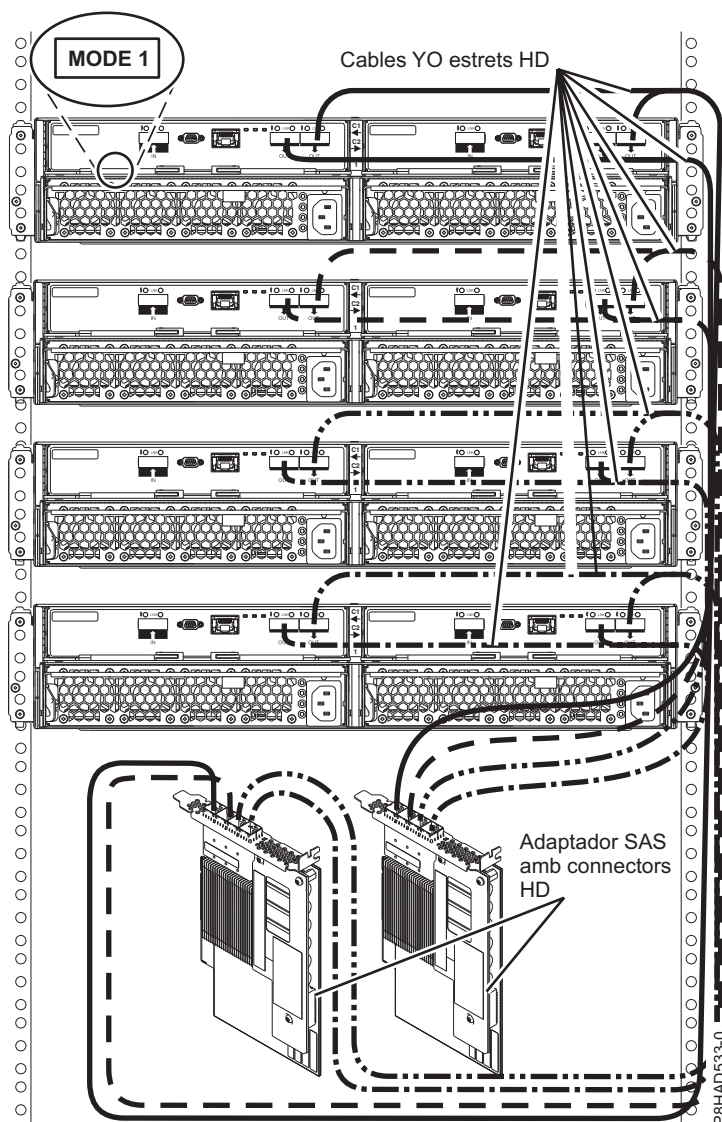
Figura 88. Connexió de mode 1 de quatre allotjaments 5887 a dos adaptadors PCIe3 SAS amb connectors estrets HD.
