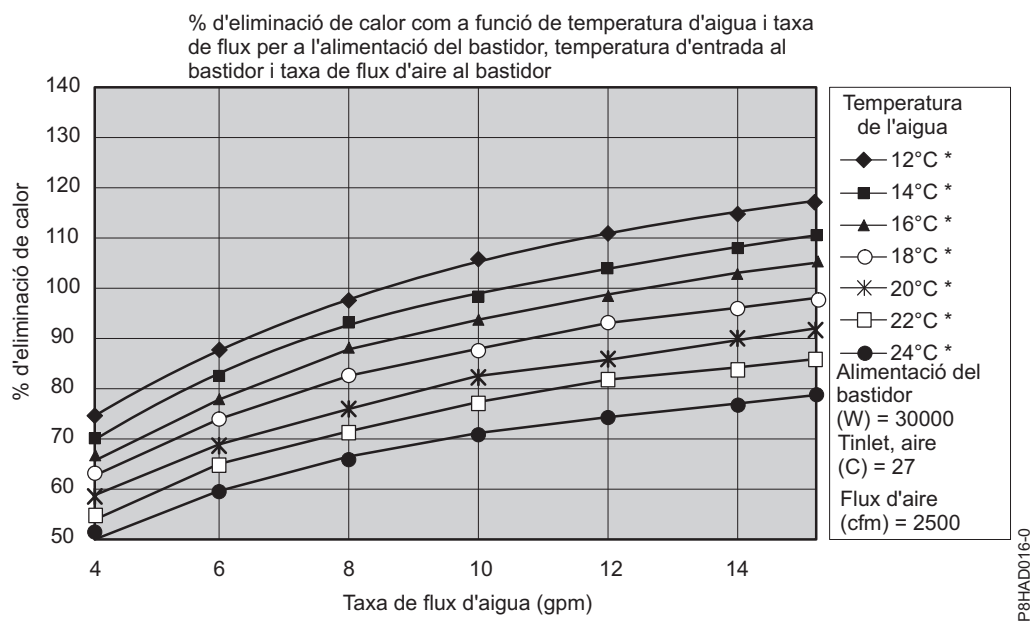
Figura 41. Rendiment habitual de l'intercanviador de calor, 30 kW de càrrega de calor
