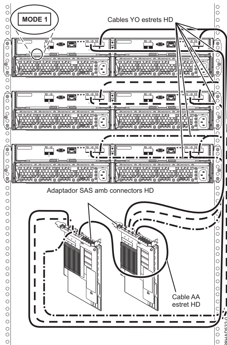
Figura 87. Connexió de mode 1 de tres allotjaments 5887 a dos adaptadors PCIe3 SAS amb connectors estrets HD.
