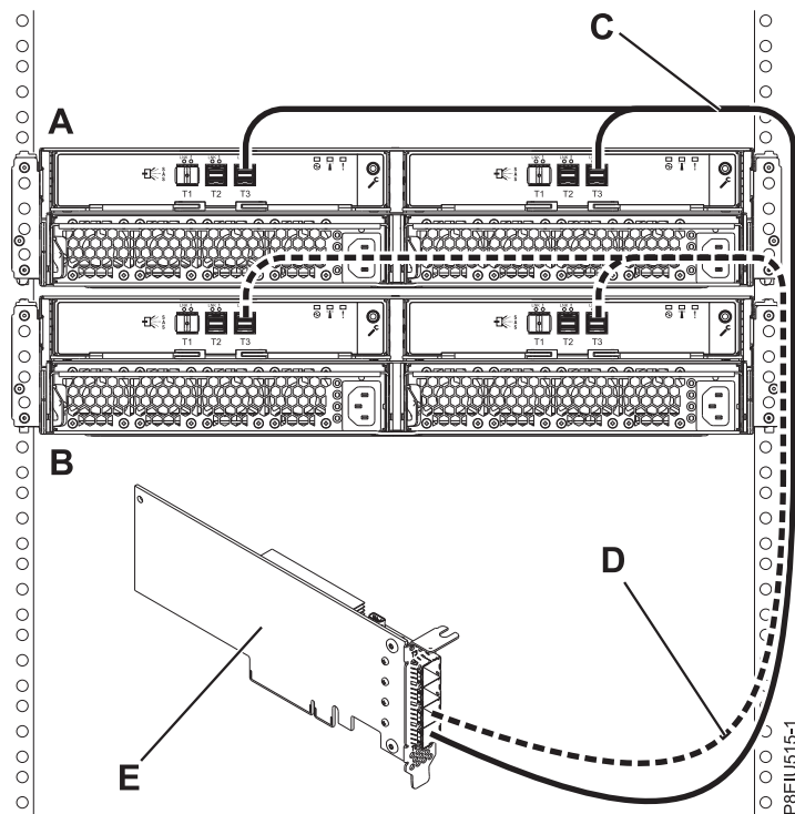
Figura 92. Connexió de mode 1 de dos allotjaments d'emmagatzematge ESLL o ESLS utilitzant cables YO12 en un adaptador SAS individual
