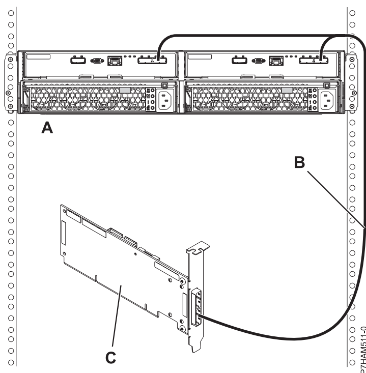
Figura 74. Connexió de mode 1 d'un allotjament 5887 utilitzant un cable YO a un adaptador SAS únic
