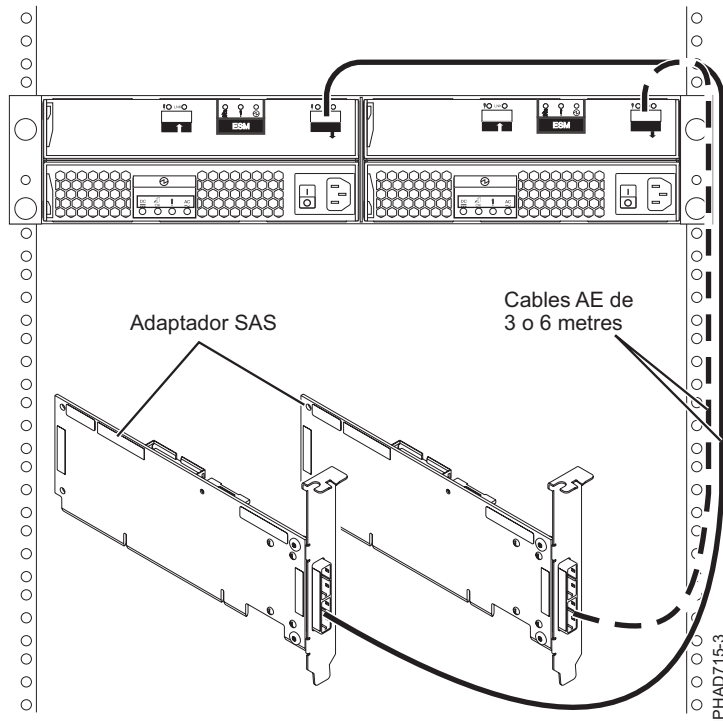
Figura 73. Dos adaptadors SAS RAID a un calaix d'expansió de discos en una configuració HA JBOD
