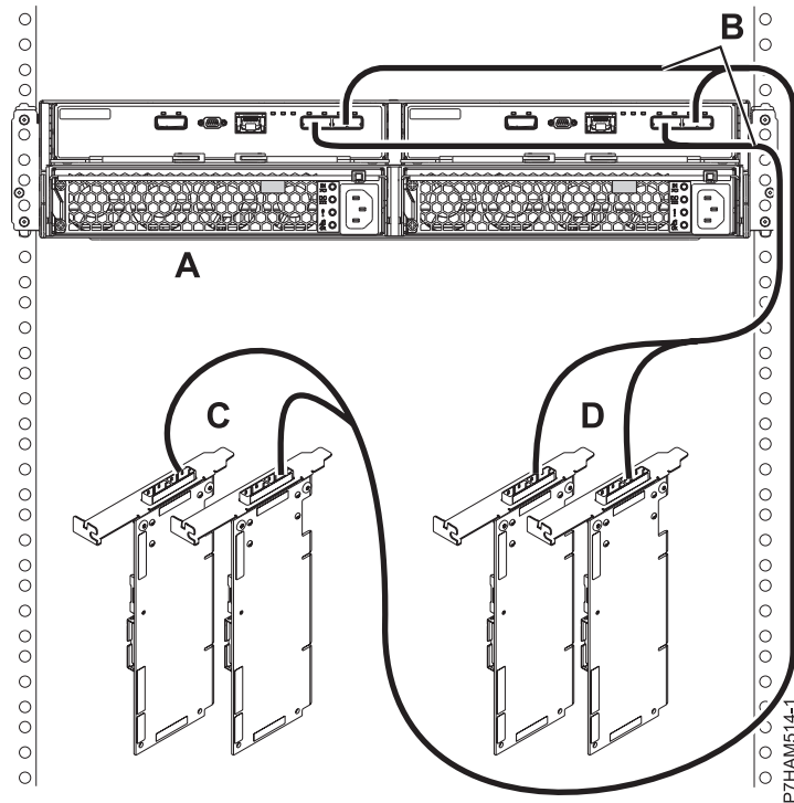
Figura 77. Connexió de mode 2 d'un allotjament 5887 utilitzant cables X a dos parells d'adaptadors SAS
