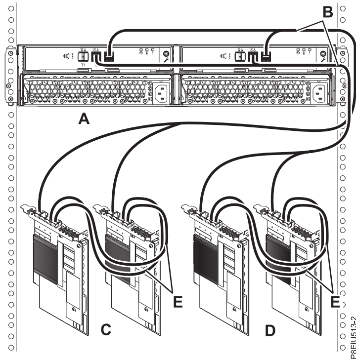
Figura 96. Connexió de mode 2 d'un allotjament d'emmagatzematge ESLL o ESLS utilitzant cables X12 a dos parells d'adaptadors SAS
