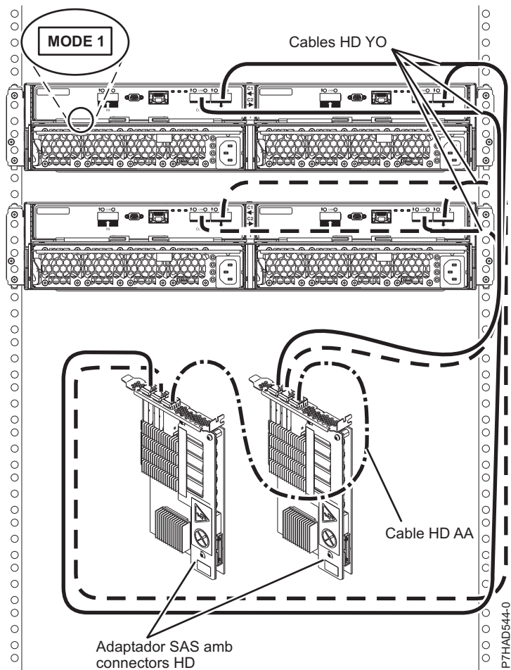
Figura 82. Connexió de mode 1 de dos allotjaments 5887 utilitzant connectors HD a dos adaptadors PCIe2 SAS
