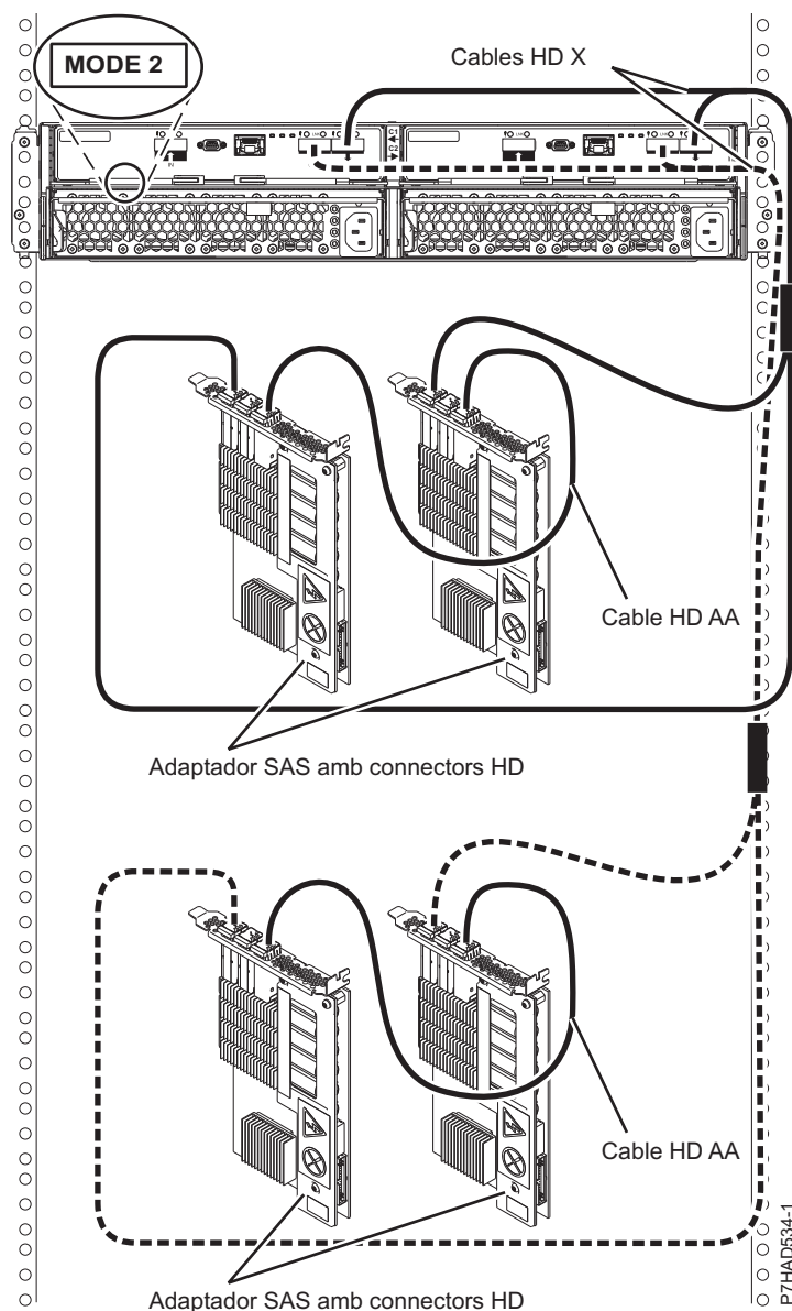
Figura 84. Connexió de mode 2 d'un allotjament 5887 utilitzant connectors HD a dos parells d'adaptadors PCIe2 SAS
