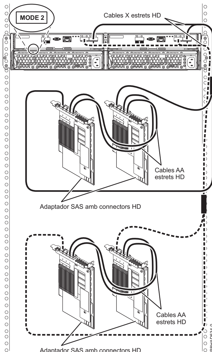
Figura 89. Connexió de mode 2 d'un allotjament 5887 a dos parells d'adaptadors PCIe3 SAS amb connectors estrets HD.
