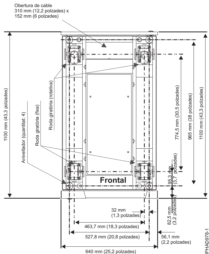
Figura 4. Ubicacions de rodes giratòries i anivelladors
