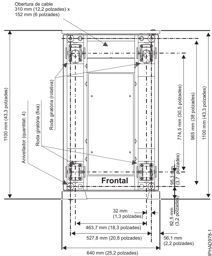
Figura 23. Ubicacions de rodes giratòries i anivelladors
