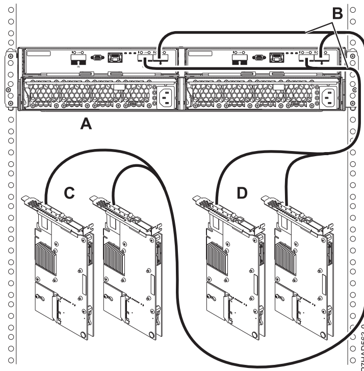
Figura 80. Connexió de dos parells d'adaptadors FC 5805 o FC 5903 a un allotjament 5887 a través del mode 2
