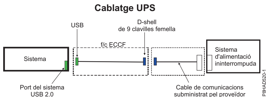
Figura 45. Cablatge UPS per als model 5148-21L, 5148-22L, 8247-21L, 8247-21L, 8247-22L, 8247-42L, 8284-22A, 8286-41A i 8286-42A
