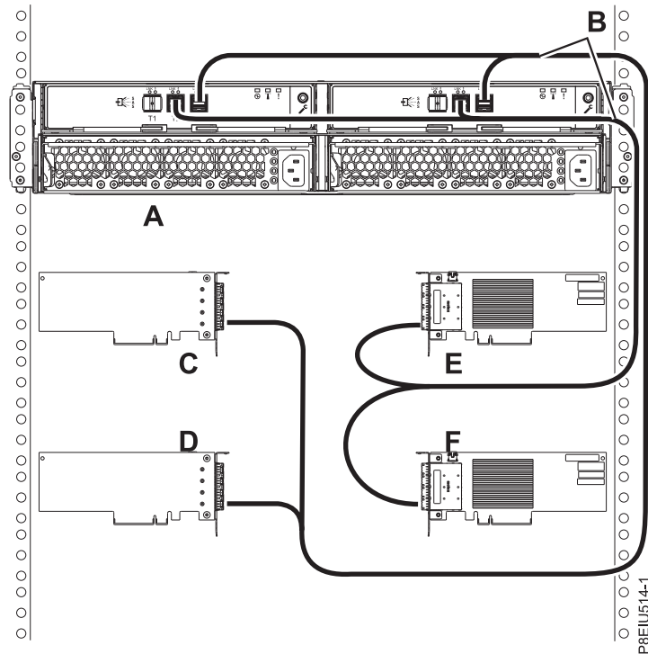
Figura 97. Connexió de mode 4 d'un allotjament d'emmagatzematge ESLL o ESLS utilitzant cables X12 a quatre adaptadors SAS independents
