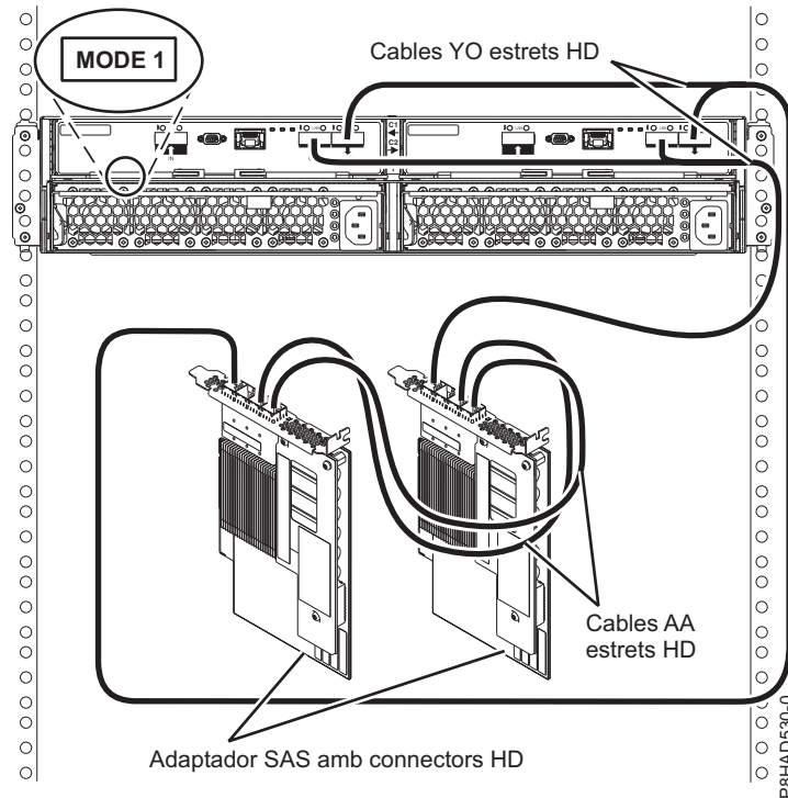
Figura 85. Connexió de mode 1 d'un allotjament 5887 a dos adaptadors PCIe3 SAS amb connectors estrets HD.
