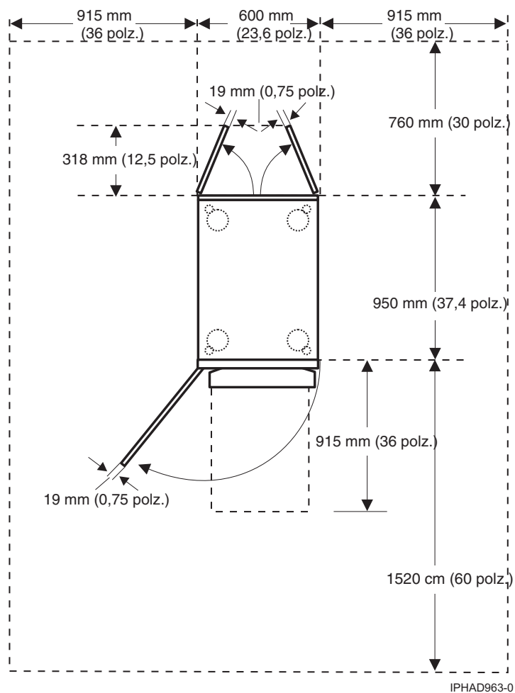
Figura 19. Vista del pla del model 0555 i 7014-S25
