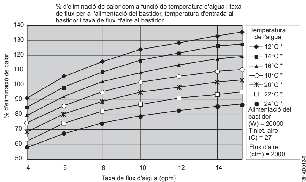
Figura 40. Rendiment habitual de l'intercanviador de calor, 20 kW de càrrega de calor
