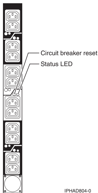
Figura 47. Gràfic de la presa d'alimentació de la PDU
