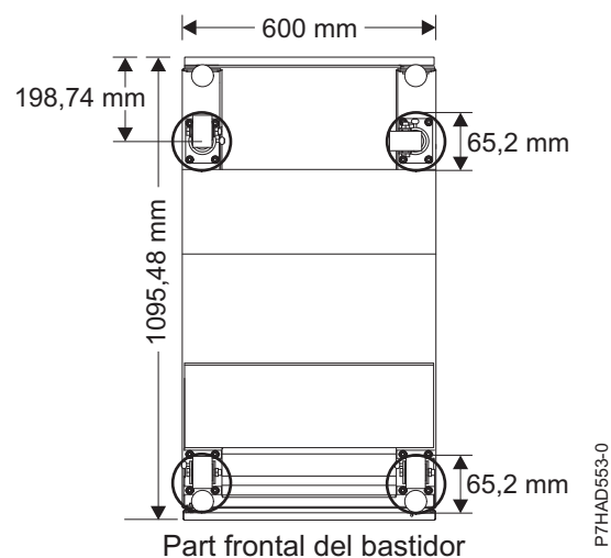
Figura 26. Ubicació de les rodes giratòries
