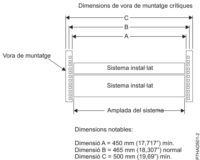
Figura 43. Dimensions de les vores de muntatge de gravetat
