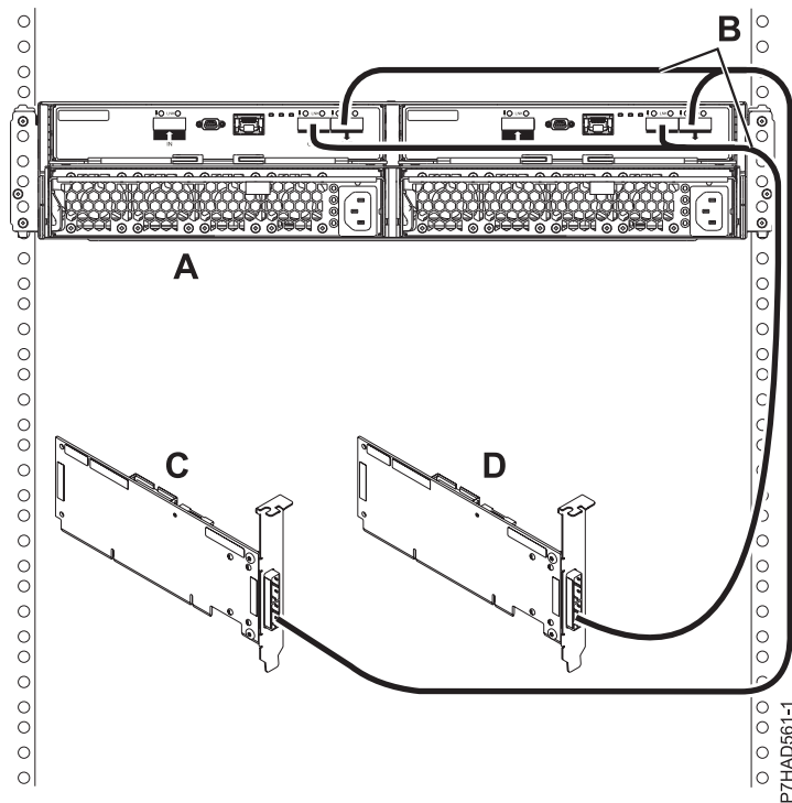
Figura 76. Connexió de mode 2 d'un allotjament 5887 utilitzant cables YO a dos adaptadors SAS duals
