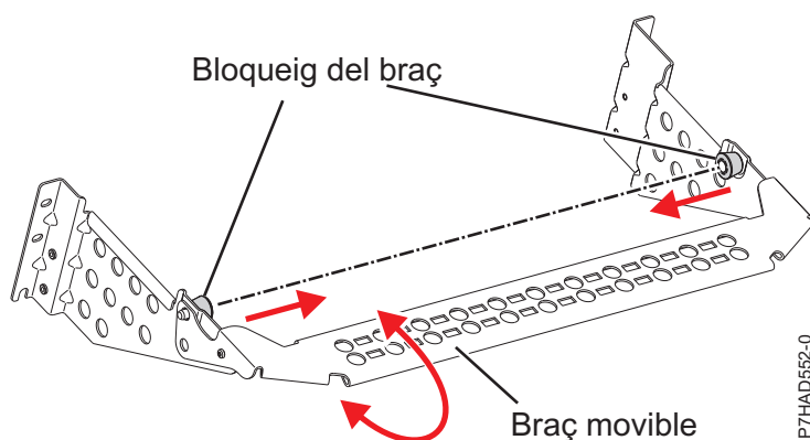
Figura 52. Peça de subjecció portacables
