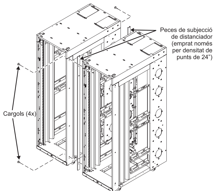
Figura 39. Connexió de diversos bastidors
