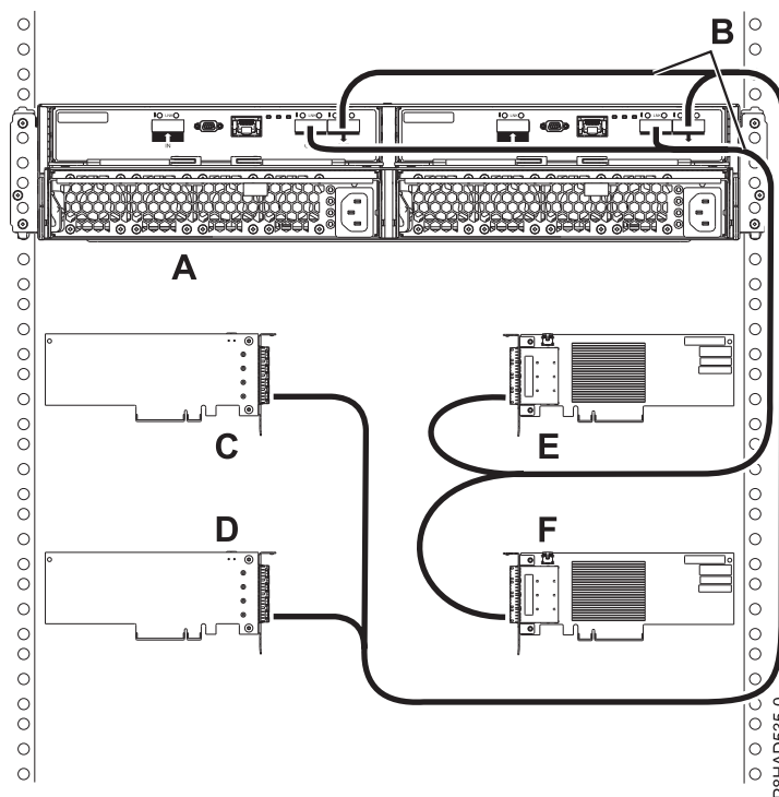
Figura 90. Connexió de mode 4 d'un allotjament 5887 utilitzant cables X a quatre adaptadors PCIe3 SAS únics amb connectors estrets HD.
