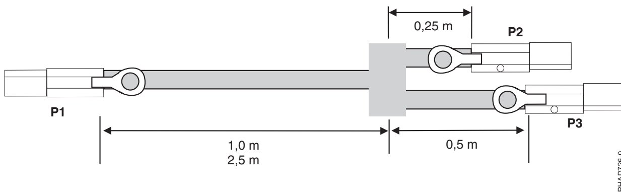
Figura 55. Longituds de cables de conjunt de cable YI SAS extern
