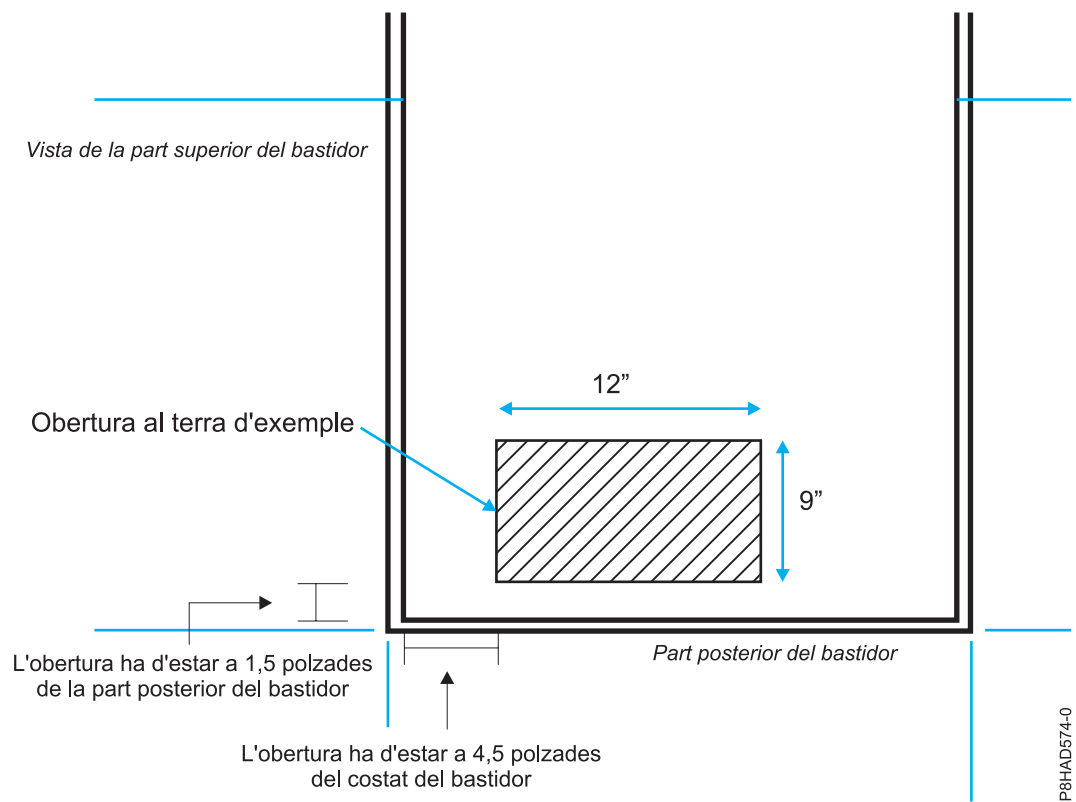
Figura 35. Obertura al terra
