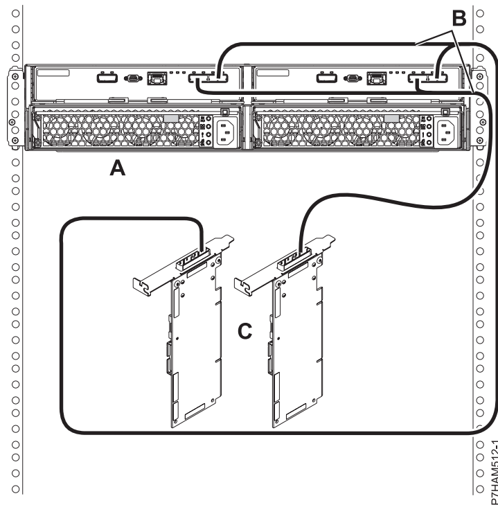
Figura 79. Connexió de mode 1 d'un allotjament 5887 utilitzant cables YO a adaptadors SAS duals
