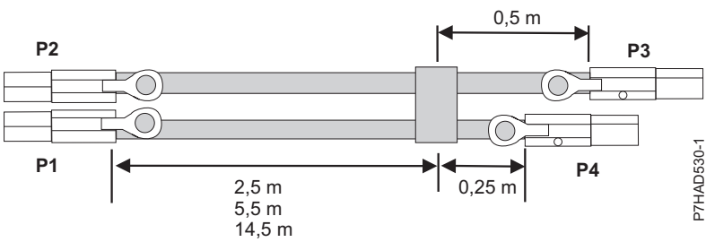
Figura 53. Longituds de cables de conjunt de cable X SAS extern
