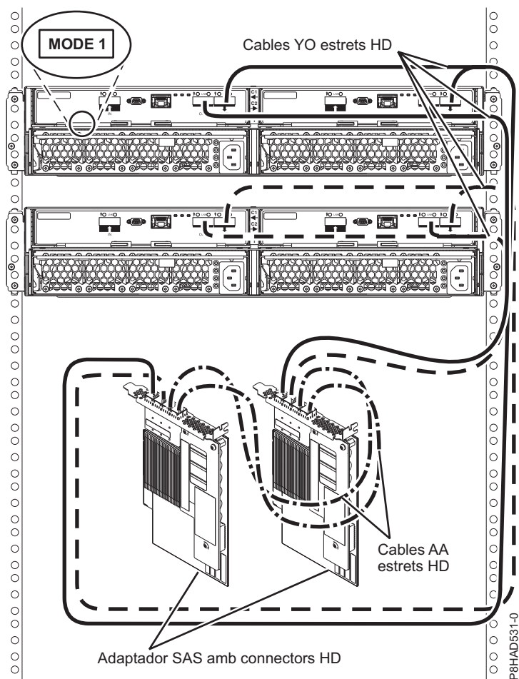
Figura 86. Connexió de mode 1 de dos allotjaments 5887 a dos adaptadors PCIe3 SAS amb connectors estrets HD.
